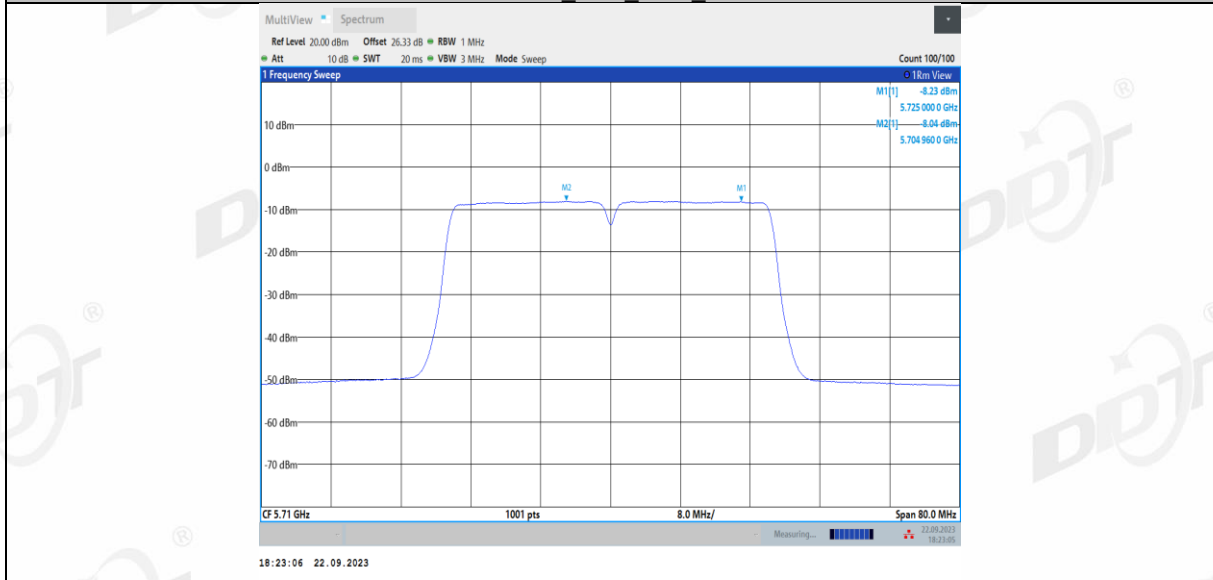
11N40MIMO Ant1 5710 UNII-3
