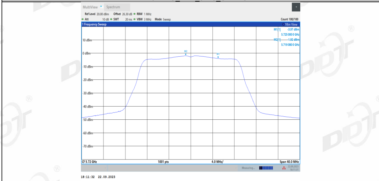
11N20MIMO Ant1 5720 UNII-3
