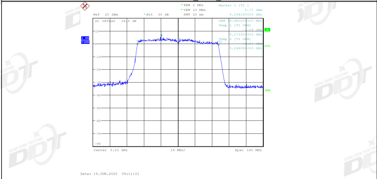
11AC80MIMO_Ant2_5210
