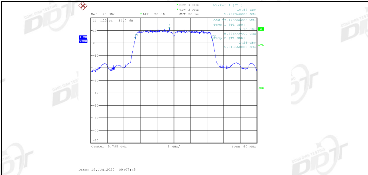
11AC40MIMO_Ant2_5795
