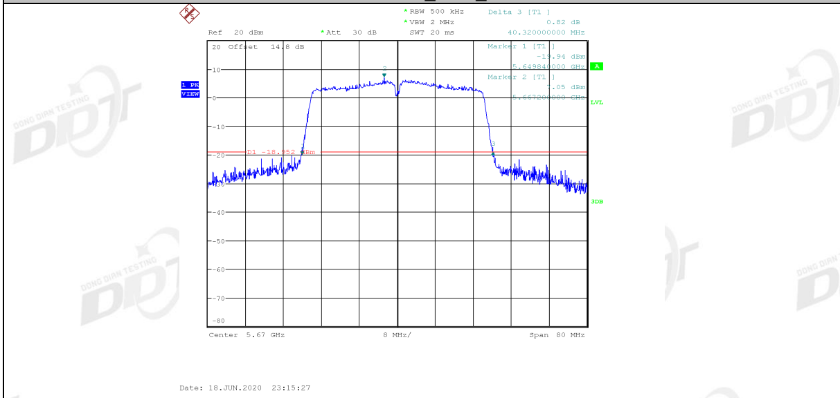
11N40MIMO_Ant2_5670
