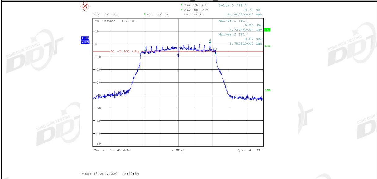
11N20MIMO_Ant2_5745
