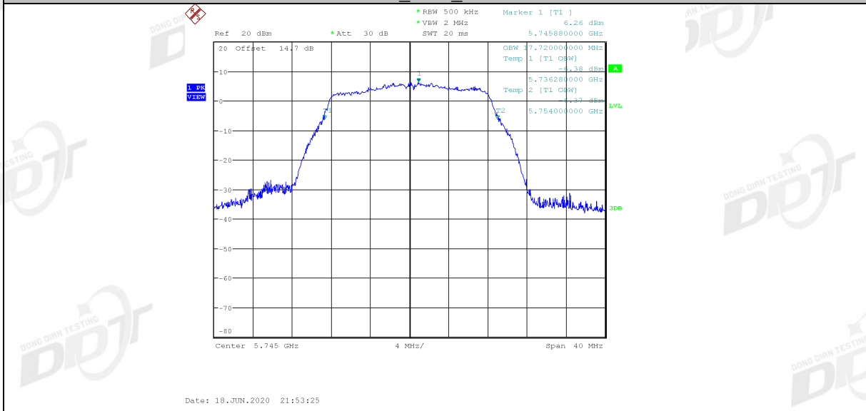
11A_Ant2_5745
