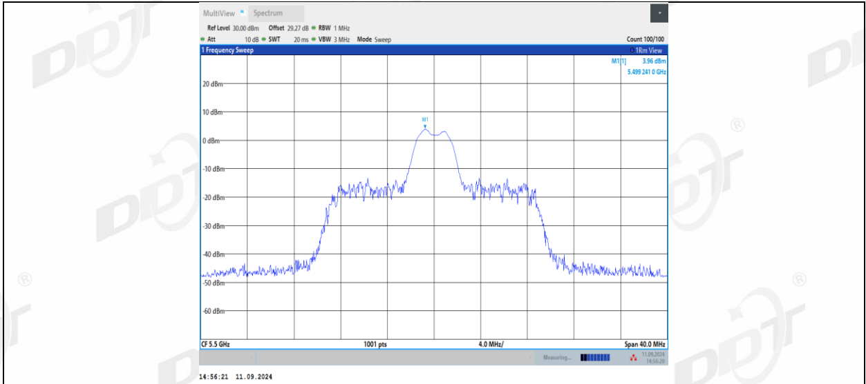
11AX20MIMO_Ant1_5500_26Tone_RU8
