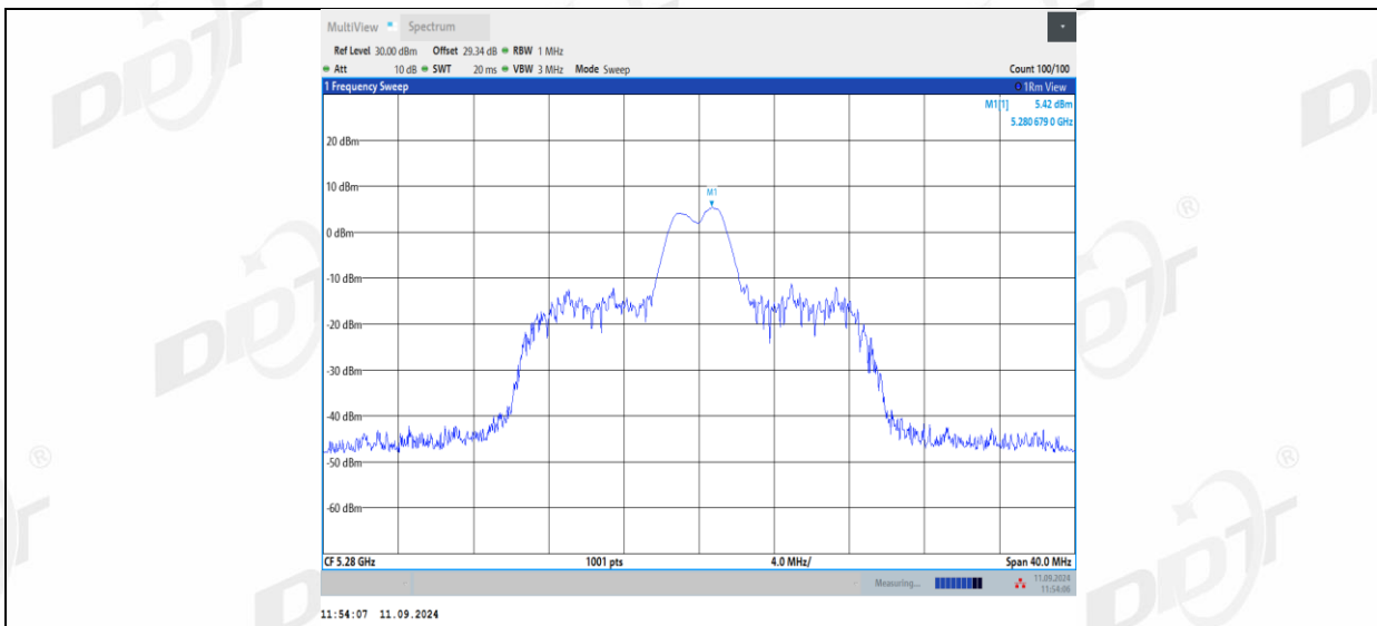
11AX20MIMO_Ant2_5280_26Tone_RU8
