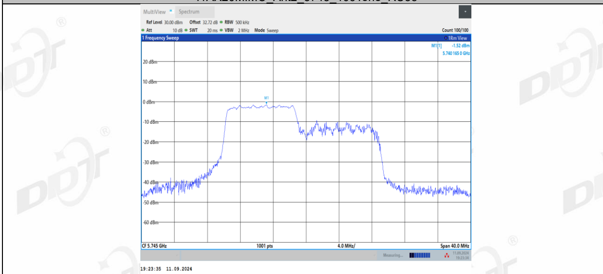
11AX20MIMO_Ant2_5745_106Tone_RU54
