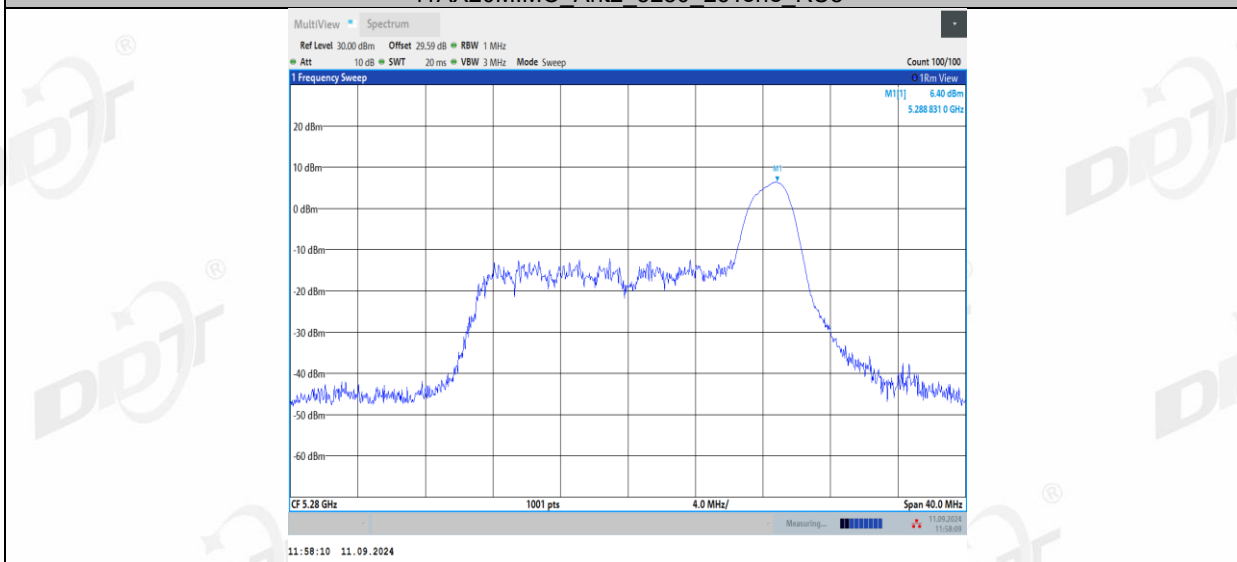
11AX20MIMO_Ant2_5280_52Tone_RU37
