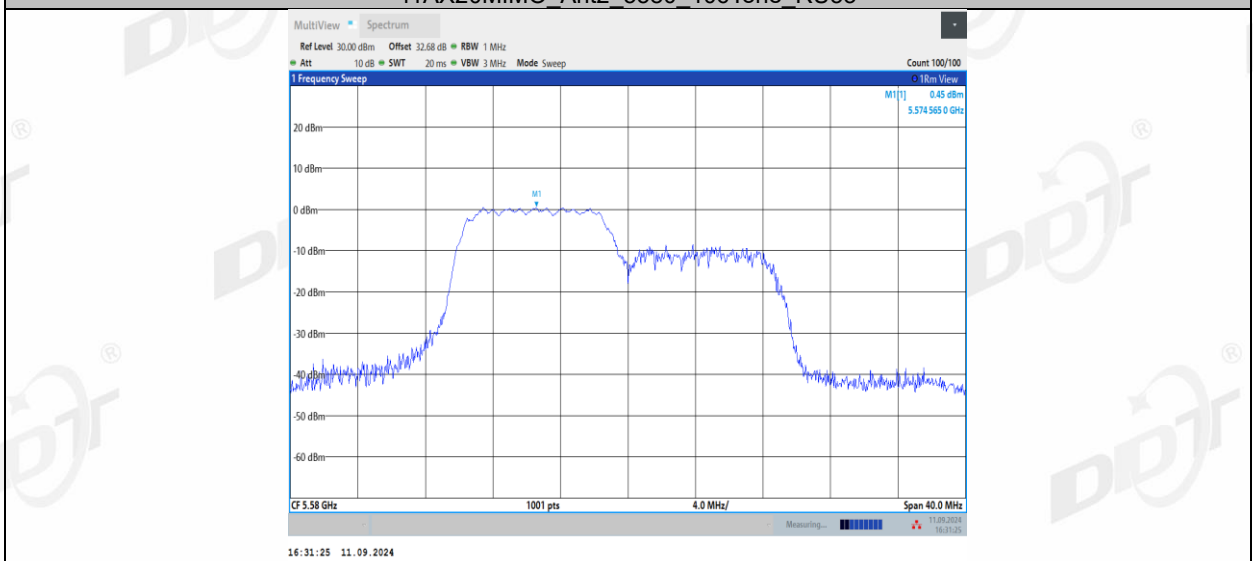
11AX20MIMO_Ant2_5580_106Tone_RU54
