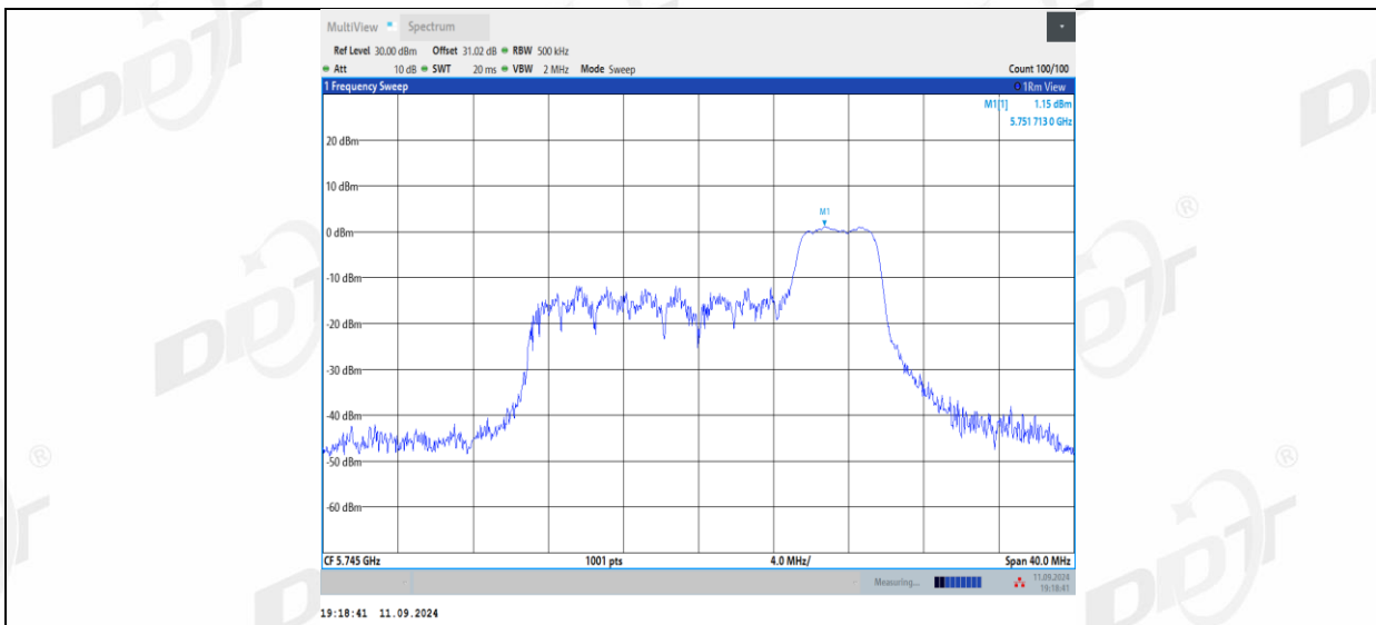
11AX20MIMO_Ant2_5745_106Tone_RU53
