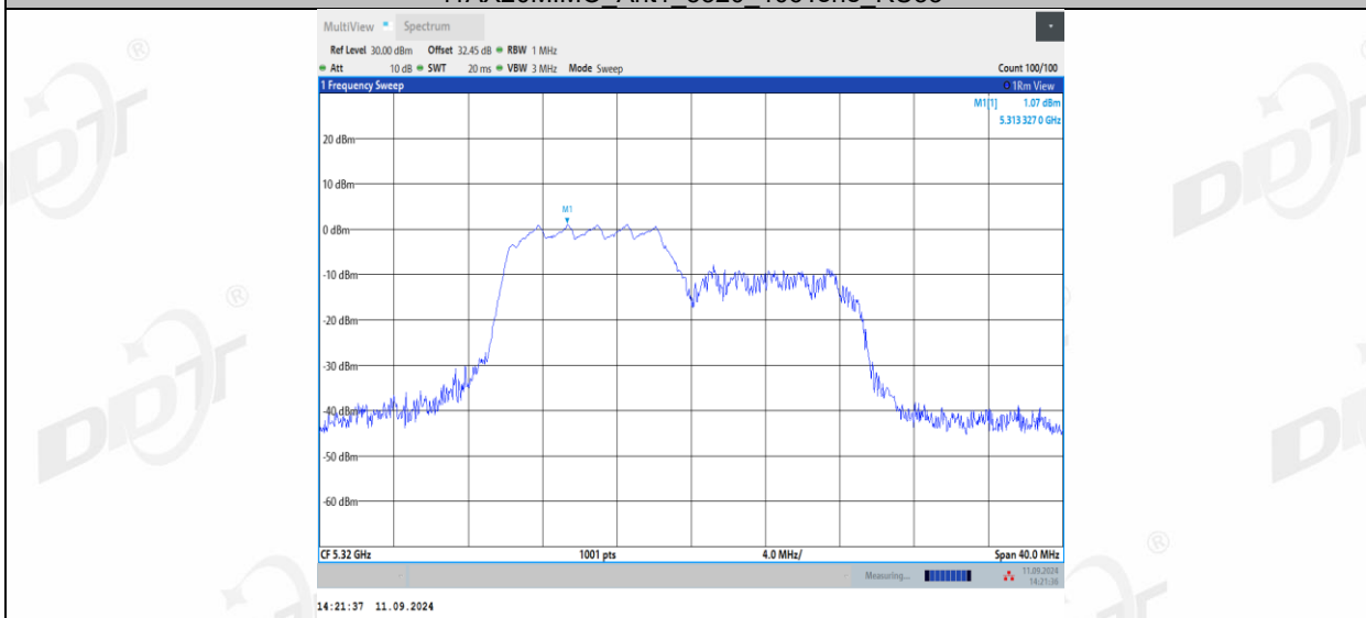
11AX20MIMO_Ant1_5320_106Tone_RU54
