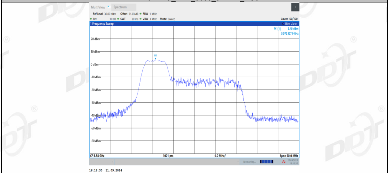
11AX20MIMO_Ant2_5580_52Tone_RU39
