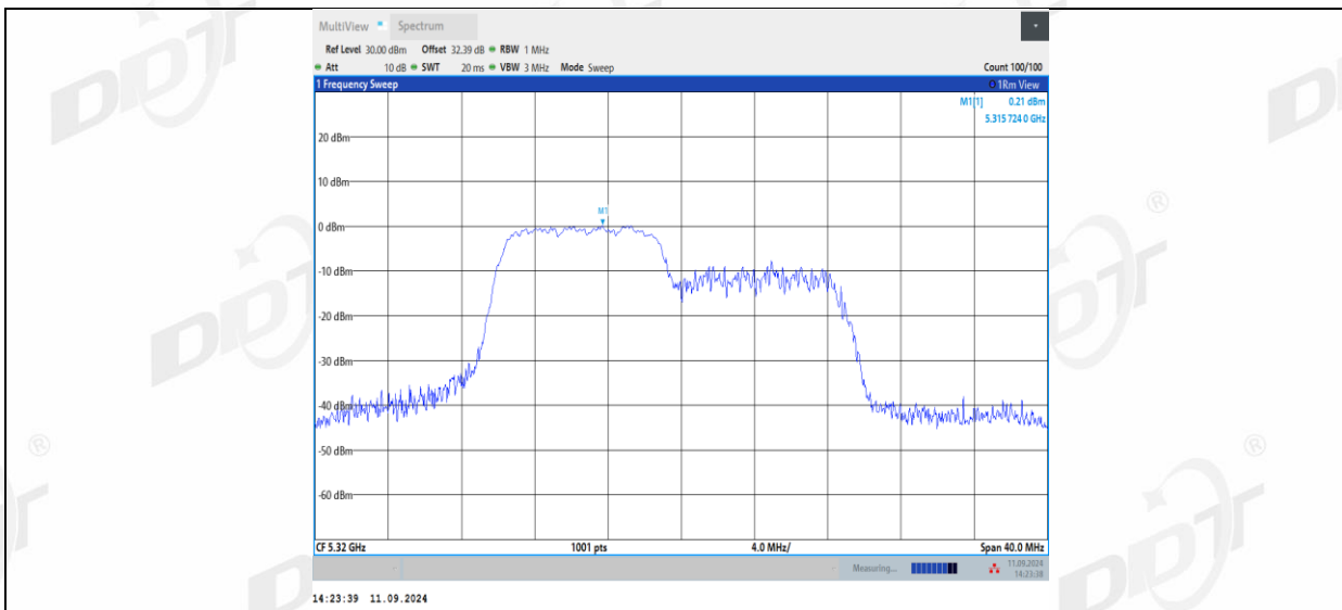
11AX20MIMO_Ant2_5320_106Tone_RU54
