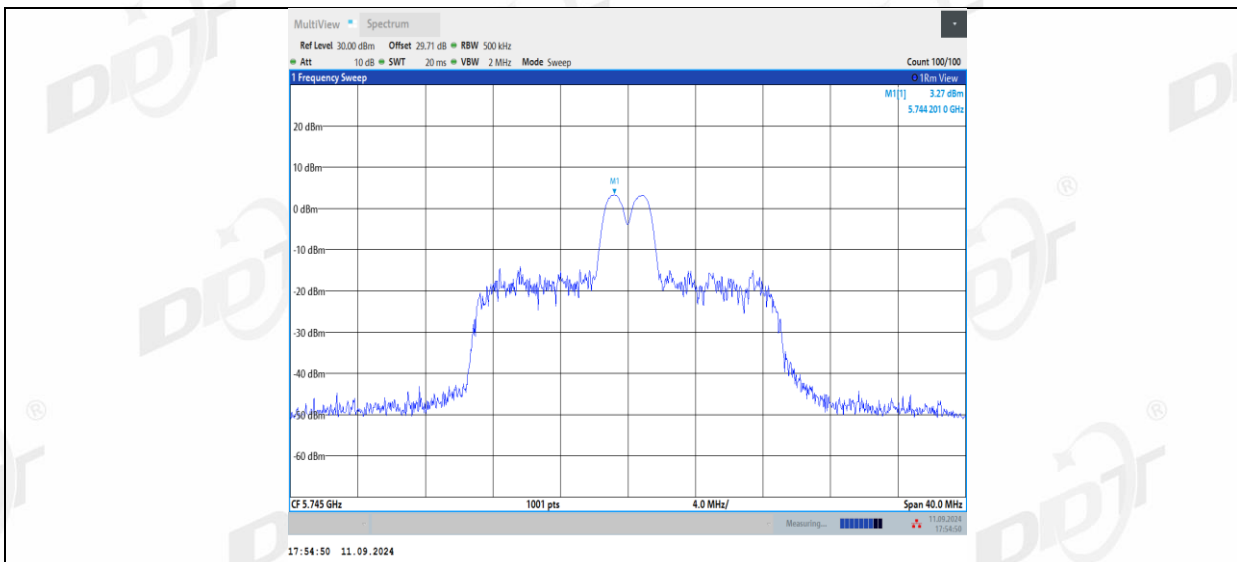
11AX20MIMO_Ant1_5745_26Tone_RU8
