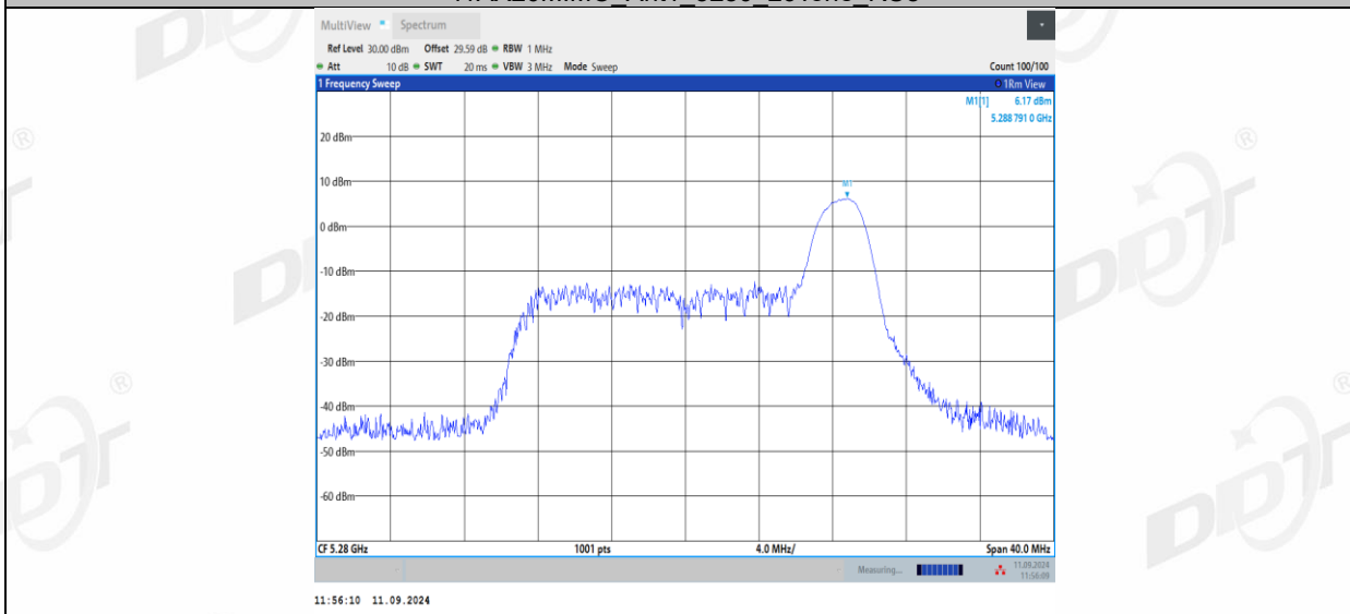
11AX20MIMO_Ant1_5280_52Tone_RU37
