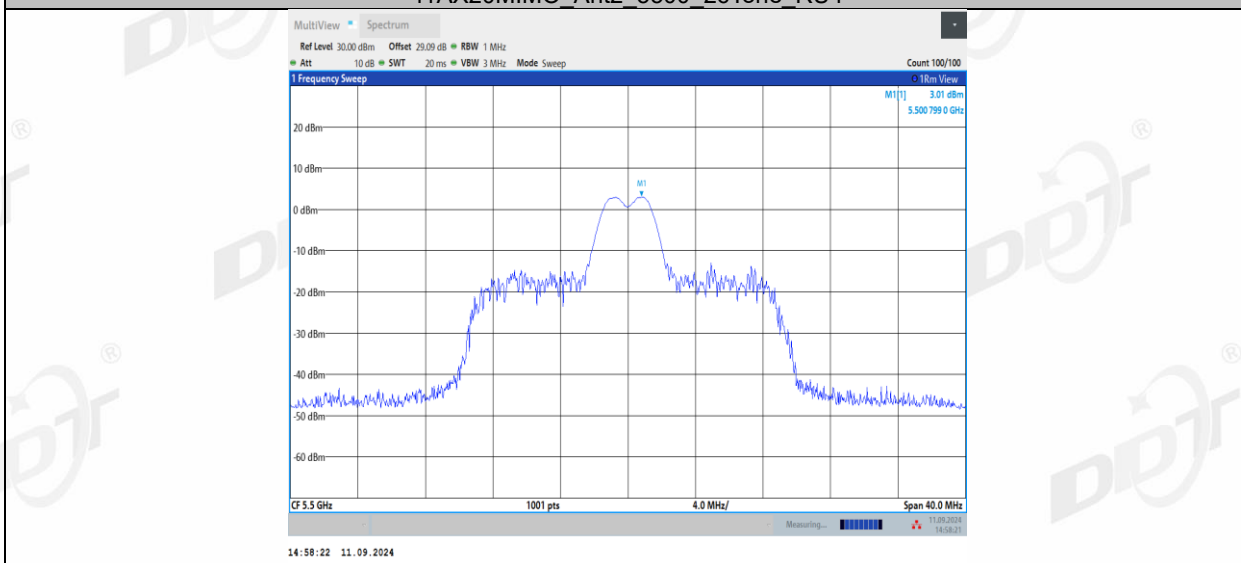
11AX20MIMO_Ant2_5500_26Tone_RU8
