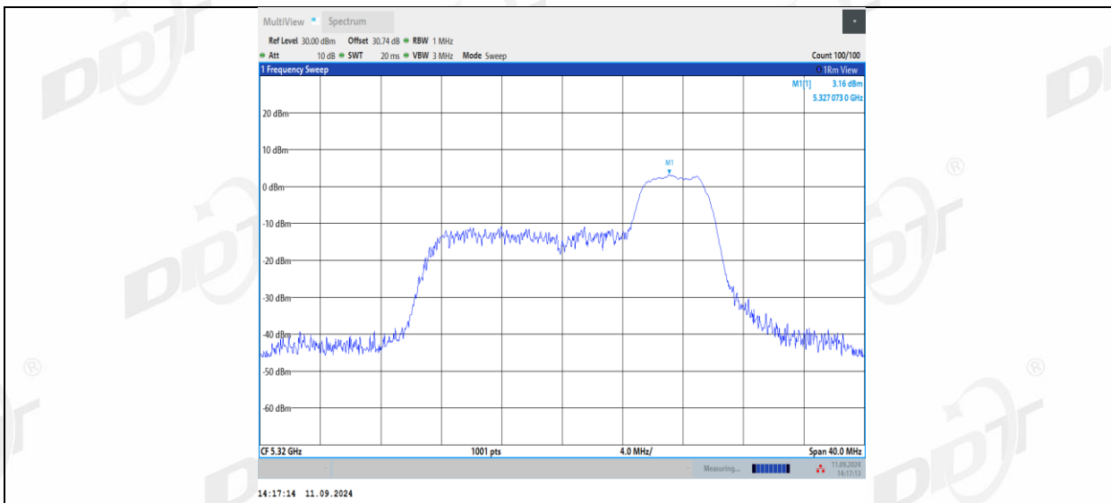
11AX20MIMO_Ant1_5320_106Tone_RU53
