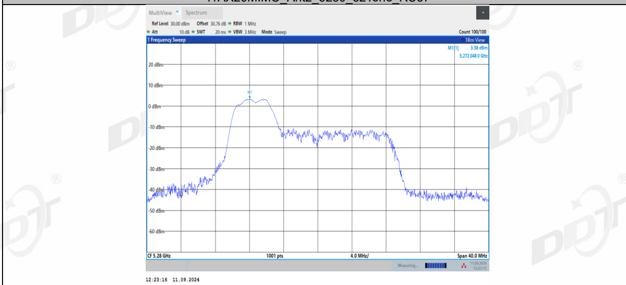
11AX20MIMO_Ant2_5280_52Tone_RU39
