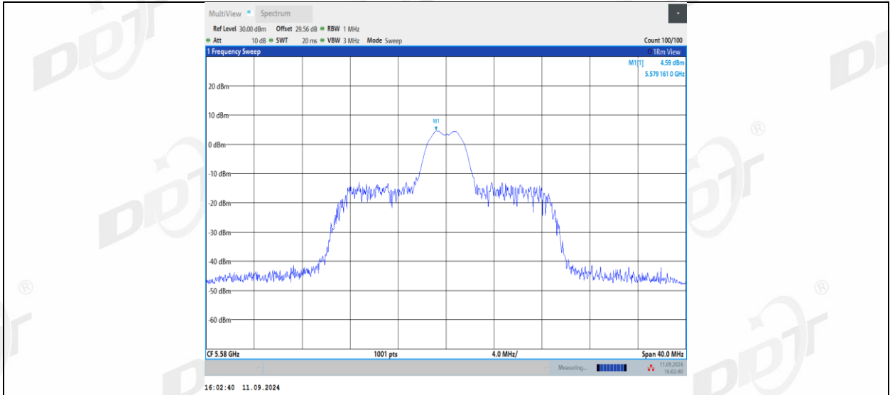
11AX20MIMO_Ant2_5580_26Tone_RU8
