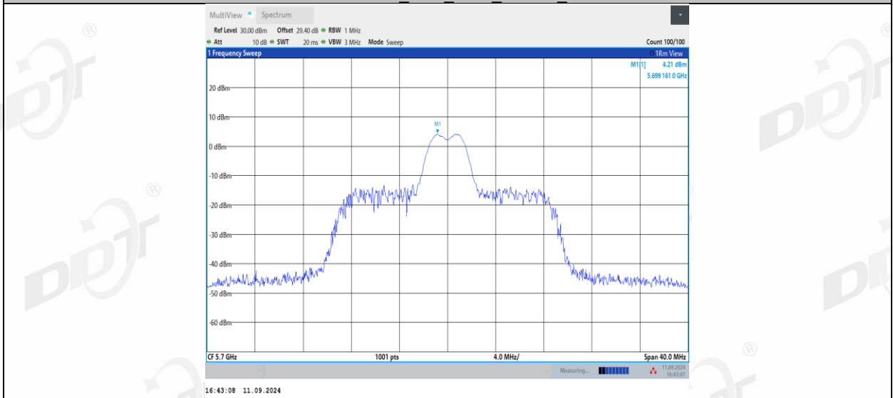
11AX20MIMO_Ant2_5700_26Tone_RU5
