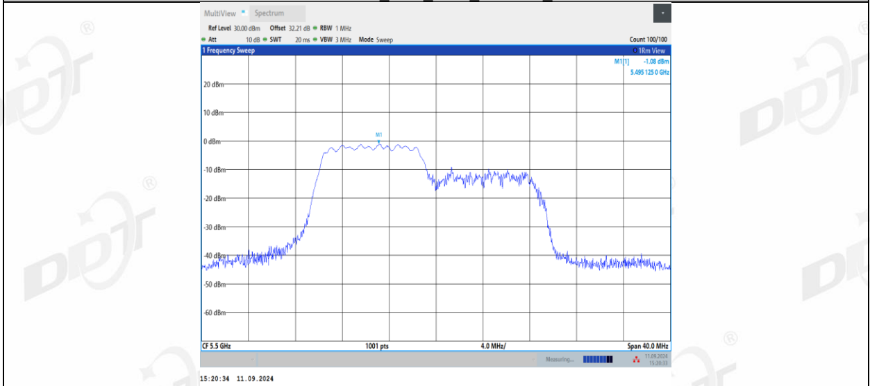
11AX20MIMO_Ant2_5500_106Tone_RU54
