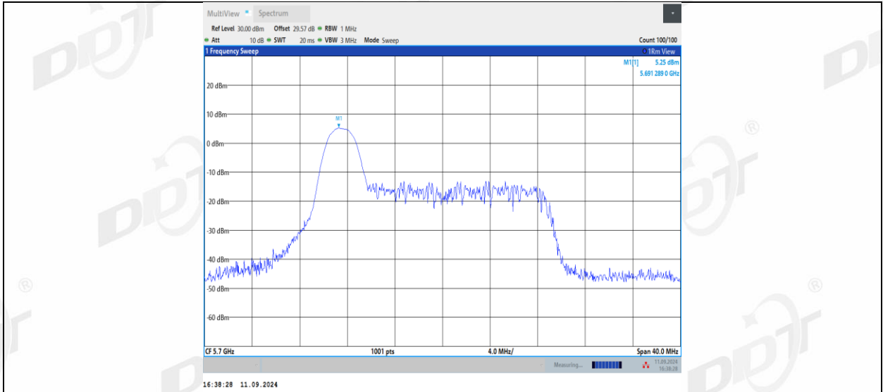
11AX20MIMO_Ant2_5700_26Tone_RU4
