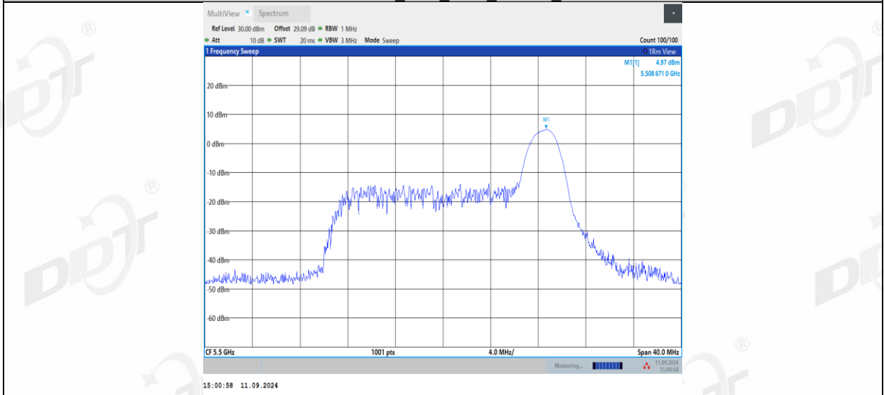
11AX20MIMO_Ant1_5500_52Tone_RU37
