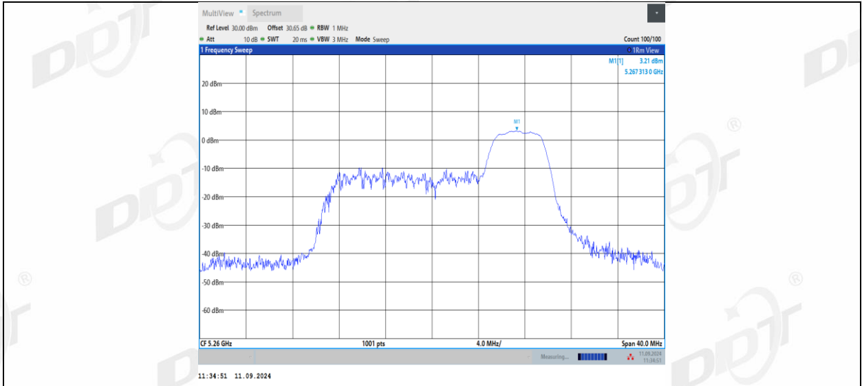
11AX20MIMO_Ant2_5260_106Tone_RU53
