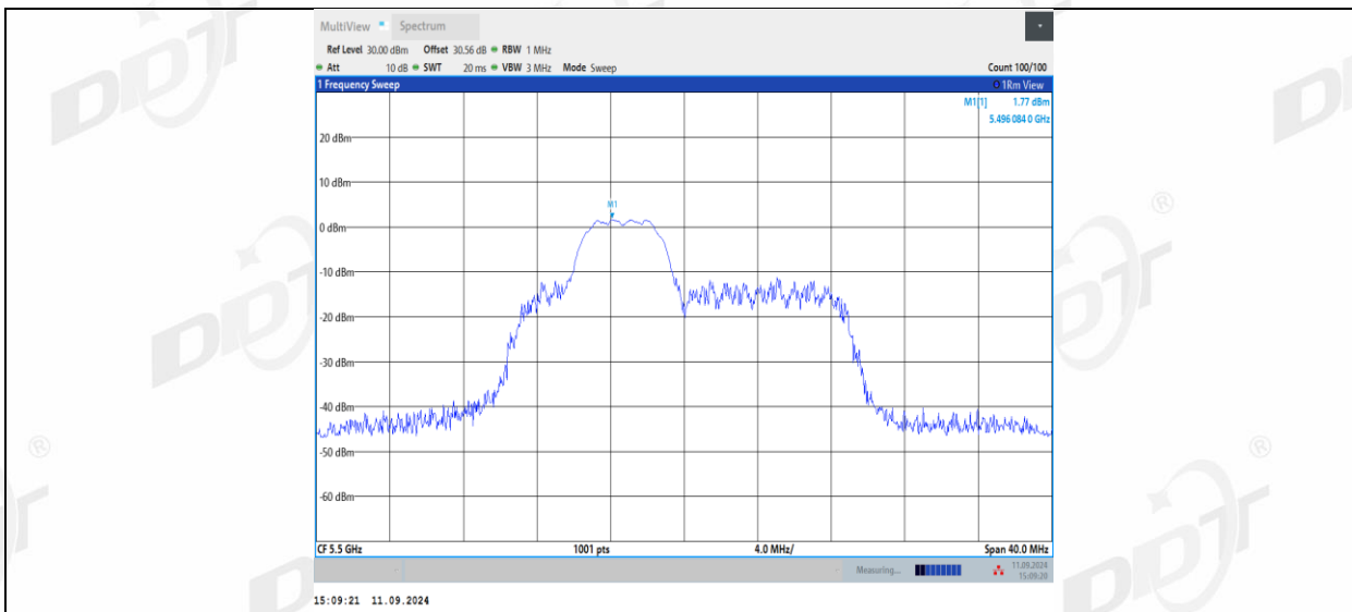
11AX20MIMO_Ant1_5500_52Tone_RU40
