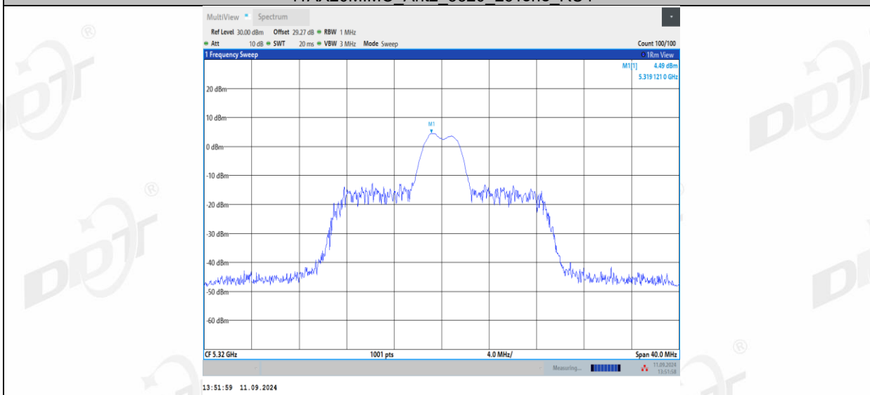
11AX20MIMO_Ant2_5320_26Tone_RU5
