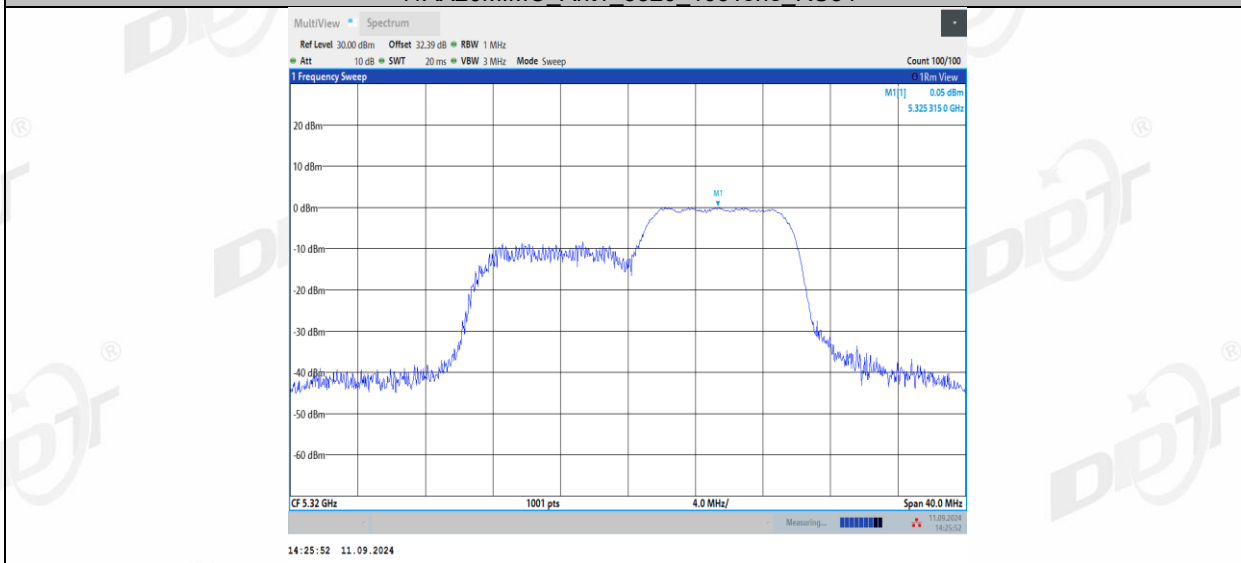
11AX20MIMO_Ant2_5320_26Tone_RU0
