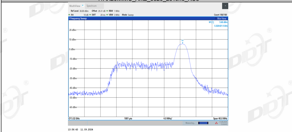
11AX20MIMO_Ant2_5320_52Tone_RU7
