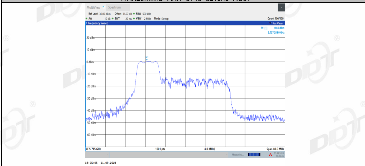
11AX20MIMO_Ant1_5745_52Tone_RU39
