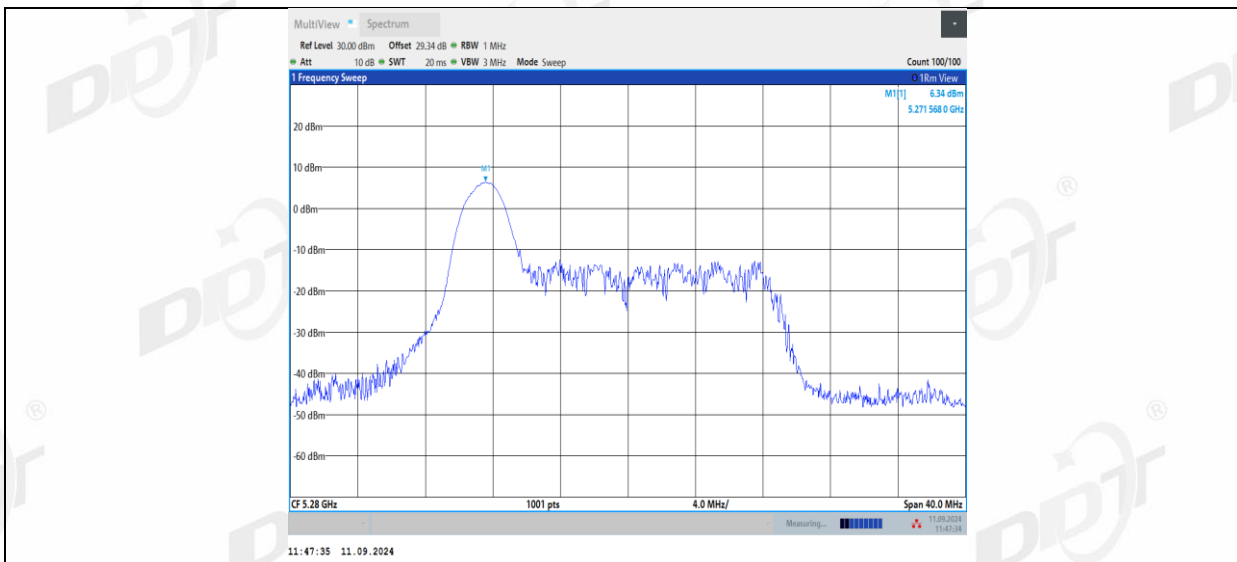
11AX20MIMO_Ant1_5280_26Tone_RU4
