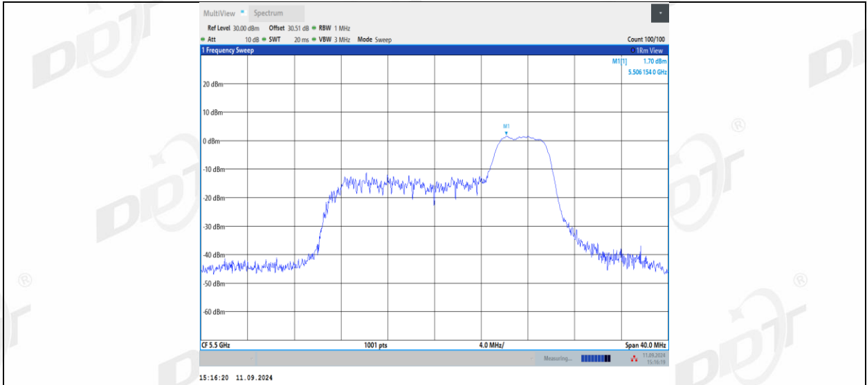
11AX20MIMO_Ant2_5500_106Tone_RU53
