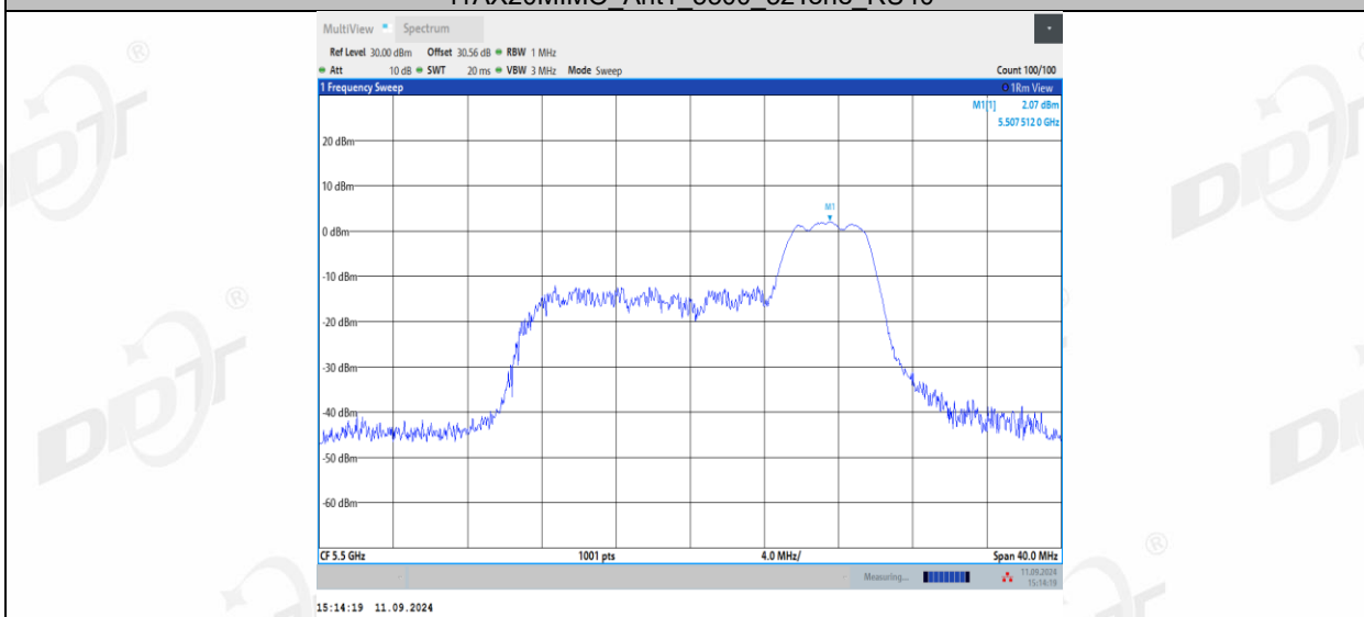
11AX20MIMO_Ant1_5500_106Tone_RU53
