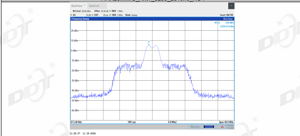
11AX20MIMO_Ant1_5280_26Tone_RU8
