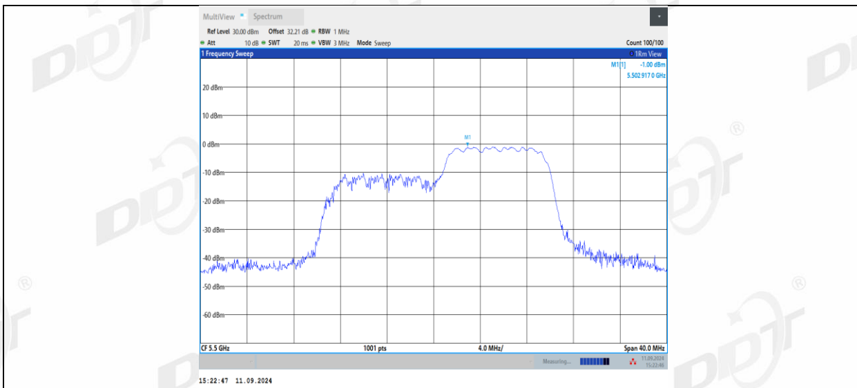
11AX20MIMO_Ant2_5500_26Tone_RU0
