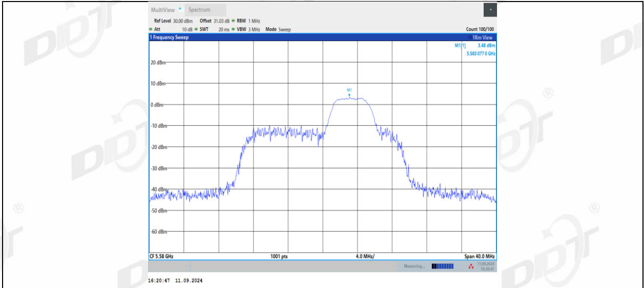
11AX20MIMO_Ant2_5580_52Tone_RU40
