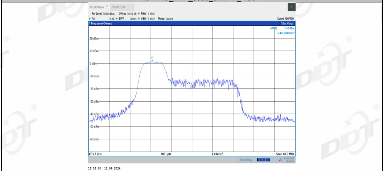
11AX20MIMO_Ant1_5500_52Tone_RU39
