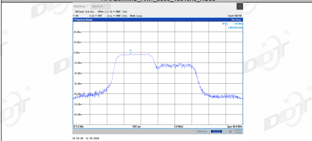
11AX20MIMO_Ant1_5500_106Tone_RU54
