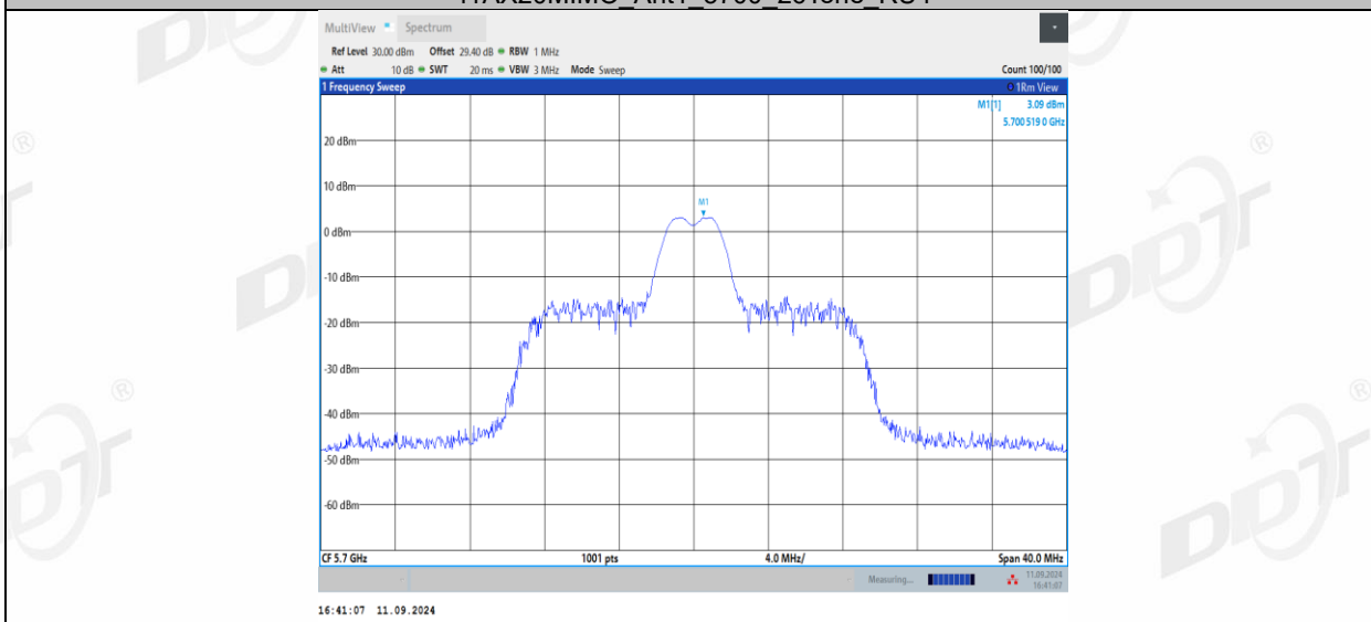
11AX20MIMO_Ant1_5700_26Tone_RU8
