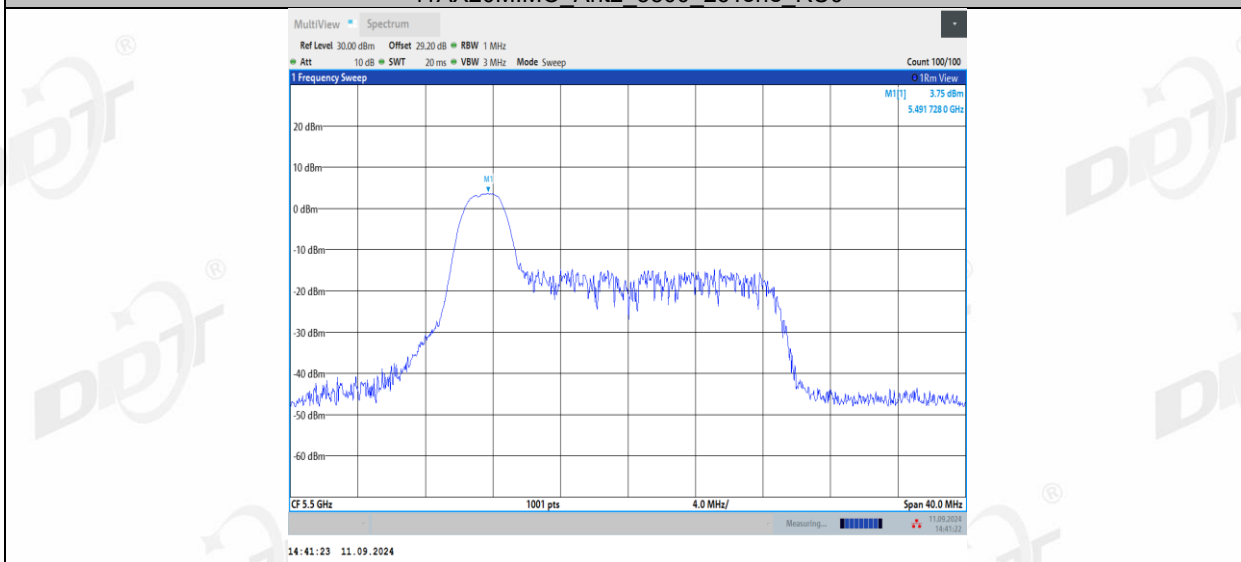
11AX20MIMO_Ant2_5500_26Tone_RU4
