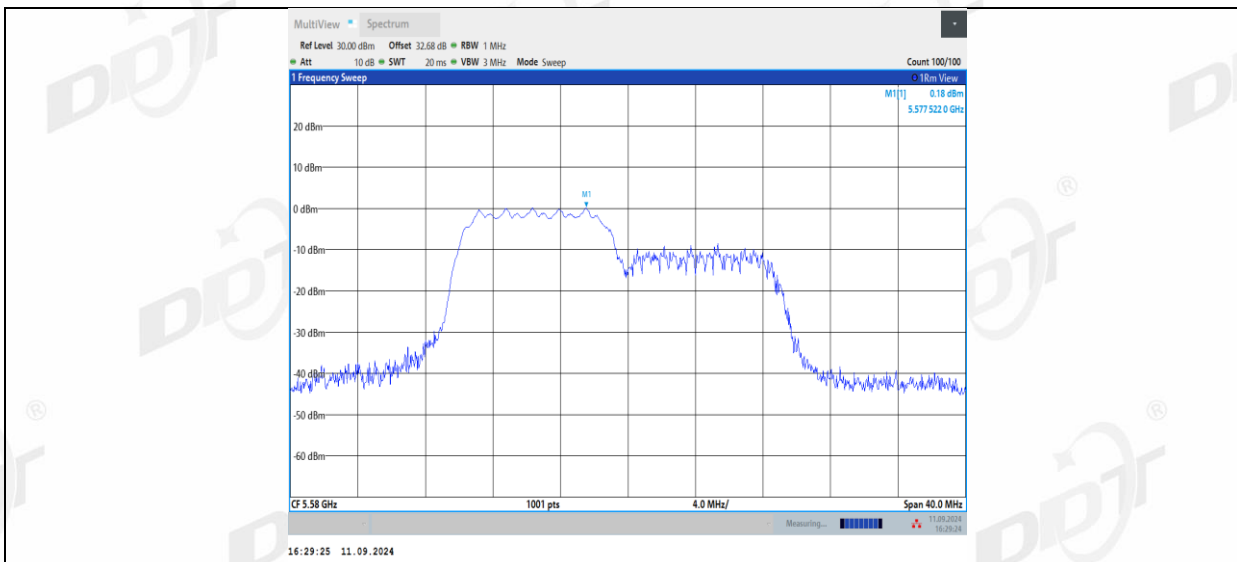
11AX20MIMO_Ant1_5580_106Tone_RU54
