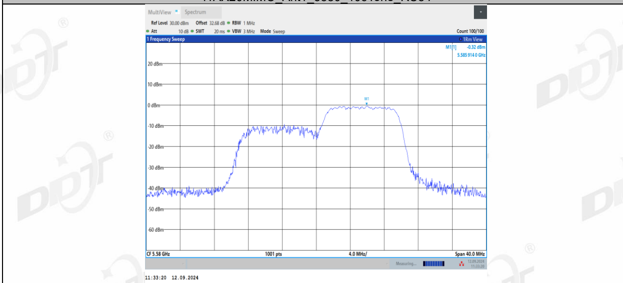
11AX20MIMO_Ant2_5580_26Tone_RU0
