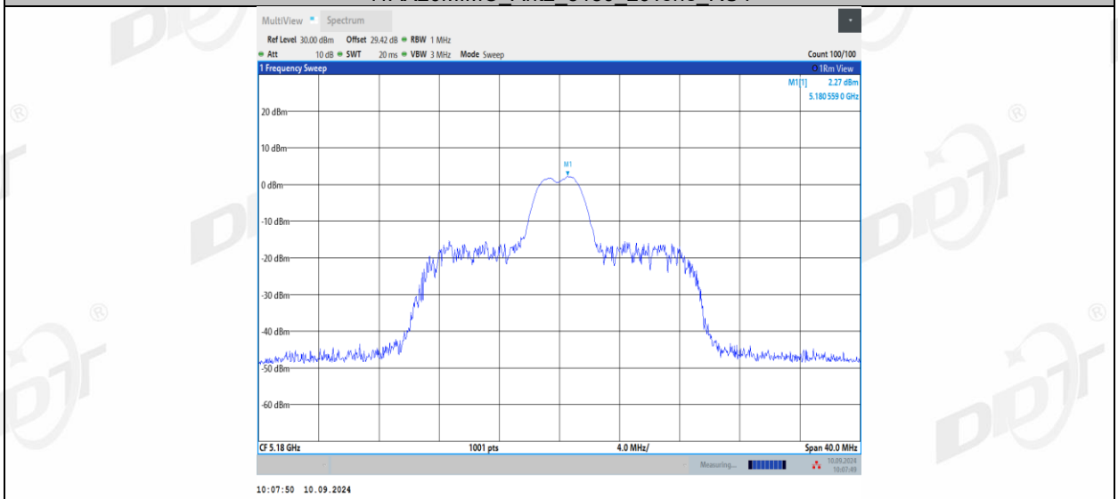
11AX20MIMO_Ant2_5180_26Tone_RU8
