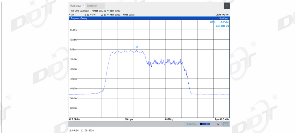
11AX20MIMO_Ant2_5240_106Tone_RU54
