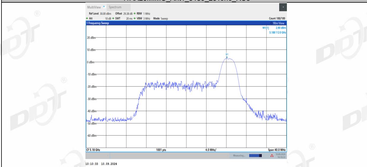
11AX20MIMO_Ant1_5180_52Tone_RU37
