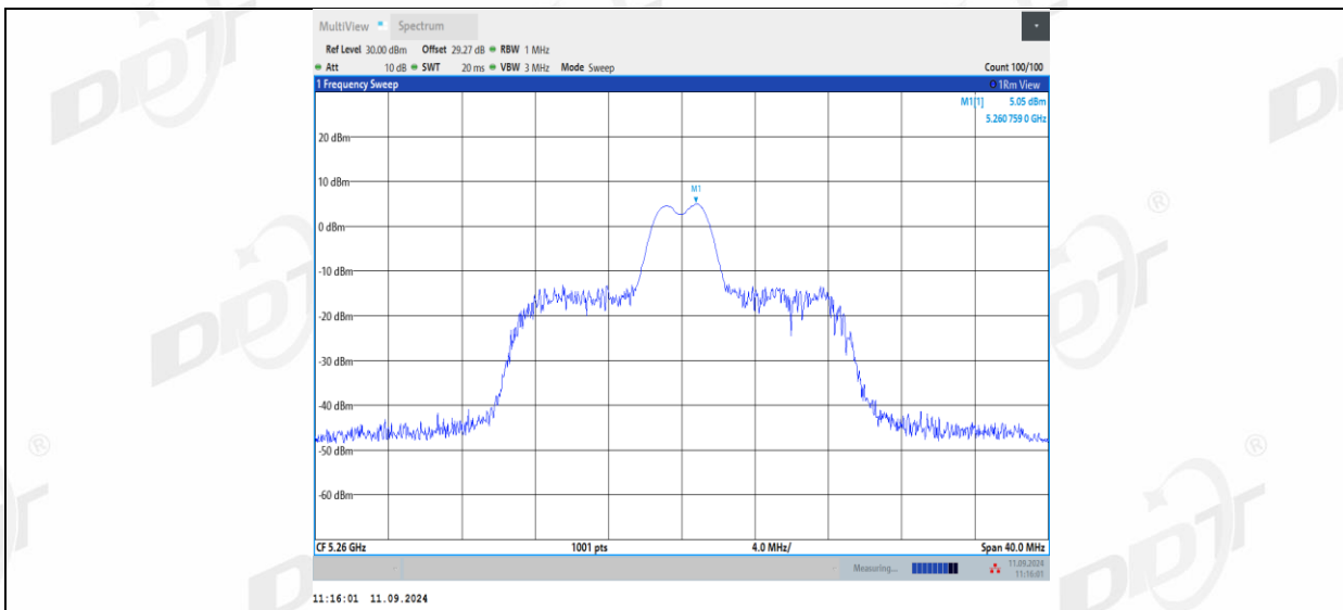
11AX20MIMO_Ant1_5260_26Tone_RU8
