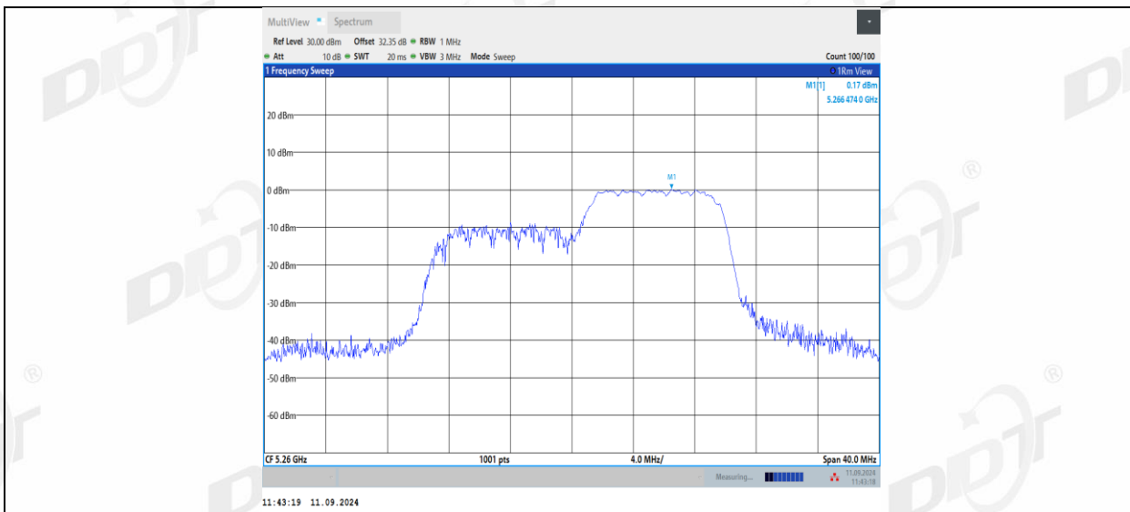
11AX20MIMO_Ant2_5260_26Tone_RU0
