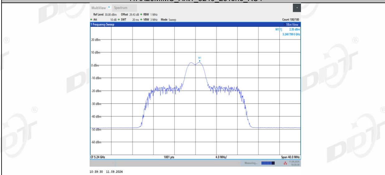
11AX20MIMO_Ant1_5240_26Tone_RU8
