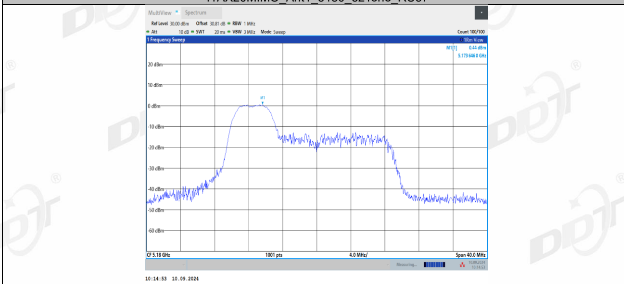
11AX20MIMO_Ant1_5180_52Tone_RU39
