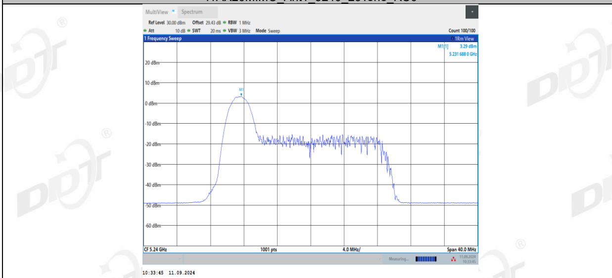
11AX20MIMO_Ant1_5240_26Tone_RU4
