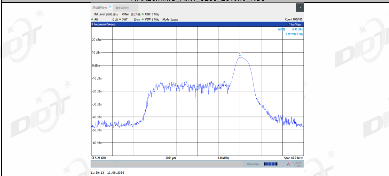
11AX20MIMO_Ant1_5260_52Tone_RU37
