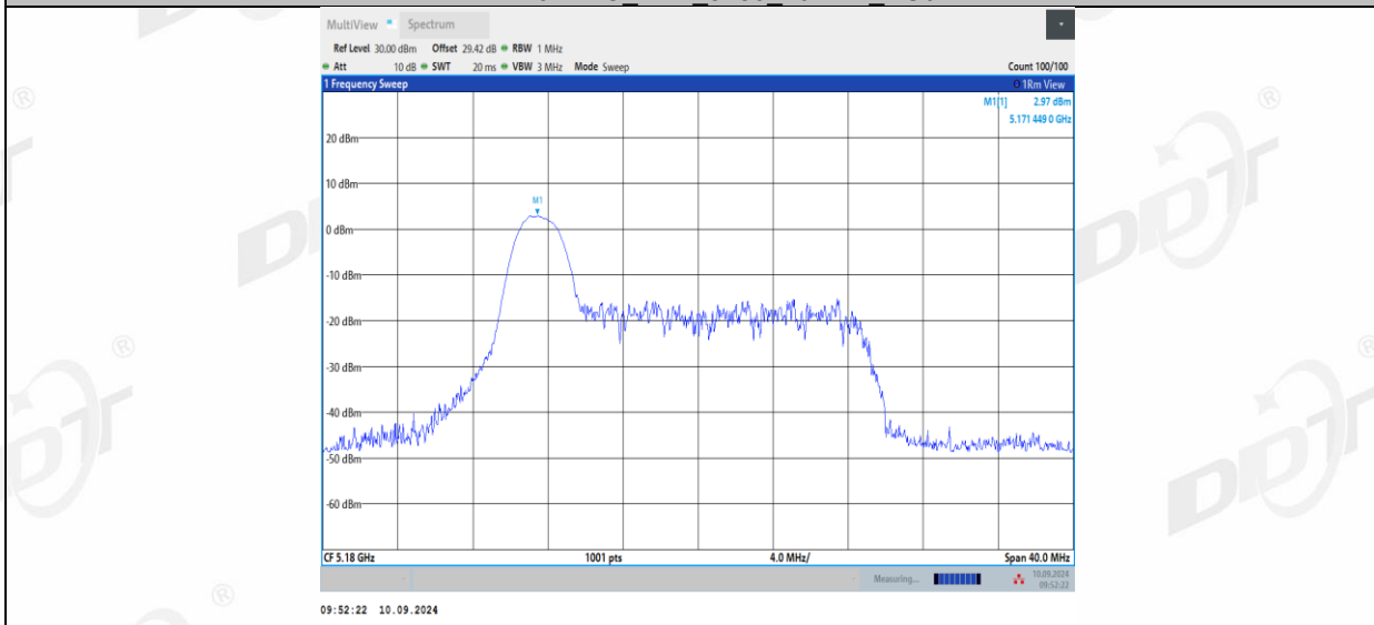
11AX20MIMO_Ant1_5180_26Tone_RU4
