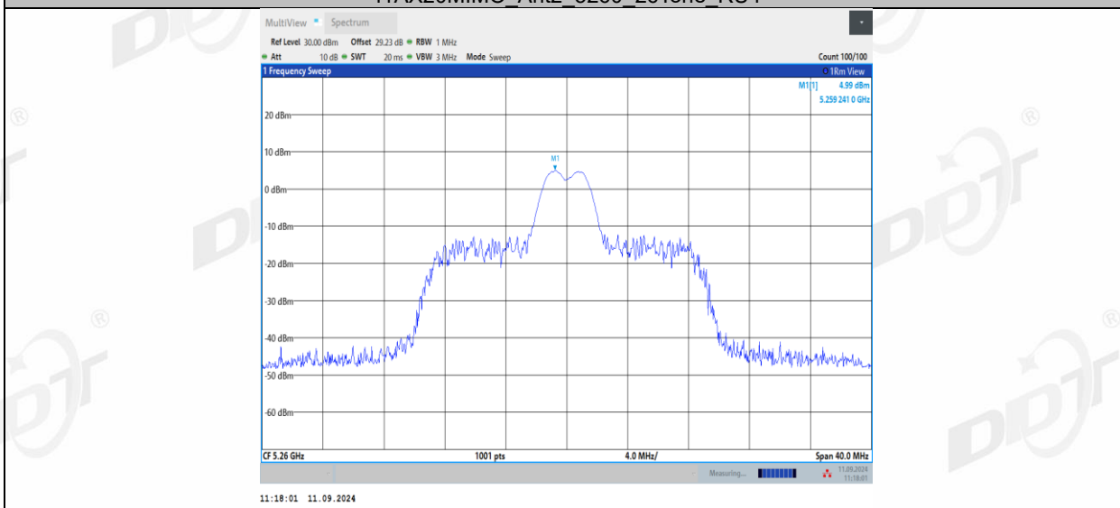
11AX20MIMO_Ant2_5260_26Tone_RU8
