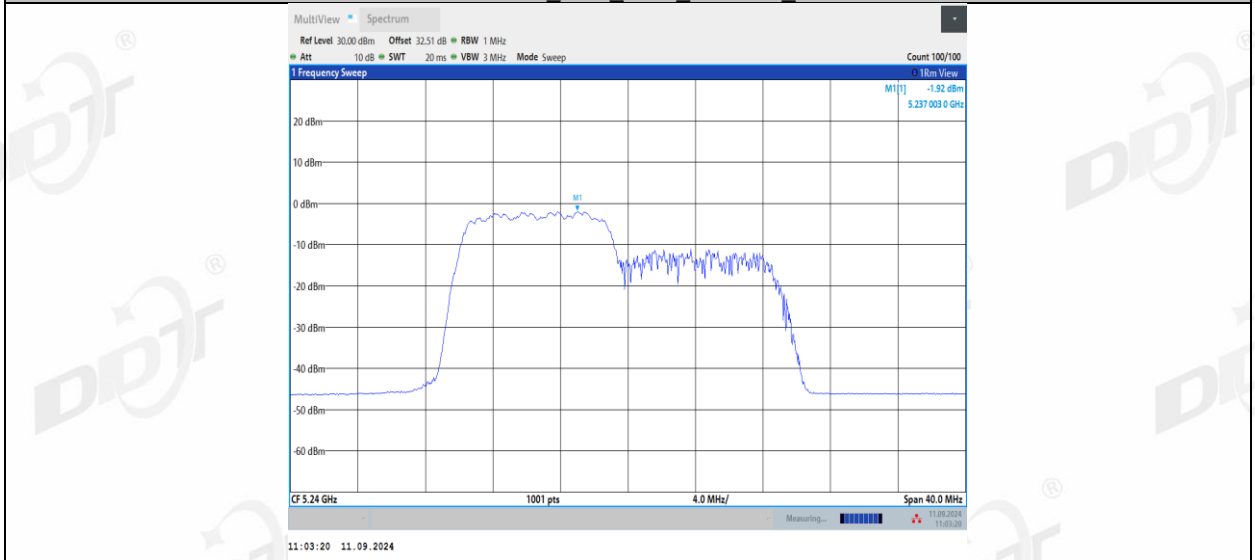
11AX20MIMO_Ant1_5240_106Tone_RU54
