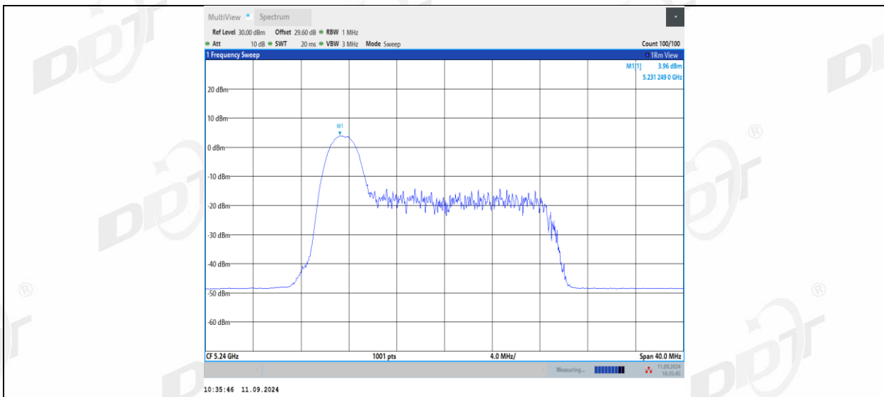
11AX20MIMO_Ant2_5240_26Tone_RU4
