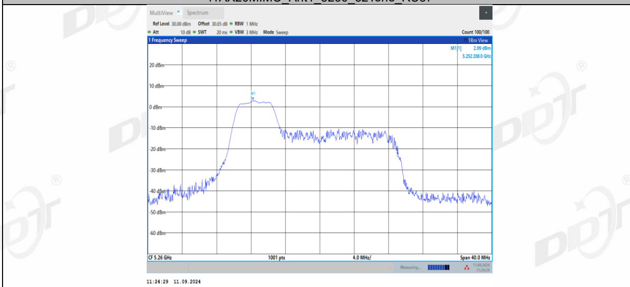
11AX20MIMO_Ant1_5260_52Tone_RU39
