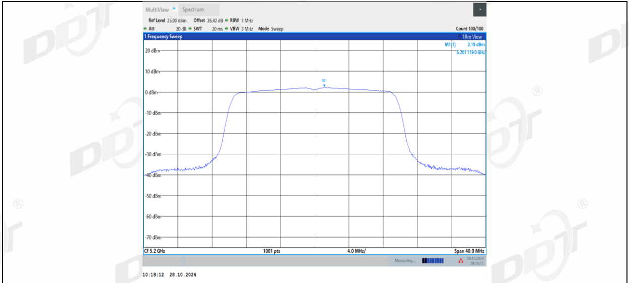
11AX20MIMO_Ant2_5200
