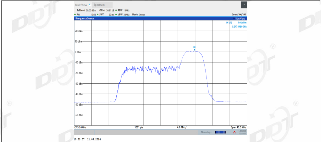
11AX20MIMO_Ant1_5240_106Tone_RU53
