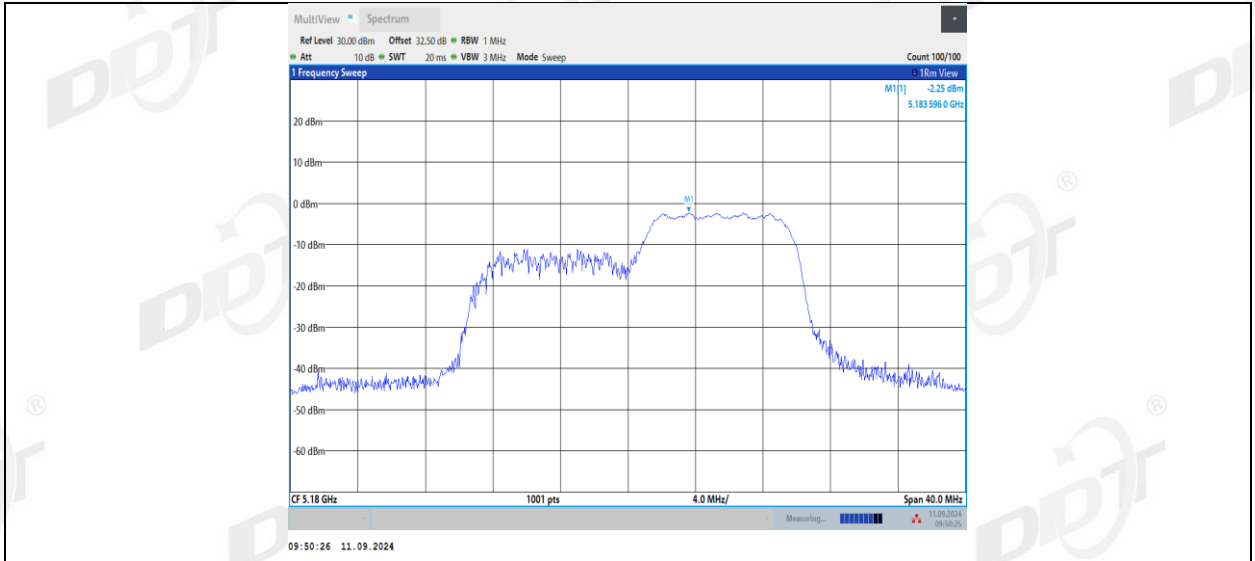
11AX20MIMO_Ant2_5180_26Tone_RU0
