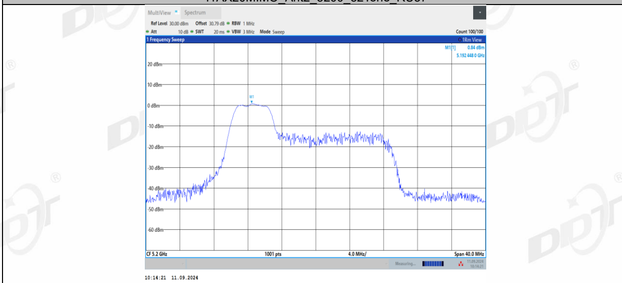
11AX20MIMO_Ant2_5200_52Tone_RU39
