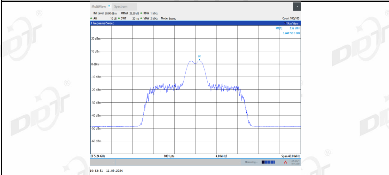
11AX20MIMO_Ant2_5240_26Tone_RU8
