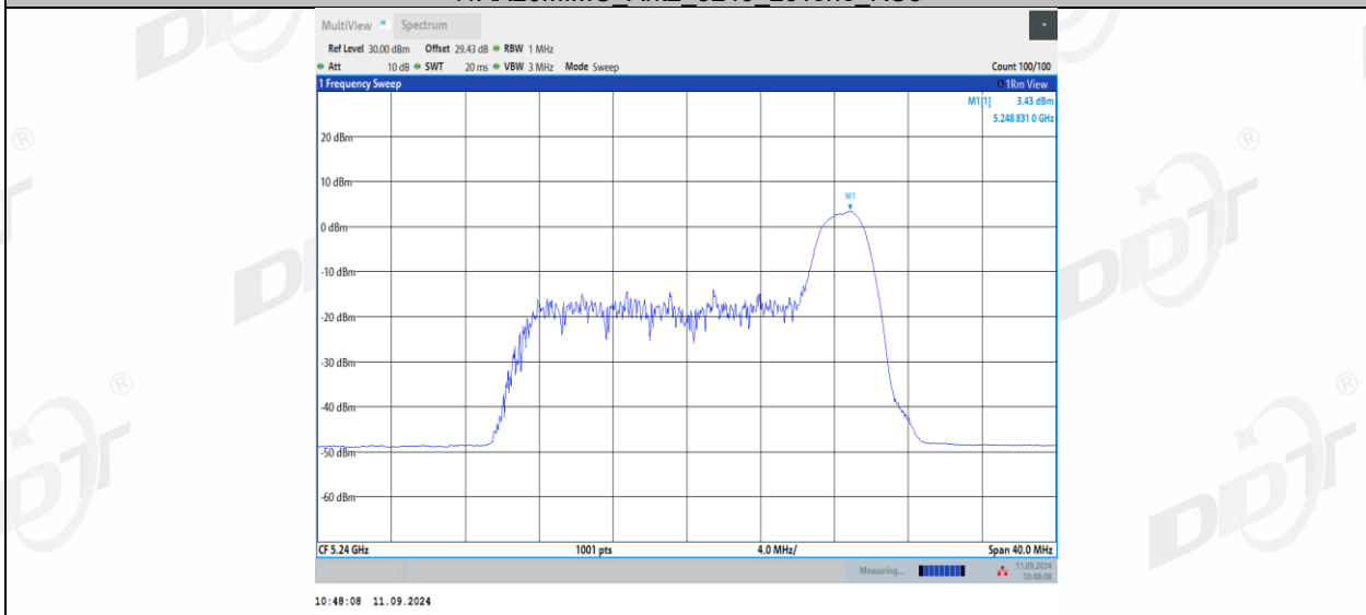
11AX20MIMO_Ant2_5240_52Tone_RU37
