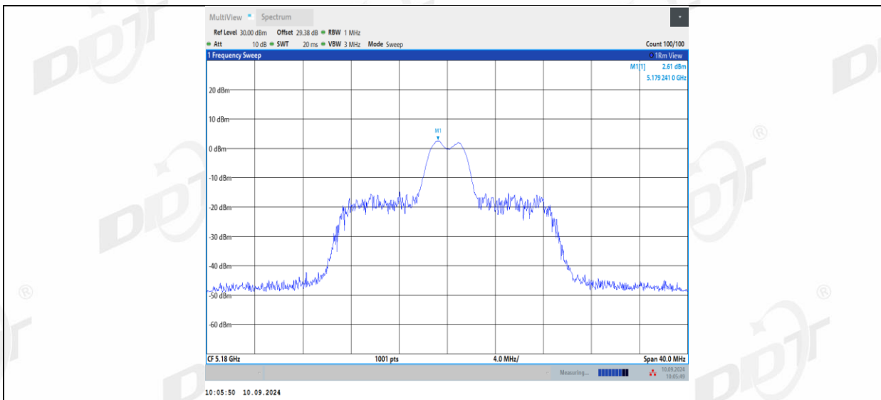
11AX20MIMO_Ant1_5180_26Tone_RU8
