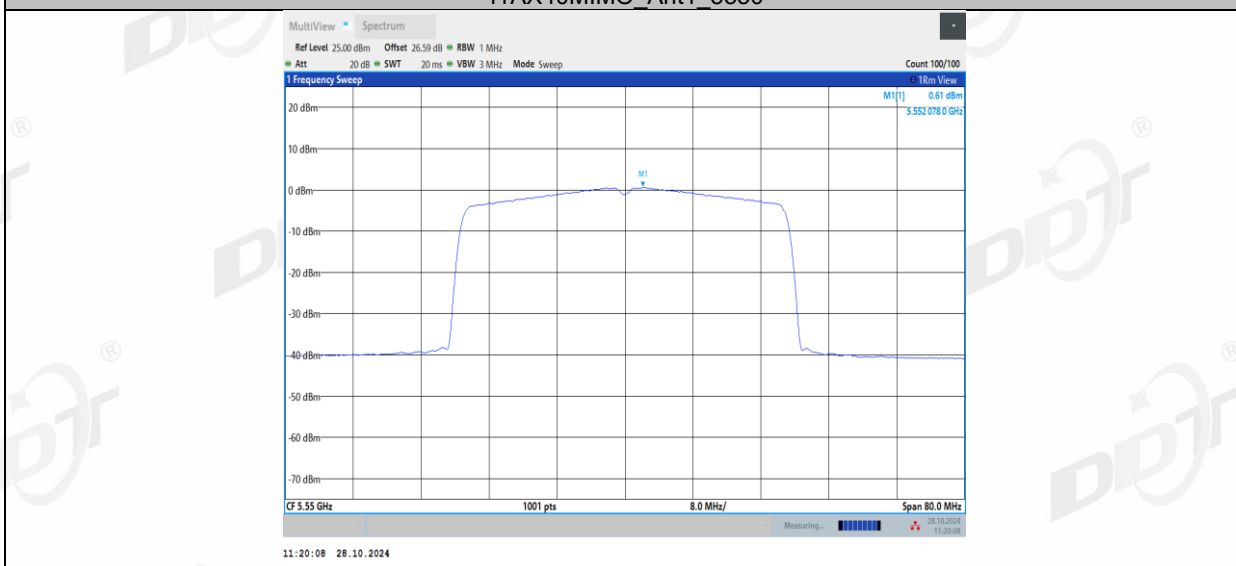
11AX40MIMO_Ant2_5550
