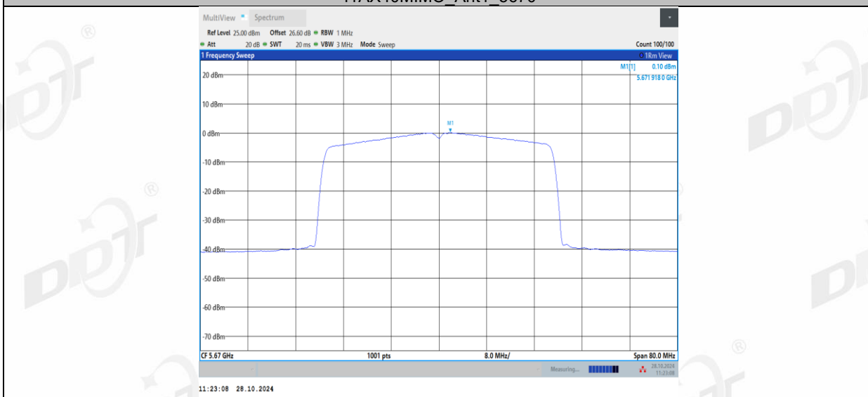
11AX40MIMO_Ant2_5670
