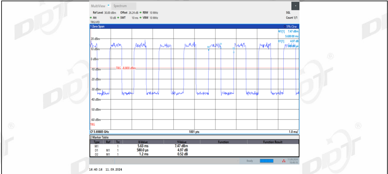
11AX20MIMO_Ant1_5700_26Tone_RU8
