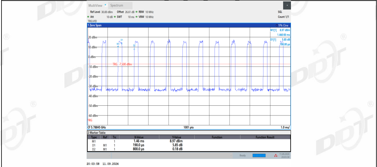
11AX20MIMO_Ant2_5785_26Tone_RU0
