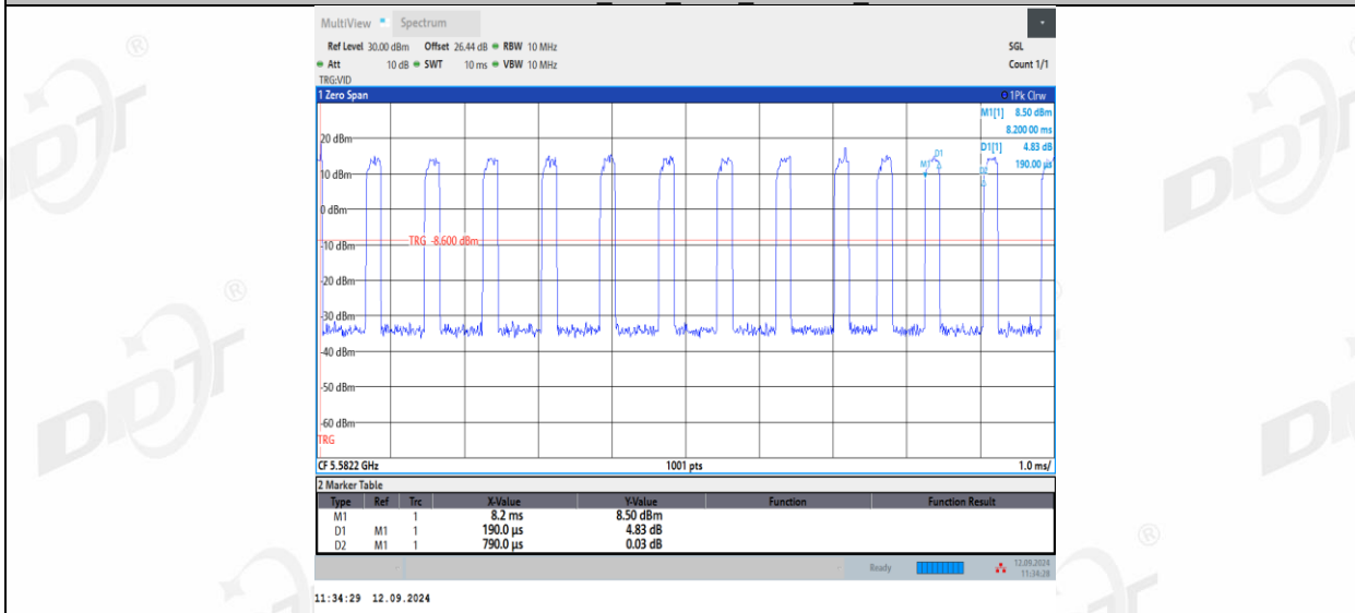
11AX20MIMO_Ant1_5700_26Tone_RU0
