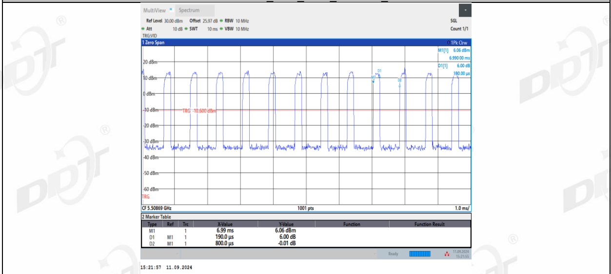
11AX20MIMO_Ant2_5500_26Tone_RU0
