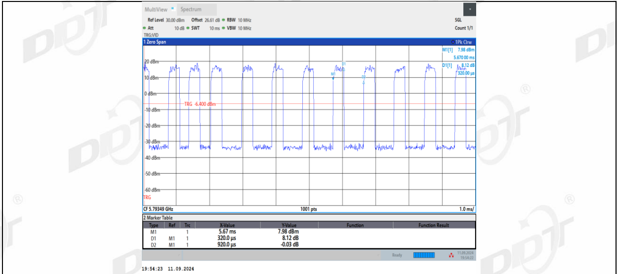
11AX20MIMO_Ant1_5785_106Tone_RU53
