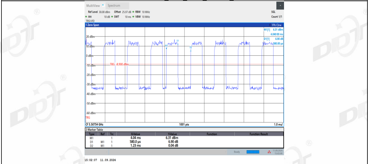
11AX20MIMO_Ant2_5500_52Tone_RU37
