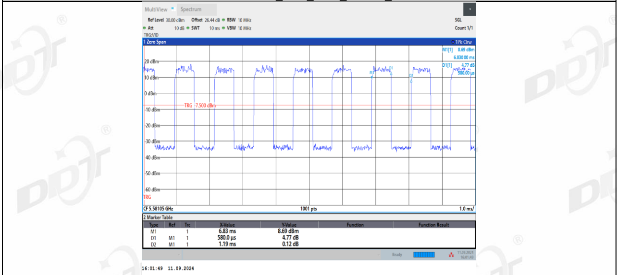
11AX20MIMO_Ant2_5580_26Tone_RU8
