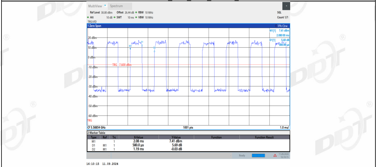
11AX20MIMO_Ant2_5580_52Tone_RU37
