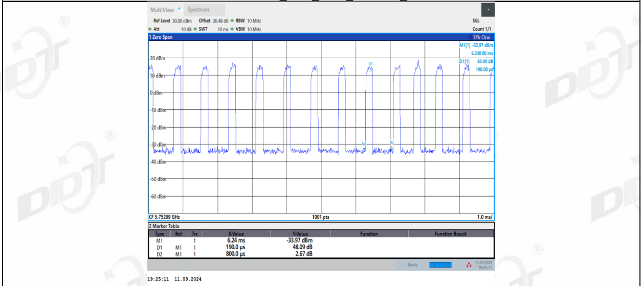
11AX20MIMO_Ant2_5745_26Tone_RU0
