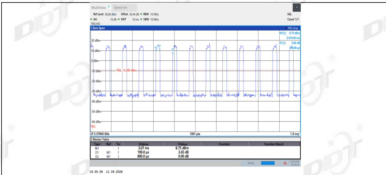
11AX20MIMO_Ant2_5580_106Tone_RU54
