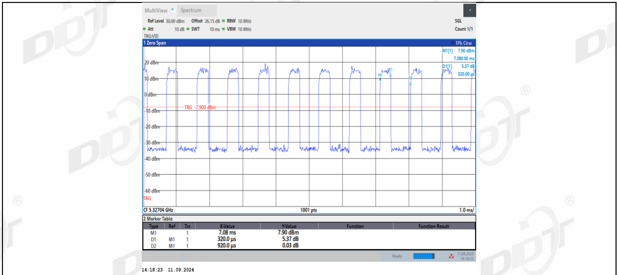
11AX20MIMO_Ant2_5320_106Tone_RU53
