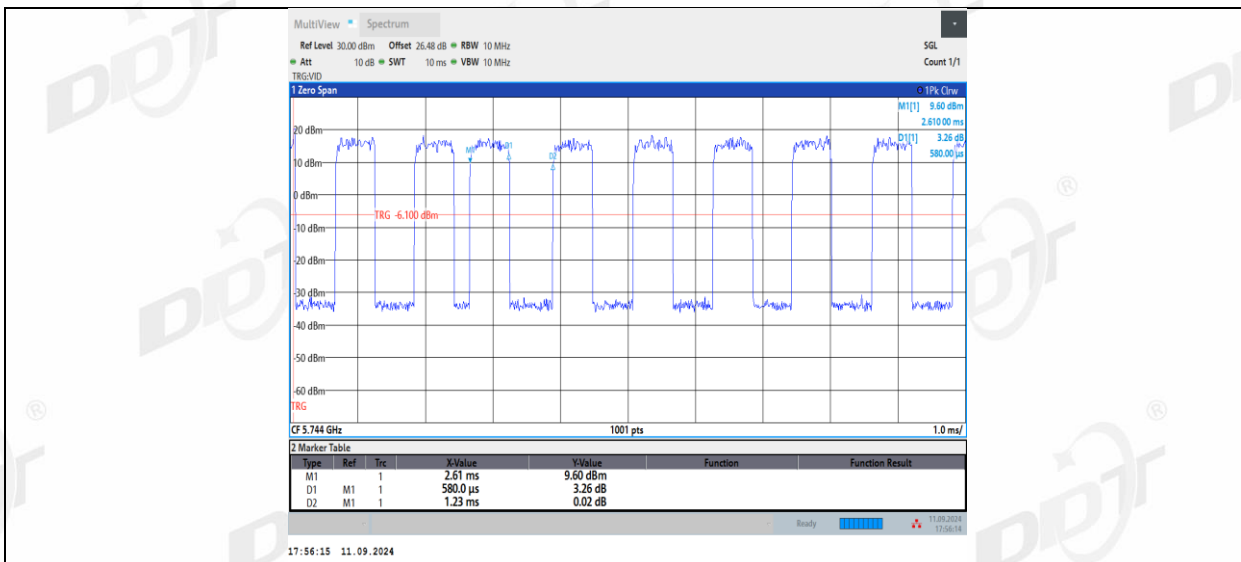
11AX20MIMO_Ant2_5745_26Tone_RU8
