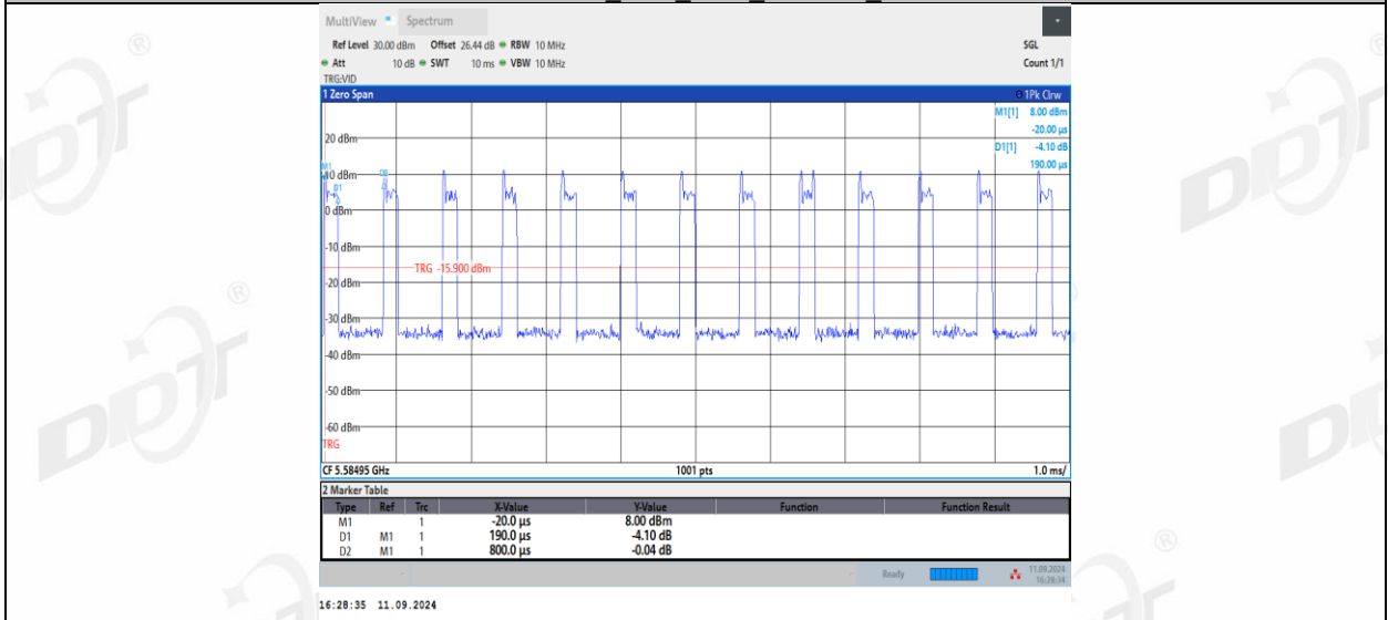
11AX20MIMO_Ant1_5580_106Tone_RU54
