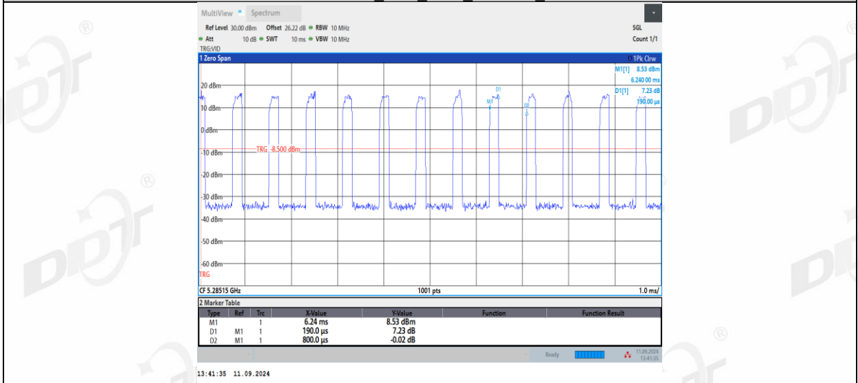
11AX20MIMO_Ant1_5320_26Tone_RU0
