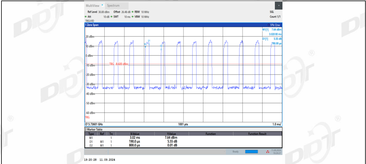
11AX20MIMO_Ant1_5745_106Tone_RU54
