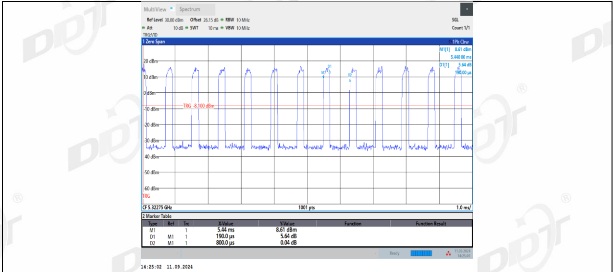
11AX20MIMO_Ant2_5320_26Tone_RU0
