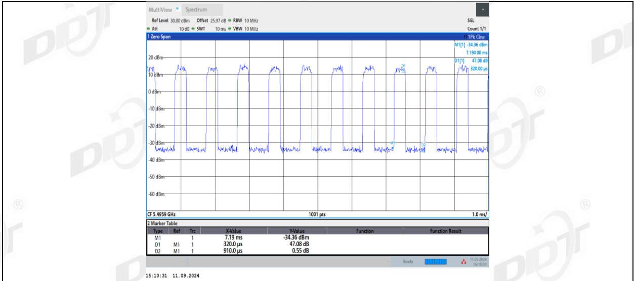
11AX20MIMO_Ant2_5500_52Tone_RU40
