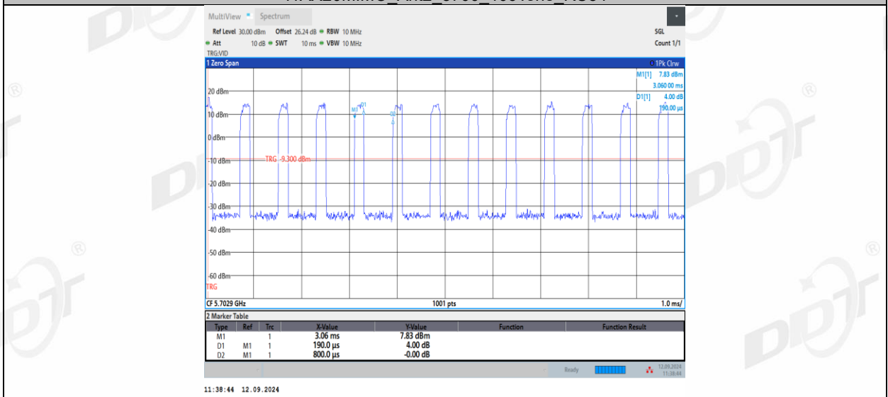
11AX20MIMO_Ant1_5745_26Tone_RU0
