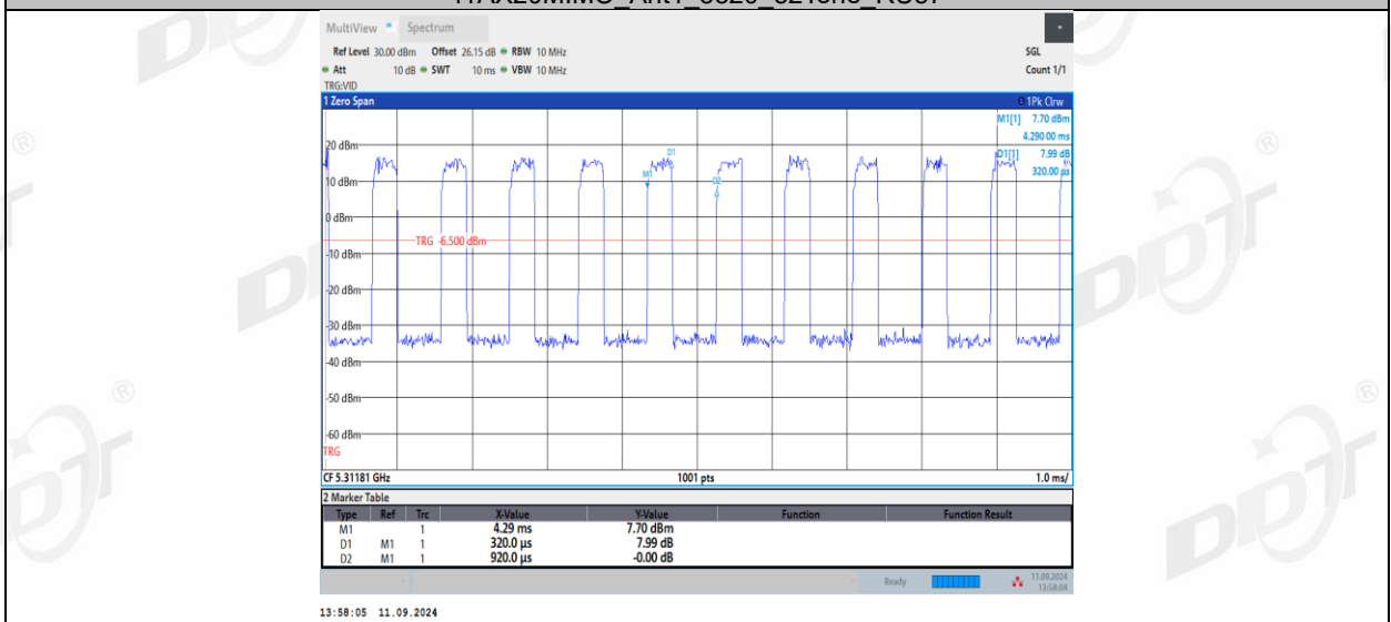
11AX20MIMO_Ant1_5320_52Tone_RU37
