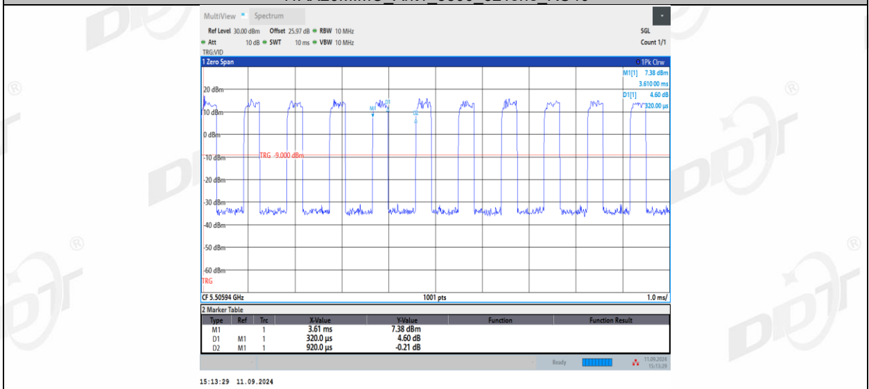
11AX20MIMO Ant1 5500_106Tone RU53
