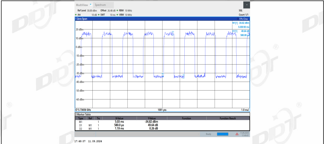
11AX20MIMO_Ant1_5745_26Tone_RU4
