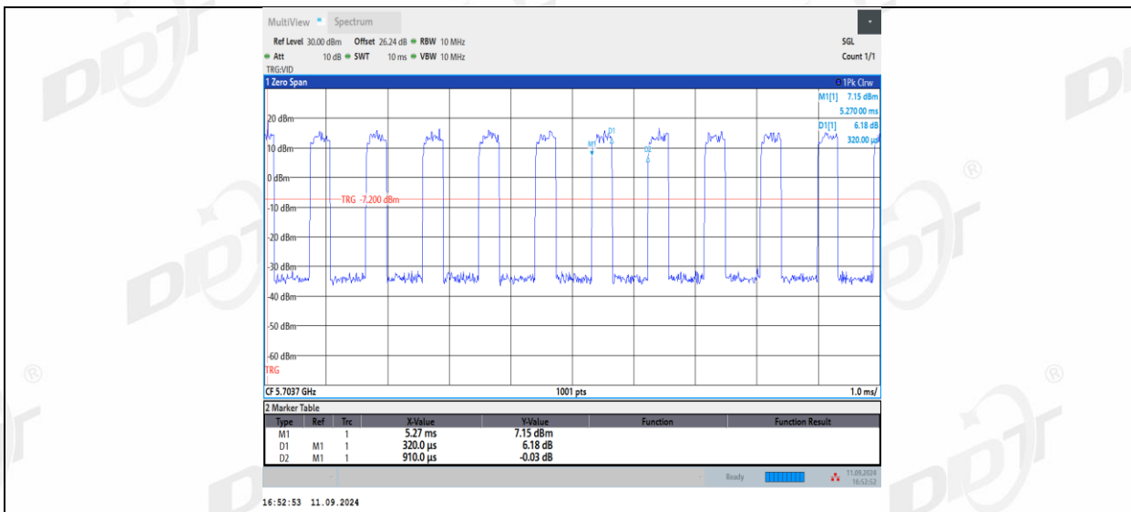
11AX20MIMO_Ant1_5700_52Tone_RU40
