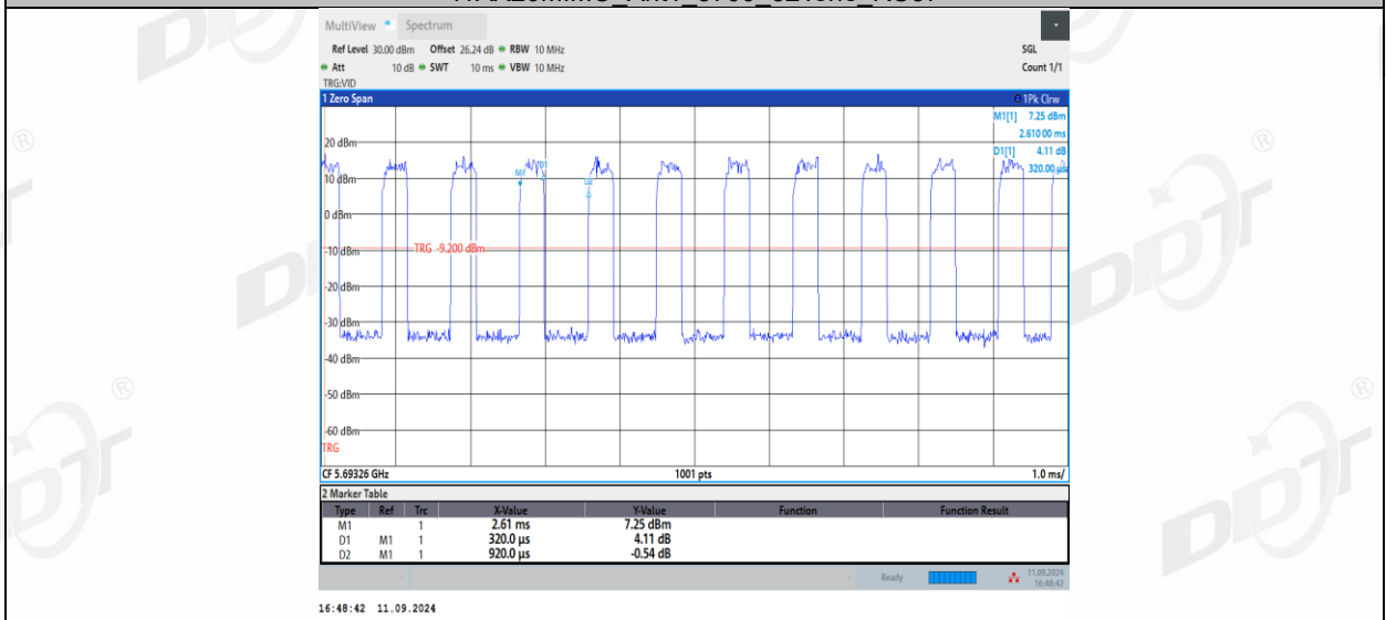
11AX20MIMO_Ant1_5700_52Tone_RU39
