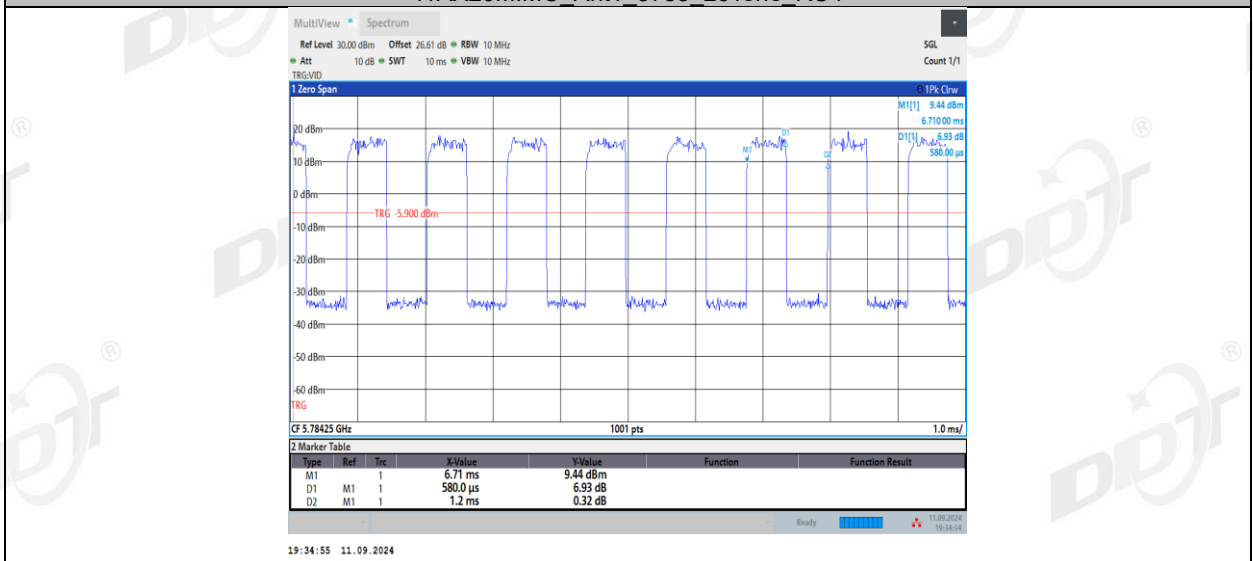
11AX20MIMO_Ant1_5785_26Tone_RU8
