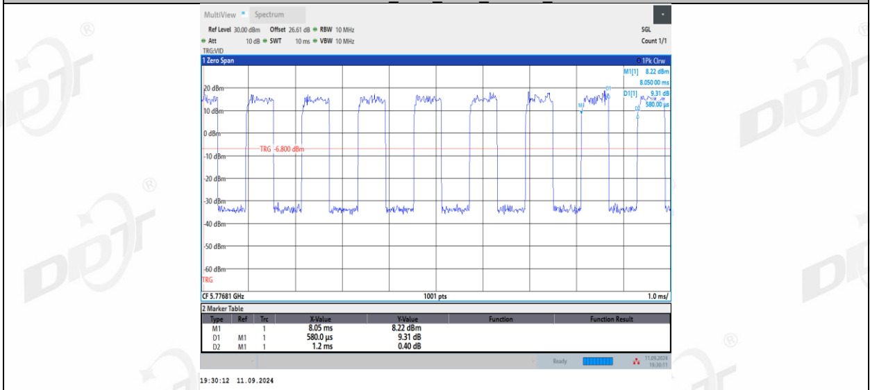
11AX20MIMO_Ant1_5785_26Tone_RU4
