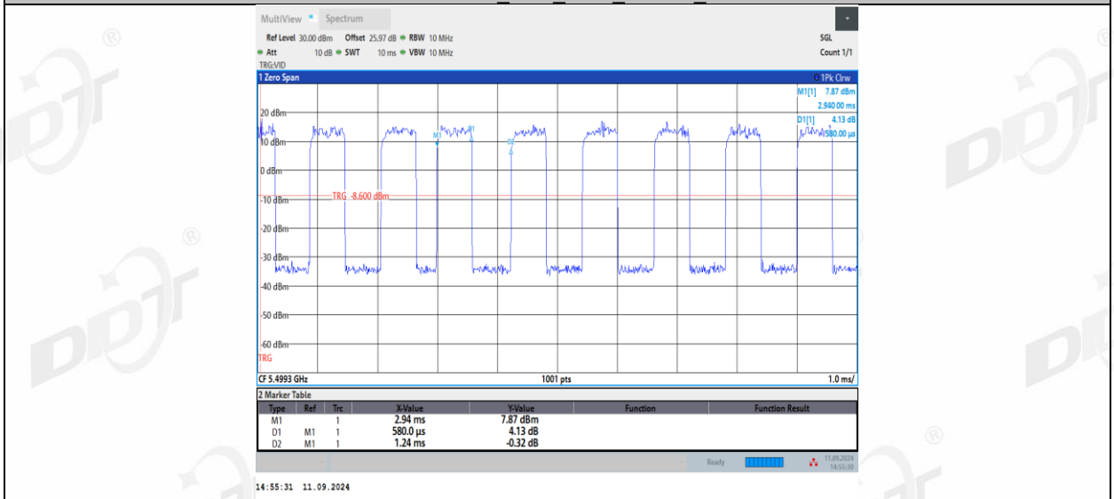
11AX20MIMO_Ant1_5500_26Tone_RU8
