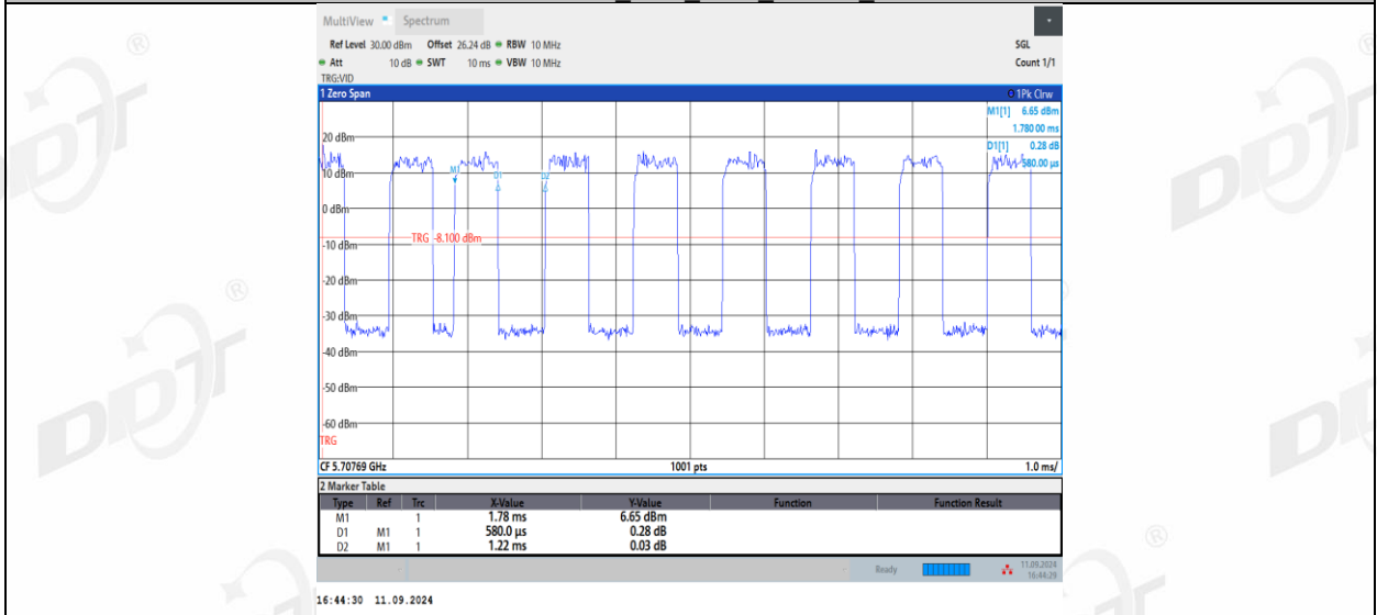
11AX20MIMO_Ant1_5700_52Tone_RU37
