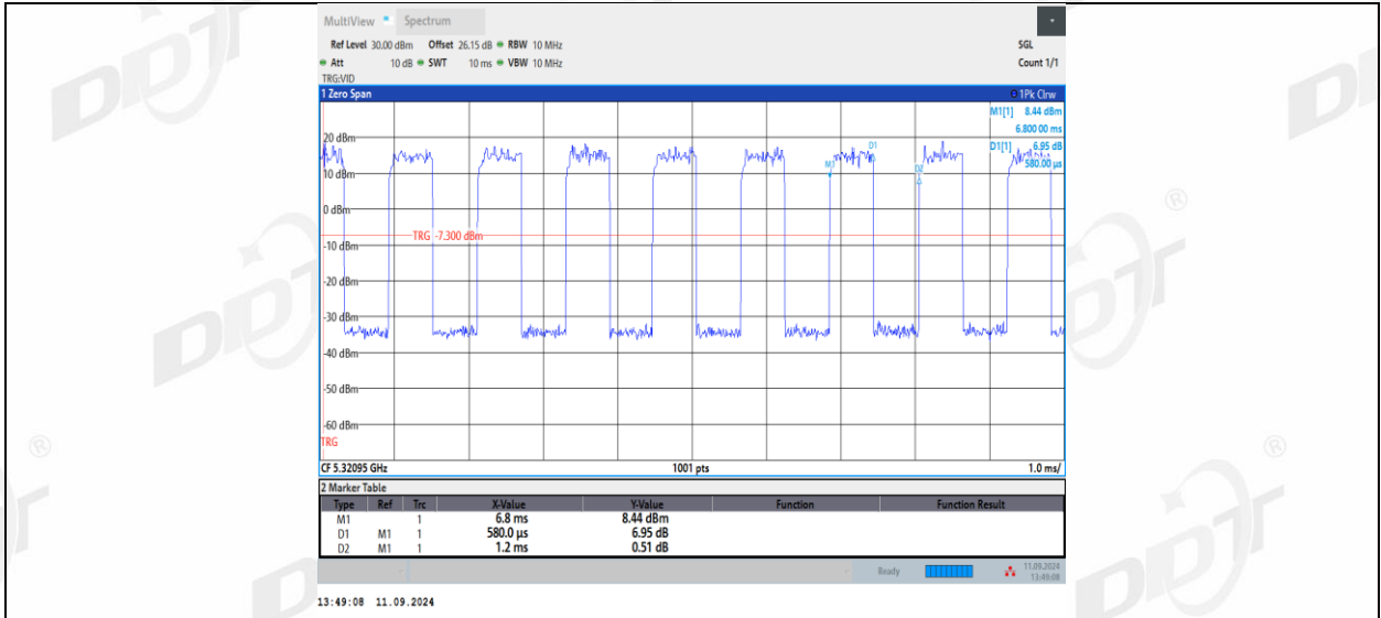
11AX20MIMO_Ant1_5320_26Tone_RU8
