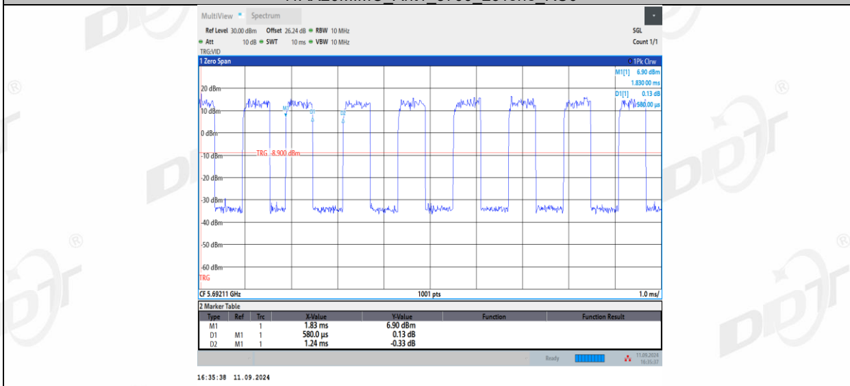
11AX20MIMO_Ant1_5700_26Tone_RU4
