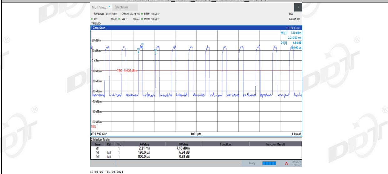
11AX20MIMO_Ant1_5700_106Tone_RU54
