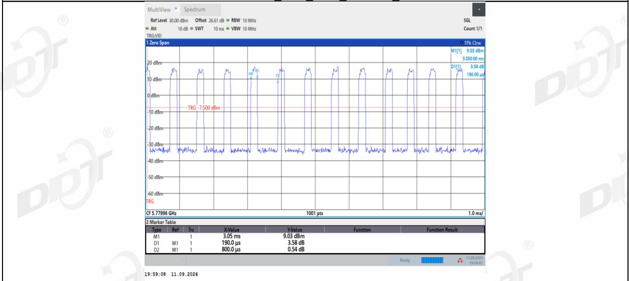
11AX20MIMO_Ant1_5785_106Tone_RU54
