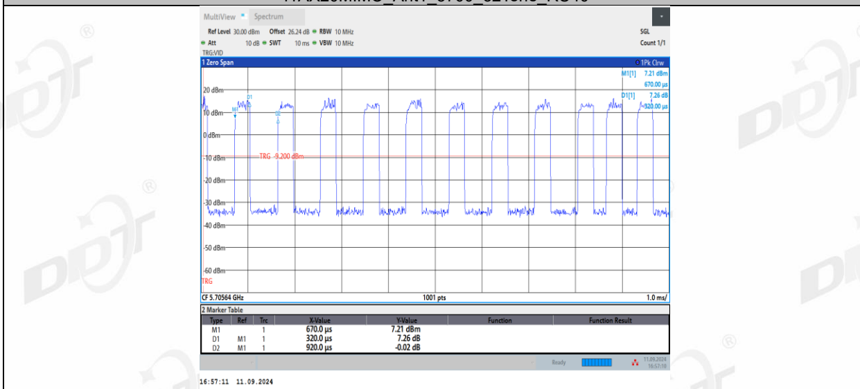
11AX20MIMO_Ant1_5700_106Tone_RU53
