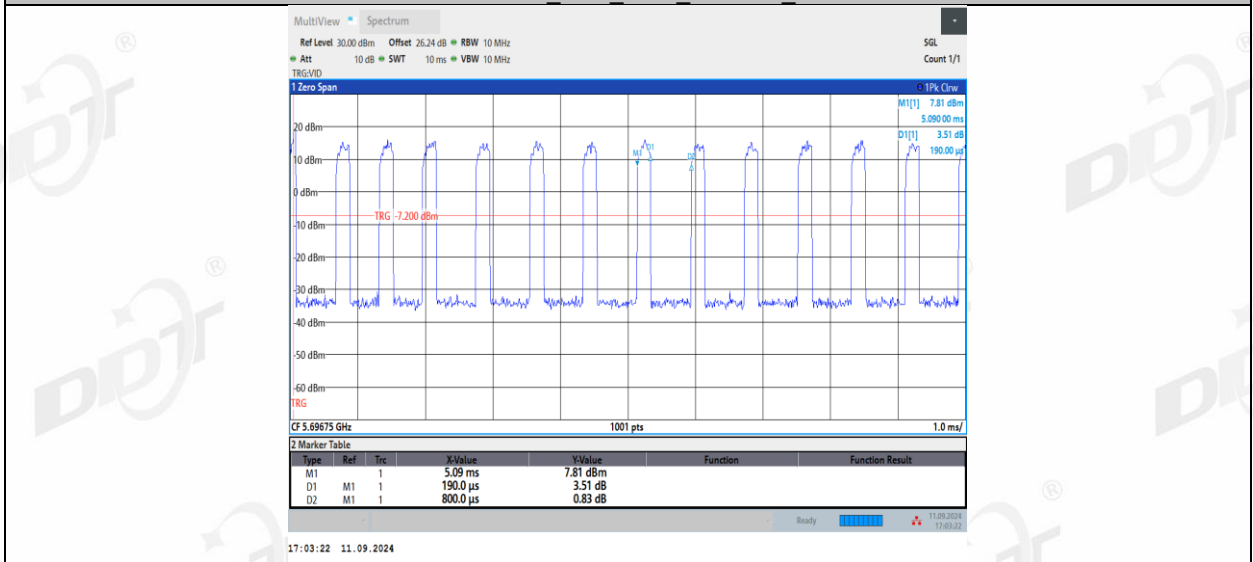
11AX20MIMO_Ant2_5700_106Tone_RU54
