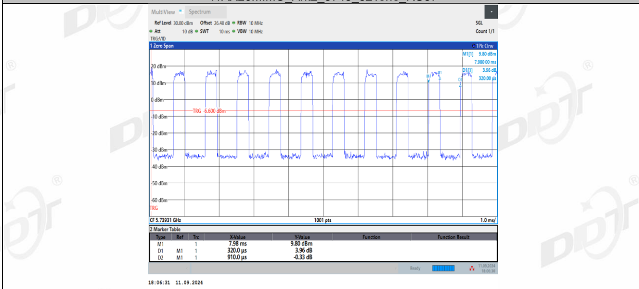
11AX20MIMO_Ant2_5745_52Tone_RU37
