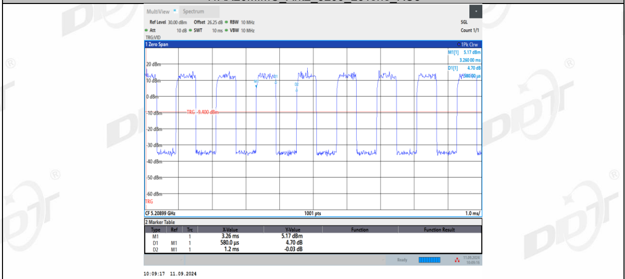
11AX20MIMO_Ant2_5200_52Tone_RU37
