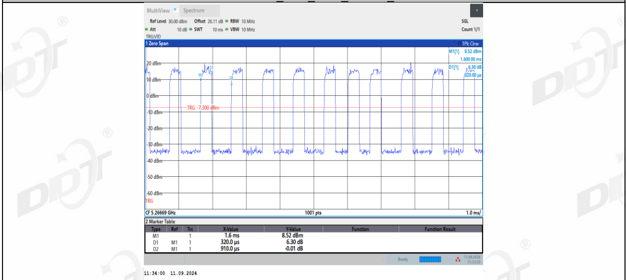
11AX20MIMO_Ant2_5260_106Tone_RU53
