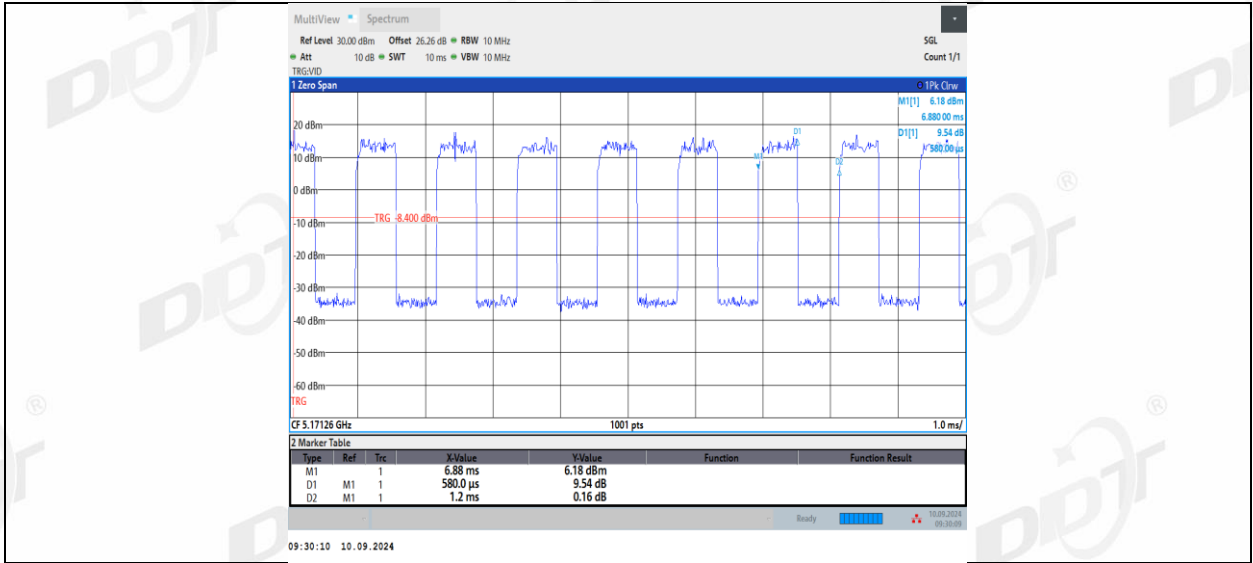
11AX20MIMO_Ant1_5180_26Tone_RU4
