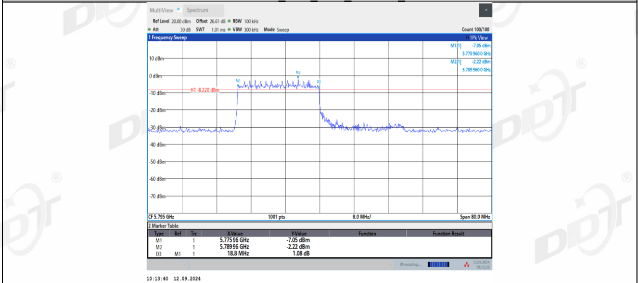
11AX40MIMO_Ant2_5795_242Tone_RU62
