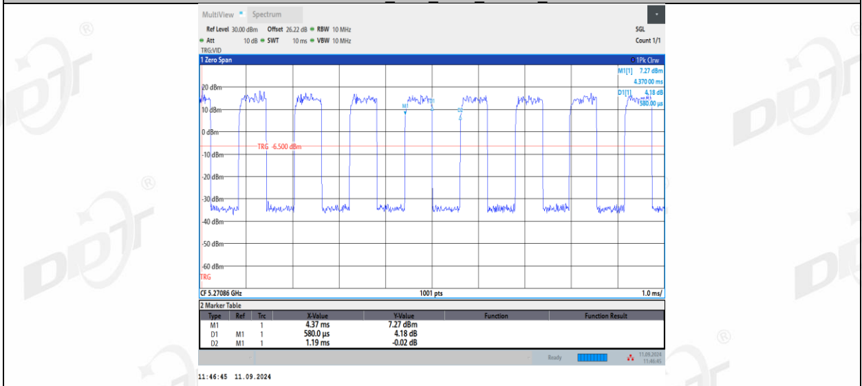
11AX20MIMO_Ant1_5280_26Tone_RU4
