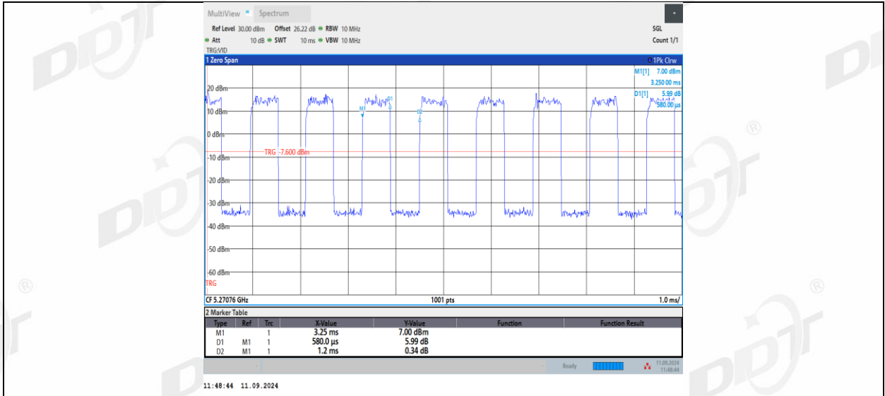
11AX20MIMO_Ant2_5280_26Tone_RU4
