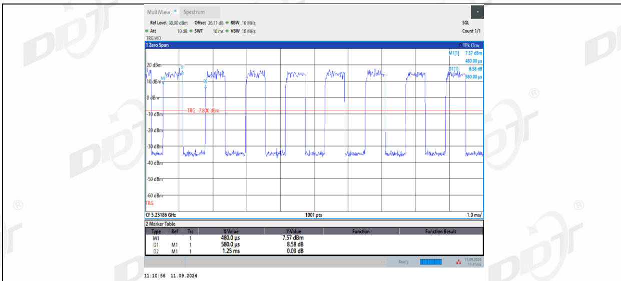
11AX20MIMO_Ant1_5260_26Tone_RU4
