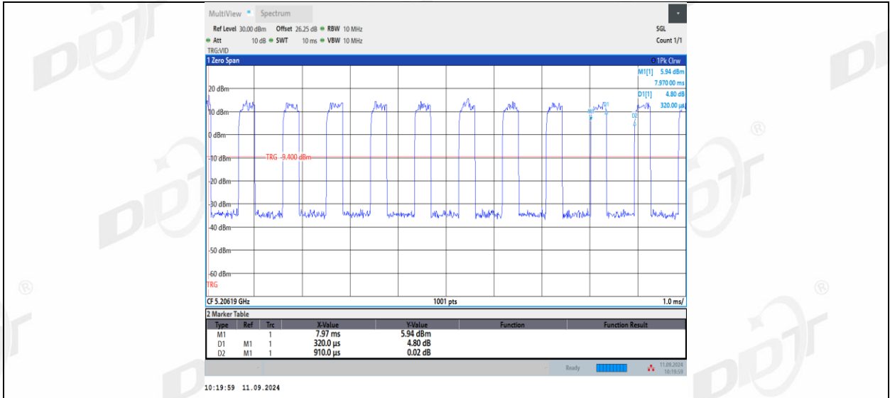
11AX20MIMO_Ant1_5200_106Tone_RU53
