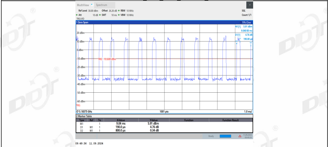
11AX20MIMO_Ant2_5180_26Tone_RU0
