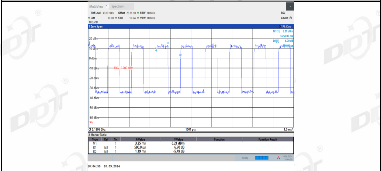
11AX20MIMO_Ant1_5180_26Tone_RU5
