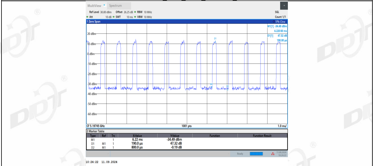
11AX20MIMO_Ant1_5200_106Tone_RU54
