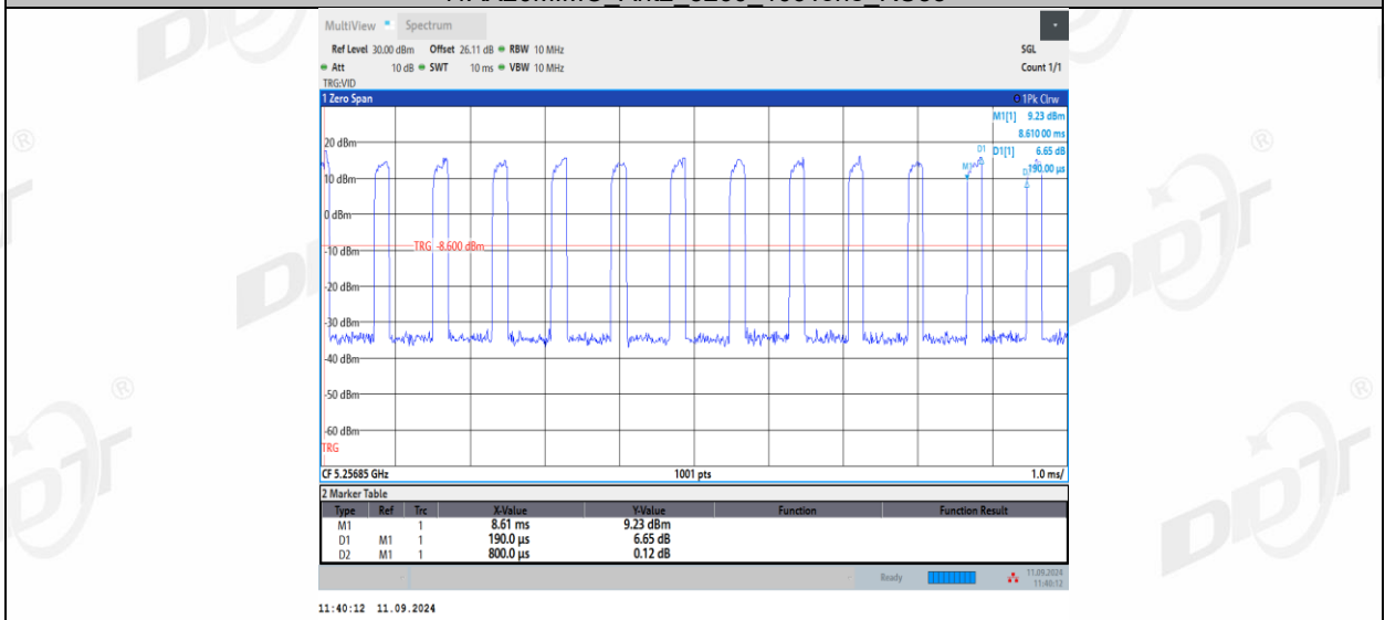
11AX20MIMO_Ant2_5260_106Tone_RU54
