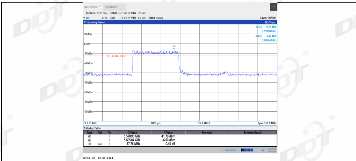
11AX80MIMO_Ant2_5610_484Tone_RU66
