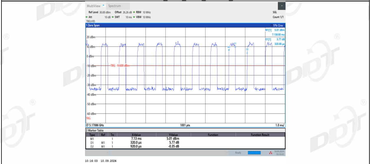
11AX20MIMO_Ant2_5180_52Tone_RU39
