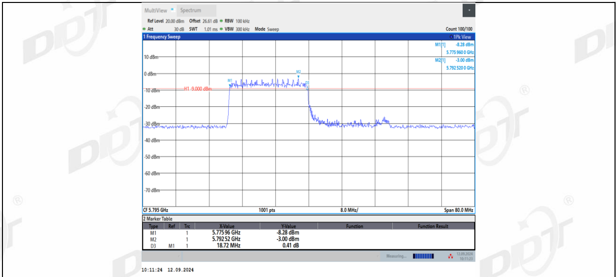
11AX40MIMO_Ant1_5795_242Tone_RU62
