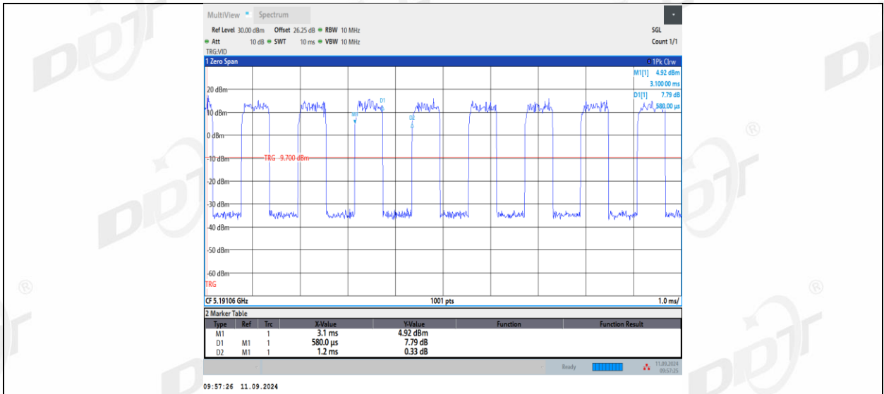
11AX20MIMO_Ant2_5200_26Tone_RU4
