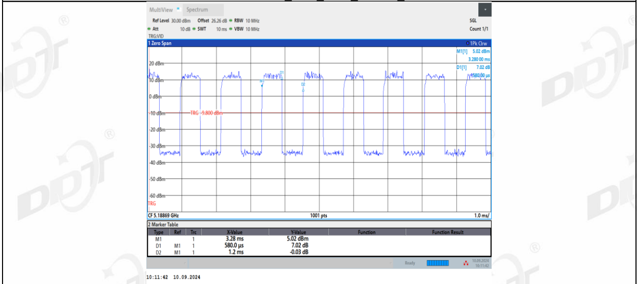
11AX20MIMO_Ant2_5180_52Tone_RU37
