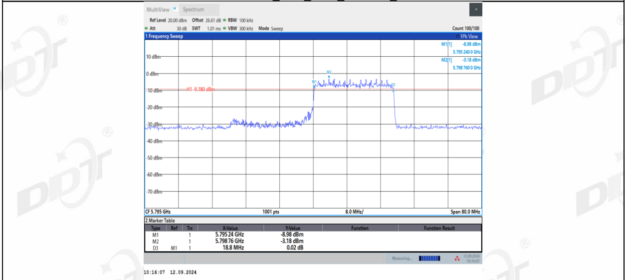
11AX40MIMO_Ant2_5795_242Tone_RU61
