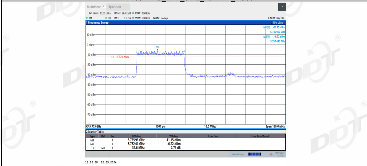
11AX80MIMO_Ant1_5775_484Tone_RU66
