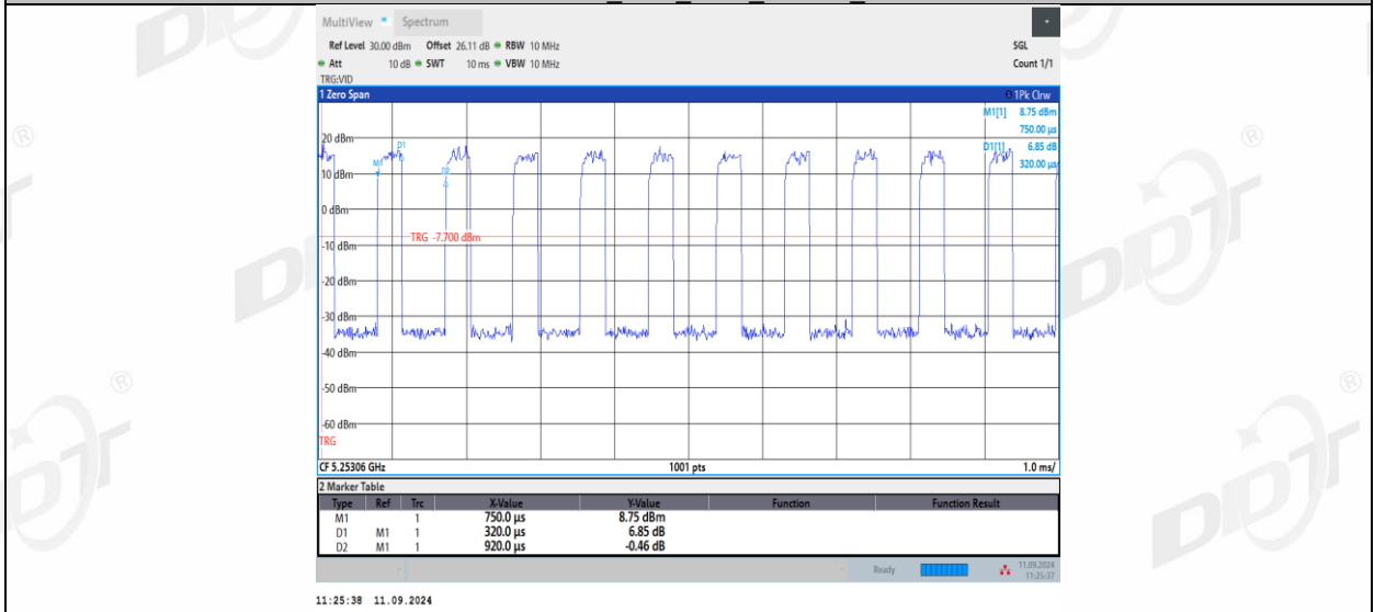
11AX20MIMO_Ant2_5260_52Tone_RU39
