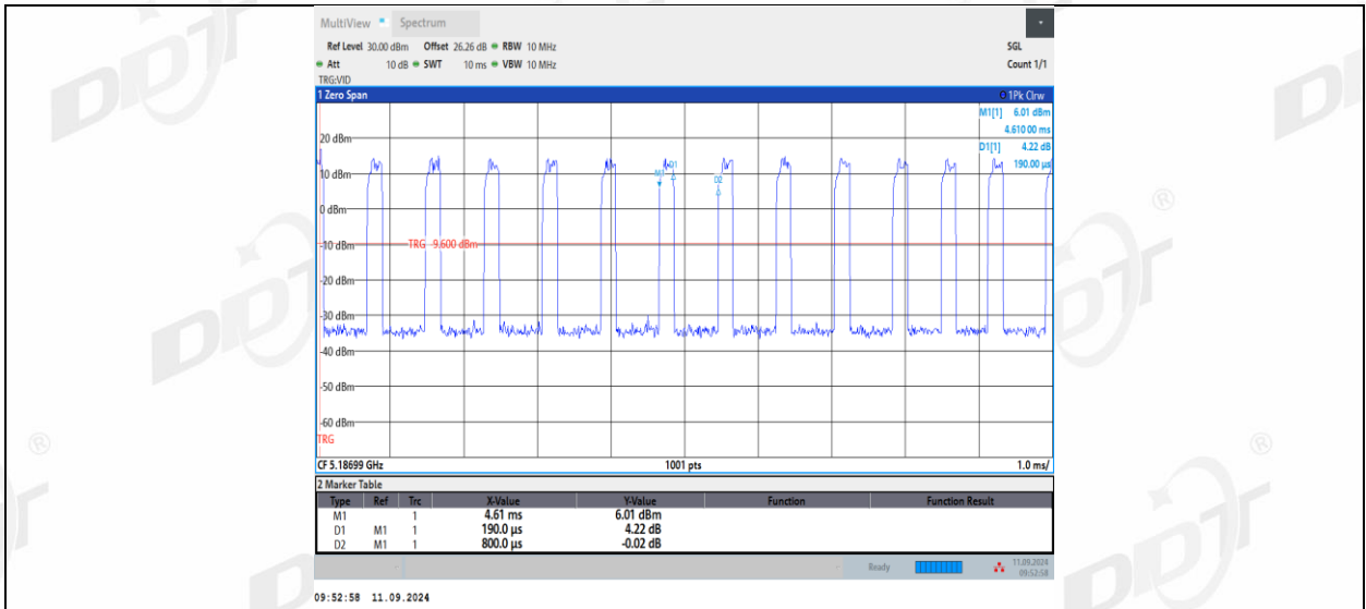
11AX20MIMO_Ant1_5200_26Tone_RU0
