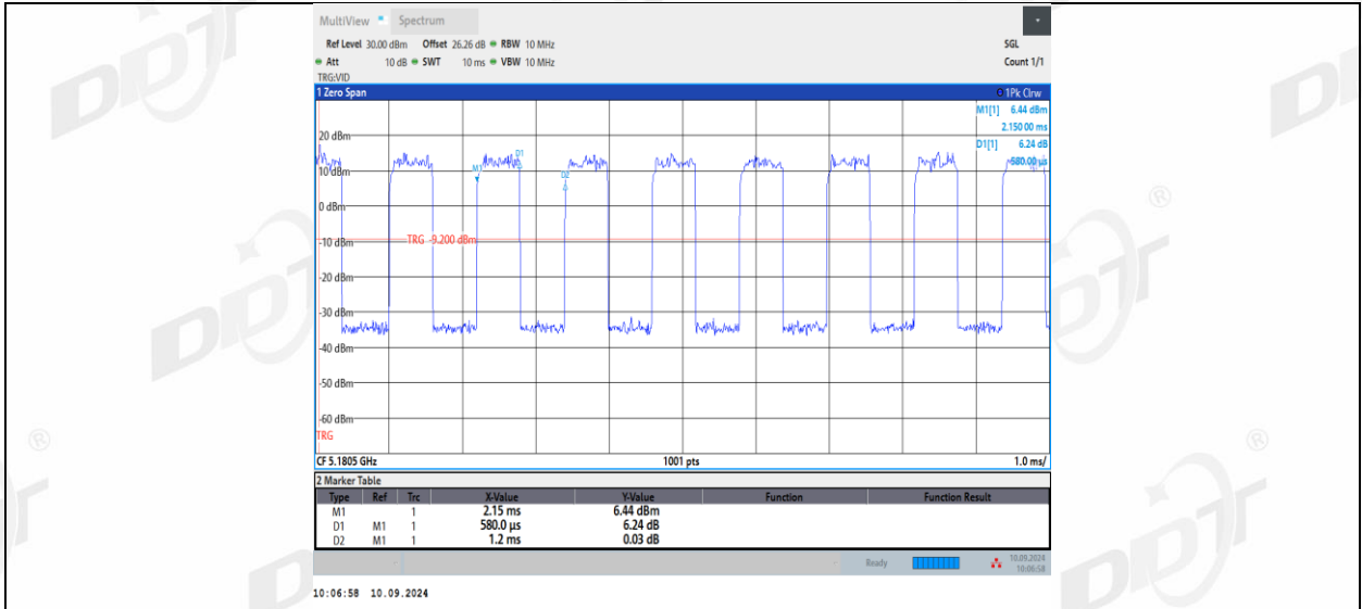
11AX20MIMO_Ant2_5180_26Tone_RU8
