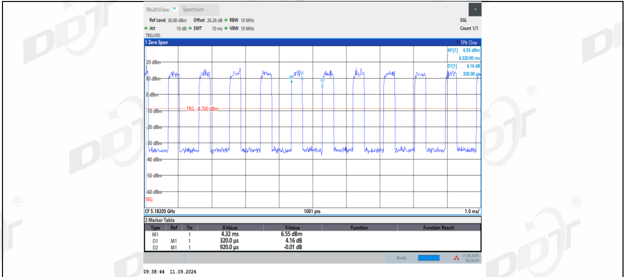
11AX20MIMO_Ant2_5180_52Tone_RU40
