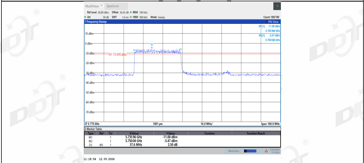
11AX80MIMO_Ant2_5775_484Tone_RU66
