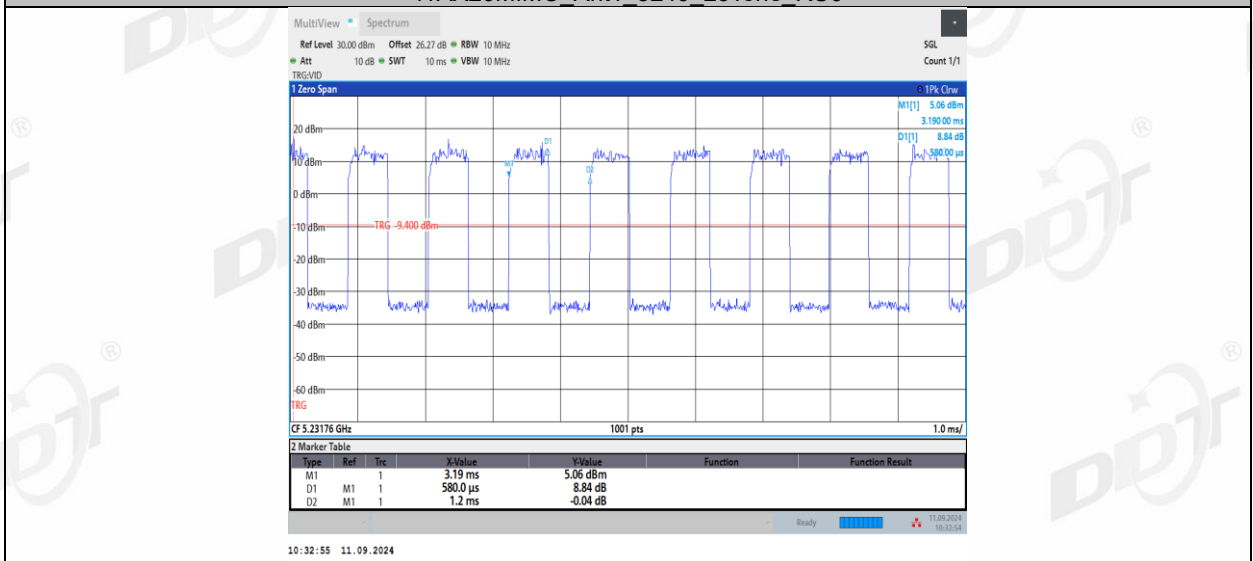
11AX20MIMO_Ant1_5240_26Tone_RU4
