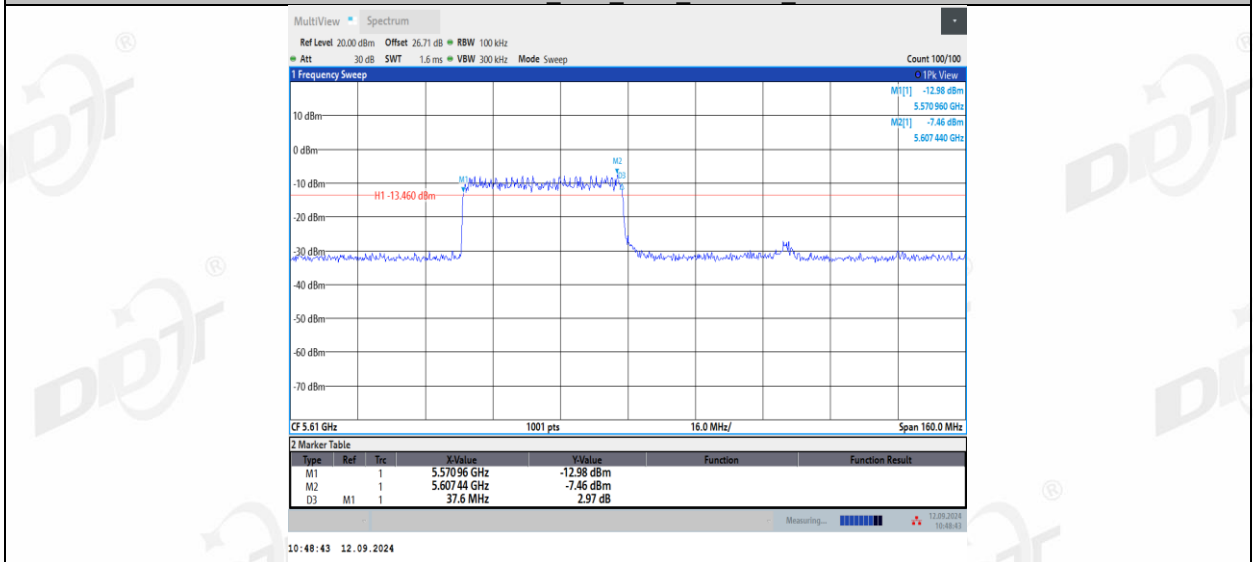
11AX80MIMO_Ant1_5610_484Tone_RU66
