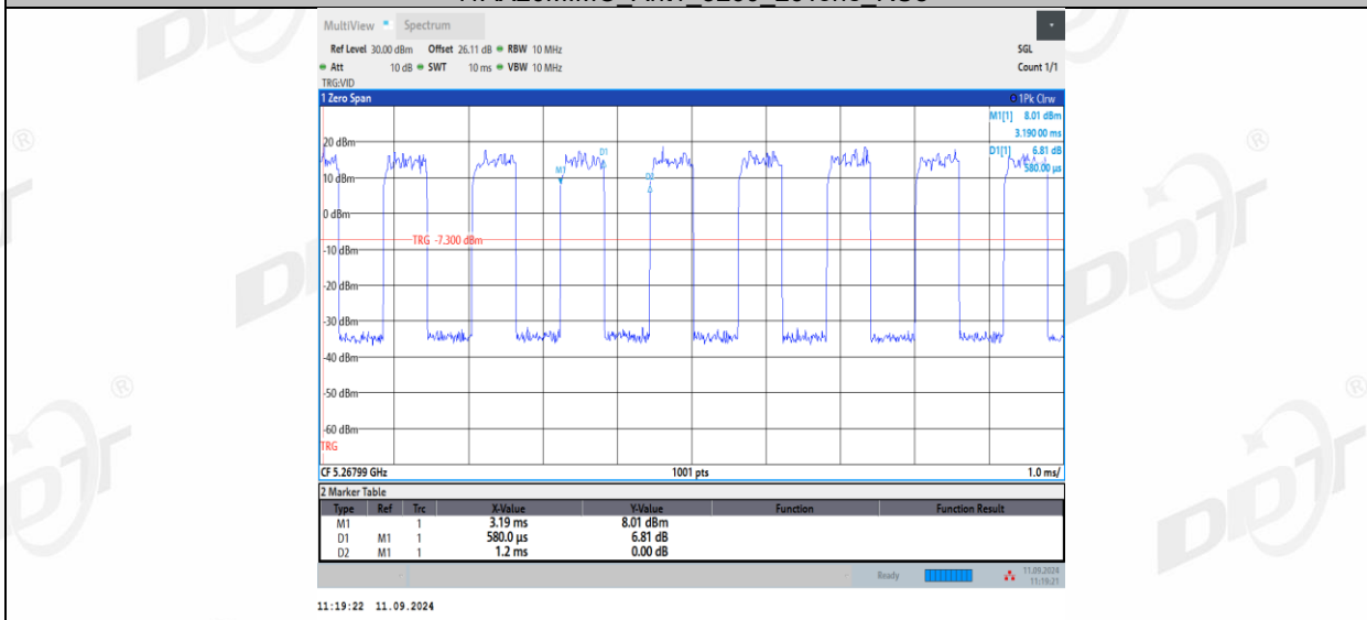
11AX20MIMO_Ant1_5260_52Tone_RU37
