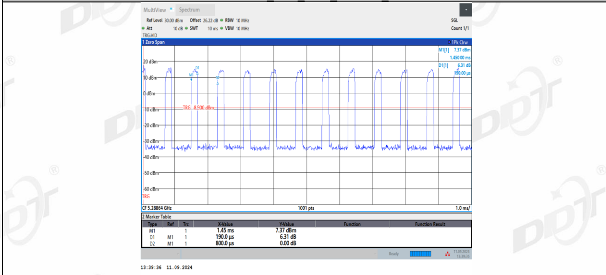
11AX20MIMO_Ant2_5280_26Tone_RU0
