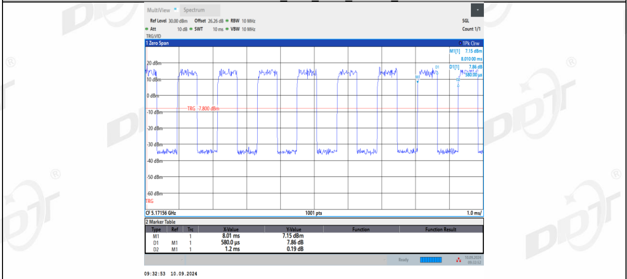
11AX20MIMO_Ant2_5180_26Tone_RU4
