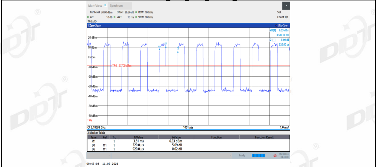
11AX20MIMO_Ant2_5180_106Tone_RU53
