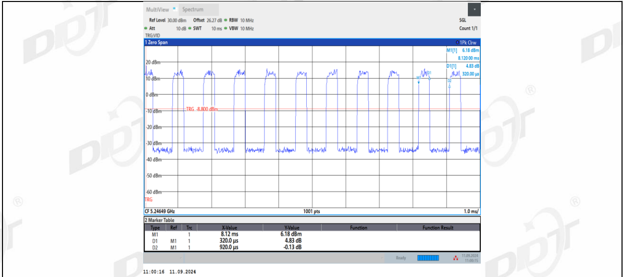
11AX20MIMO_Ant2_5240_106Tone_RU53
