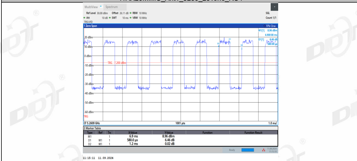
11AX20MIMO_Ant1_5260_26Tone_RU5
