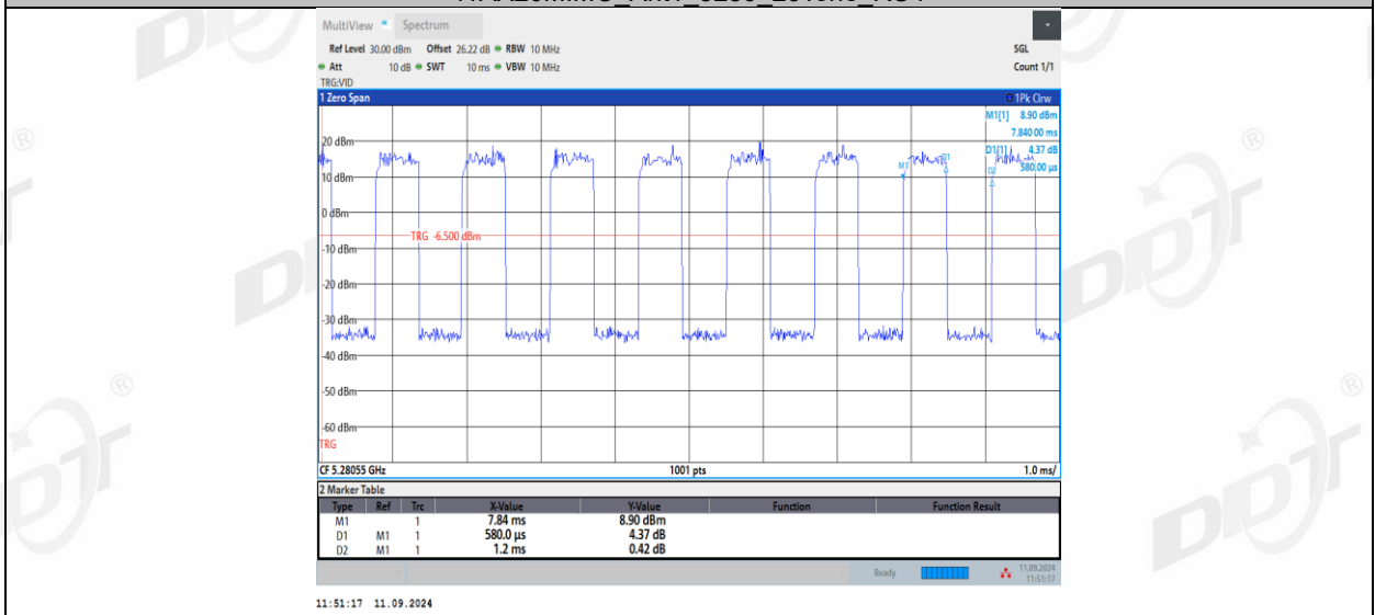
11AX20MIMO_Ant1_5280_26Tone_RU8
