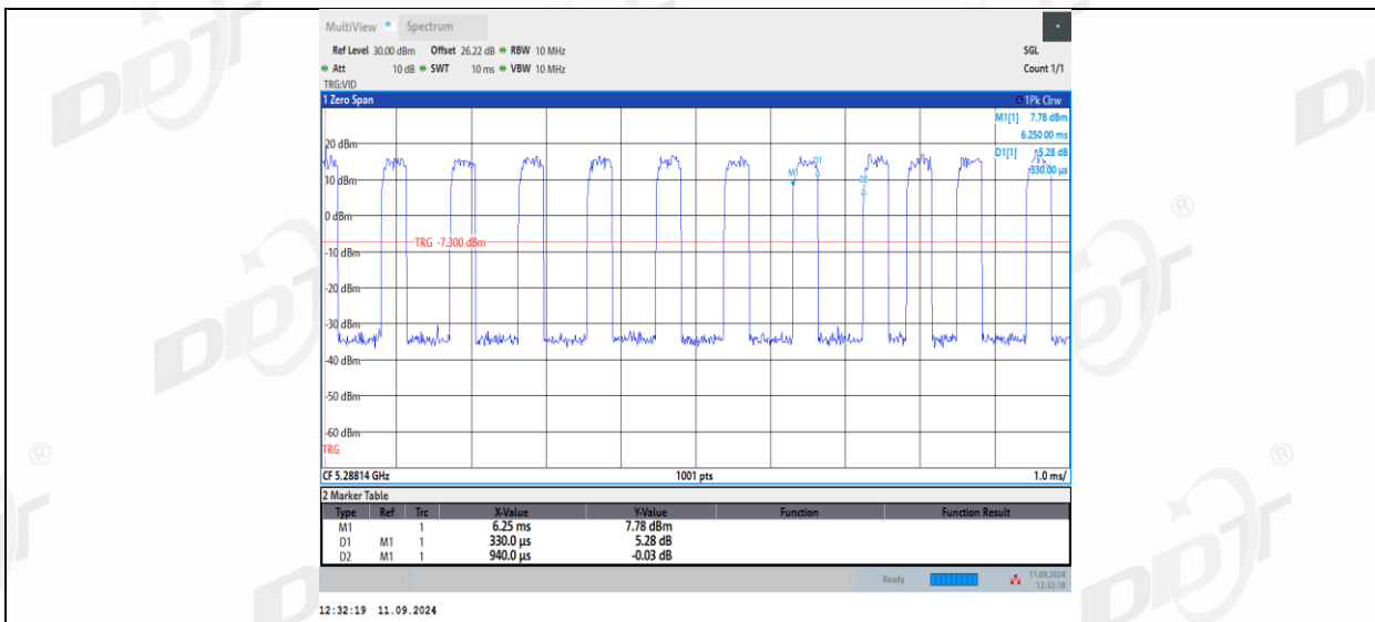
11AX20MIMO_Ant1_5280_106Tone_RU53
