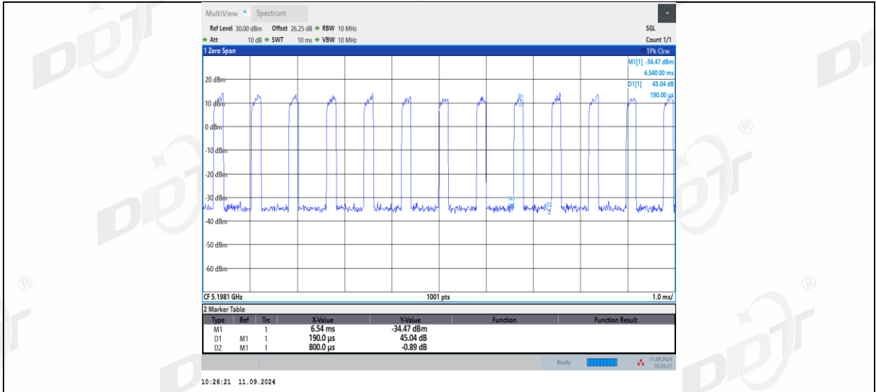
11AX20MIMO_Ant2_5200_106Tone_RU54
