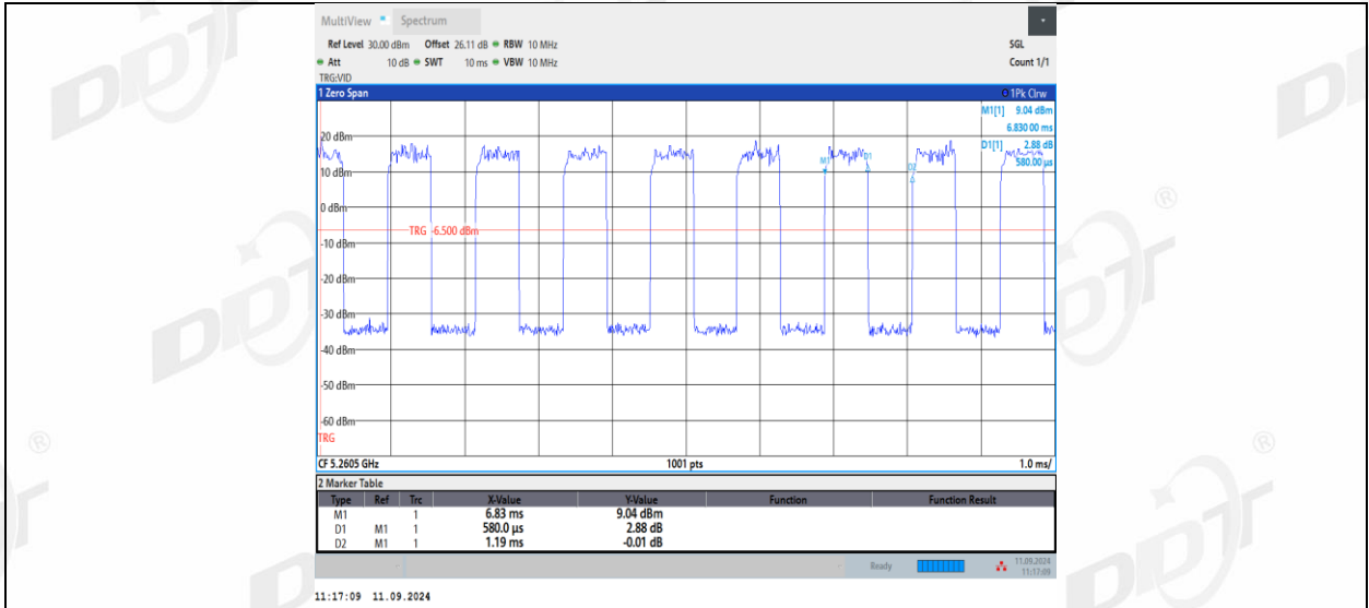
11AX20MIMO_Ant2_5260_26Tone_RU8
