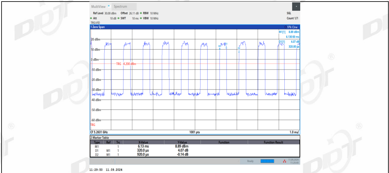
11AX20MIMO_Ant2_5260_52Tone_RU40
