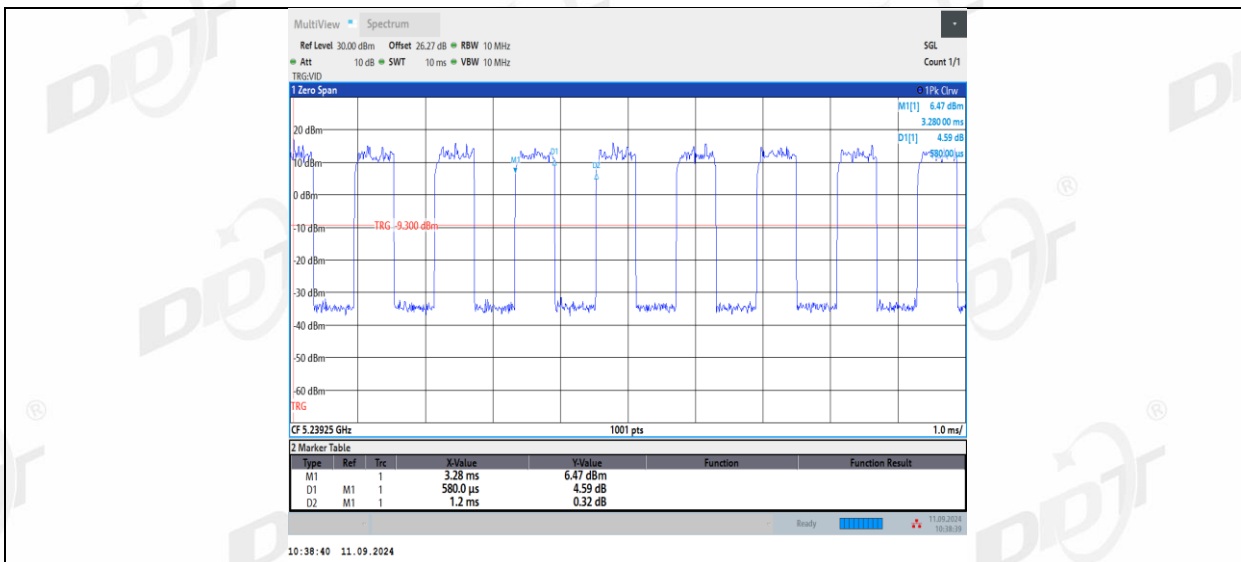
11AX20MIMO_Ant1_5240_26Tone_RU8
