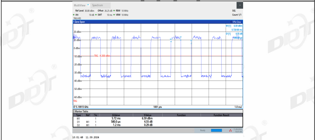
11AX20MIMO_Ant2_5200_26Tone_RU5
