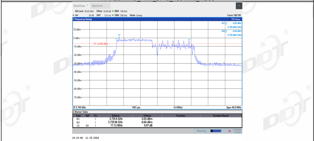
11AX20MIMO_Ant1_5745_106Tone_RU54
