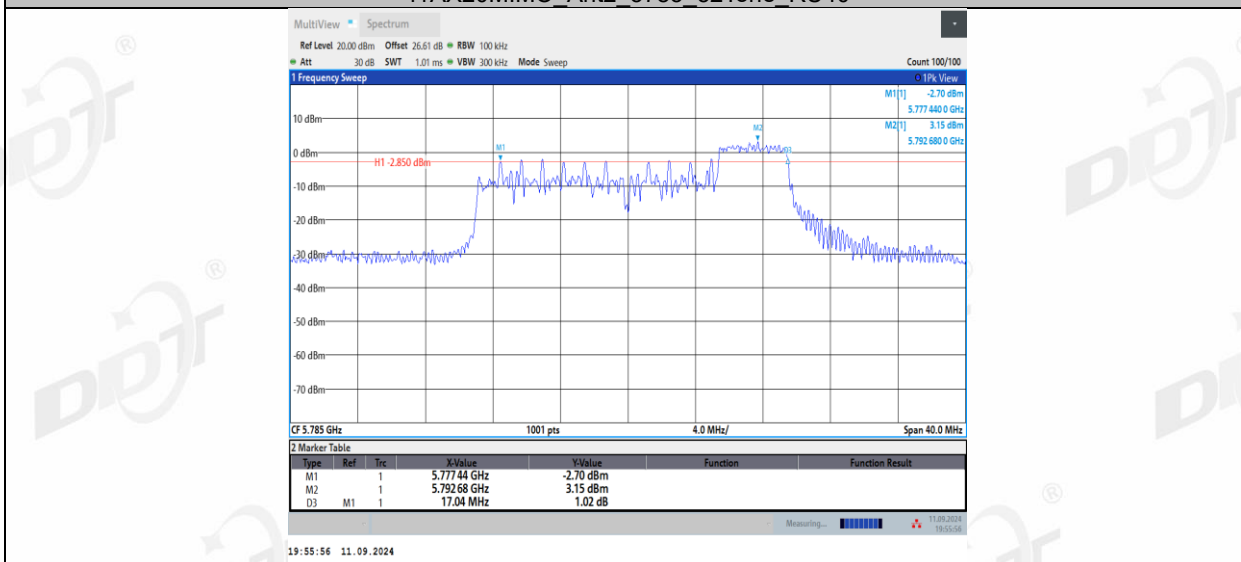
11AX20MIMO_Ant2_5785_106Tone_RU53
