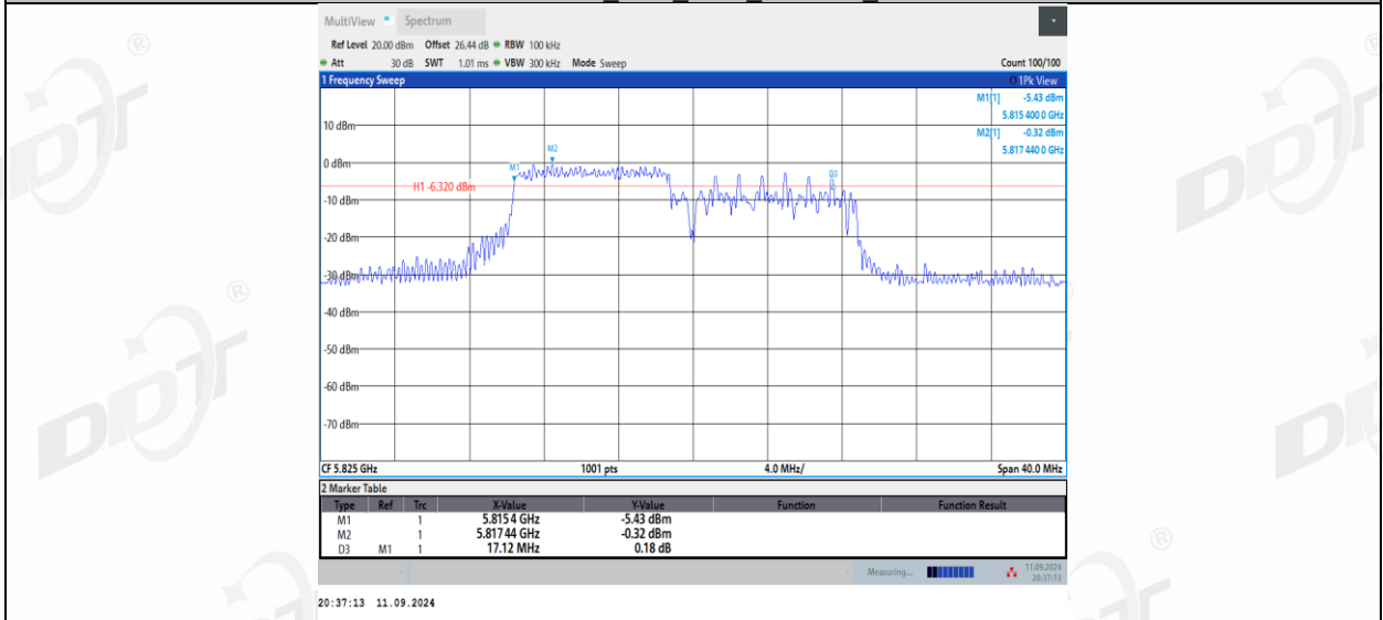
11AX20MIMO_Ant1_5825_106Tone_RU54
