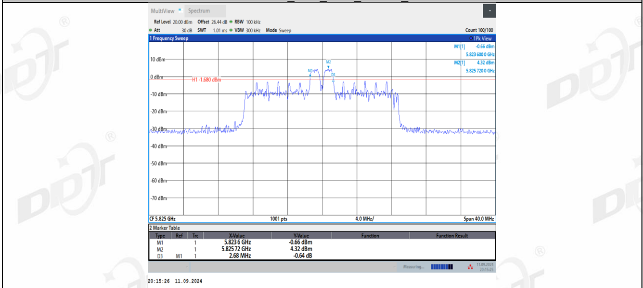
11AX20MIMO_Ant2_5825_26Tone_RU8
