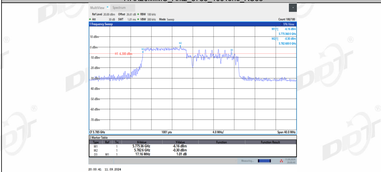
11AX20MIMO_Ant2_5785_106Tone_RU54
