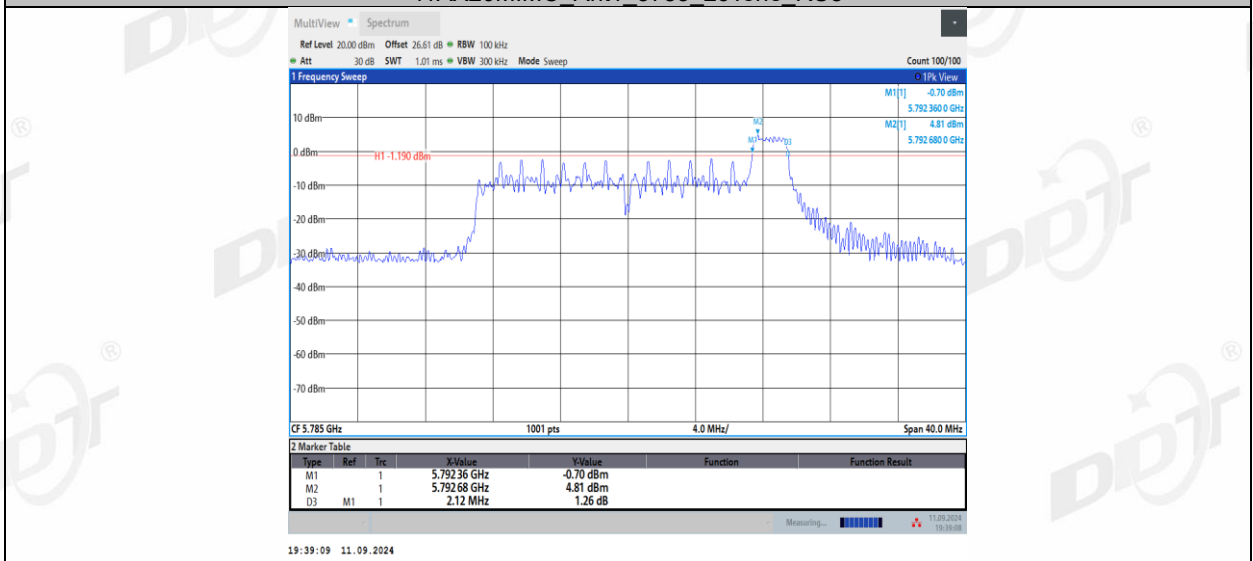
11AX20MIMO_Ant1_5785_52Tone_RU37
