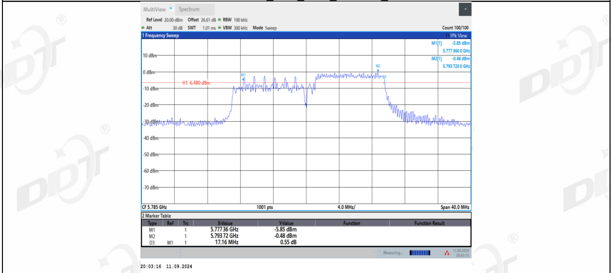
11AX20MIMO_Ant2_5785_26Tone_RU0
