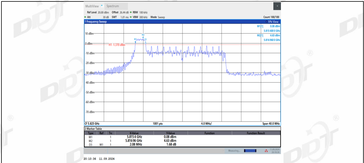
11AX20MIMO_Ant2_5825_26Tone_RU4
