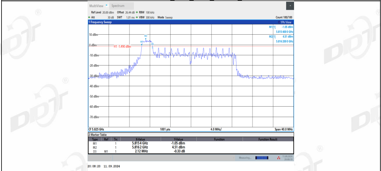
11AX20MIMO_Ant1_5825_26Tone_RU4
