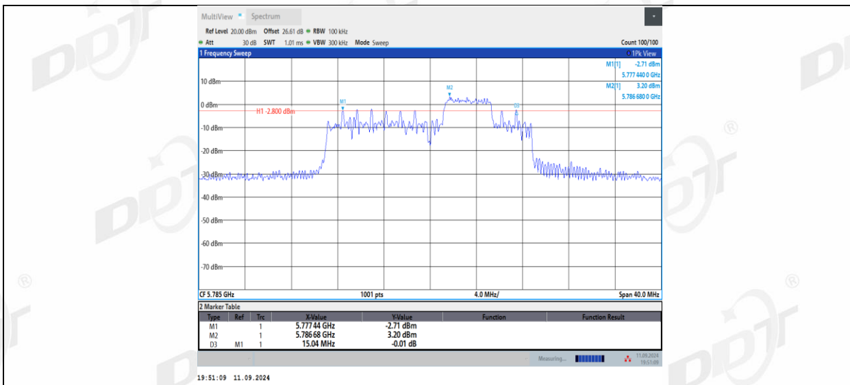
11AX20MIMO_Ant2_5785_52Tone_RU40
