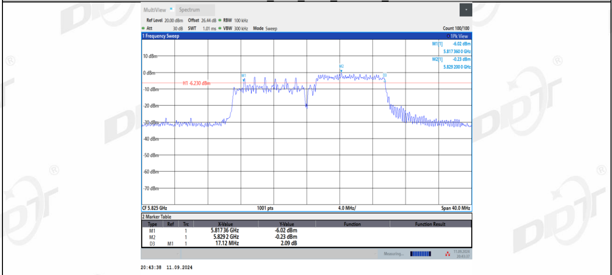
11AX20MIMO_Ant2_5825_26Tone_RU0
