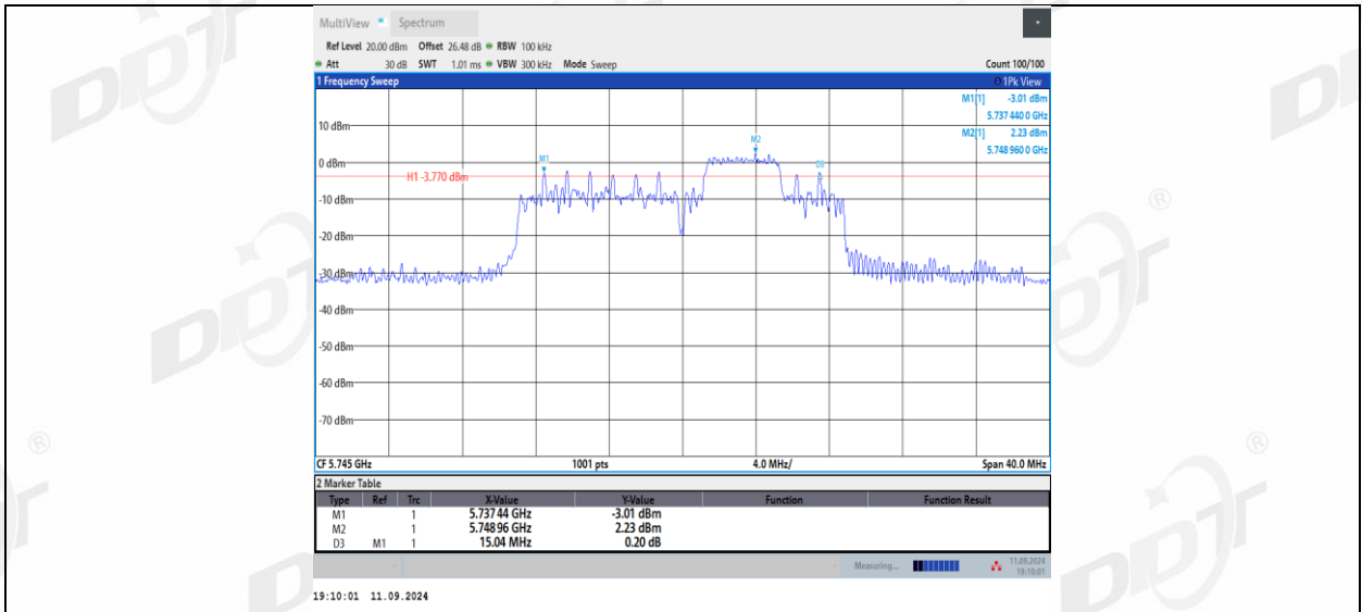
11AX20MIMO_Ant1_5745_52Tone_RU40
