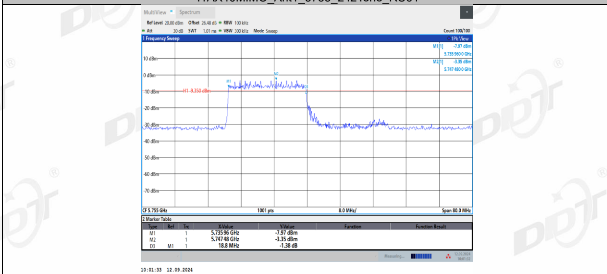
11AX40MIMO_Ant1_5755_242Tone_RU62
