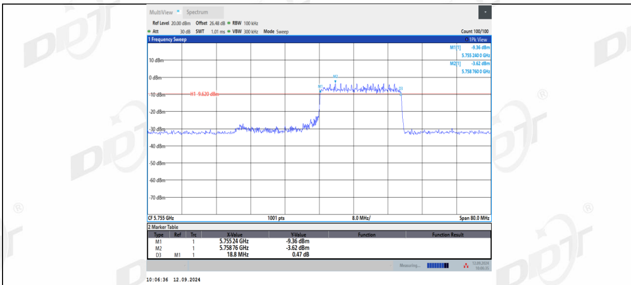
11AX40MIMO_Ant2_5755_242Tone_RU61
