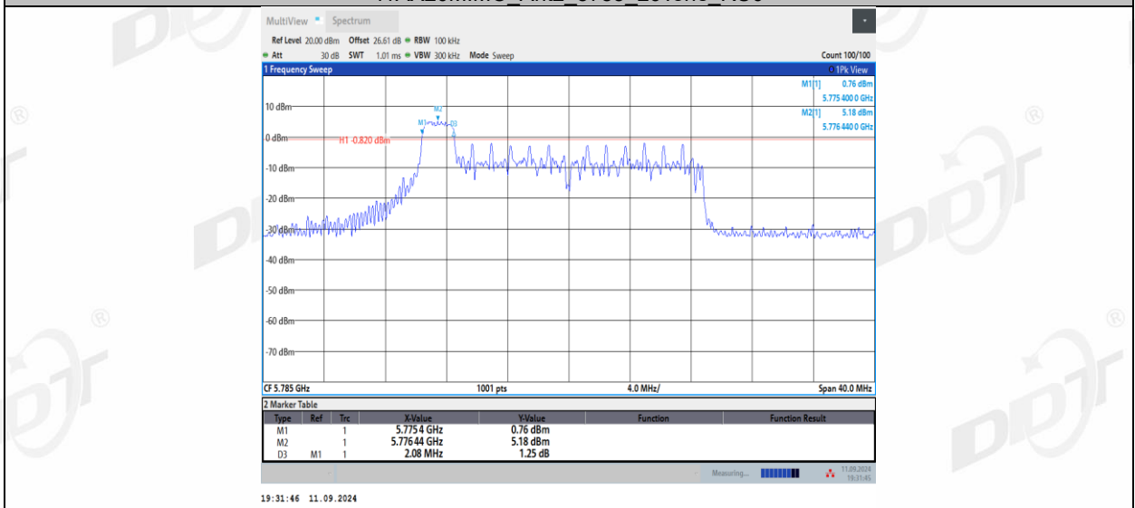
11AX20MIMO_Ant2_5785_26Tone_RU4
