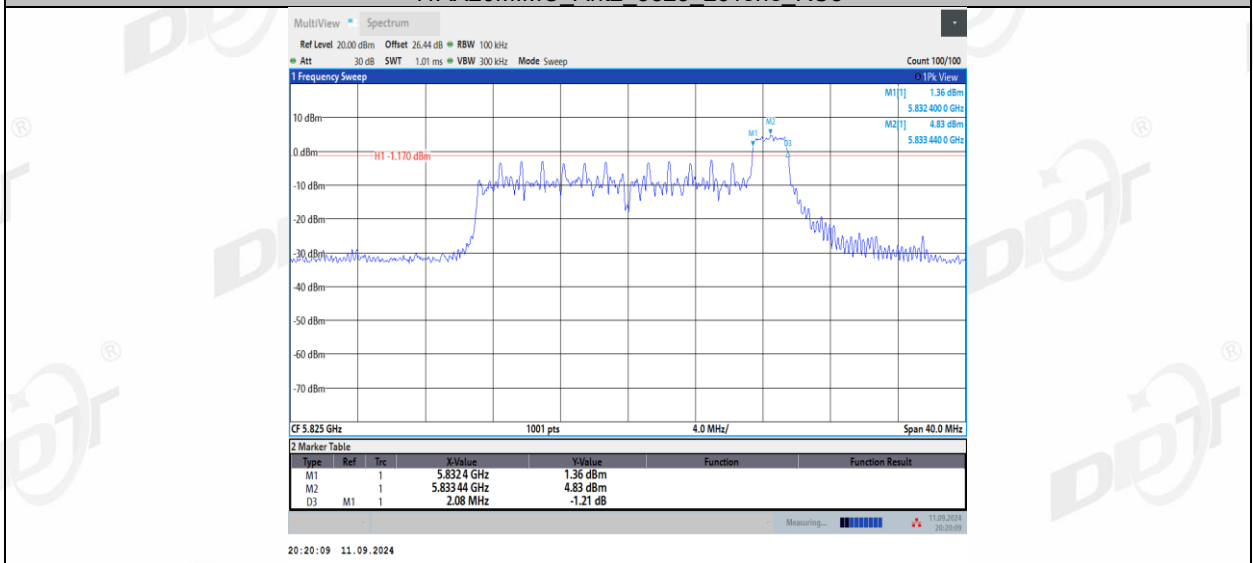
11AX20MIMO_Ant2_5825_52Tone_RU37
