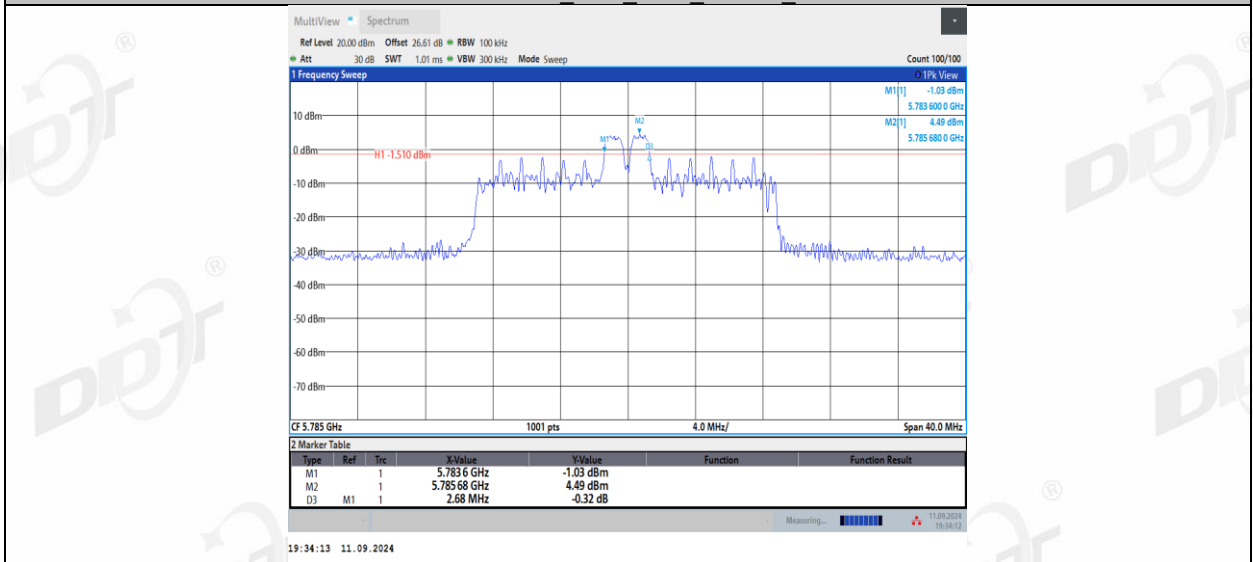
11AX20MIMO_Ant1_5785_26Tone_RU8
