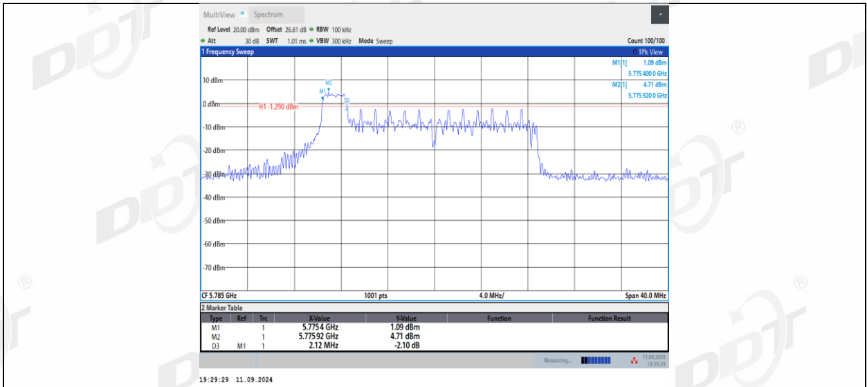
11AX20MIMO_Ant1_5785_26Tone_RU4
