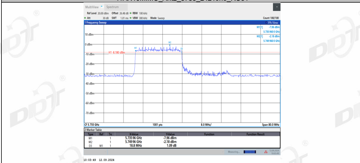
11AX40MIMO_Ant2_5755_242Tone_RU62
