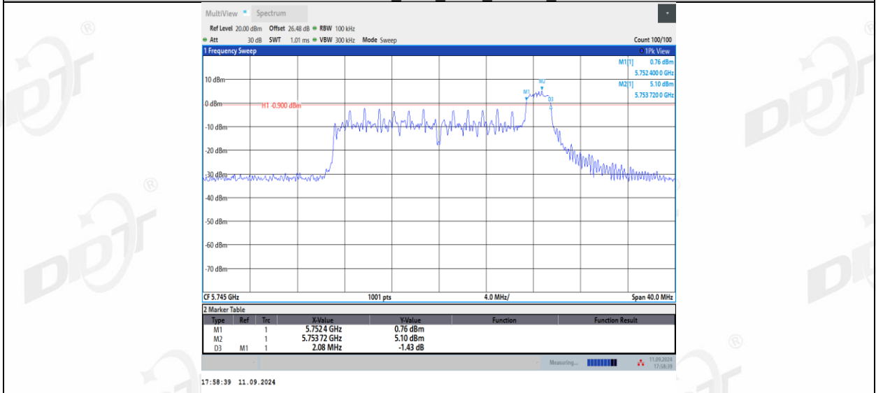
11AX20MIMO_Ant1_5745_52Tone_RU37
