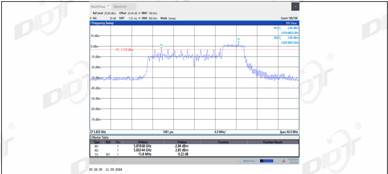
11AX20MIMO_Ant1_5825_106Tone_RU53
