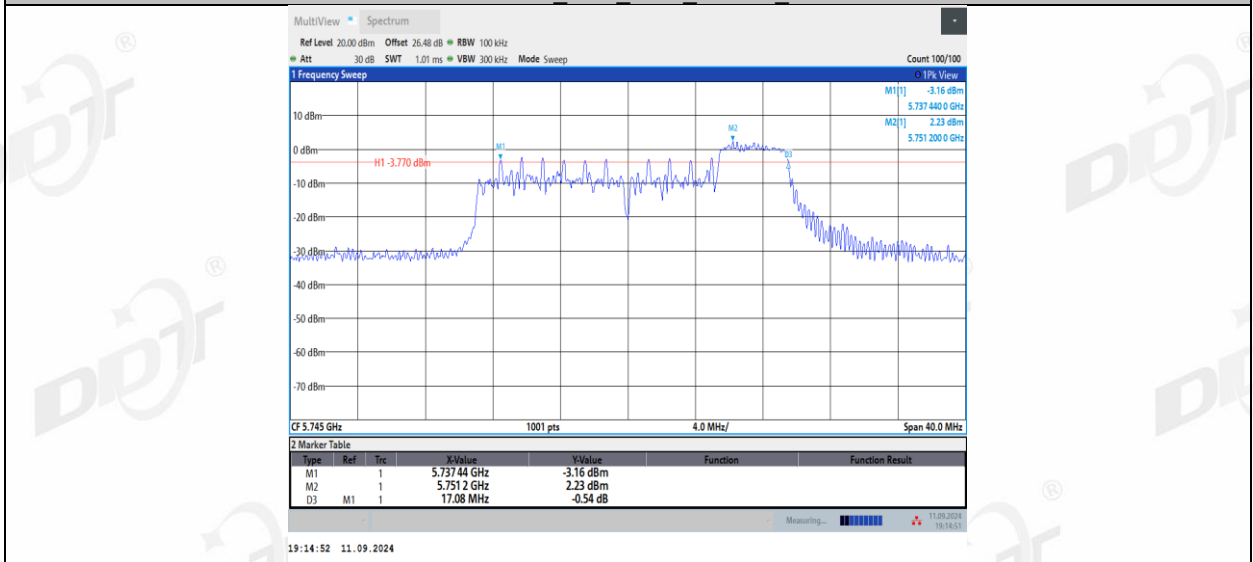
11AX20MIMO_Ant1_5745_106Tone_RU53
