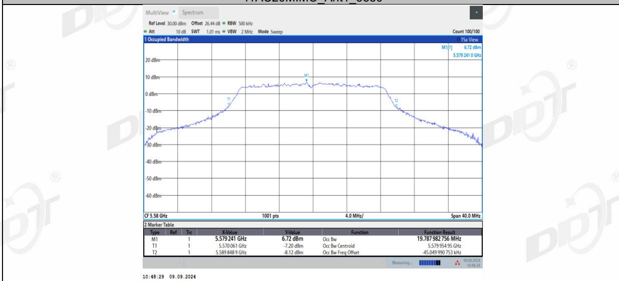
11AC20MIMO_Ant2_5580
