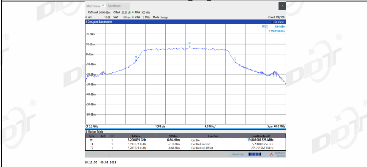
11AC20MIMO_Ant2_5200
