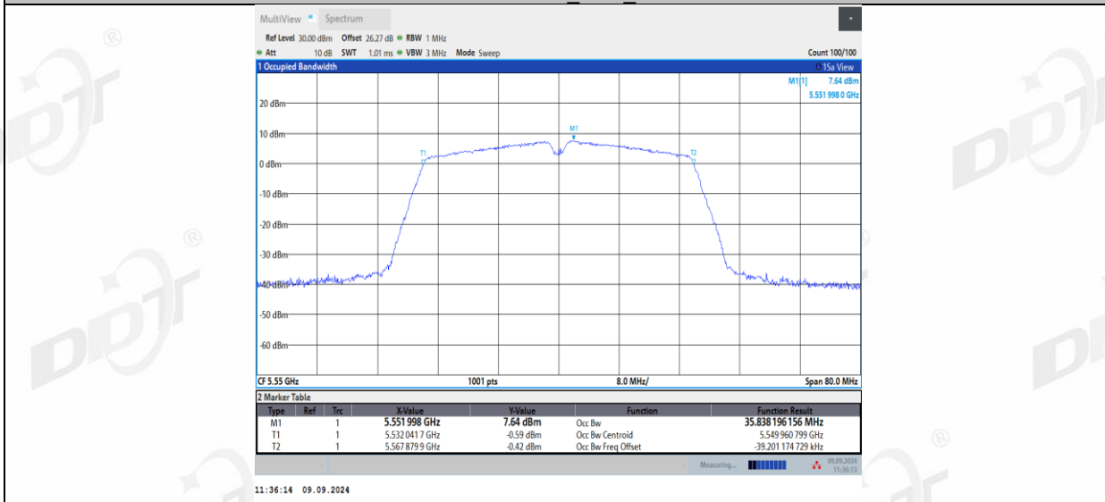
11AC40MIMO_Ant2_5550
