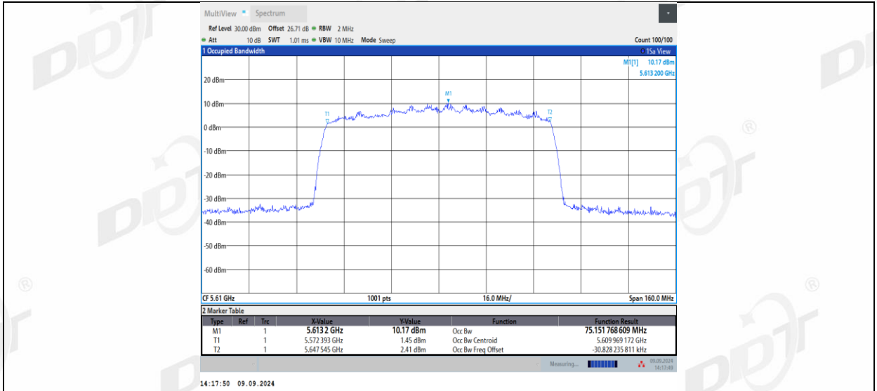
11AC80MIMO_Ant2_5610
