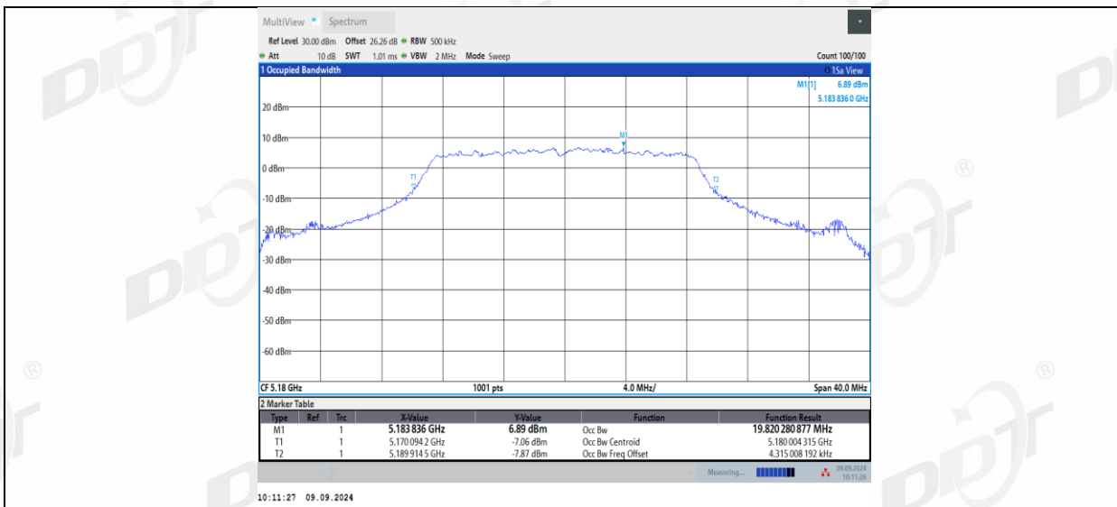
11AC20MIMO_Ant2_5180
