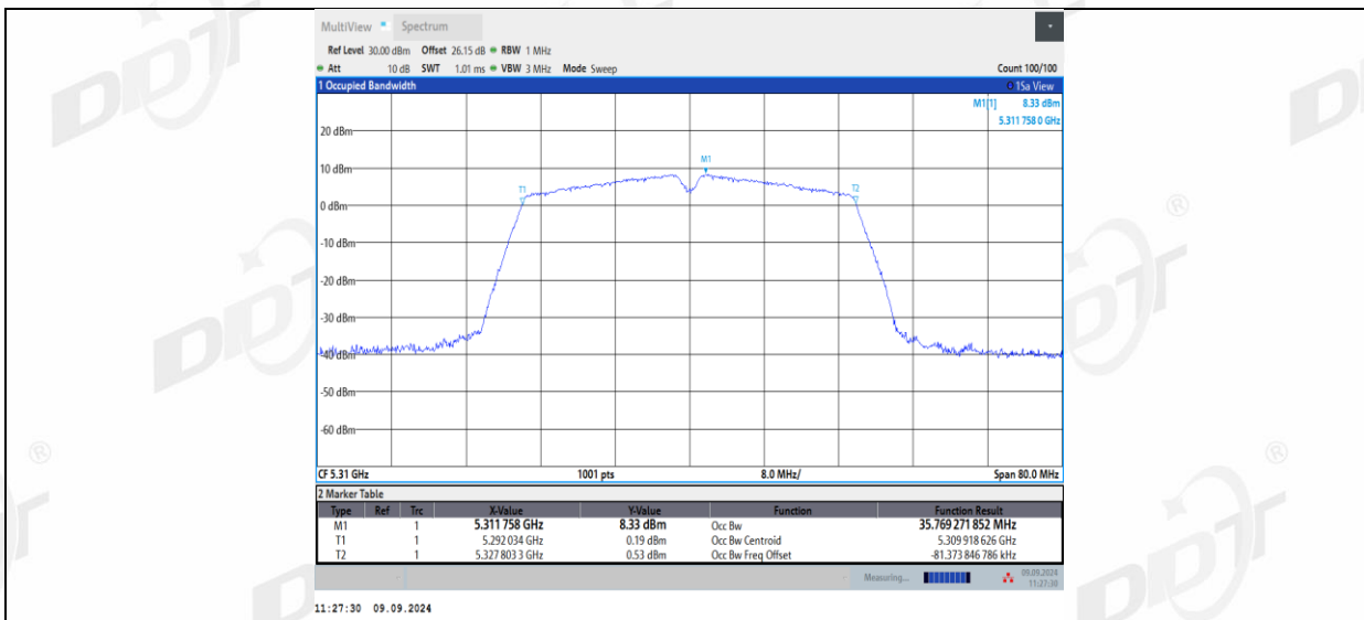
11AC40MIMO_Ant2_5310
