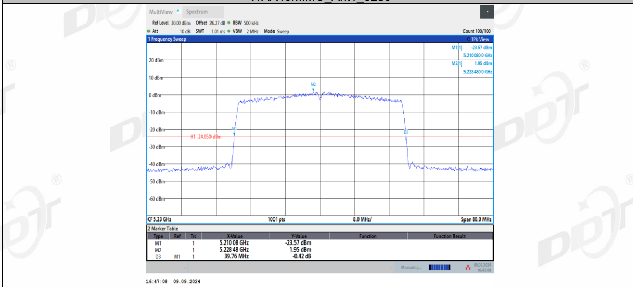
11AX40MIMO_Ant2_5230
