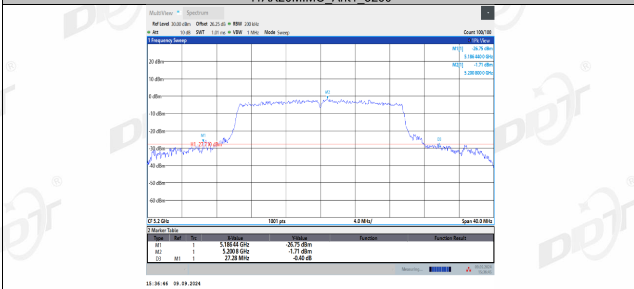
11AX20MIMO_Ant2_5200
