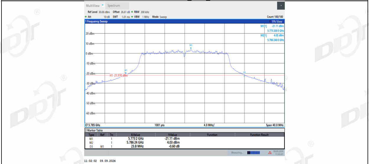
11AC20MIMO_Ant2_5785
