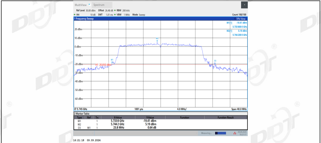
11AX20MIMO_Ant2_5745
