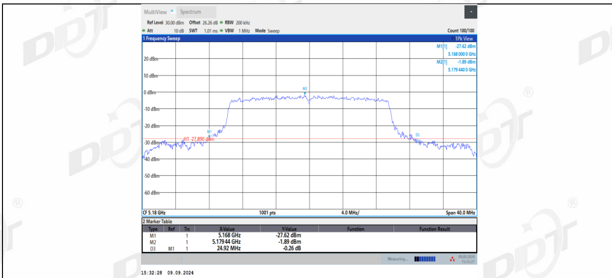
11AX20MIMO_Ant2_5180
