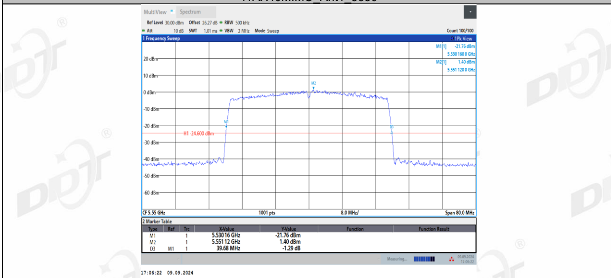
11AX40MIMO_Ant2_5550
