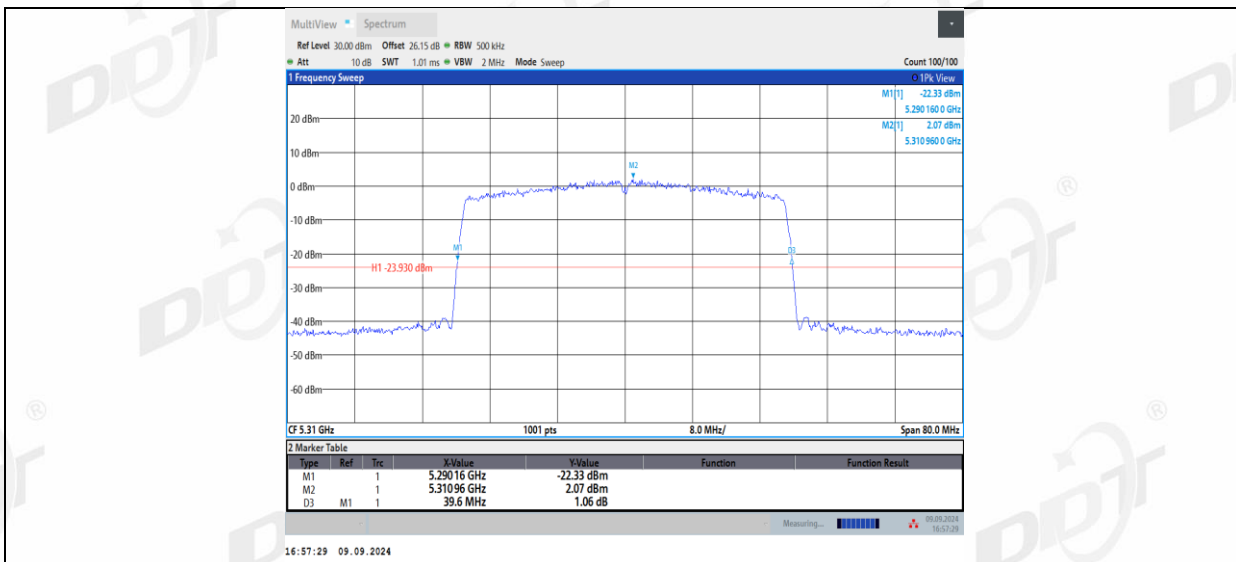
11AX40MIMO_Ant2_5310
