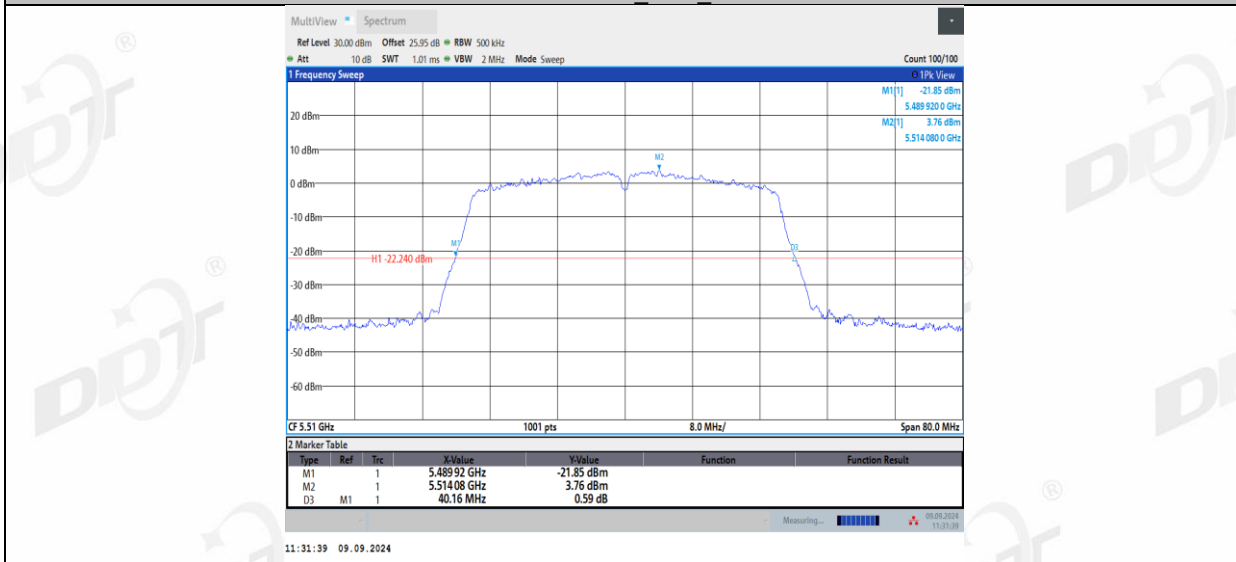
11AC40MIMO_Ant2_5510
