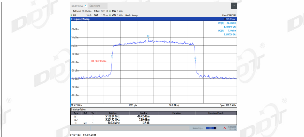
11AX80MIMO_Ant2_5210
