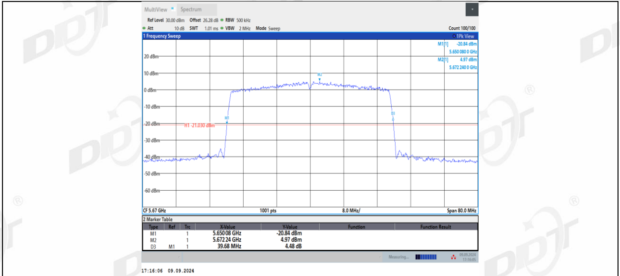
11AX40MIMO_Ant2_5670
