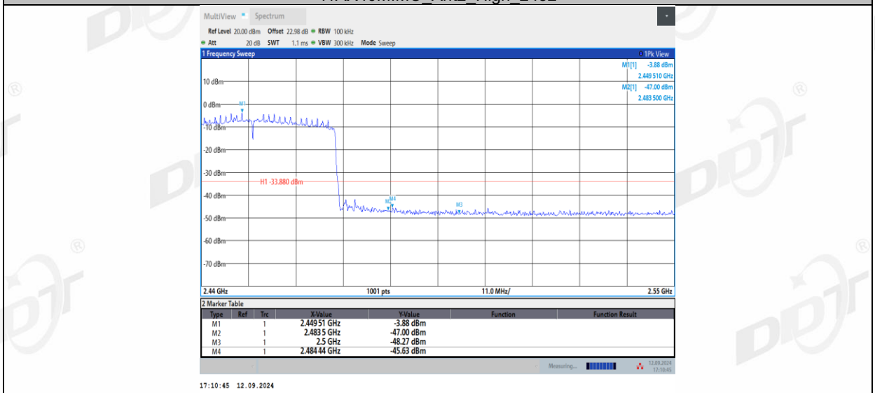
11AX40MIMO_Ant2_High_2452
