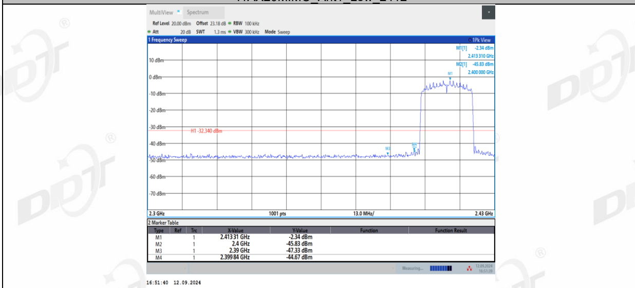
11AX20MIMO_Ant2_Low_2412
