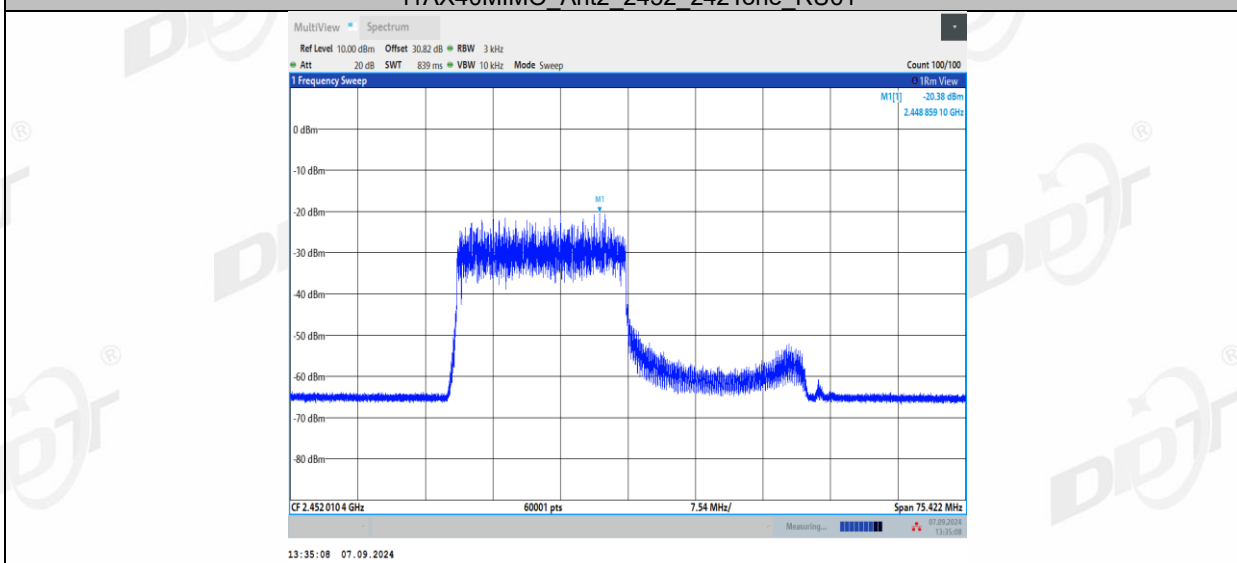
11AX40MIMO_Ant2_2452_242Tone_RU62
