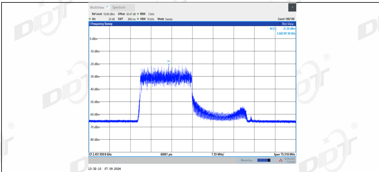
11AX40MIMO_Ant1_2452_242Tone_RU62
