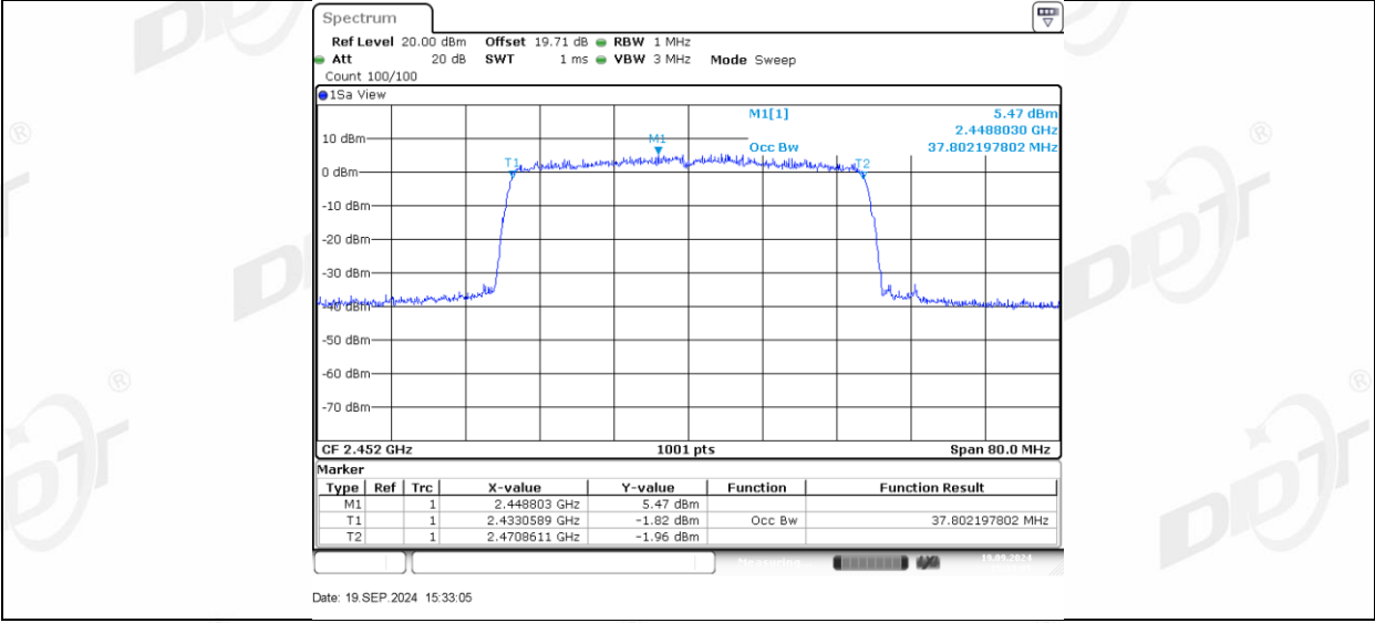
11AX40MIMO_Ant2_2452
