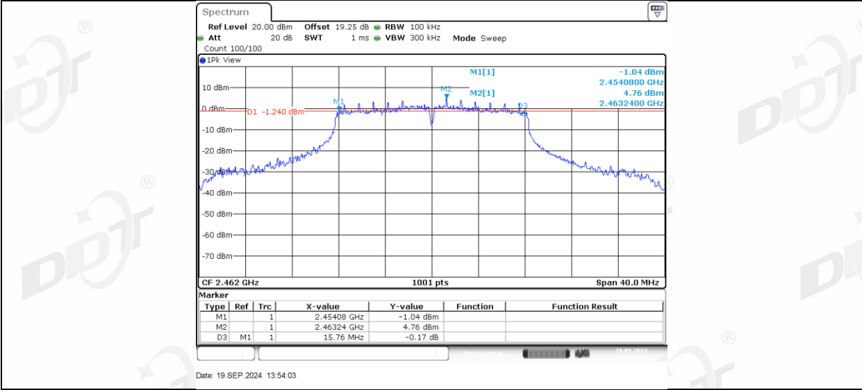
11G Ant2_2462
