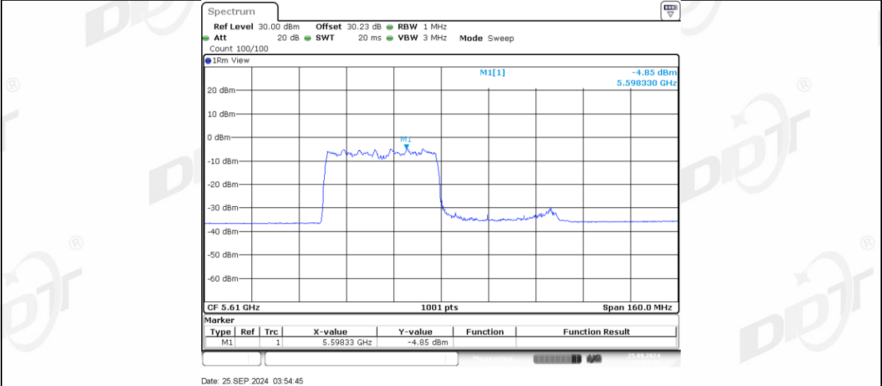
11AX80MIMO_Ant2_5610_484Tone_RU66
