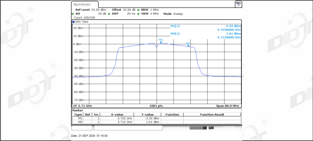
11N40MIMO_Ant2_5710_UNII-2C
