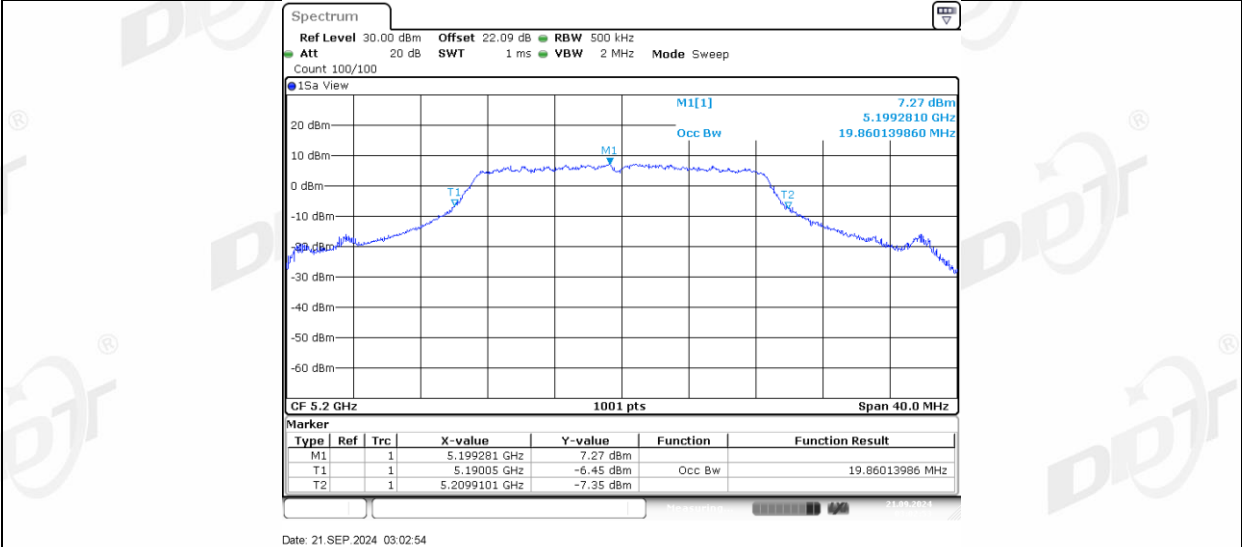
11AC20MIMO_Ant2_5200
