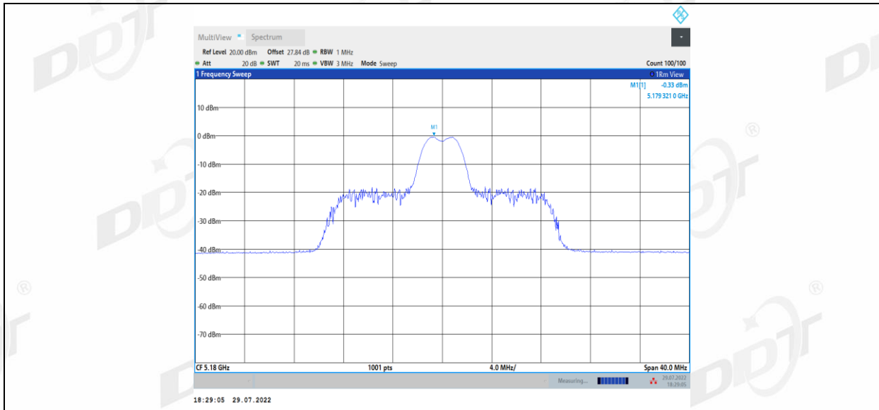
11AX20MIMO_Ant1_5180_26Tone_RU8
