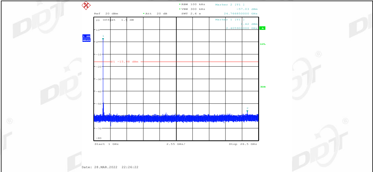
GFSK_Ant1_2442_0~Reference
