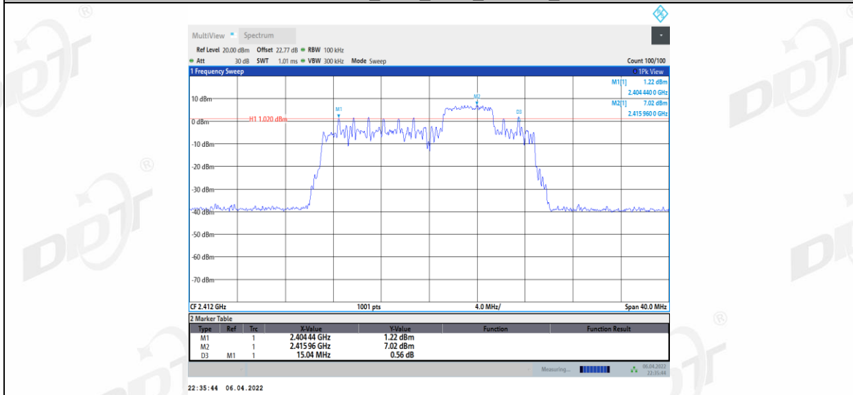
11AX20MIMO_Ant2_2412_52Tone_RU40
