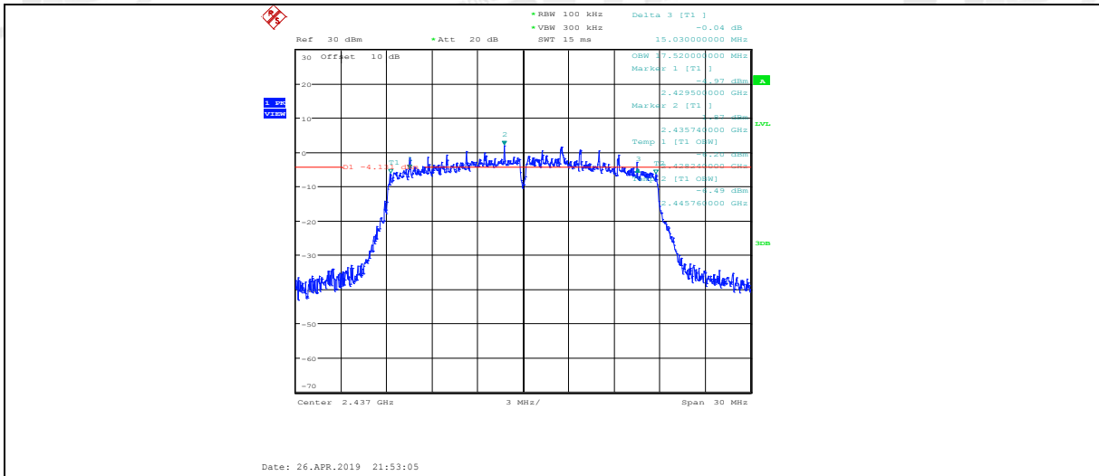
11N20MIMO_ANT2_2437_6dB Bandwidth
