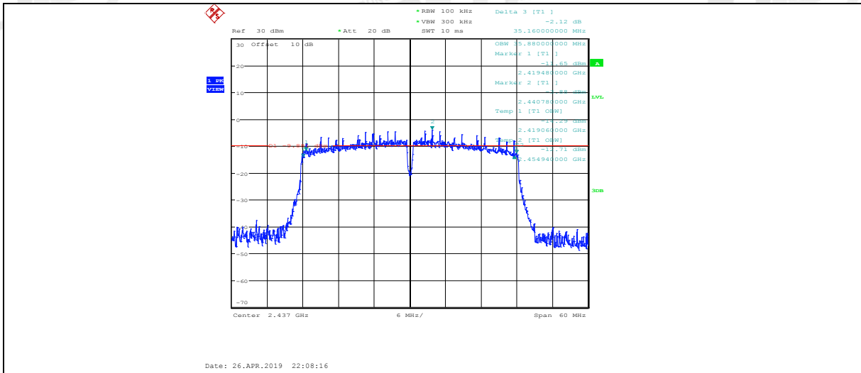
11N40MIMO_ANT2_2437_6dB Bandwidth
