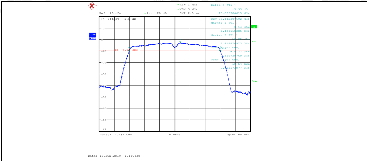
11N40MIMO_ANT2_2437_99% Bandwidth
