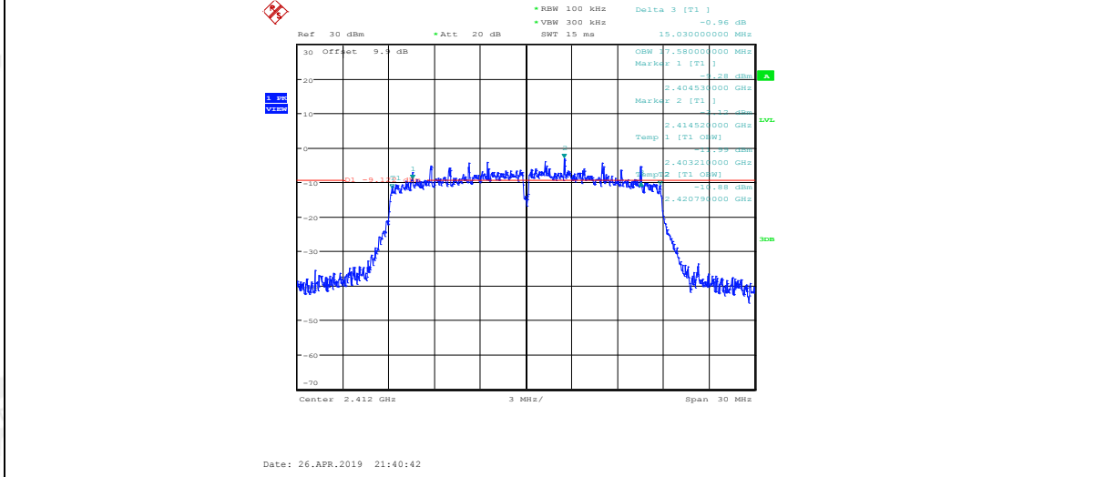
11N20MIMO_ANT2_2412_6dB Bandwidth
