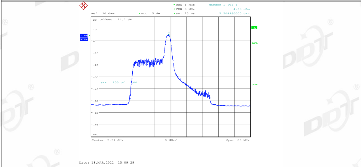
11AX40MIMO_Ant1_5510_26Tone_RU17
