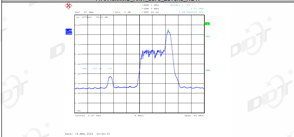
11AX40MIMO_Ant1_5670_52Tone_RU37
