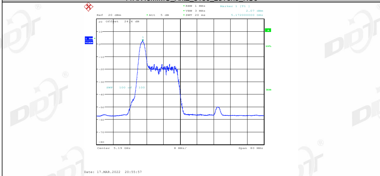
11AX40MIMO_Ant2_5190_26Tone_RU8
