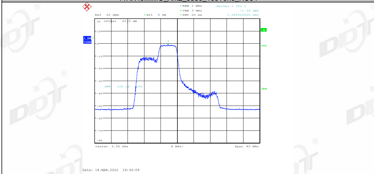
11AX40MIMO_Ant2_5550_106Tone_RU55
