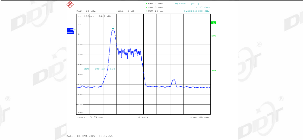
11AX40MIMO_Ant2_5550_26Tone_RU8
