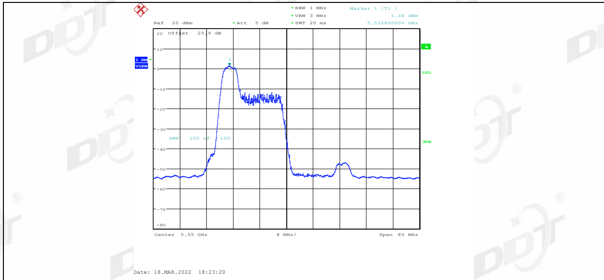
11AX40MIMO_Ant2_5550_52Tone_RU40
