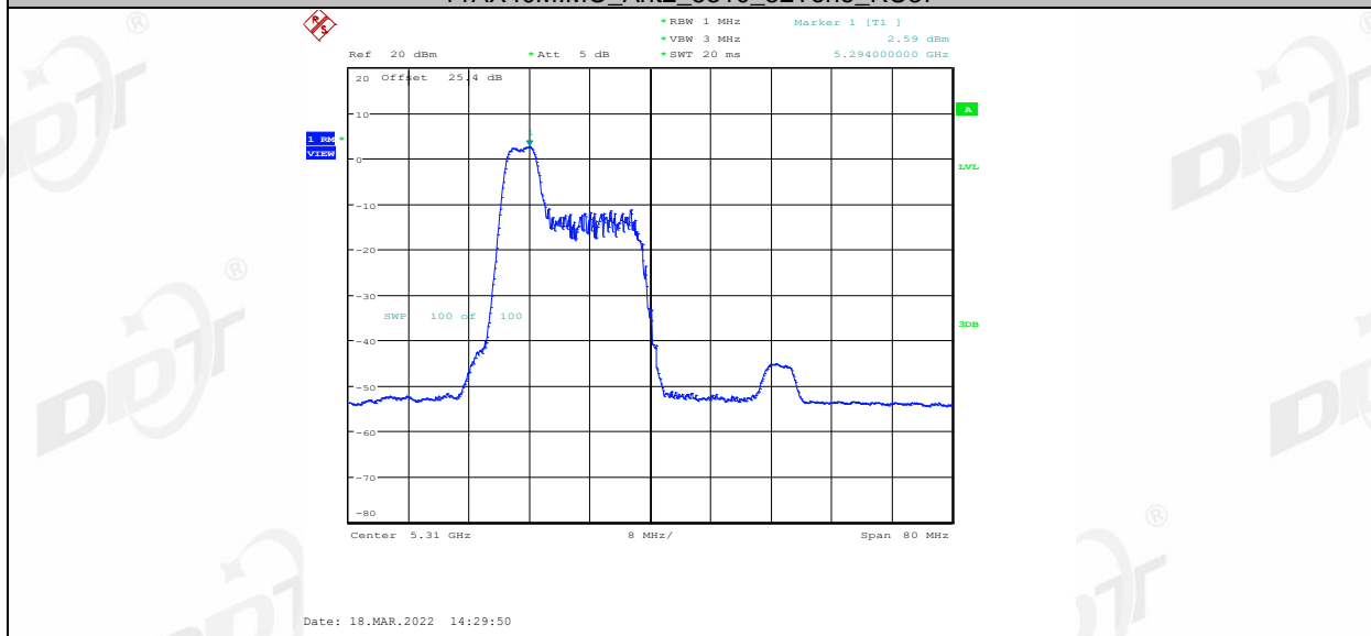
11AX40MIMO_Ant2_5310_52Tone_RU40
