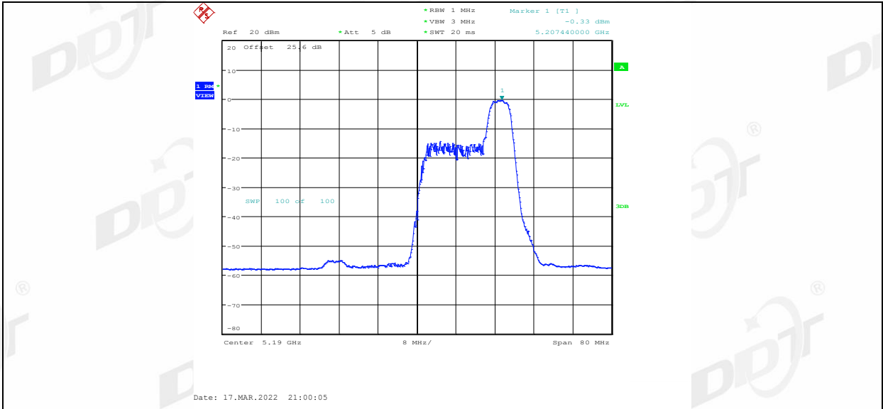
11AX40MIMO_Ant2_5190_106Tone_RU53
