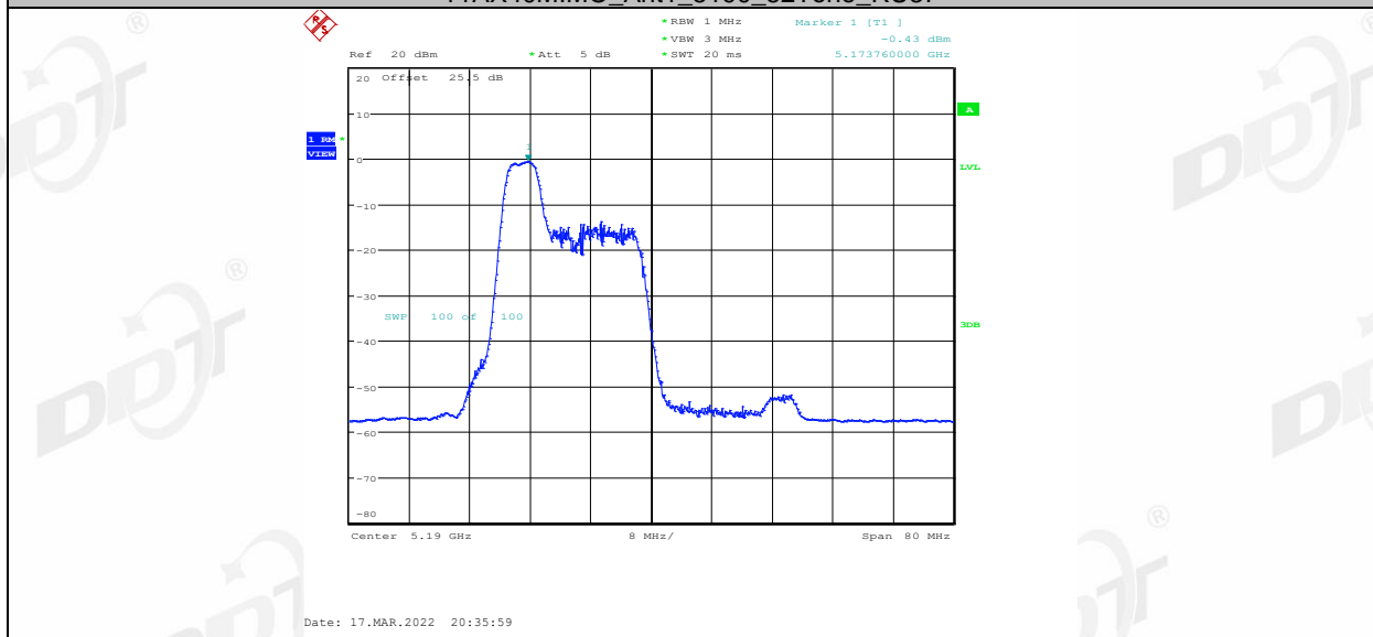
11AX40MIMO_Ant1_5190_52Tone_RU40
