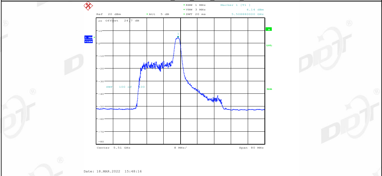
11AX40MIMO_Ant2_5510_26Tone_RU17
