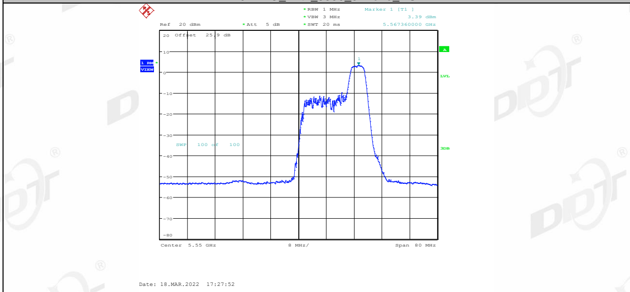
11AX40MIMO_Ant1_5550_106Tone_RU53
