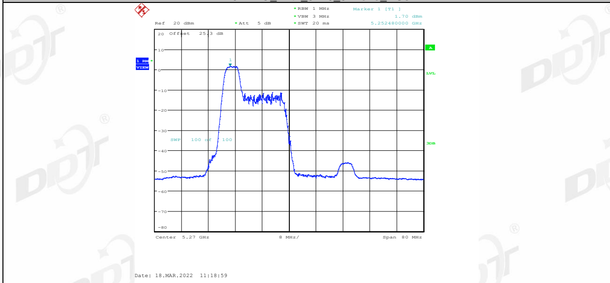
11AX40MIMO_Ant2_5270_52Tone_RU40
