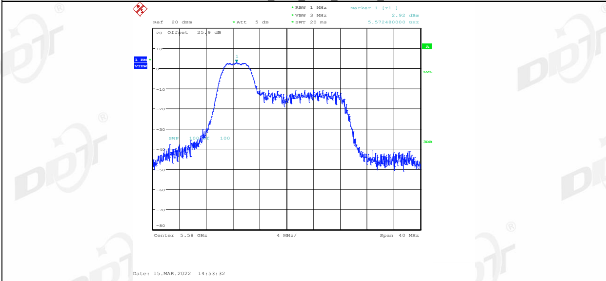
11AX20MIMO_Ant1_5580_52Tone_RU38
