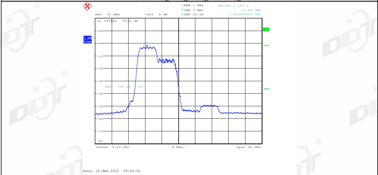
11AX40MIMO_Ant2_5230_106Tone_RU54
