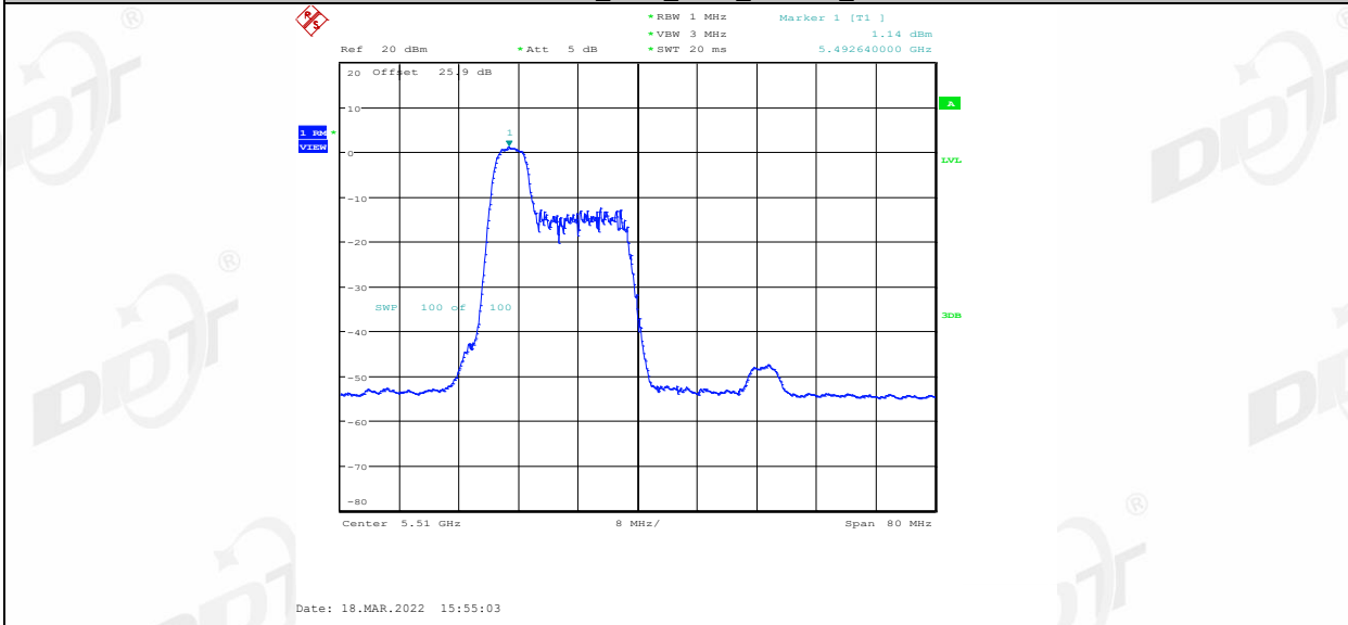
11AX40MIMO_Ant2_5510_52Tone_RU40
