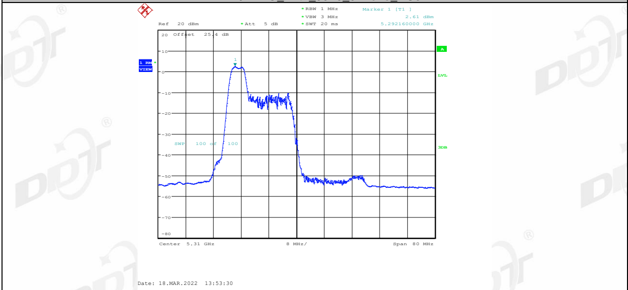
11AX40MIMO_Ant1_5310_52Tone_RU40
