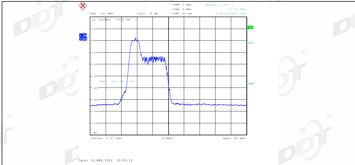
11AX40MIMO_Ant2_5670_52Tone_RU40
