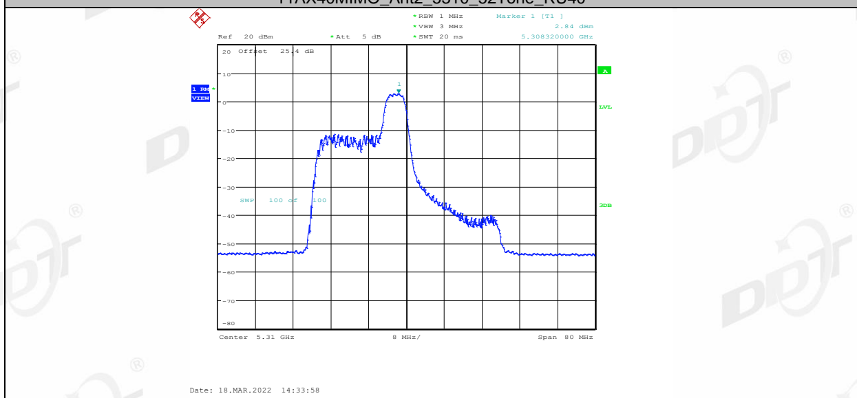
11AX40MIMO_Ant2_5310_52Tone_RU44
