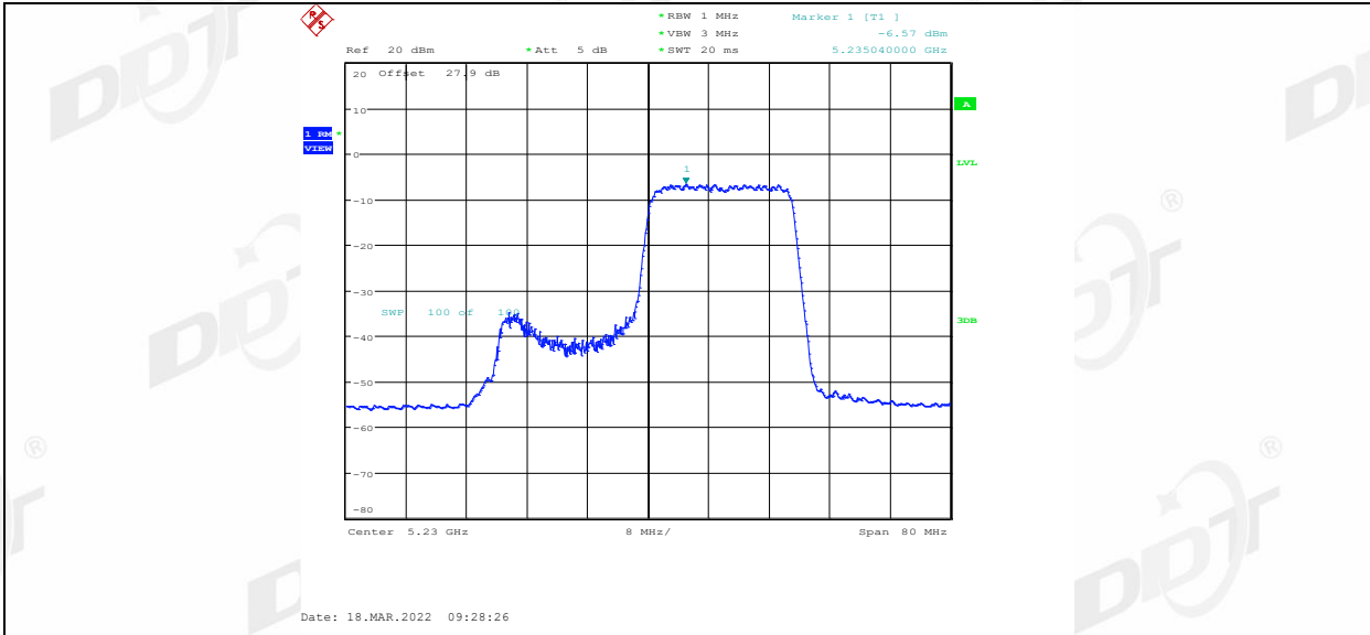
11AX40MIMO_Ant2_5230_26Tone_RU0
