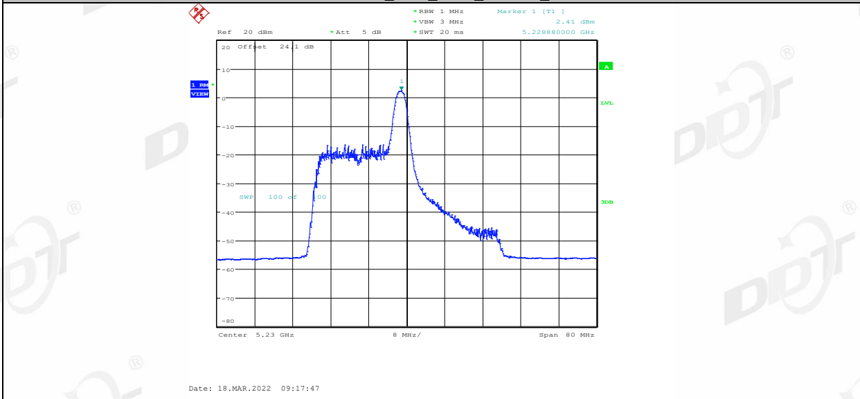
11AX40MIMO_Ant1_5230_26Tone_RU17
