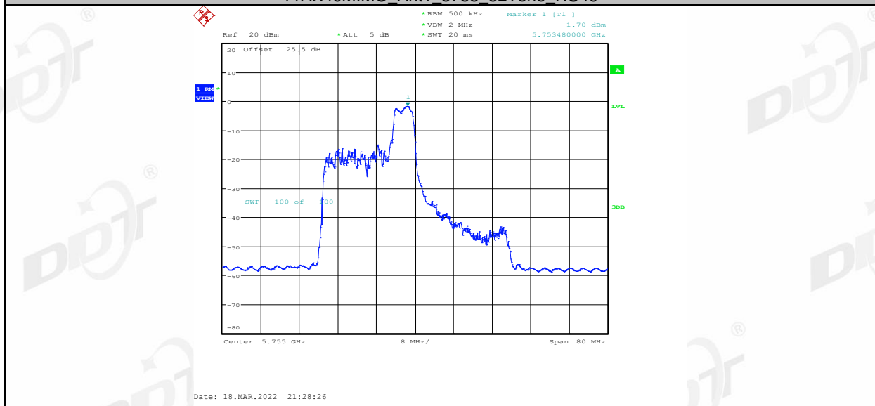
11AX40MIMO_Ant1_5755_52Tone_RU44
