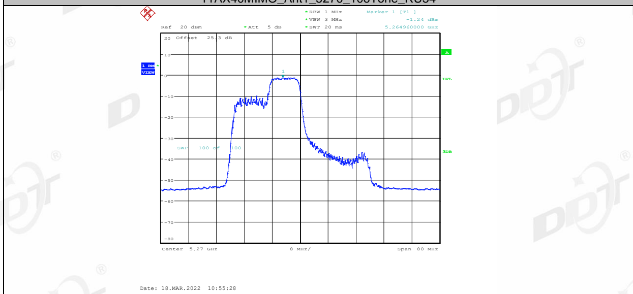
11AX40MIMO_Ant1_5270_106Tone_RU55
