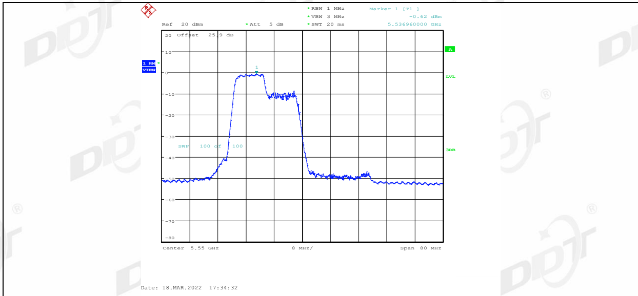
11AX40MIMO_Ant1_5550_106Tone_RU54
