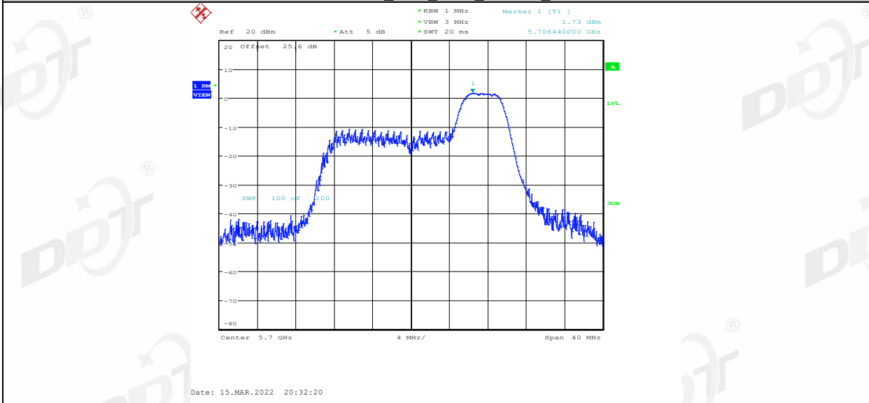
11AX20MIMO_Ant1_5700_106Tone_RU53
