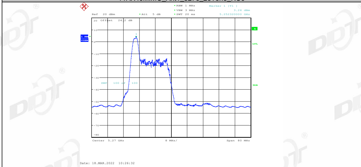
11AX40MIMO_Ant1_5270_26Tone_RU8
