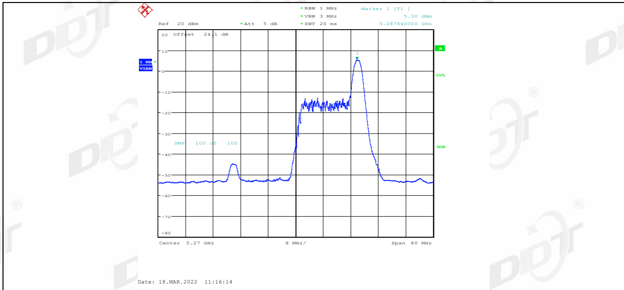
11AX40MIMO_Ant2_5270_52Tone_RU37
