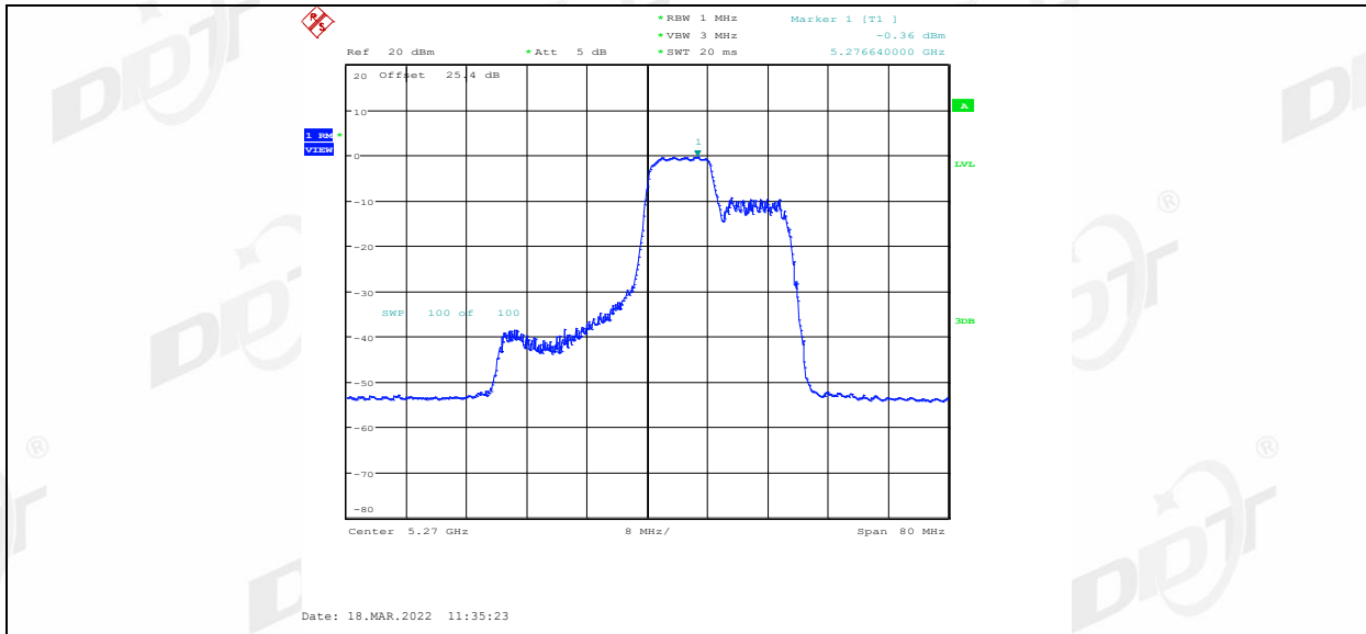
11AX40MIMO_Ant2_5270_106Tone_RU56
