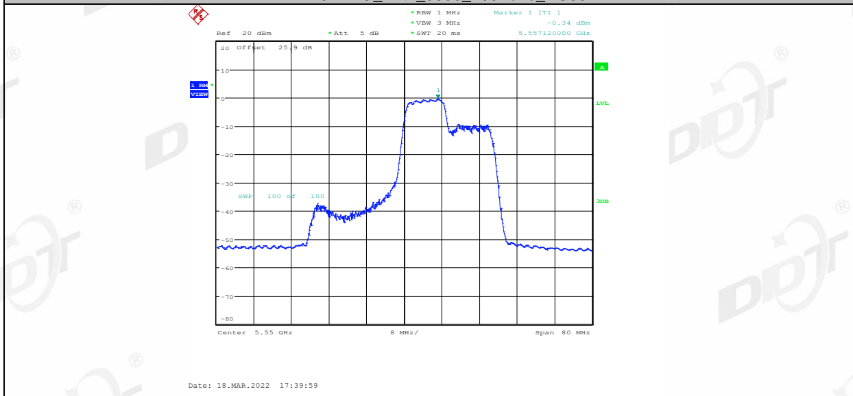
11AX40MIMO_Ant1_5550_106Tone_RU56
