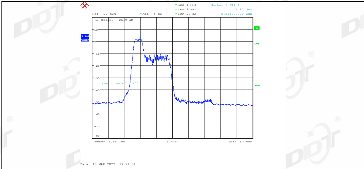
11AX40MIMO_Ant1_5550_52Tone_RU40
