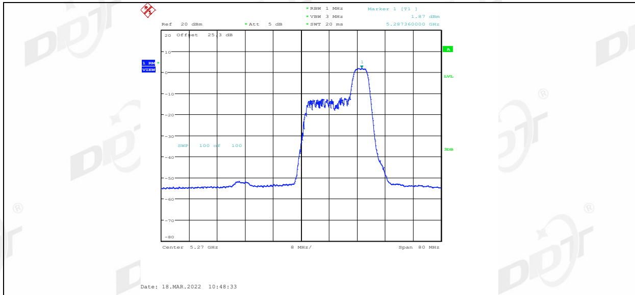
11AX40MIMO_Ant1_5270_106Tone_RU53
