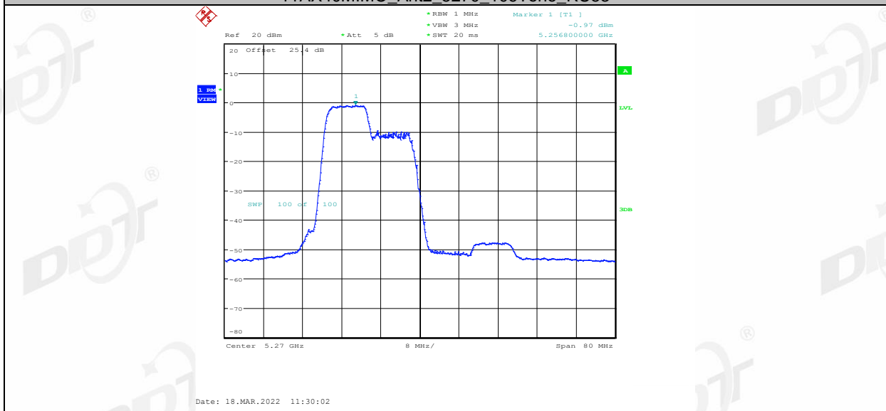
11AX40MIMO_Ant2_5270_106Tone_RU54
