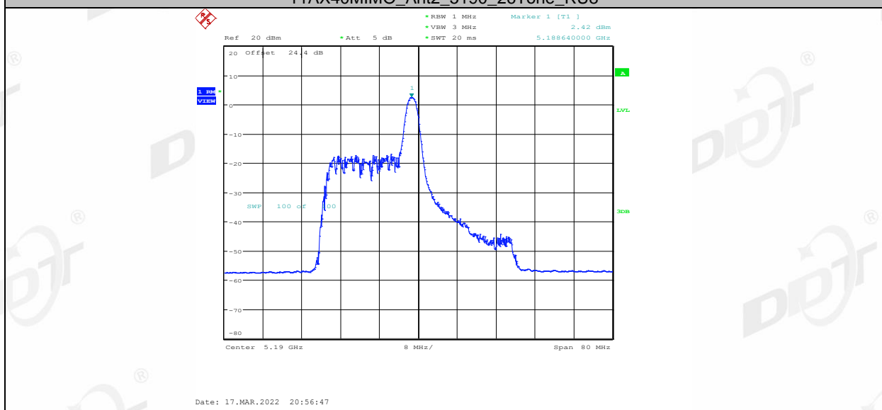
11AX40MIMO_Ant2_5190_26Tone_RU17
