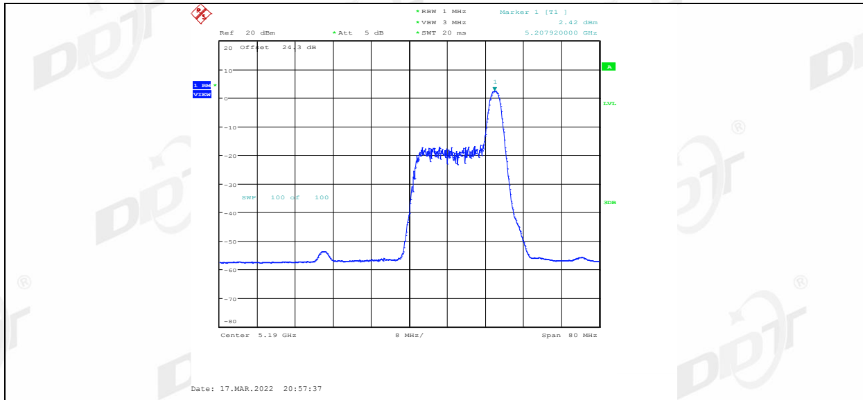
11AX40MIMO_Ant2_5190_52Tone_RU37
