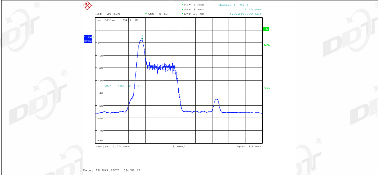
11AX40MIMO_Ant2_5230_26Tone_RU8
