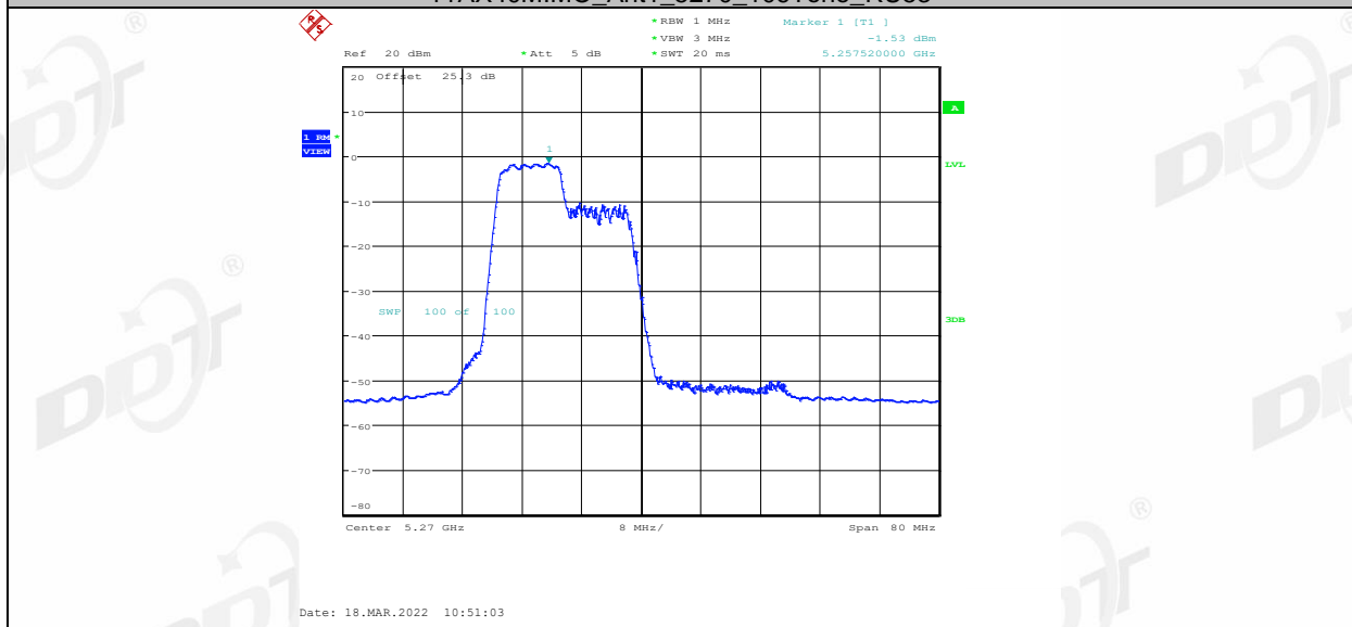
11AX40MIMO_Ant1_5270_106Tone_RU54
