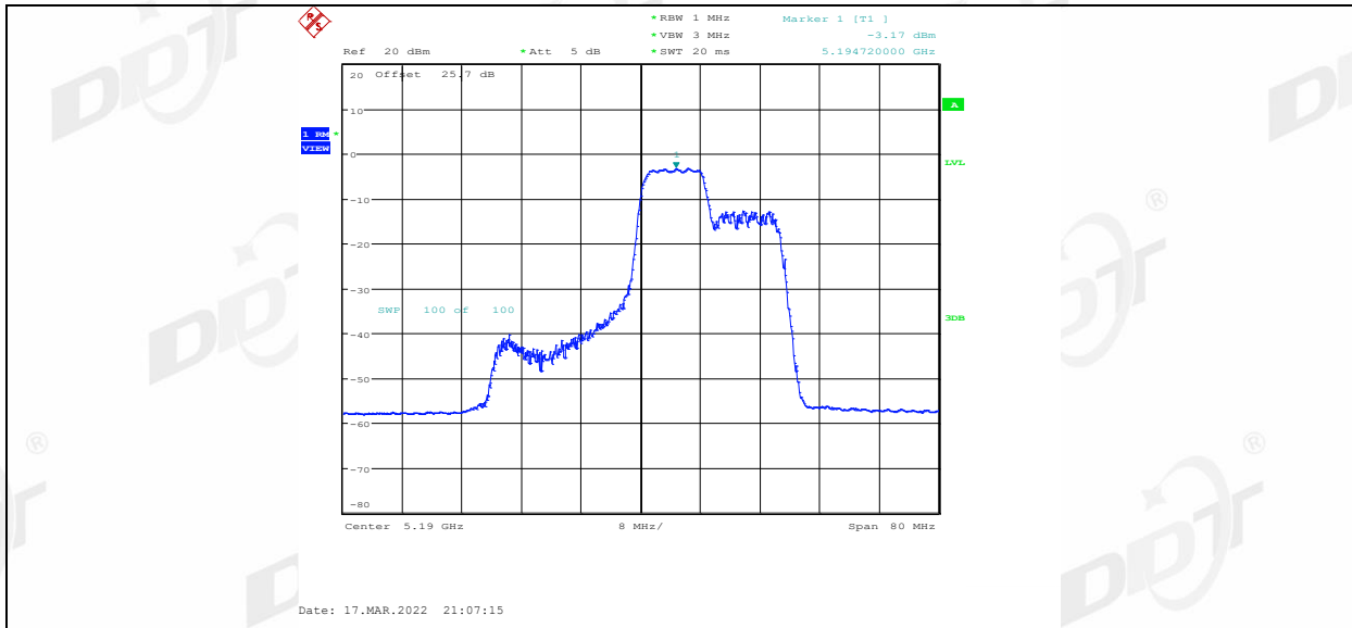
11AX40MIMO_Ant2_5190_106Tone_RU56
