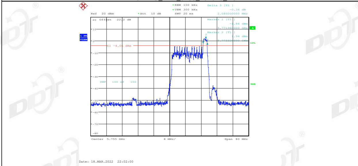
11AX40MIMO_Ant2_5755_52Tone_RU37
