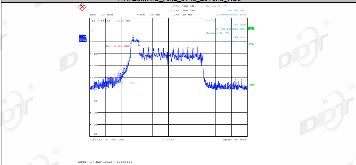
11AX20MIMO_Ant2_5745_26Tone_RU4
