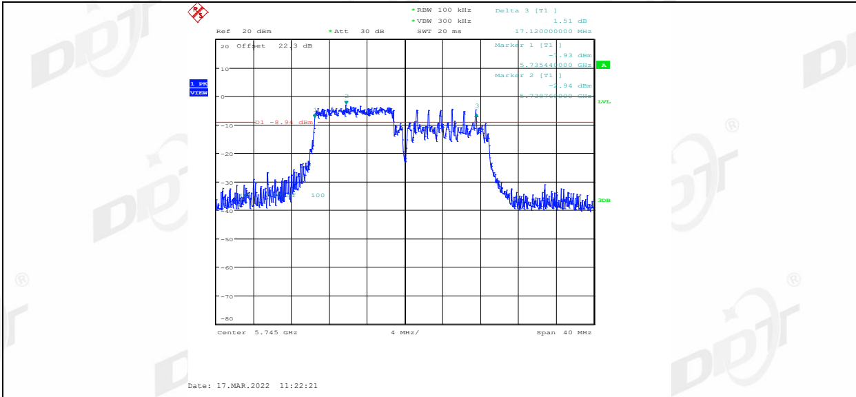
11AX20MIMO_Ant1_5745_106Tone_RU54
