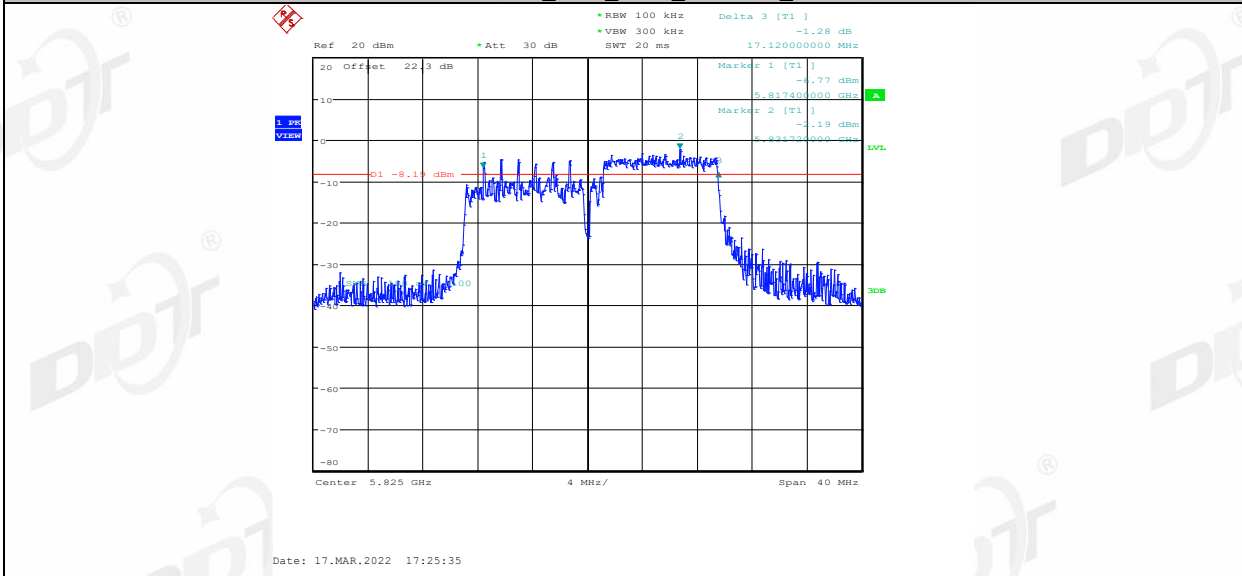
11AX20MIMO_Ant2_5825_26Tone_RU0
