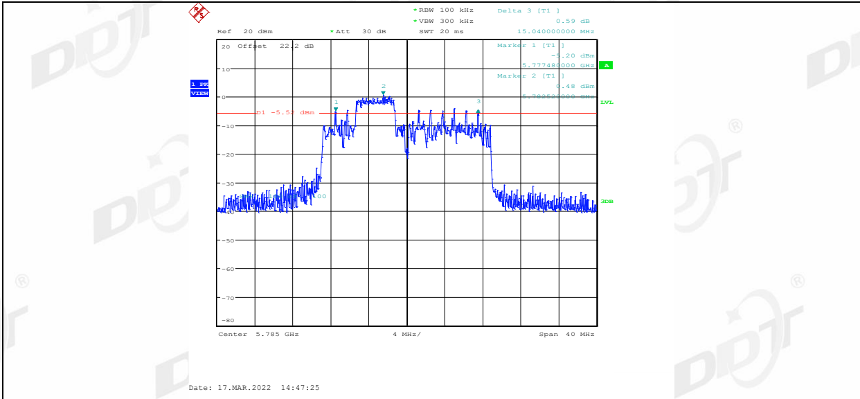
11AX20MIMO_Ant2_5785_52Tone_RU39
