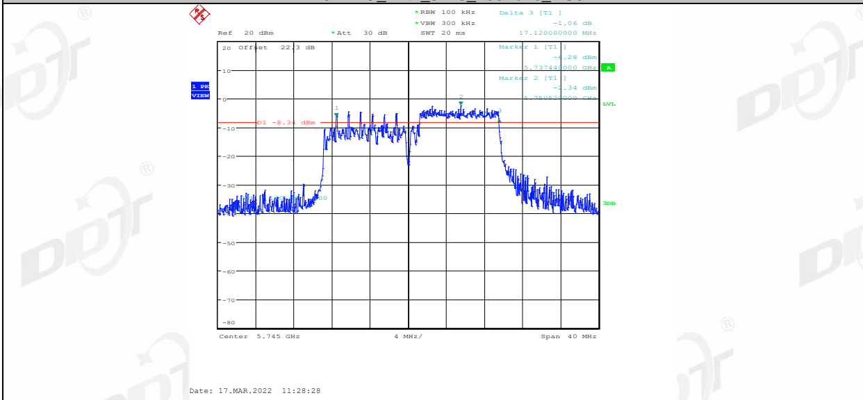
11AX20MIMO_Ant2_5745_26Tone_RU0
