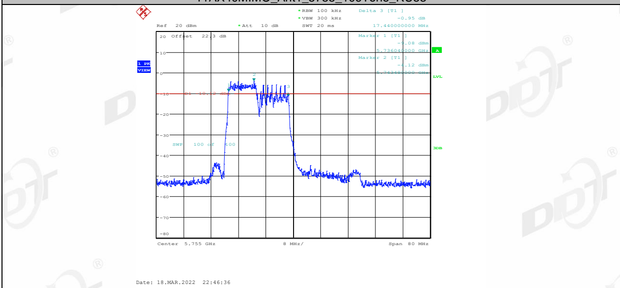
11AX40MIMO_Ant1_5755_106Tone_RU54
