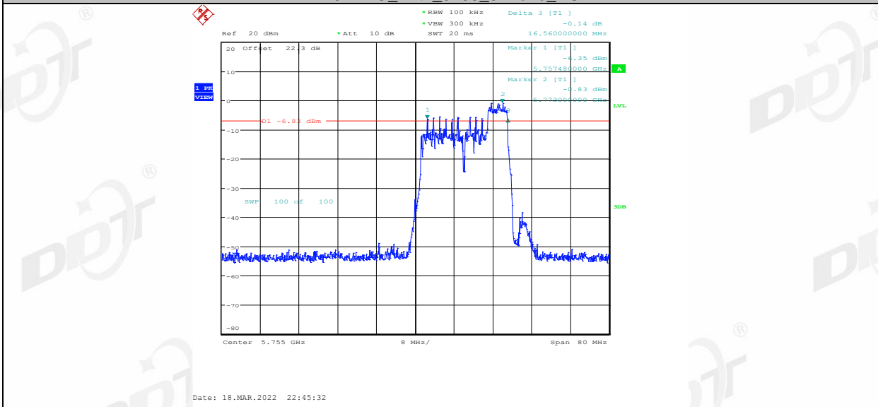
11AX40MIMO_Ant1_5755_106Tone_RU53
