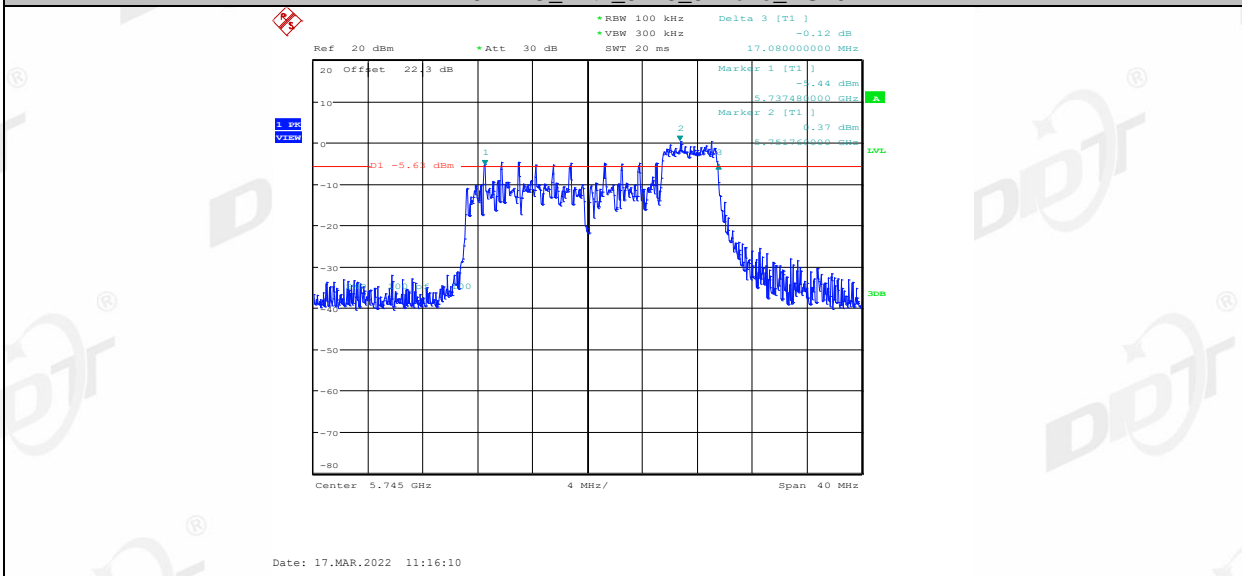
11AX20MIMO_Ant1_5745_106Tone_RU53
