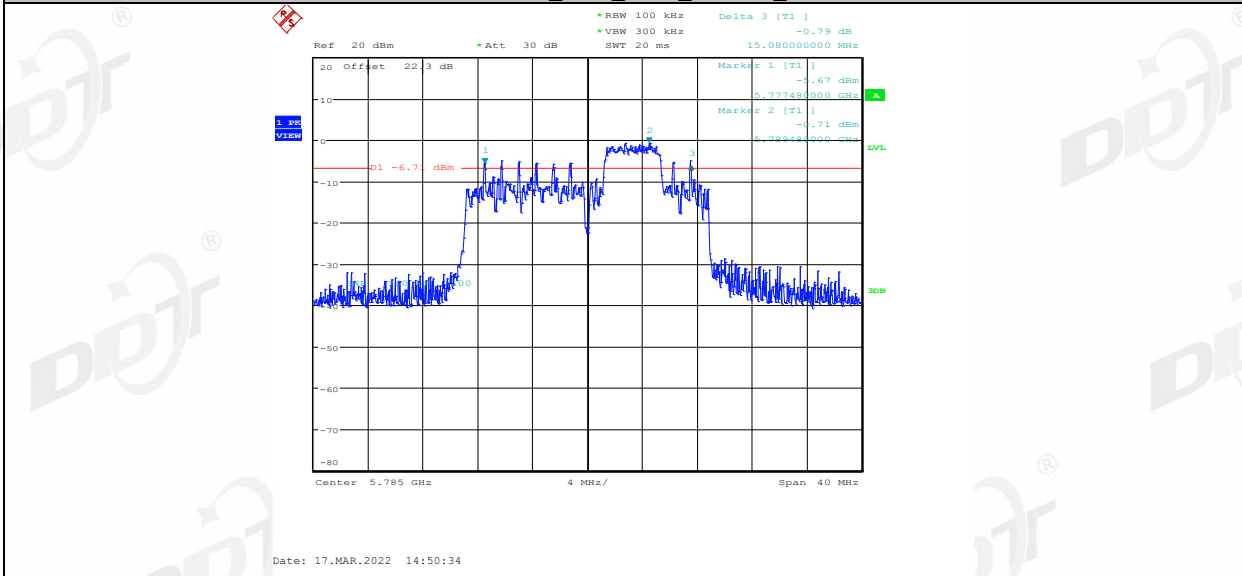
11AX20MIMO_Ant1_5785_52Tone_RU40
