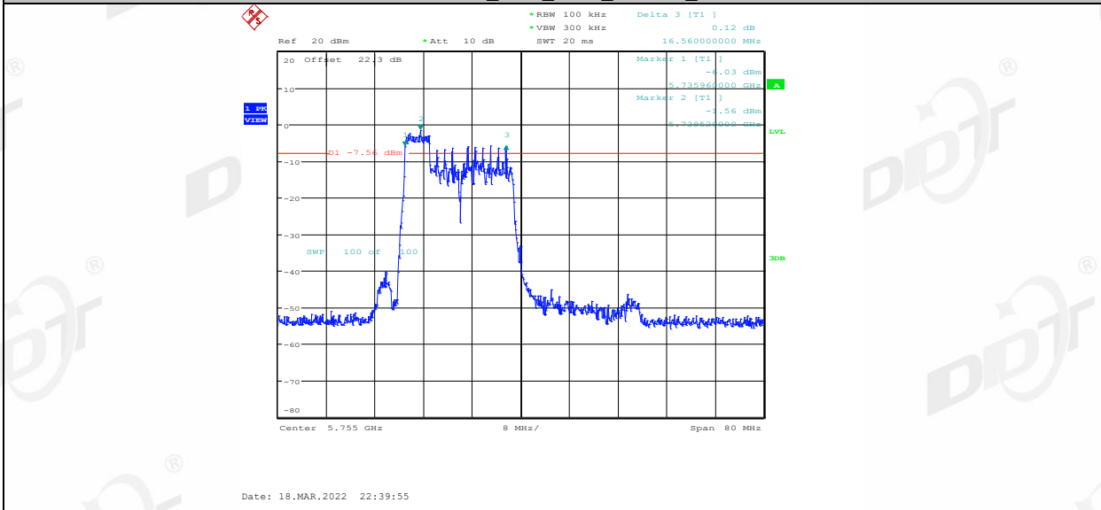
11AX40MIMO_Ant1_5755_52Tone_RU40
