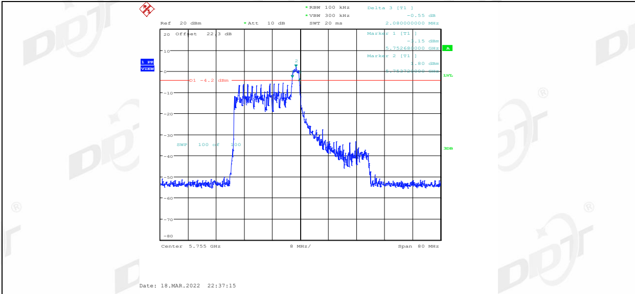
11AX40MIMO_Ant1_5755_26Tone_RU17
