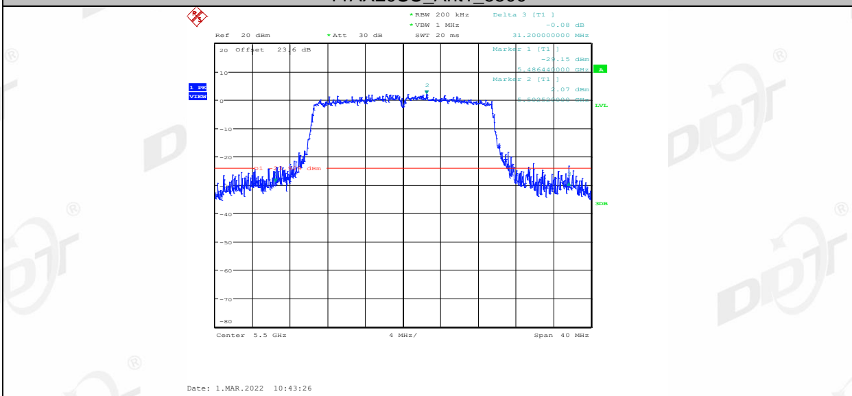
11AX20SU_Ant2_5500
