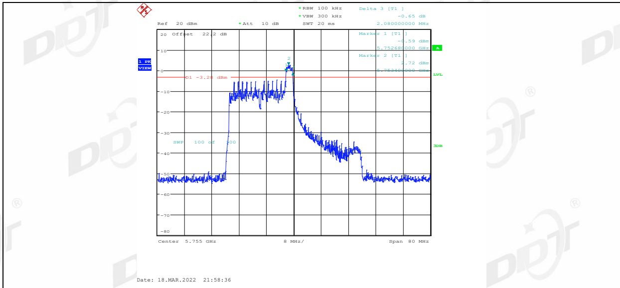
11AX40MIMO_Ant2_5755_26Tone_RU17
