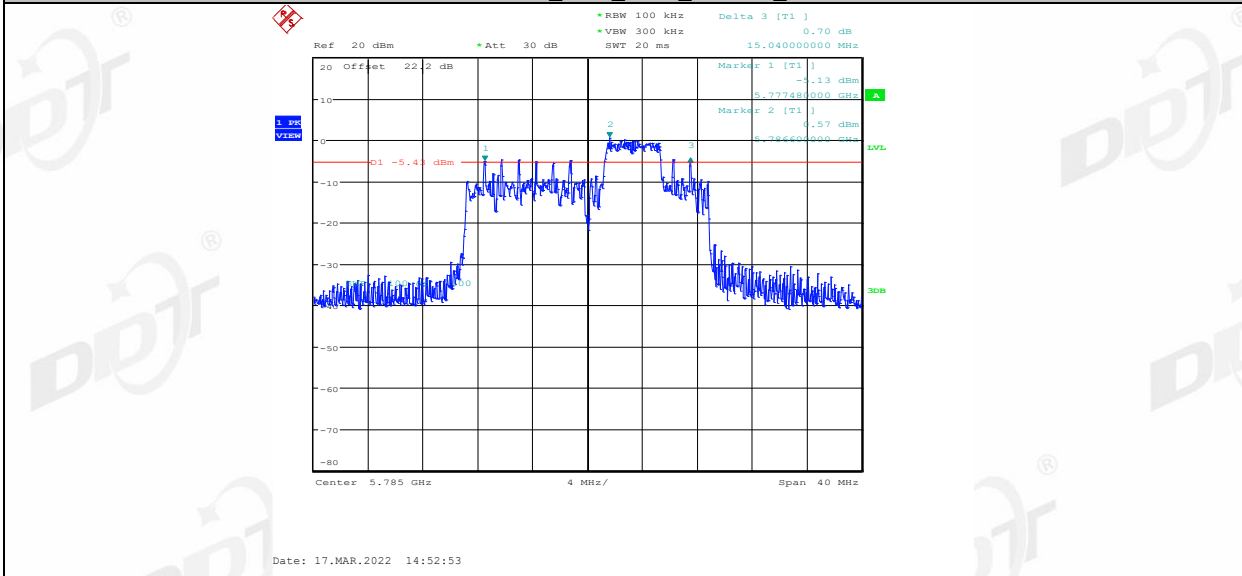
11AX20MIMO_Ant2_5785_52Tone_RU40
