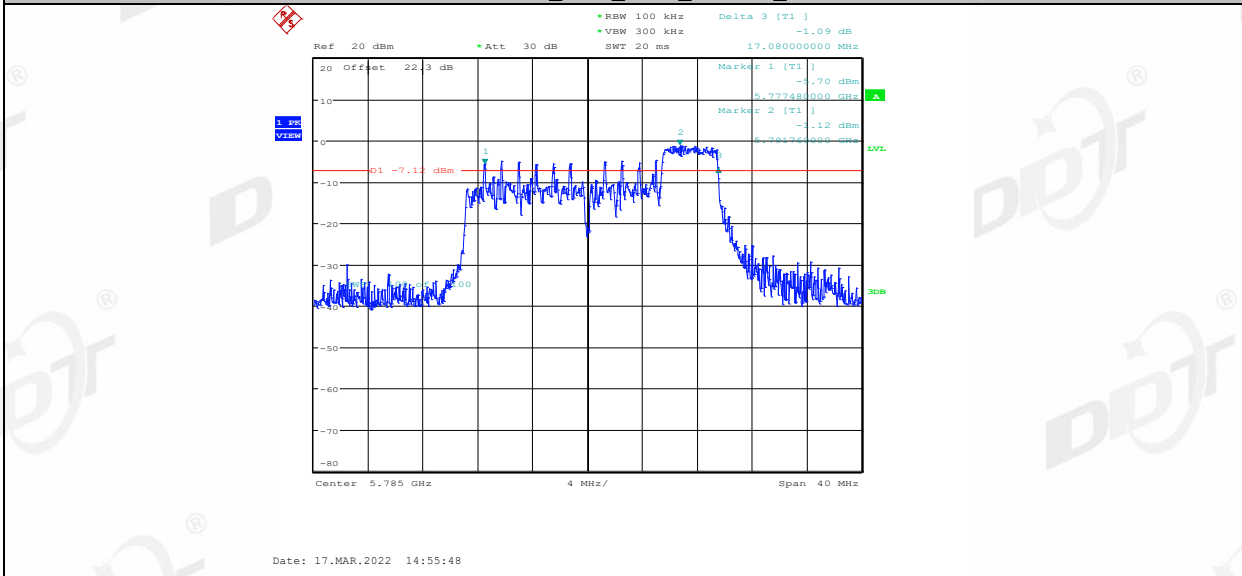
11AX20MIMO_Ant1_5785_106Tone_RU53
