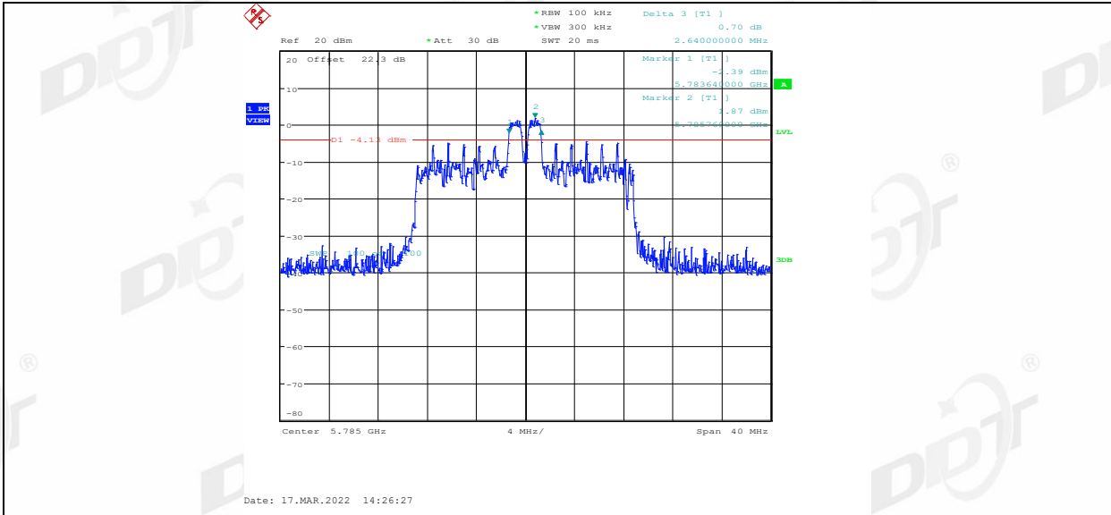
11AX20MIMO_Ant1_5785_26Tone_RU8
