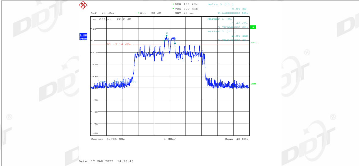
11AX20MIMO_Ant2_5785_26Tone_RU8
