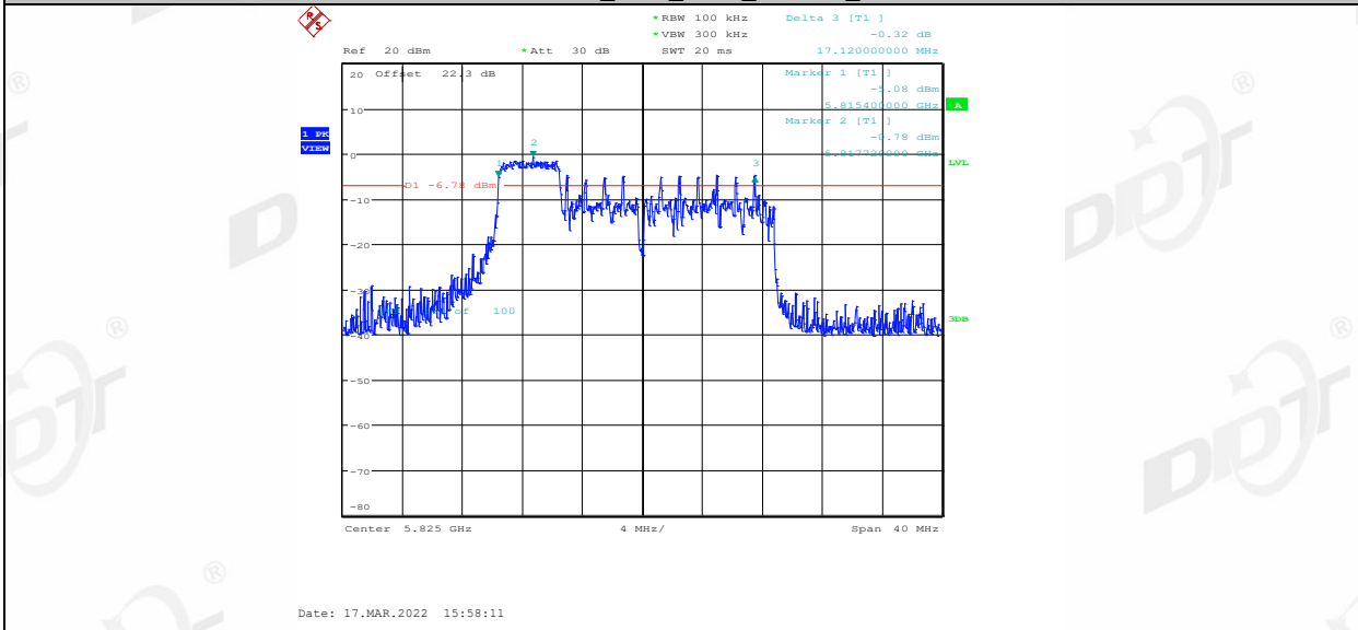
11AX20MIMO_Ant1_5825_52Tone_RU38
