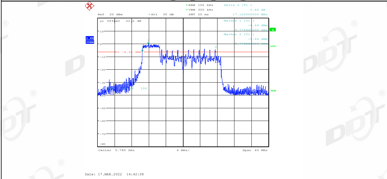
11AX20MIMO_Ant2_5785_52Tone_RU38
