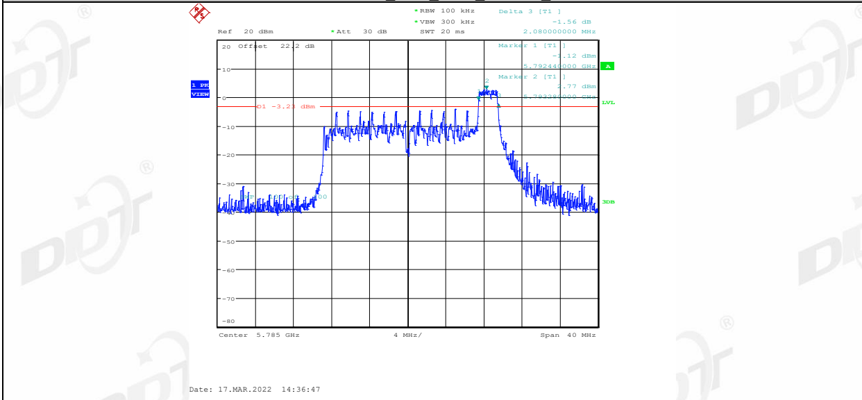
11AX20MIMO_Ant2_5785_52Tone_RU37
