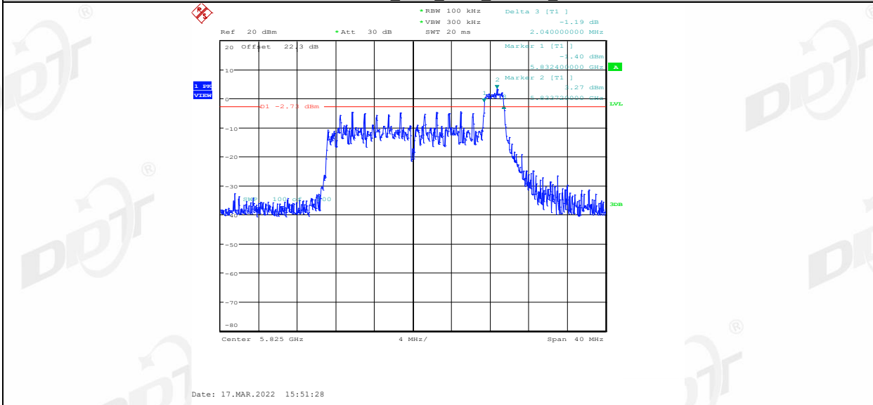
11AX20MIMO_Ant1_5825_52Tone_RU37
