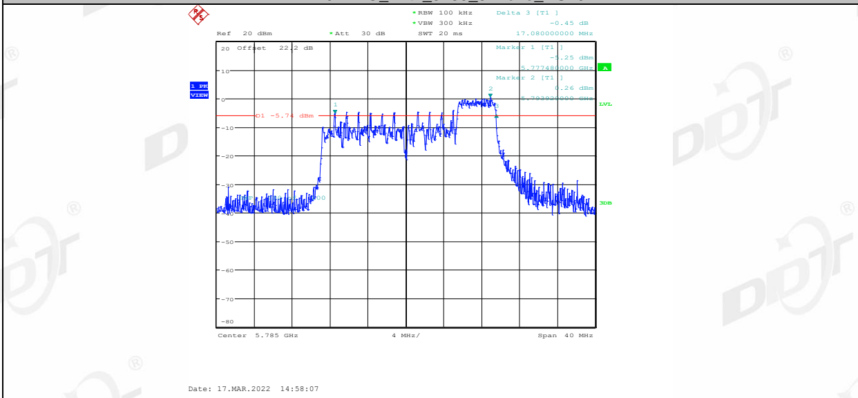
11AX20MIMO_Ant2_5785_106Tone_RU53
