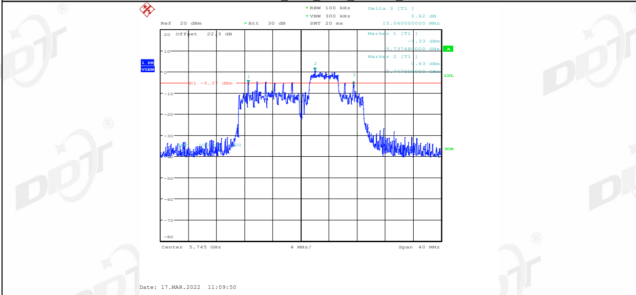
11AX20MIMO_Ant1_5745_52Tone_RU40
