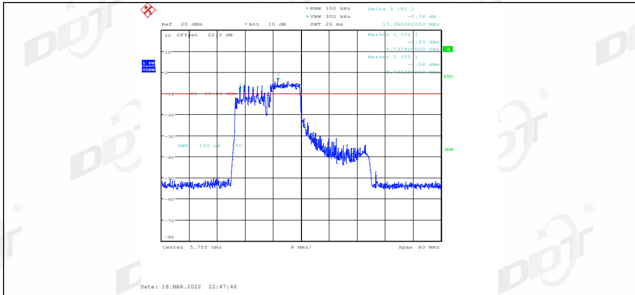
11AX40MIMO_Ant1_5755_106Tone_RU55
