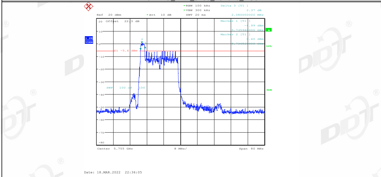
11AX40MIMO_Ant1_5755_26Tone_RU8
