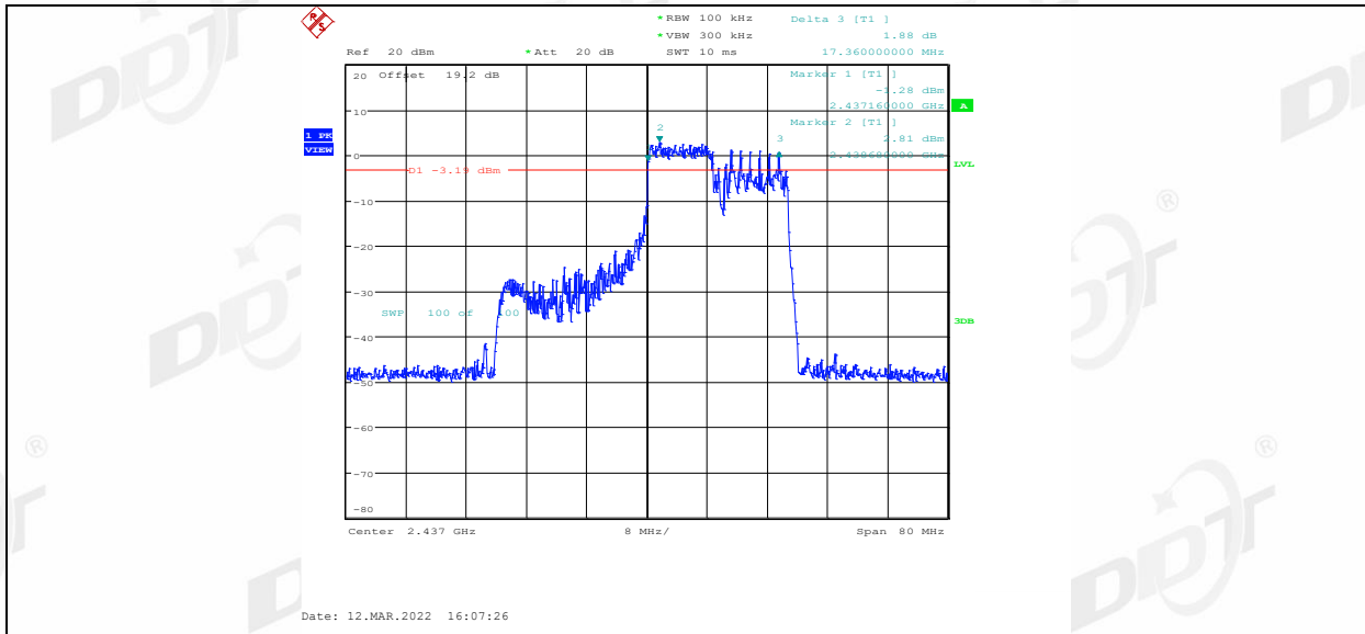
11AX40MIMO_Ant1_2437_106Tone_RU56
