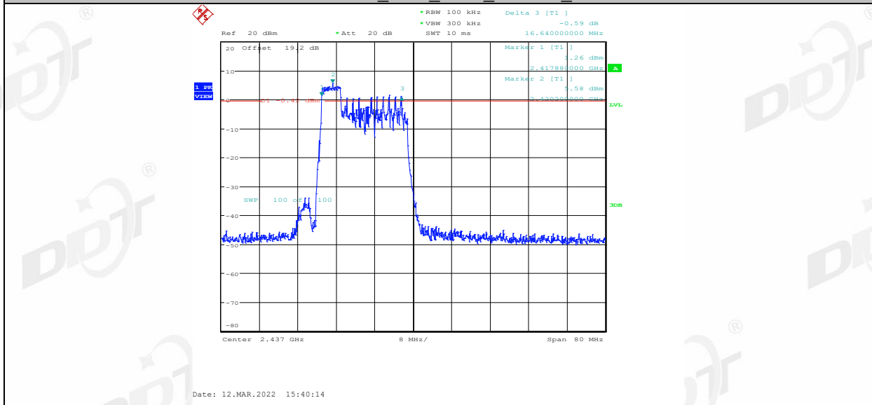
11AX40MIMO_Ant2_2437_52Tone_RU40
