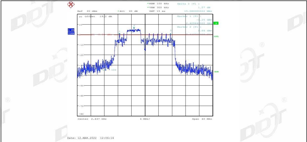
11AX20MIMO_Ant1_2437_52Tone_RU39
