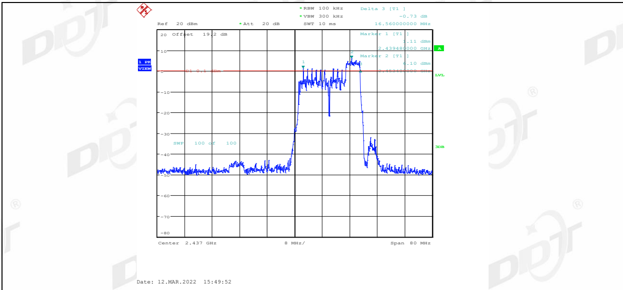
11AX40MIMO_Ant1_2437_106Tone_RU53
