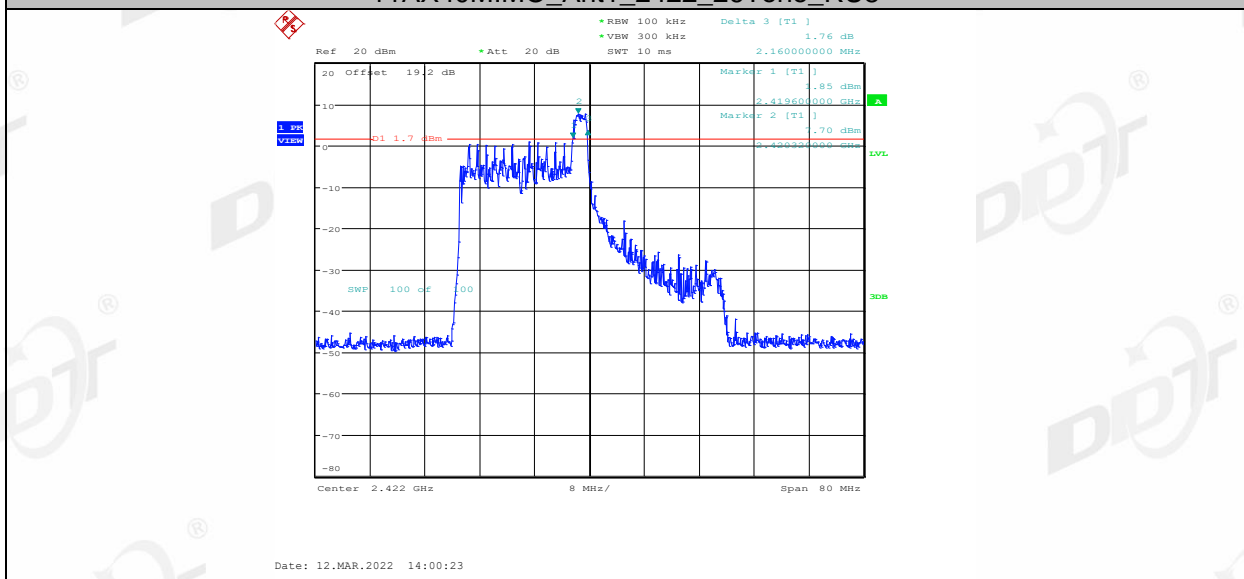
11AX40MIMO_Ant1_2422_26Tone_RU17
