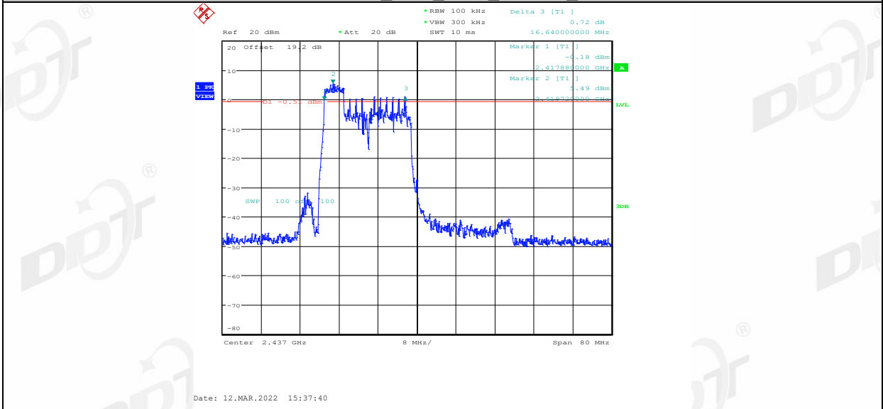
11AX40MIMO_Ant1_2437_52Tone_RU40
