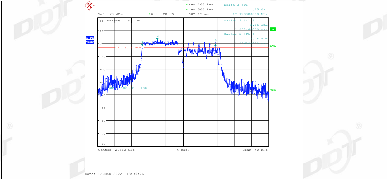
11AX20MIMO_Ant1_2462_106Tone_RU54
