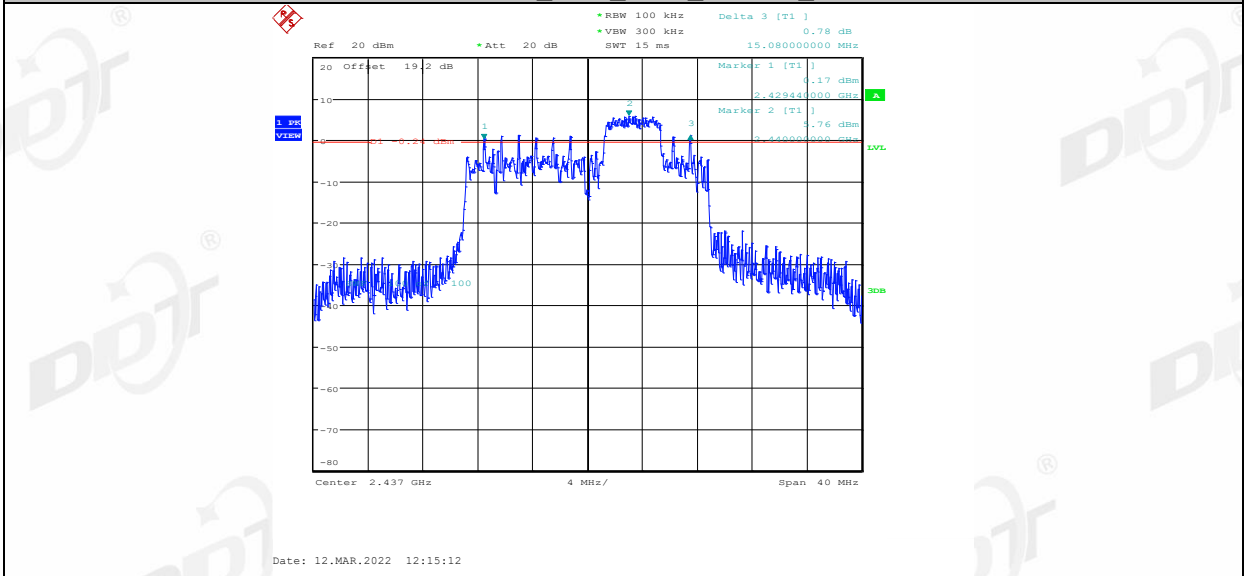
11AX20MIMO_Ant2_2437_52Tone_RU40
