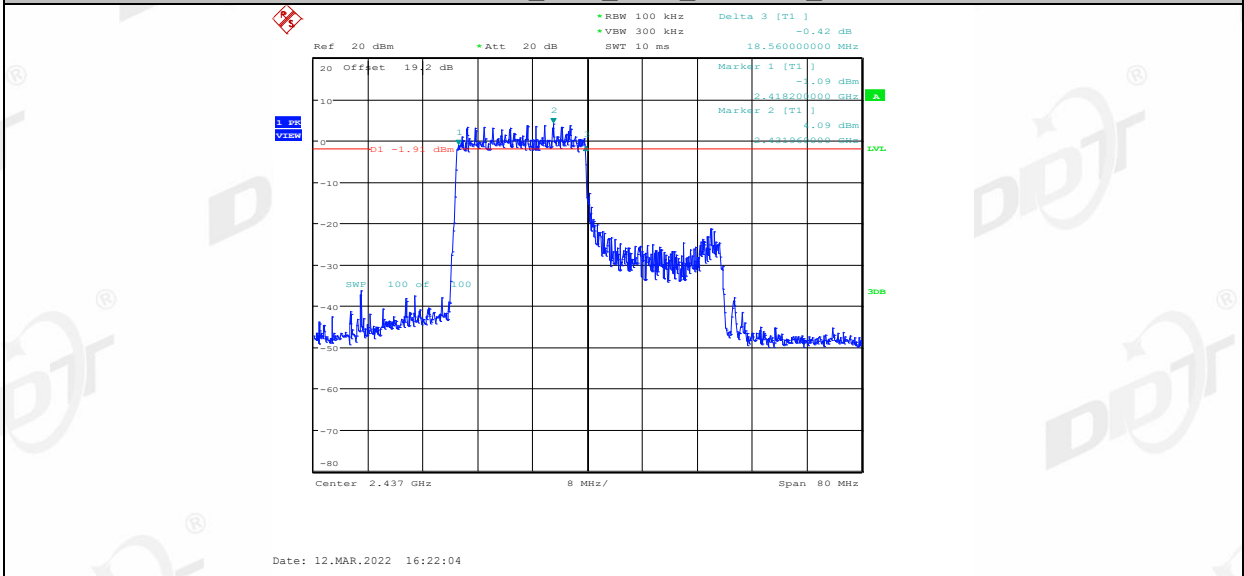
11AX40MIMO_Ant2_2437_242Tone_RU62
