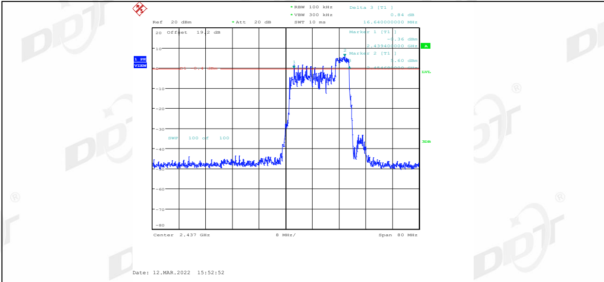
11AX40MIMO_Ant2_2437_106Tone_RU53
