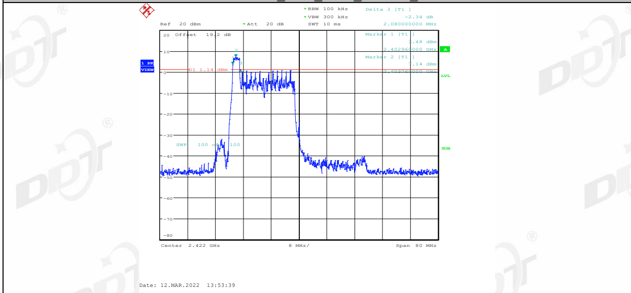
11AX40MIMO_Ant1_2422_26Tone_RU8
