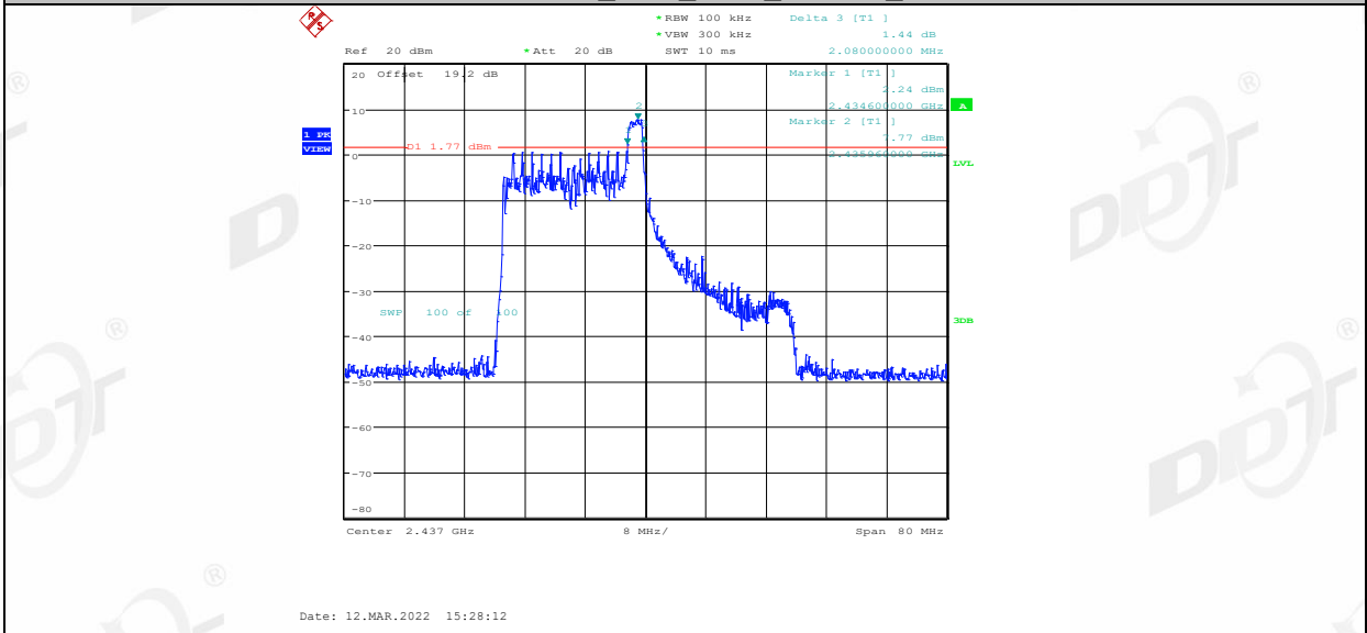
11AX40MIMO_Ant1_2437_26Tone_RU17
