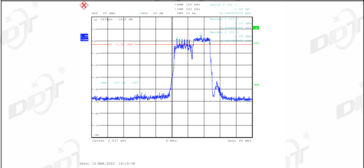
11AX40MIMO_Ant2_2437_242Tone_RU61
