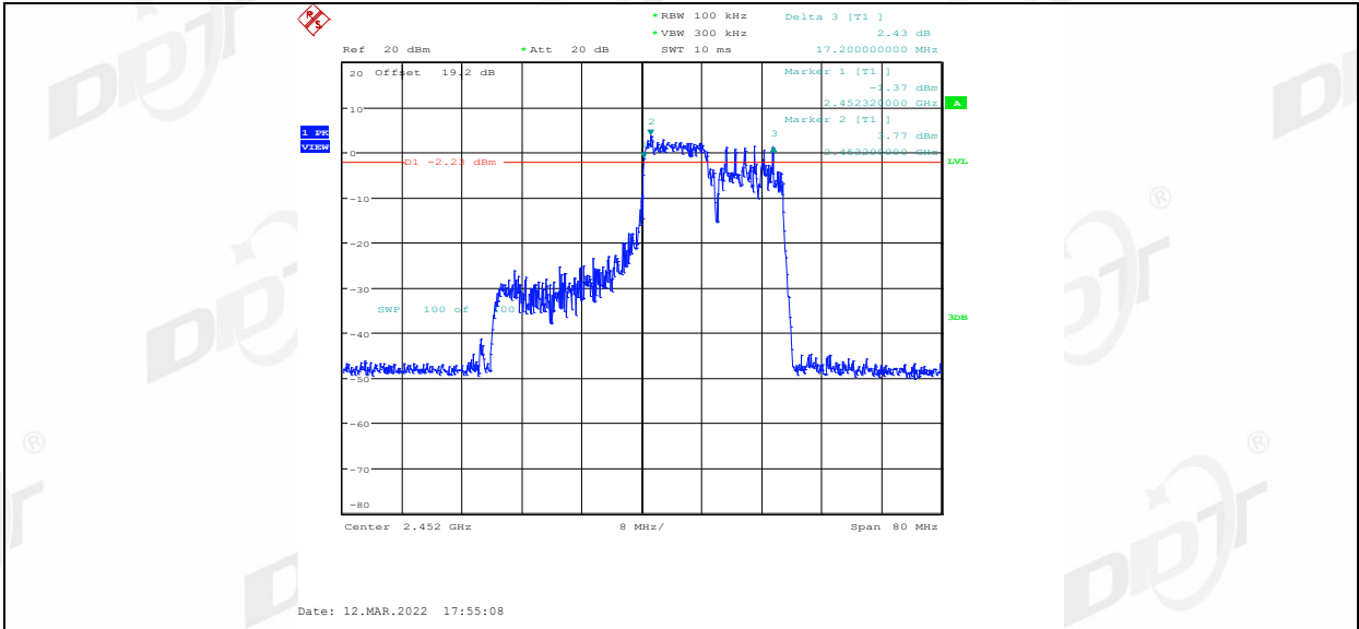
11AX40MIMO_Ant2_2452_106Tone_RU56
