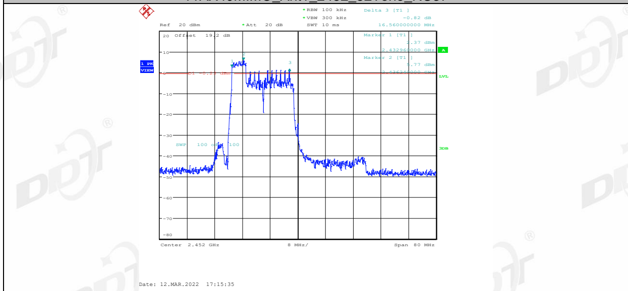
11AX40MIMO_Ant1_2452_52Tone_RU40
