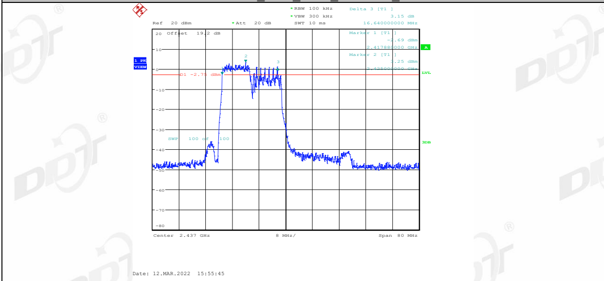
11AX40MIMO_Ant1_2437_106Tone_RU54
