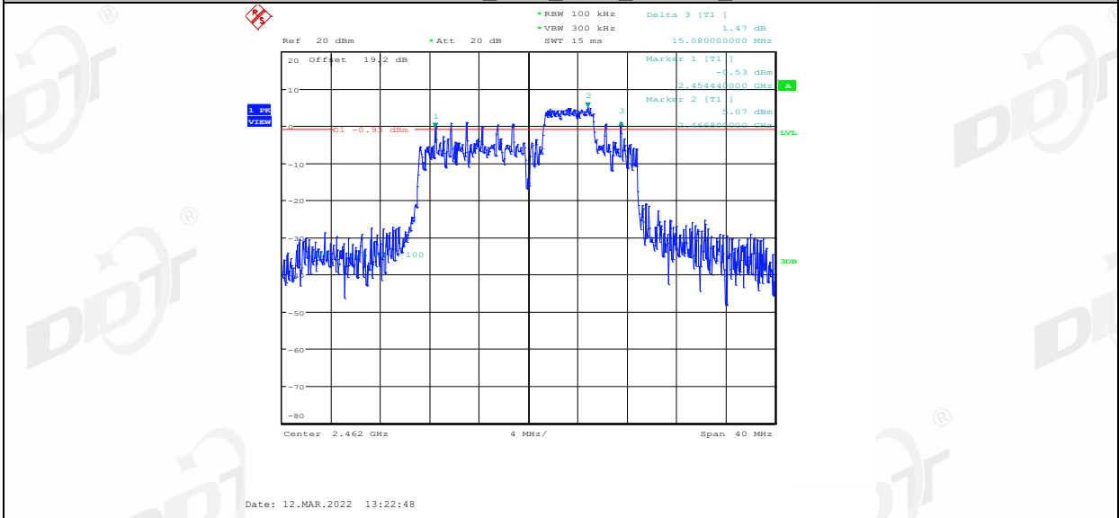
11AX20MIMO_Ant1_2462_52Tone_RU40
