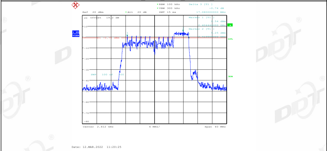
11AX20MIMO_Ant2_2412_106Tone_RU53
