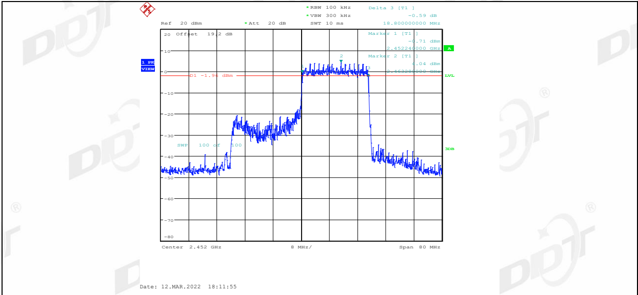
11AX40MIMO_Ant2_2452_26Tone_RU0
