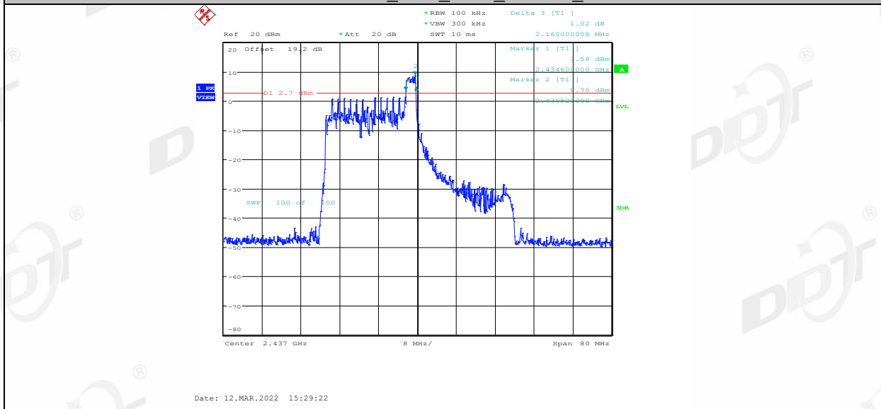
11AX40MIMO_Ant2_2437_26Tone_RU17
