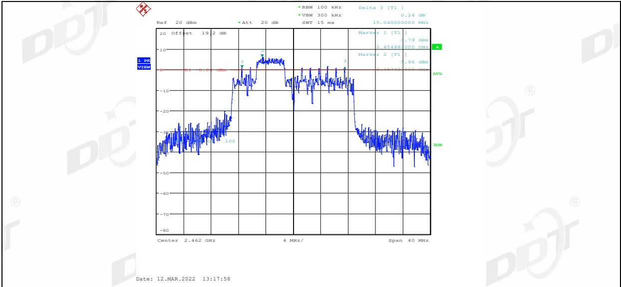
11AX20MIMO_Ant2_2462_52Tone_RU39
