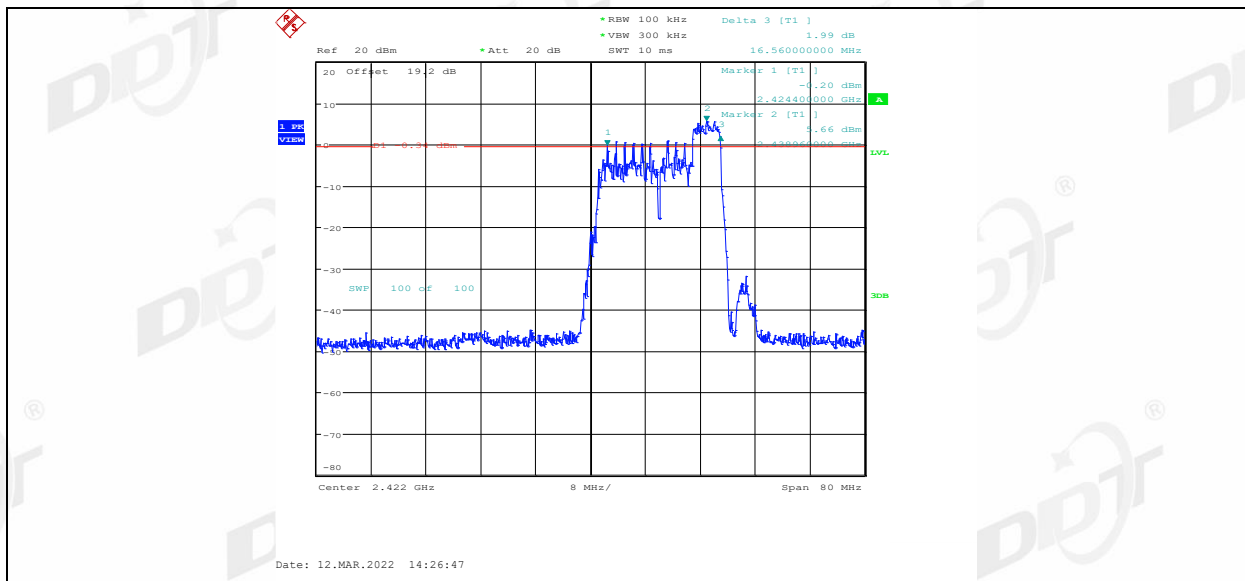
11AX40MIMO_Ant1_2422_106Tone_RU53
