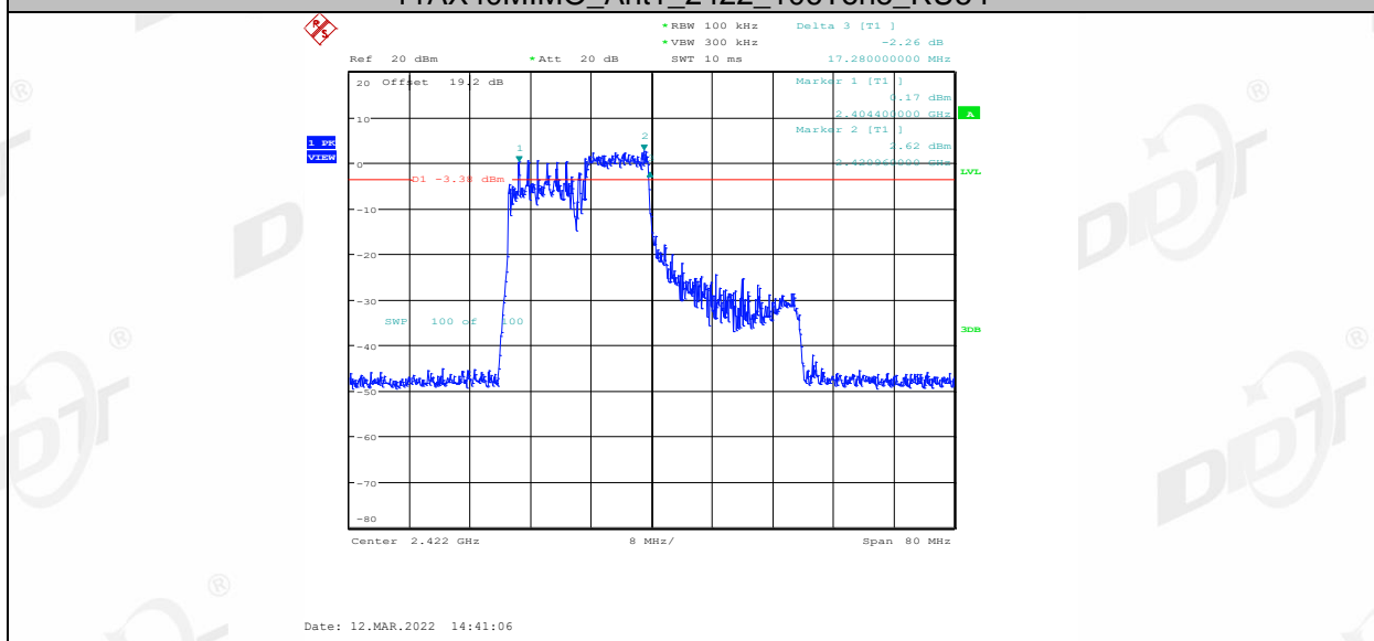
11AX40MIMO_Ant1_2422_106Tone_RU55
