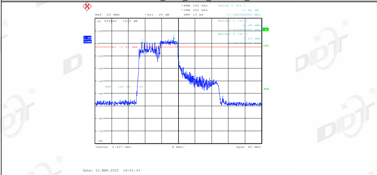
11AX40MIMO_Ant1_2437_106Tone_RU55
