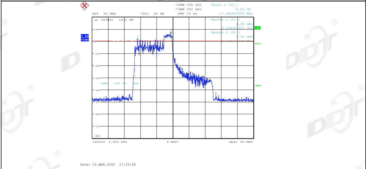
11AX40MIMO_Ant2_2452_52Tone_RU44
