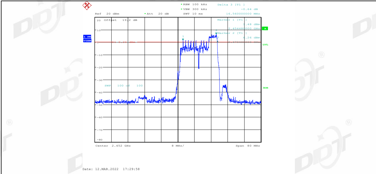
11AX40MIMO_Ant1_2452_106Tone_RU53
