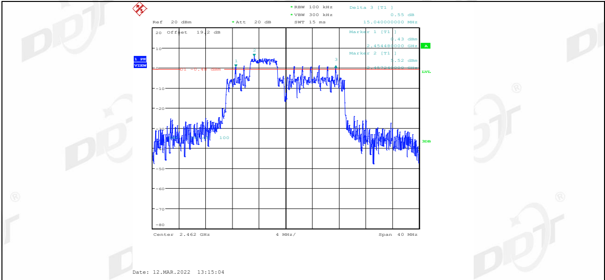
11AX20MIMO_Ant1_2462_52Tone_RU39
