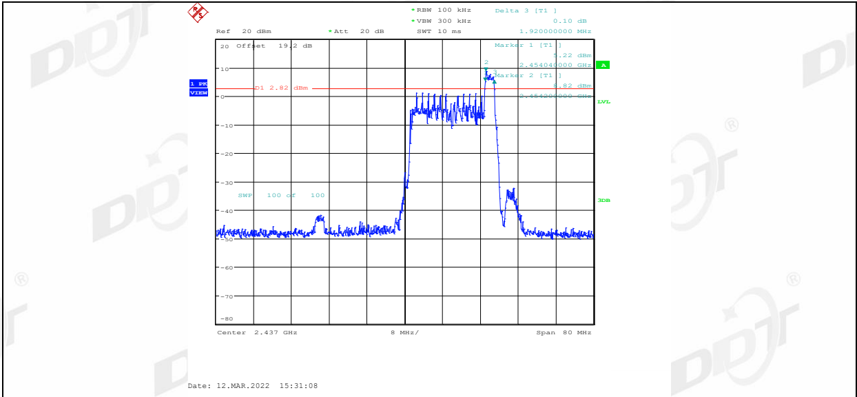
11AX40MIMO_Ant1_2437_52Tone_RU37
