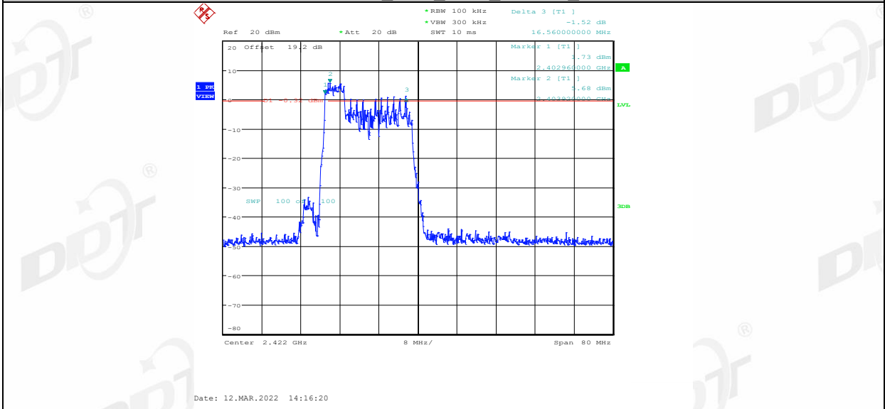
11AX40MIMO_Ant2_2422_52Tone_RU40
