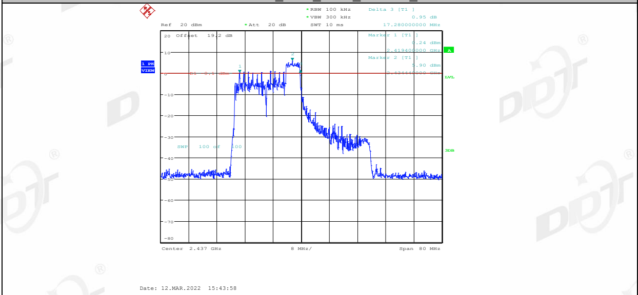
11AX40MIMO_Ant1_2437_52Tone_RU44
