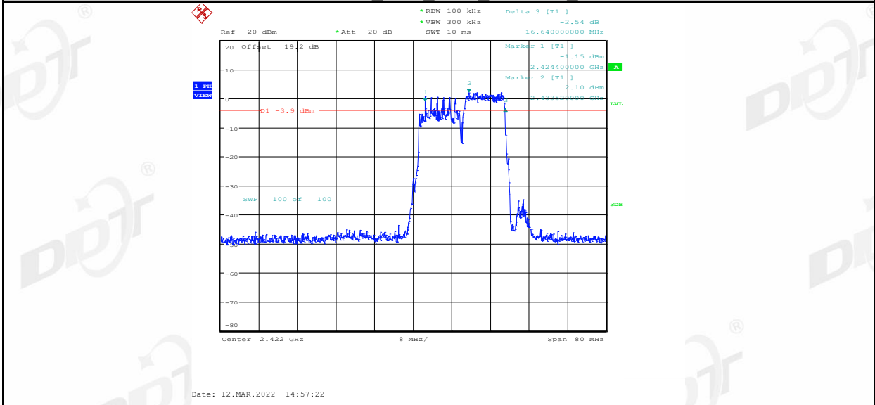
11AX40MIMO_Ant2_2422_242Tone_RU61
