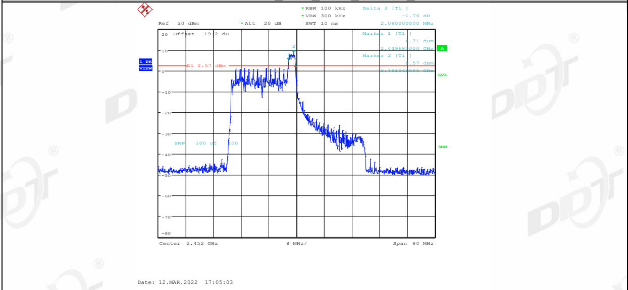
11AX40MIMO_Ant2_2452_26Tone_RU17
