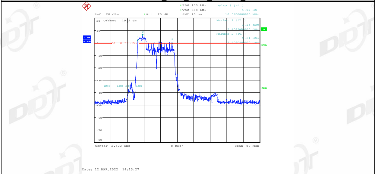
11AX40MIMO_Ant1_2422_52Tone_RU40
