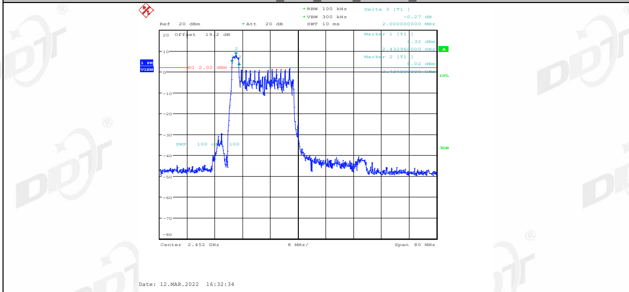
11AX40MIMO_Ant1_2452_26Tone_RU8
