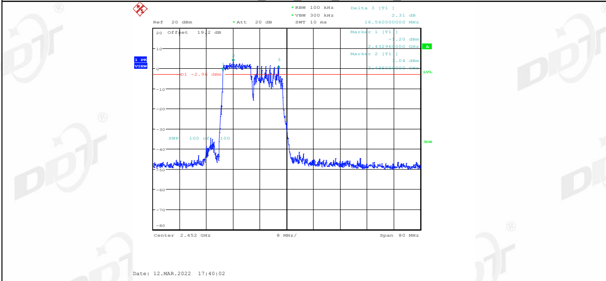
11AX40MIMO_Ant2_2452_106Tone_RU54
