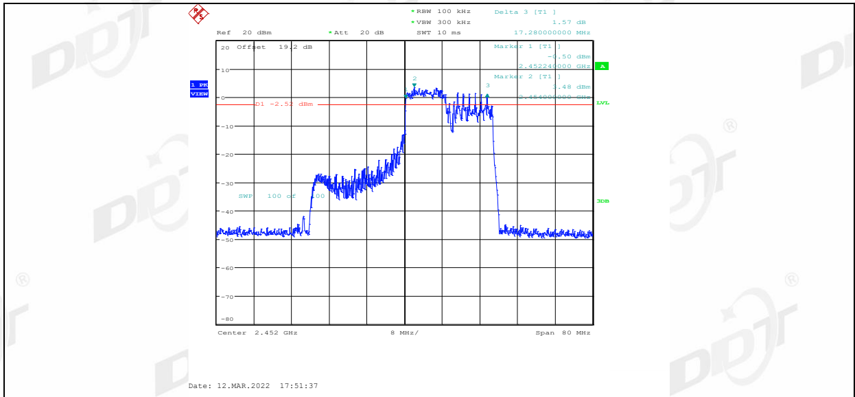
11AX40MIMO_Ant1_2452_106Tone_RU56
