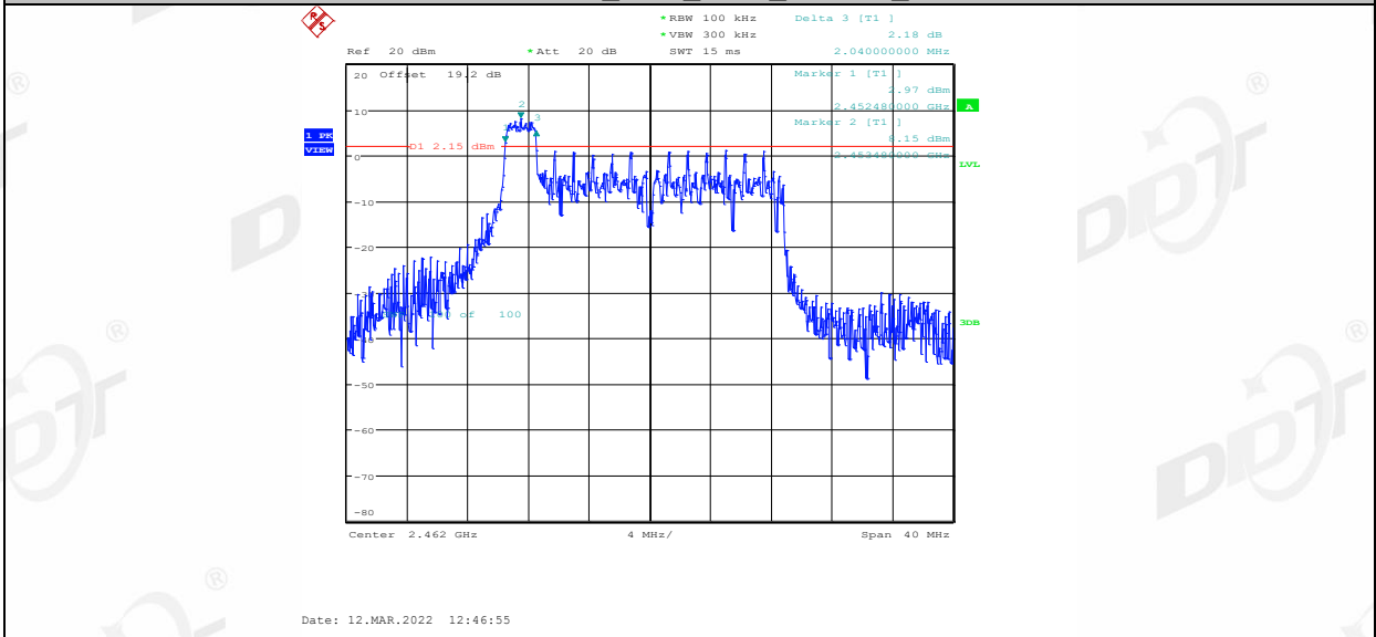
11AX20MIMO_Ant1_2462_26Tone_RU4
