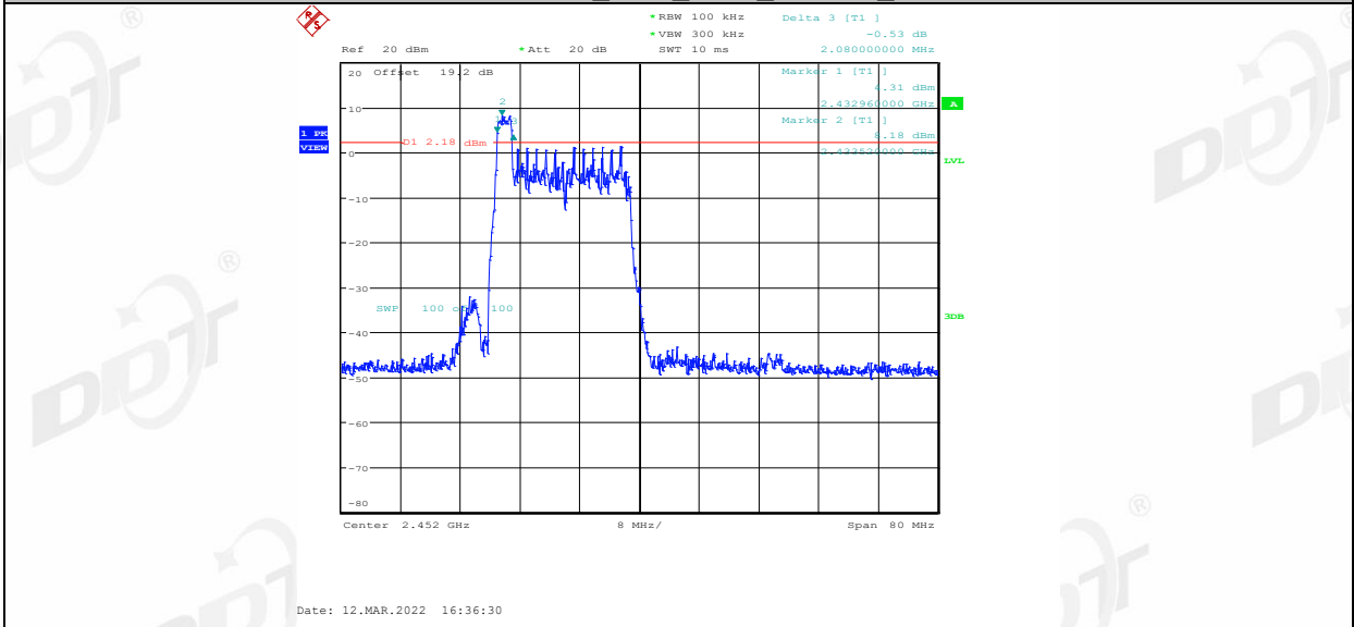
11AX40MIMO_Ant2_2452_26Tone_RU8
