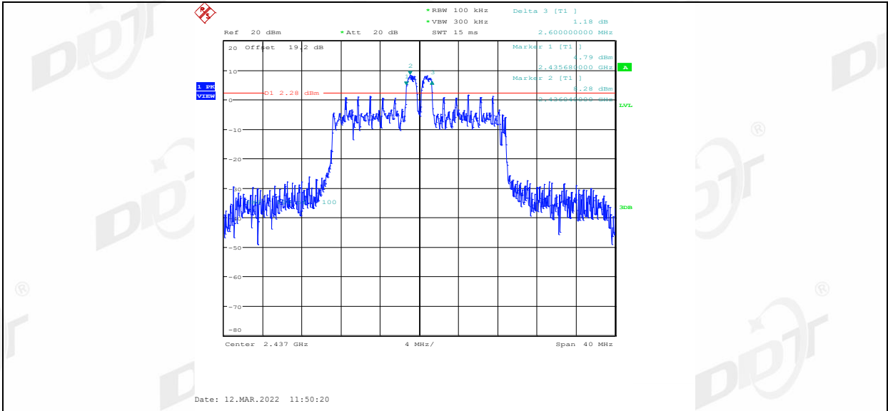
11AX20MIMO_Ant2_2437_26Tone_RU8
