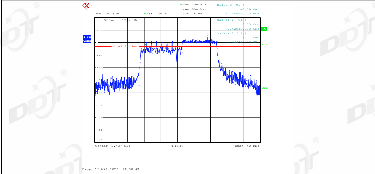
11AX20MIMO_Ant2_2437_26Tone_RU0
