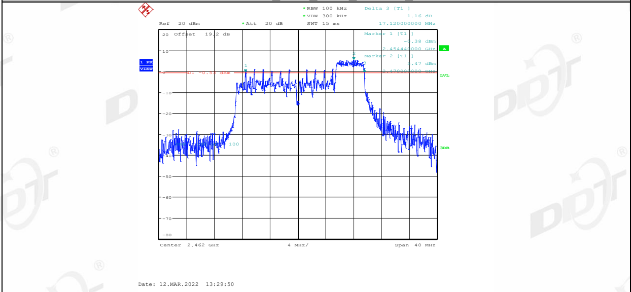
11AX20MIMO_Ant1_2462_106Tone_RU53
