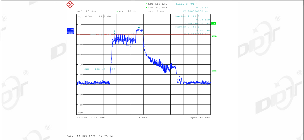
11AX40MIMO_Ant2_2422_52Tone_RU44
