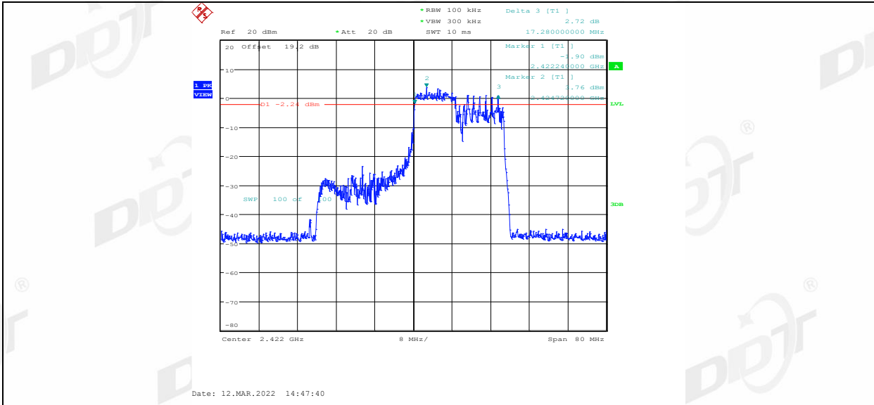
11AX40MIMO_Ant1_2422_106Tone_RU56
