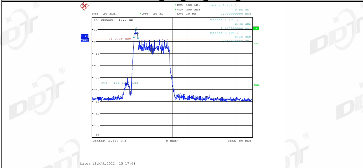
11AX40MIMO_Ant2_2437_26Tone_RU8
