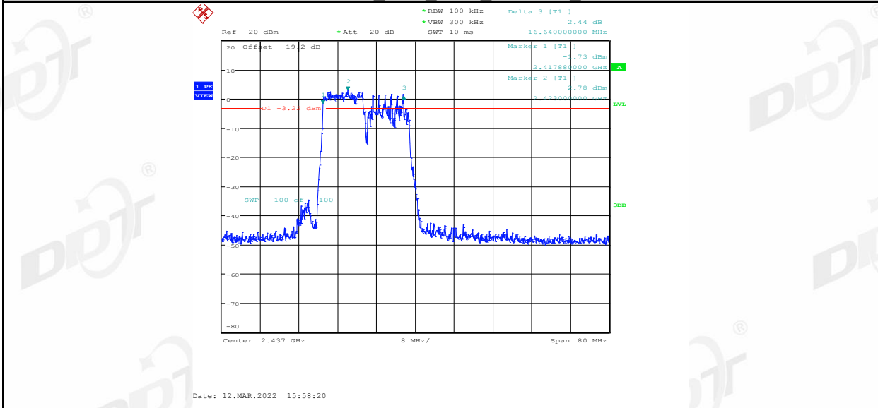
11AX40MIMO_Ant2_2437_106Tone_RU54
