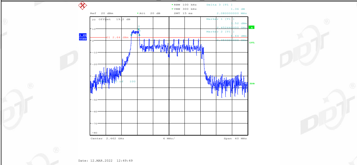
11AX20MIMO_Ant2_2462_26Tone_RU4
