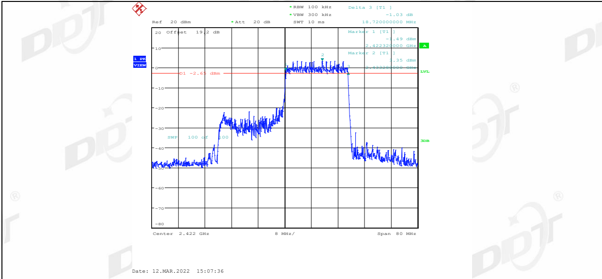
11AX40MIMO_Ant2_2422_26Tone_RU0
