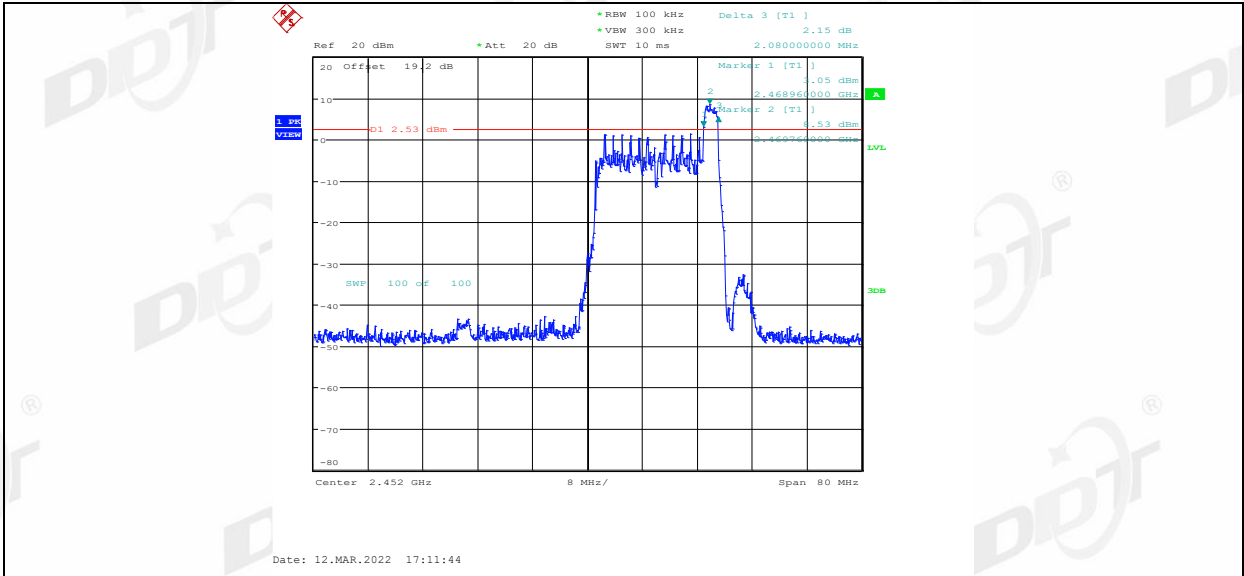
11AX40MIMO_Ant2_2452_52Tone_RU37
