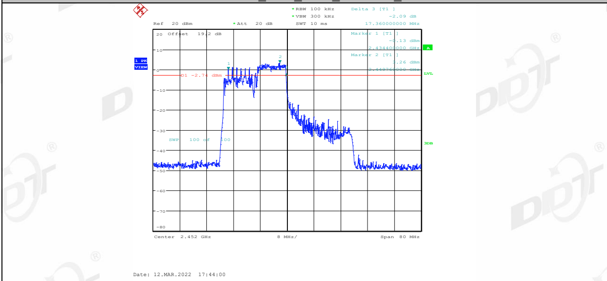
11AX40MIMO_Ant1_2452_106Tone_RU55
