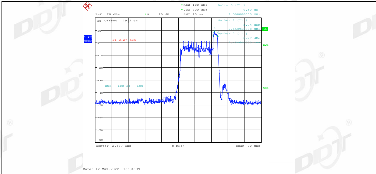
11AX40MIMO_Ant2_2437_52Tone_RU37
