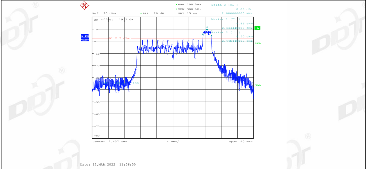
11AX20MIMO_Ant2_2437_52Tone_RU37
