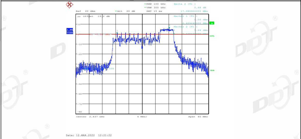
11AX20MIMO_Ant2_2437_106Tone_RU53
