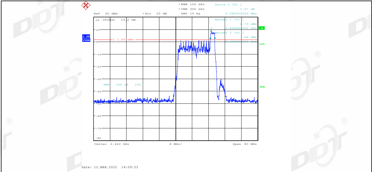
11AX40MIMO_Ant2_2422_52Tone_RU37
