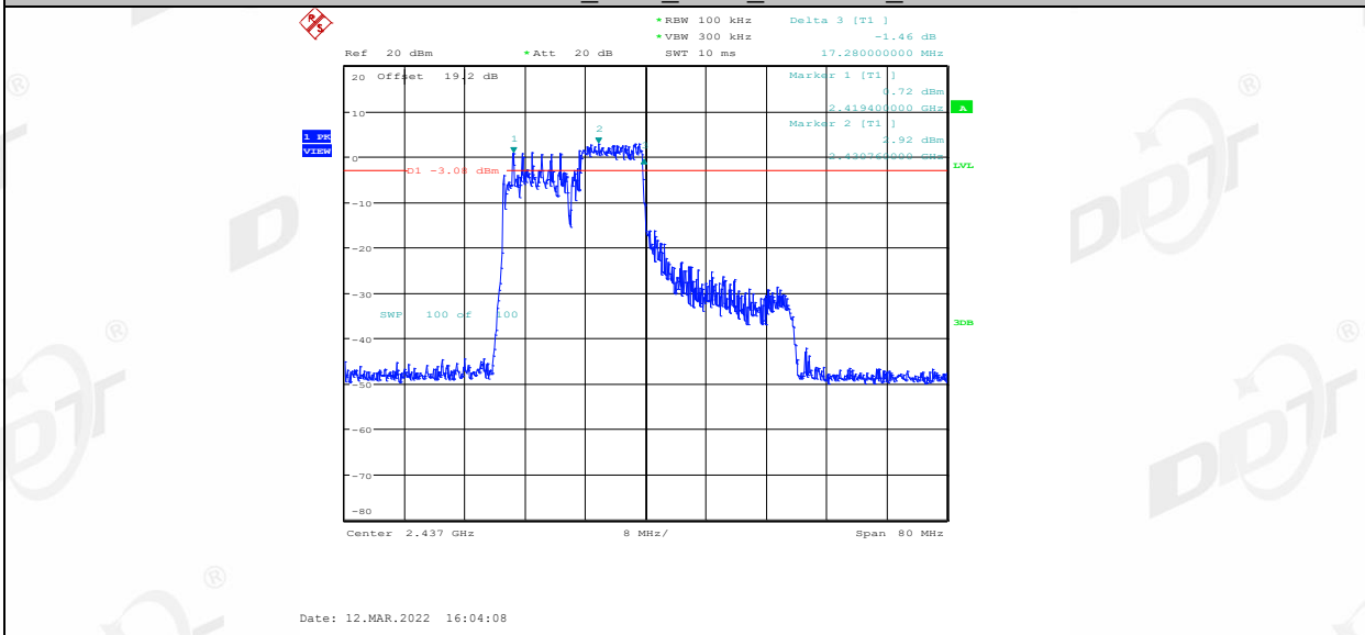
11AX40MIMO_Ant2_2437_106Tone_RU55
