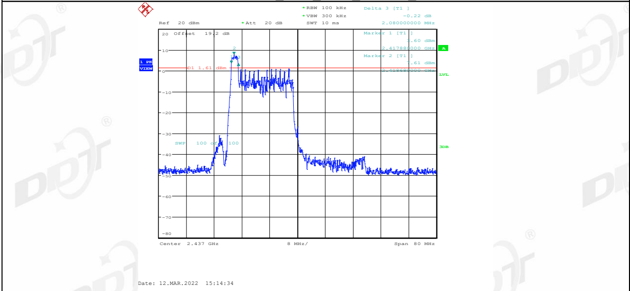
11AX40MIMO_Ant1_2437_26Tone_RU8
