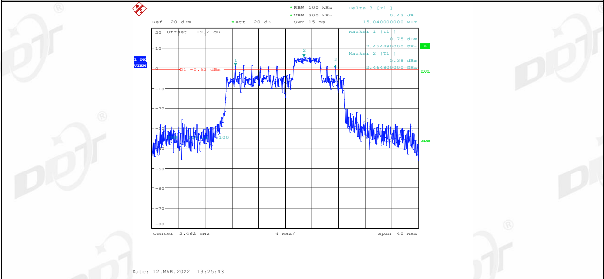
11AX20MIMO_Ant2_2462_106Tone_RU53
