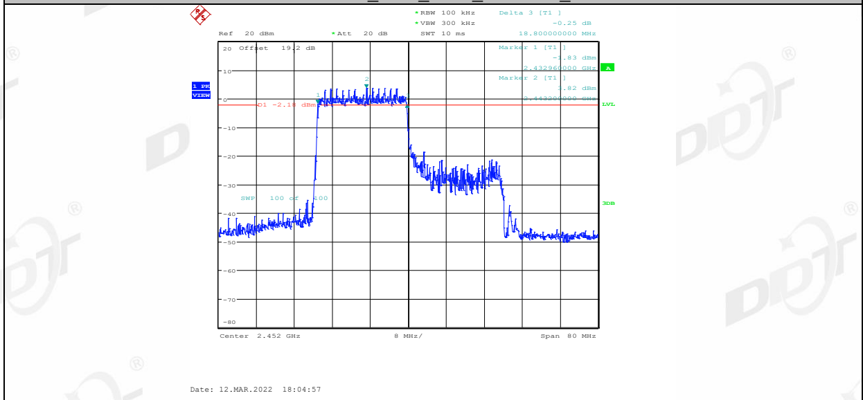
11AX40MIMO_Ant1_2452_242Tone_RU62
