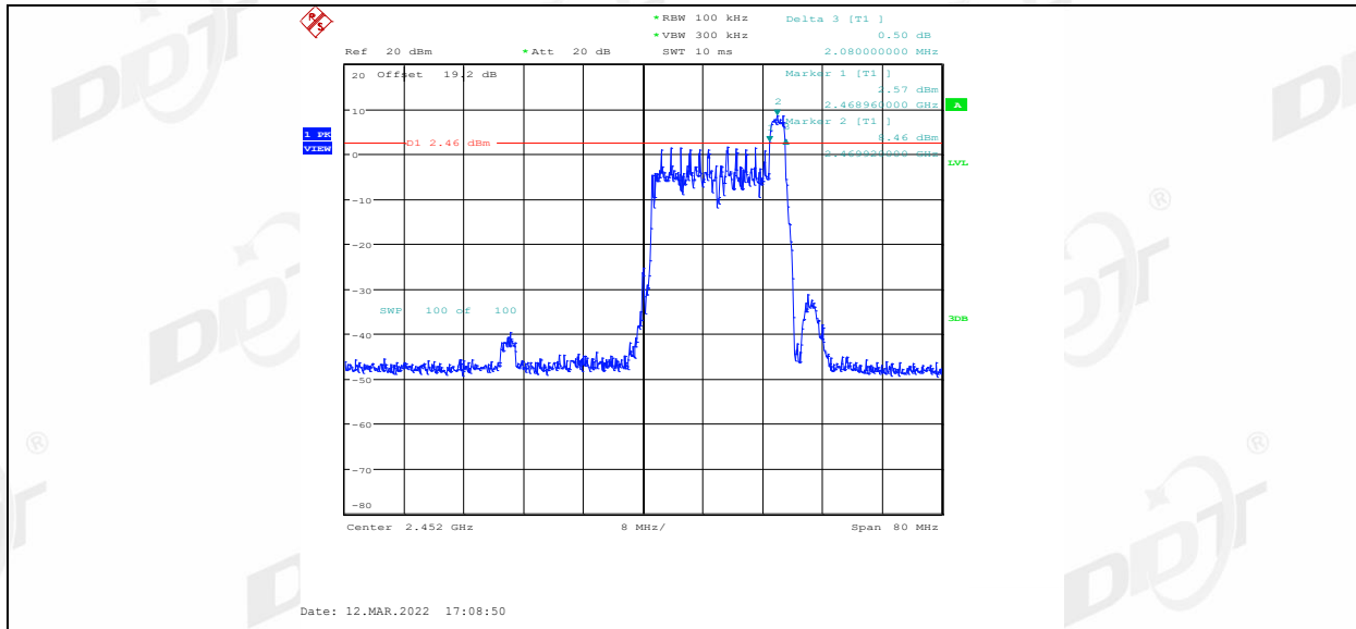
11AX40MIMO_Ant1_2452_52Tone_RU37
