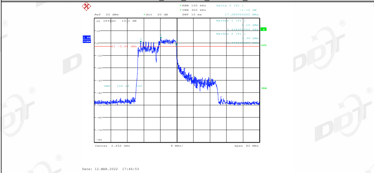
11AX40MIMO_Ant2_2452_106Tone_RU55
