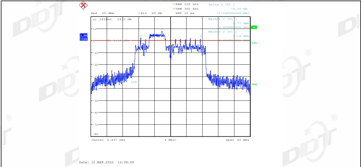
11AX20MIMO_Ant2_2437_52Tone_RU39
