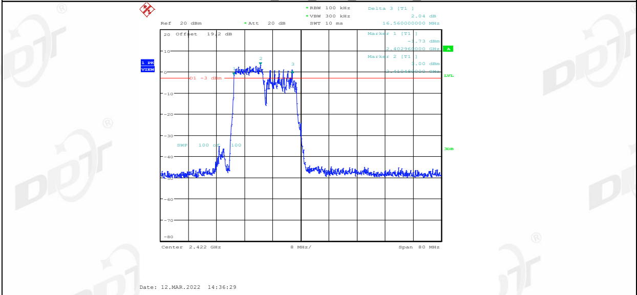
11AX40MIMO_Ant2_2422_106Tone_RU54
