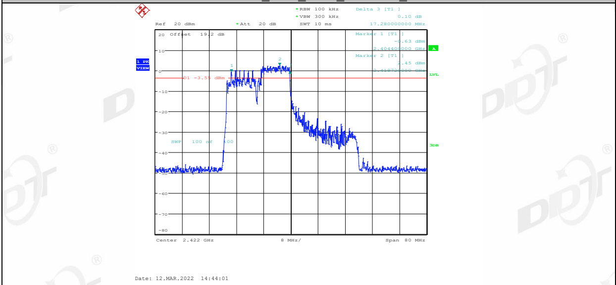
11AX40MIMO_Ant2_2422_106Tone_RU55
