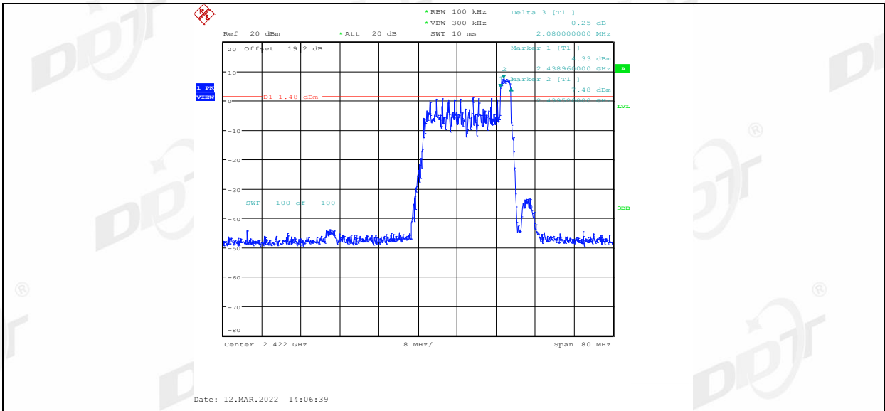
11AX40MIMO_Ant1_2422_52Tone_RU37
