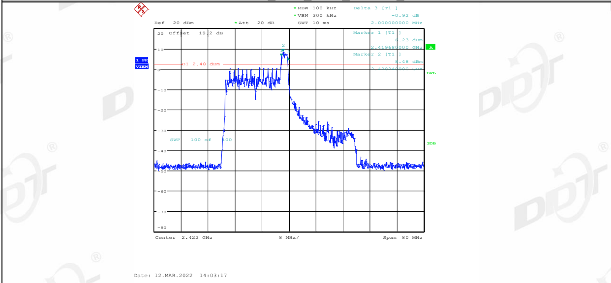
11AX40MIMO_Ant2_2422_26Tone_RU17
