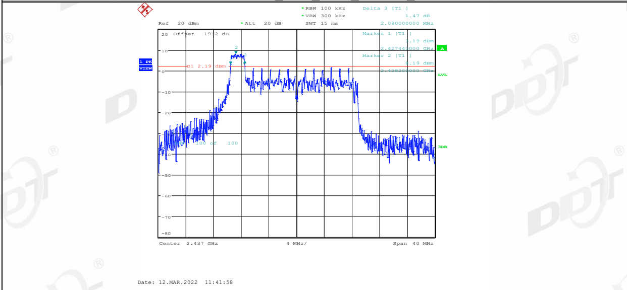
11AX20MIMO_Ant2_2437_26Tone_RU4
