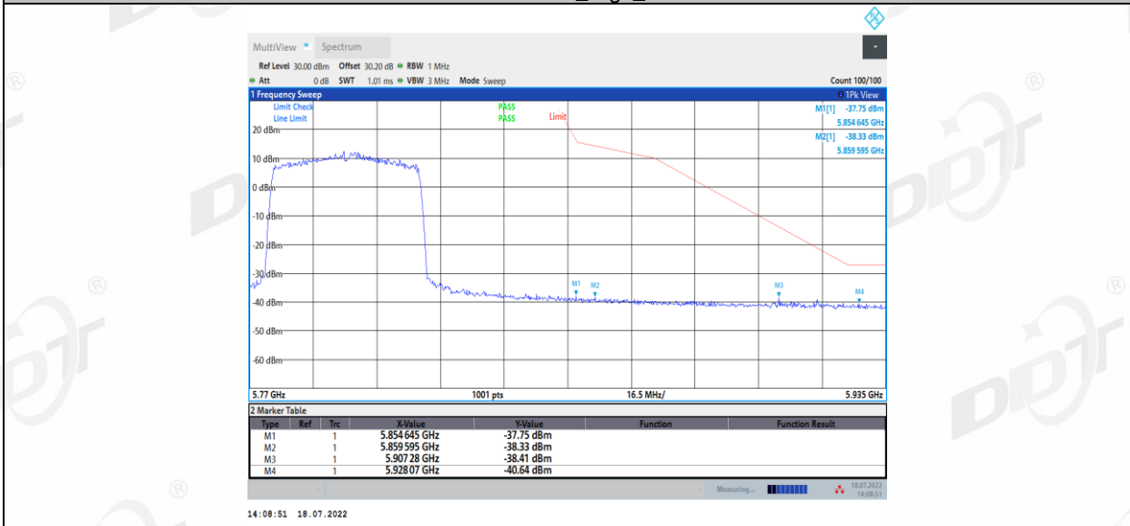
11AX80MIMO_Low_5775
