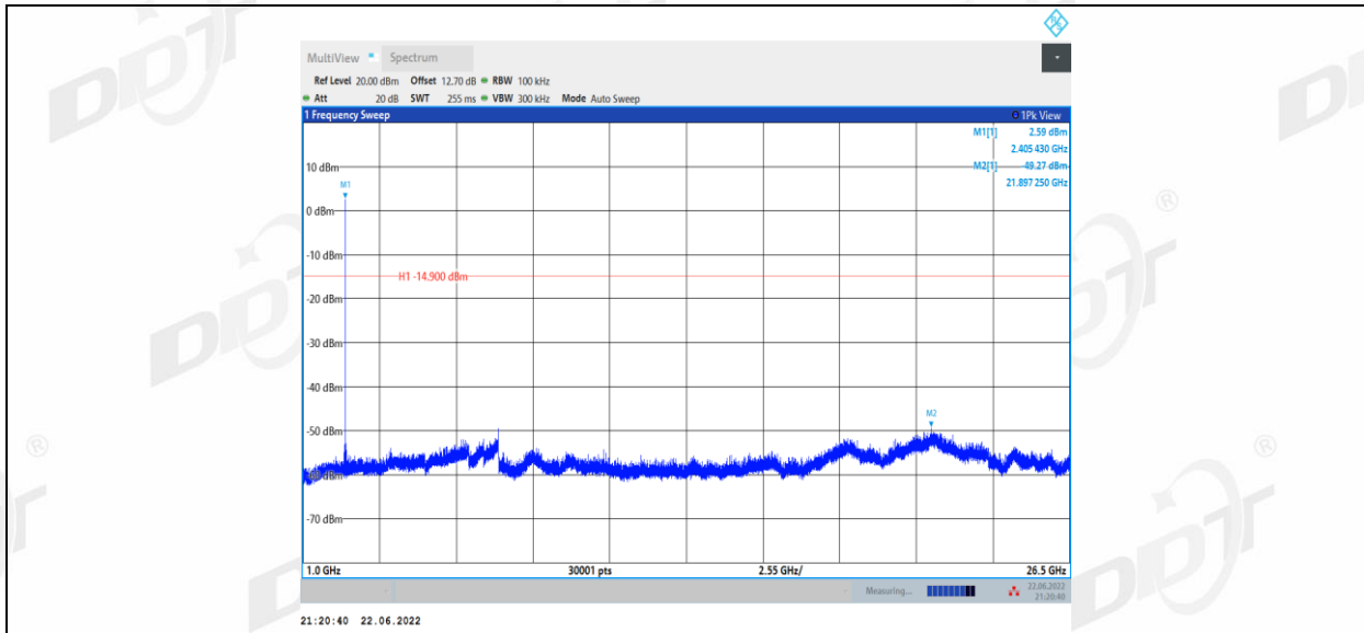
GFSK_Ant1_2442_0~Reference
