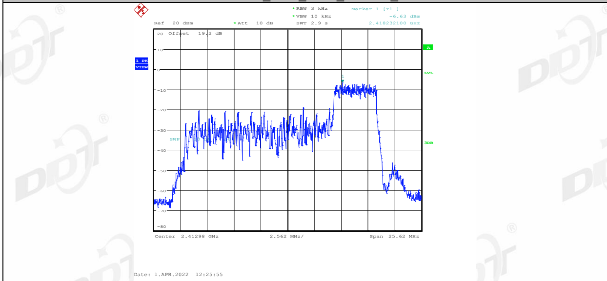
11AX20MIMO_Ant1_2412_106Tone_RU53
