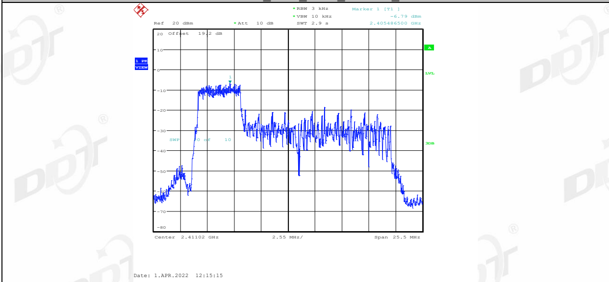
11AX20MIMO_Ant1_2412_52Tone_RU38
