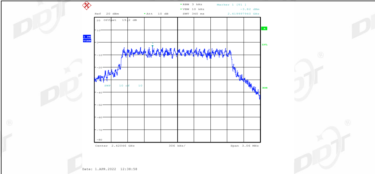
11AX20MIMO_Ant2_2412_52Tone_RU37
