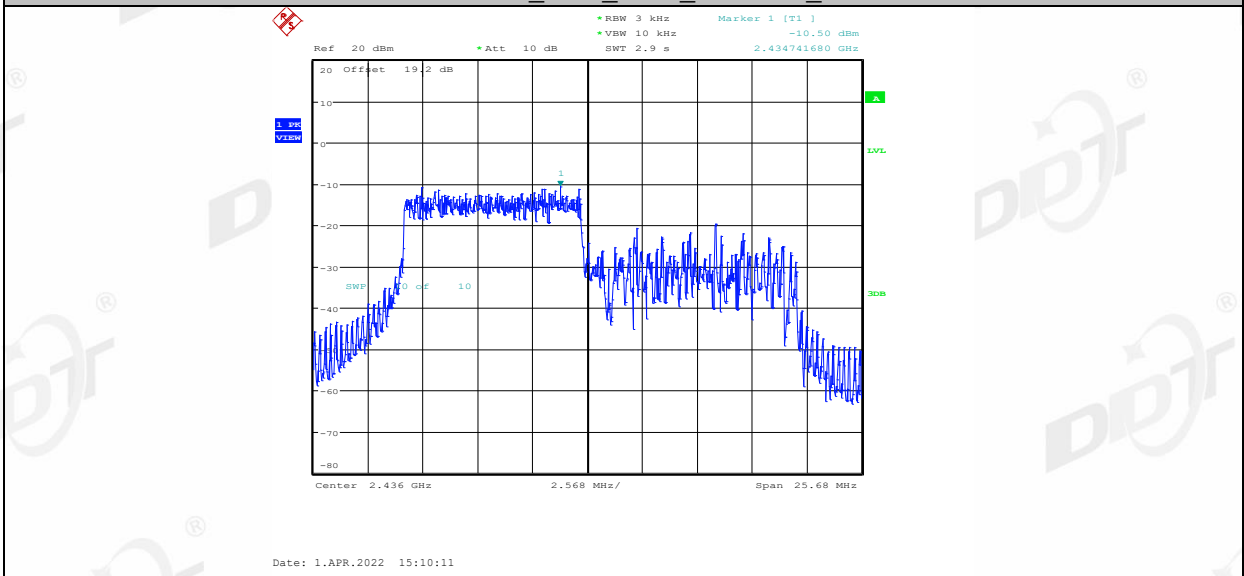
11AX20MIMO_Ant1_2437_106Tone_RU54
