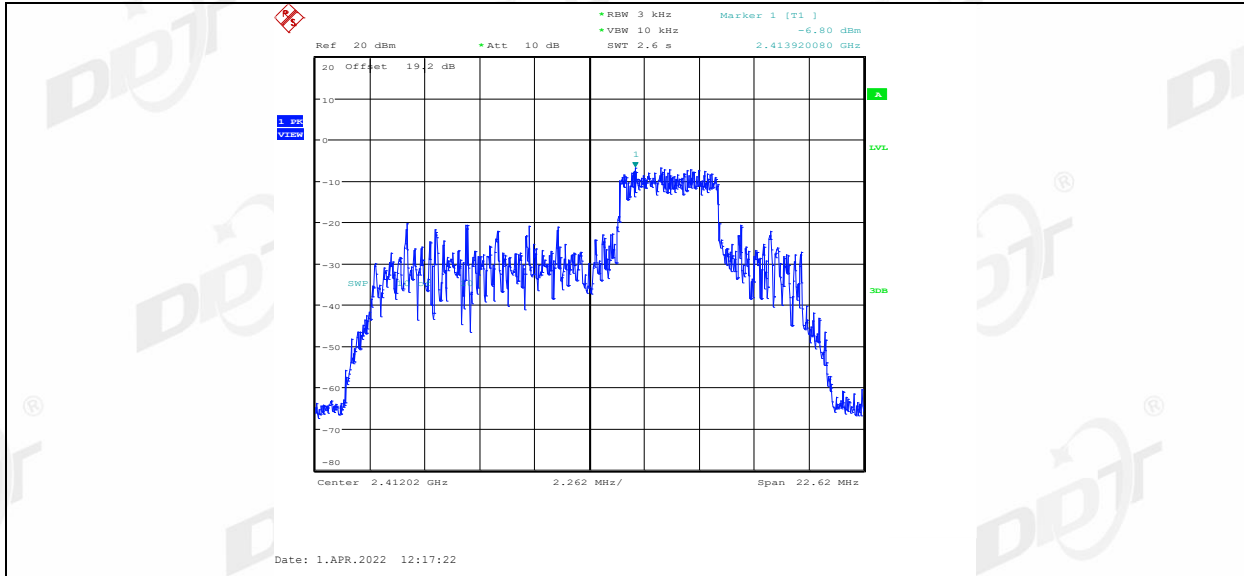
11AX20MIMO_Ant1_2412_52Tone_RU40
