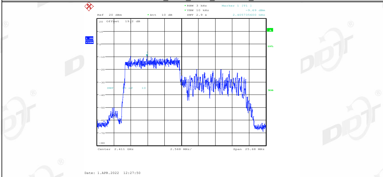
11AX20MIMO_Ant1_2412_106Tone_RU54
