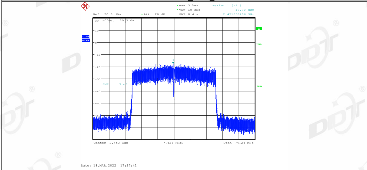
11AX40MIMO_Ant2_2452
