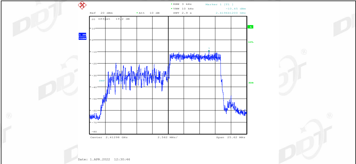
11AX20MIMO_Ant2_2412_26Tone_RU0
