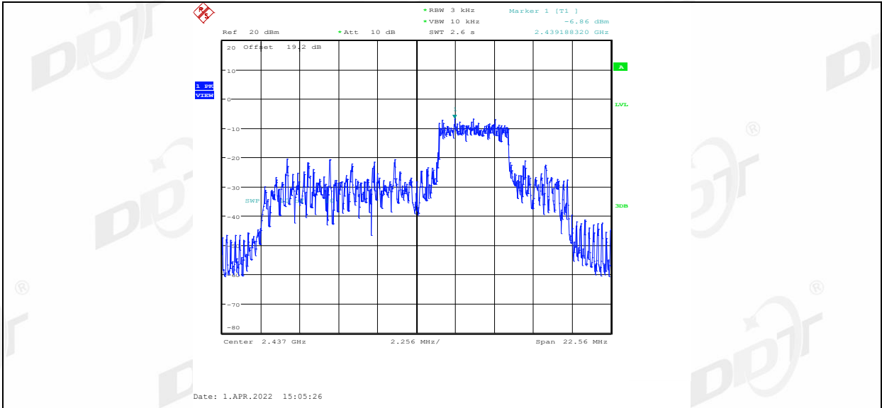
11AX20MIMO_Ant1_2437_52Tone_RU40
