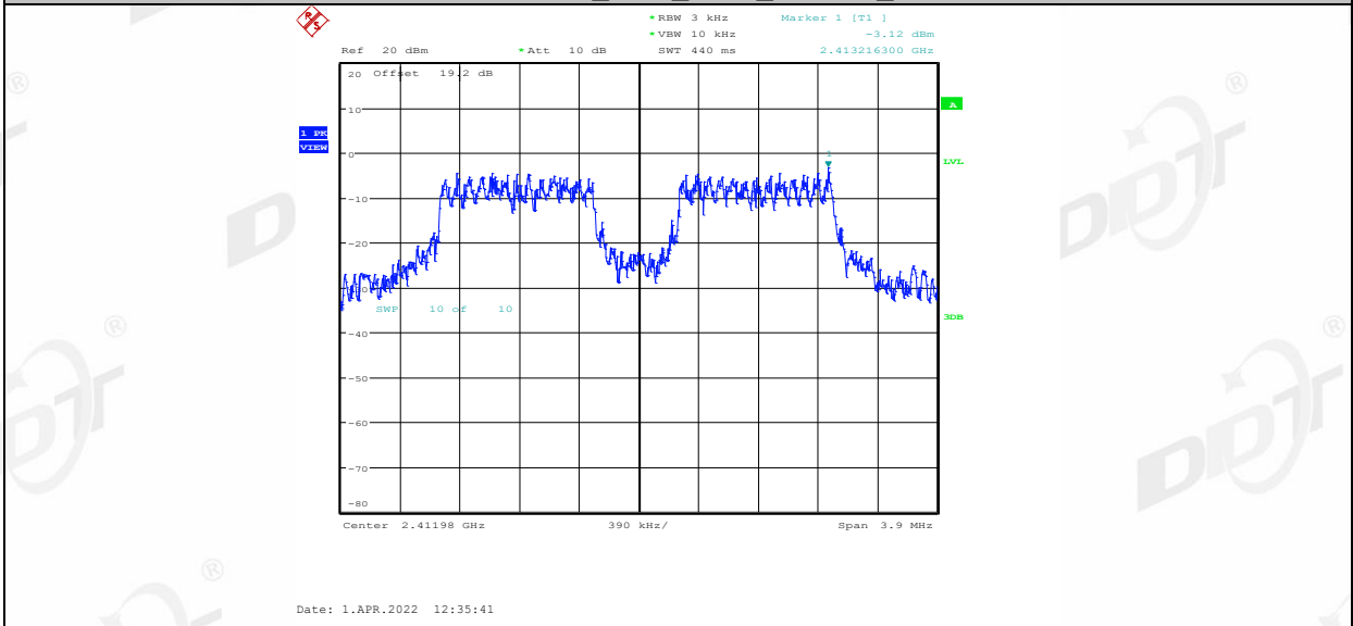
11AX20MIMO_Ant2_2412_26Tone_RU8
