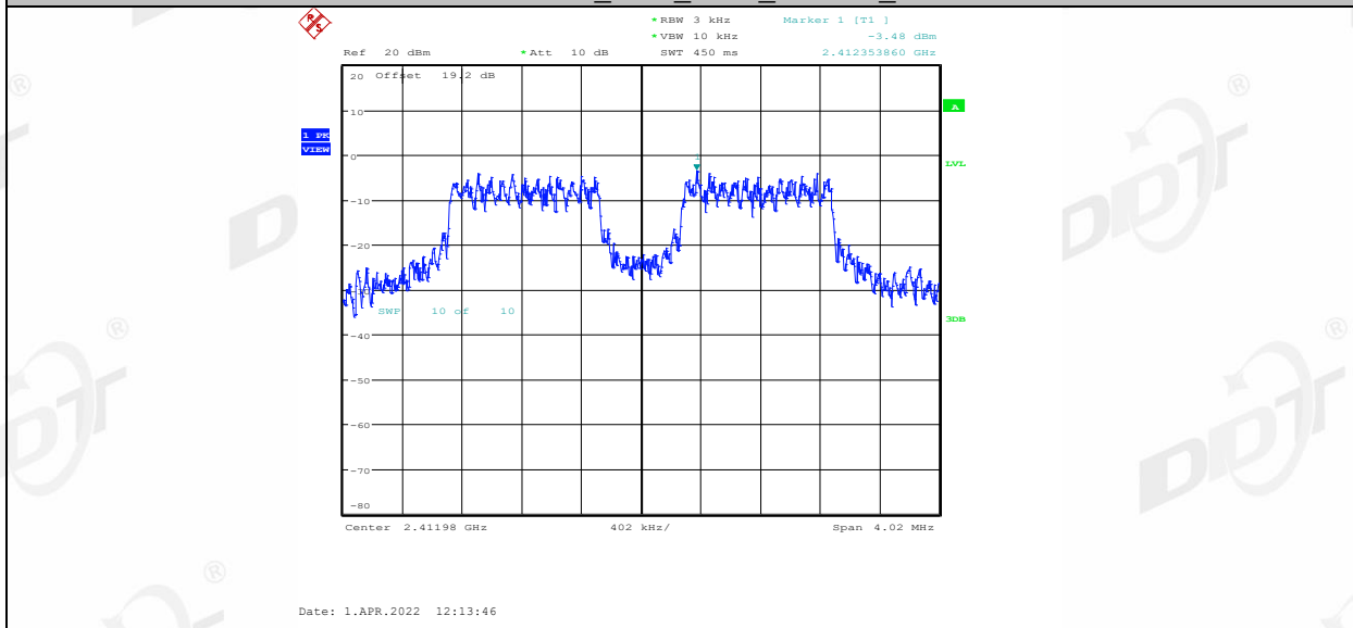
11AX20MIMO_Ant1_2412_26Tone_RU8
