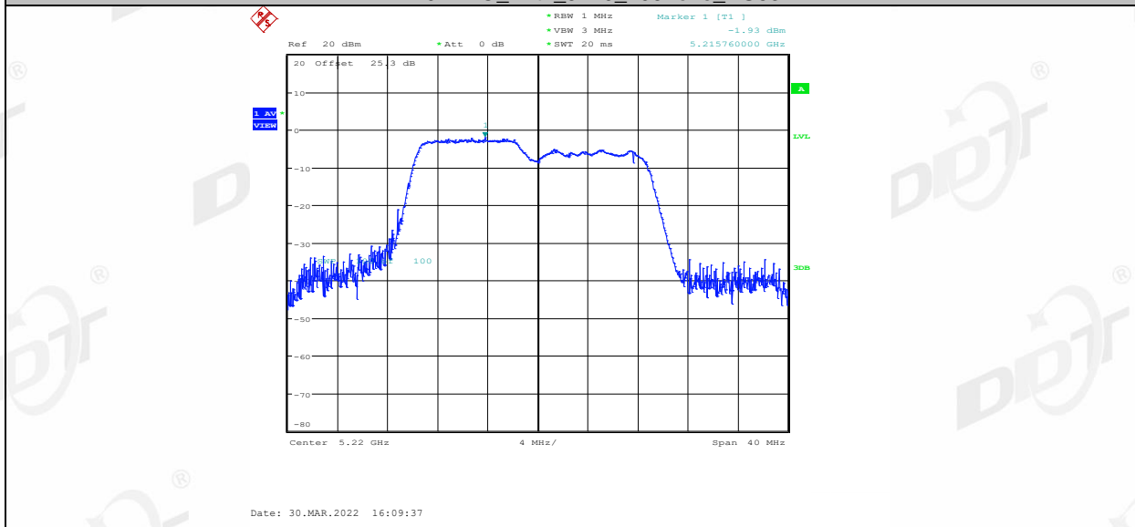
11AX20MIMO_Ant1_5220_106Tone_RU54
