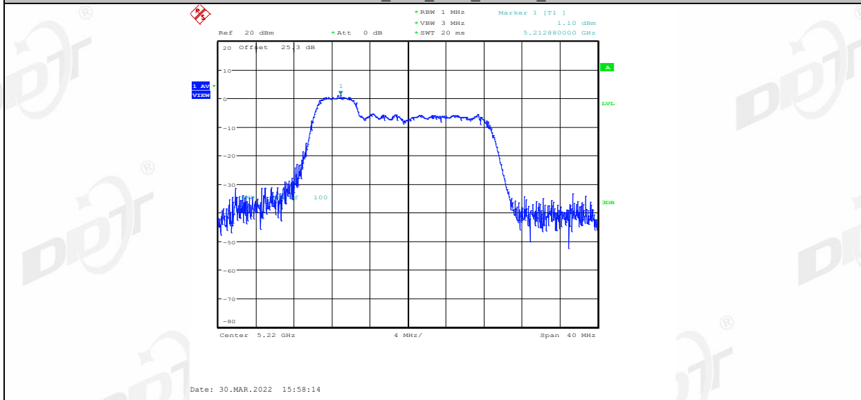
11AX20MIMO_Ant1_5220_52Tone_RU38
