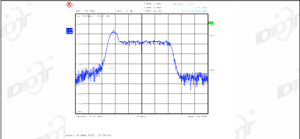
11AX20MIMO_Ant2_5220_26Tone_RU4
