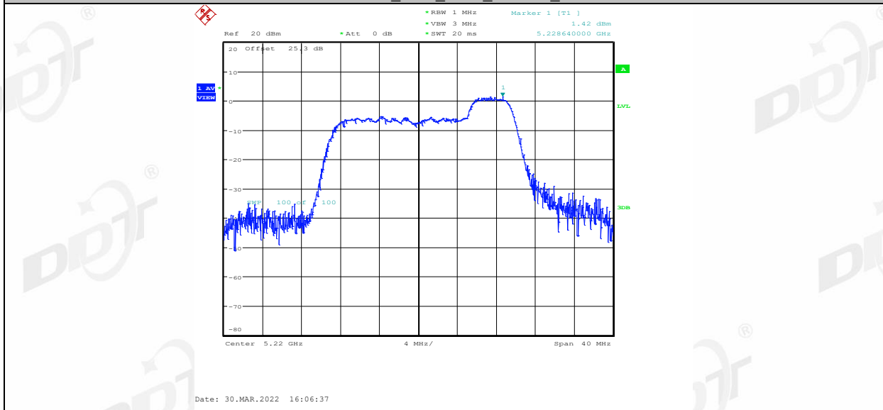
11AX20MIMO_Ant1_5220_106Tone_RU53
