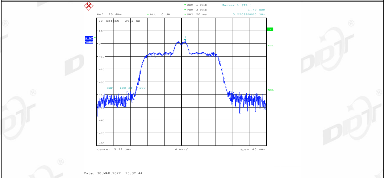
11AX20MIMO_Ant2_5220_26Tone_RU8
