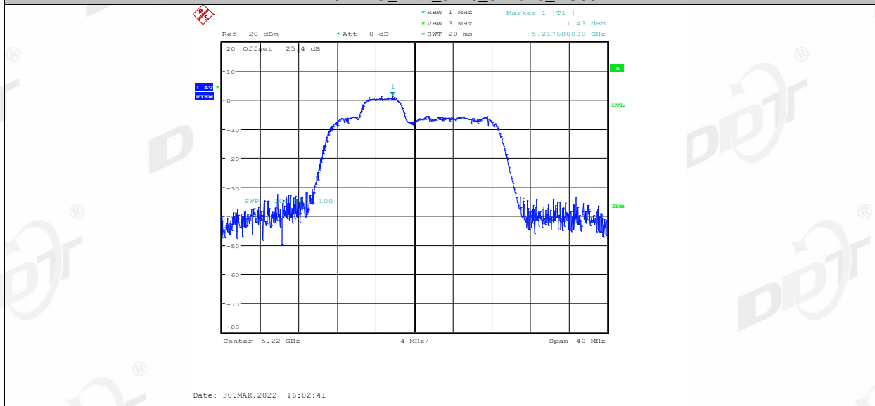
11AX20MIMO_Ant1_5220_52Tone_RU39
