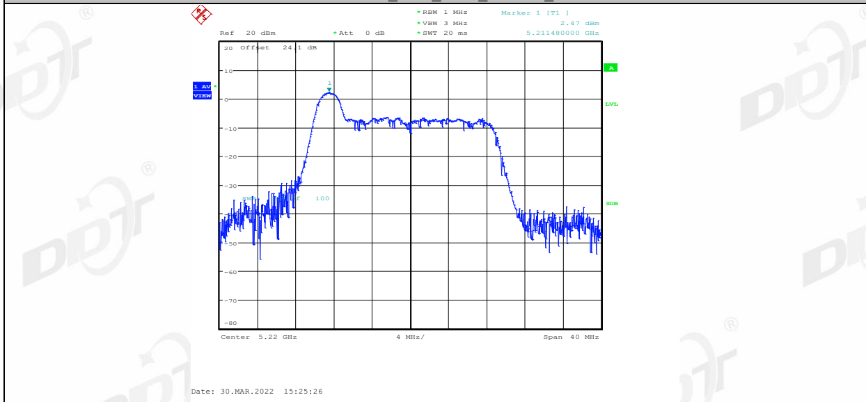
11AX20MIMO_Ant1_5220_26Tone_RU4
