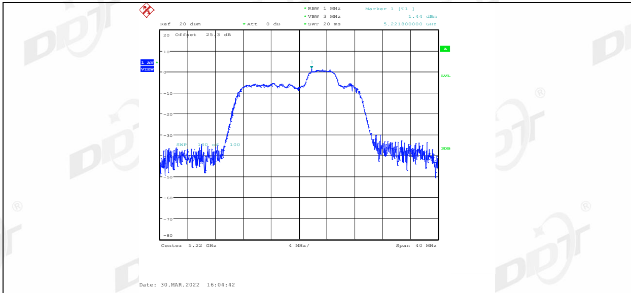
11AX20MIMO_Ant1_5220_52Tone_RU40
