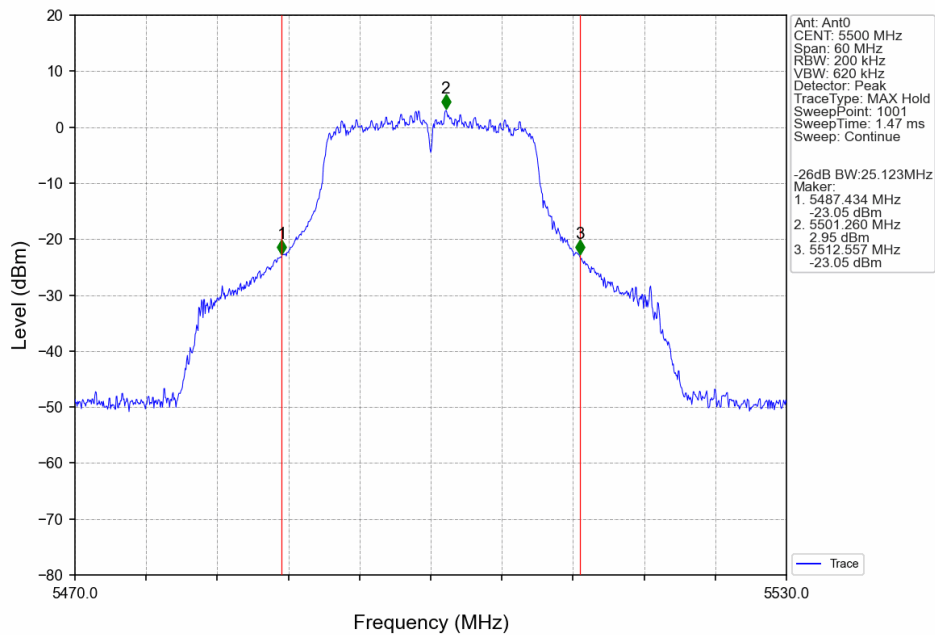
802.11ac(VHT20)_LCH_5500MHz_Ant0_NTNV
