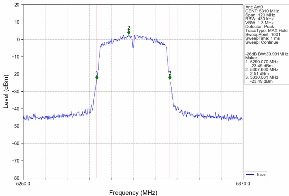
802.11n(HT40)_HCH_5310MHz_Ant0_NTNV
