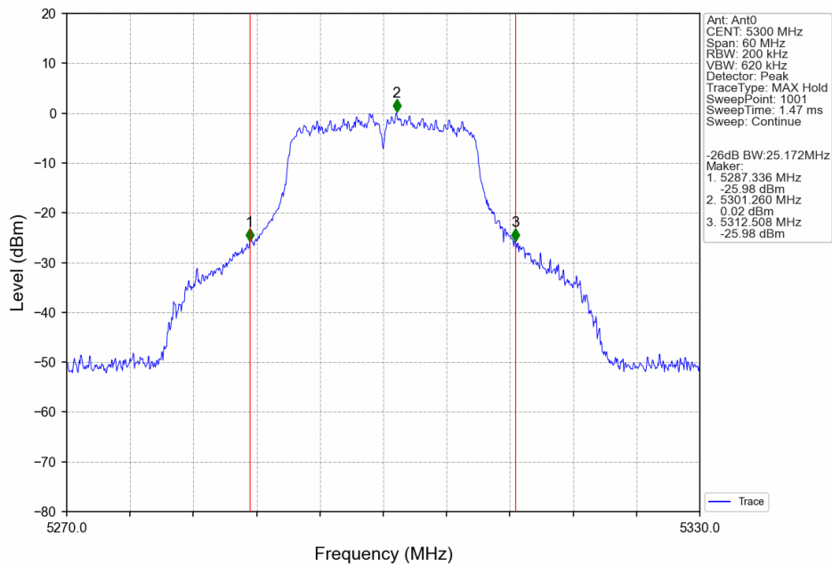
802.11ac(VHT20)_MCH_5300MHz_Ant0_NTNV
