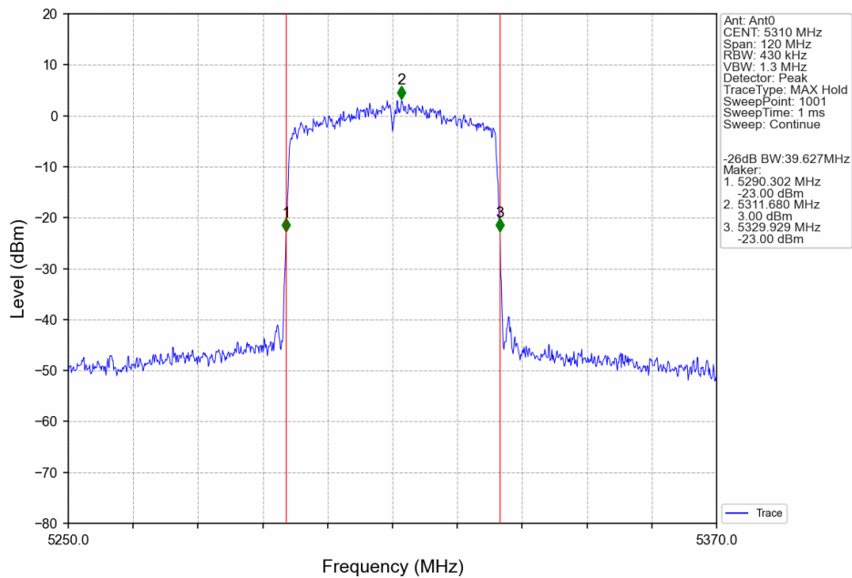
802.11ax(HEW40)_HCH_5310MHz_RU484_Left_Ant0_NTNV
