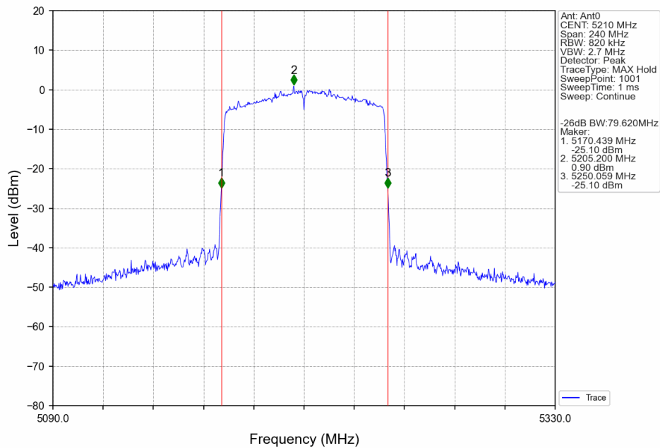
802.11ac(VHT80)_MCH_5210MHz_Ant0_NTNV
