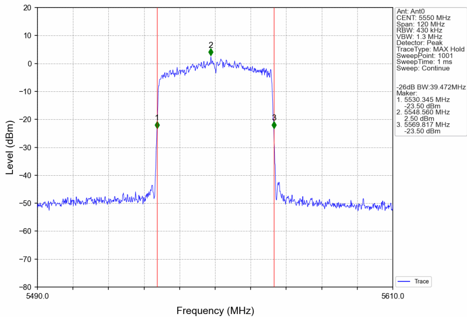
802.11ax(HEW40)_MCH_5550MHz_RU484_Left_Ant0_NTNV
