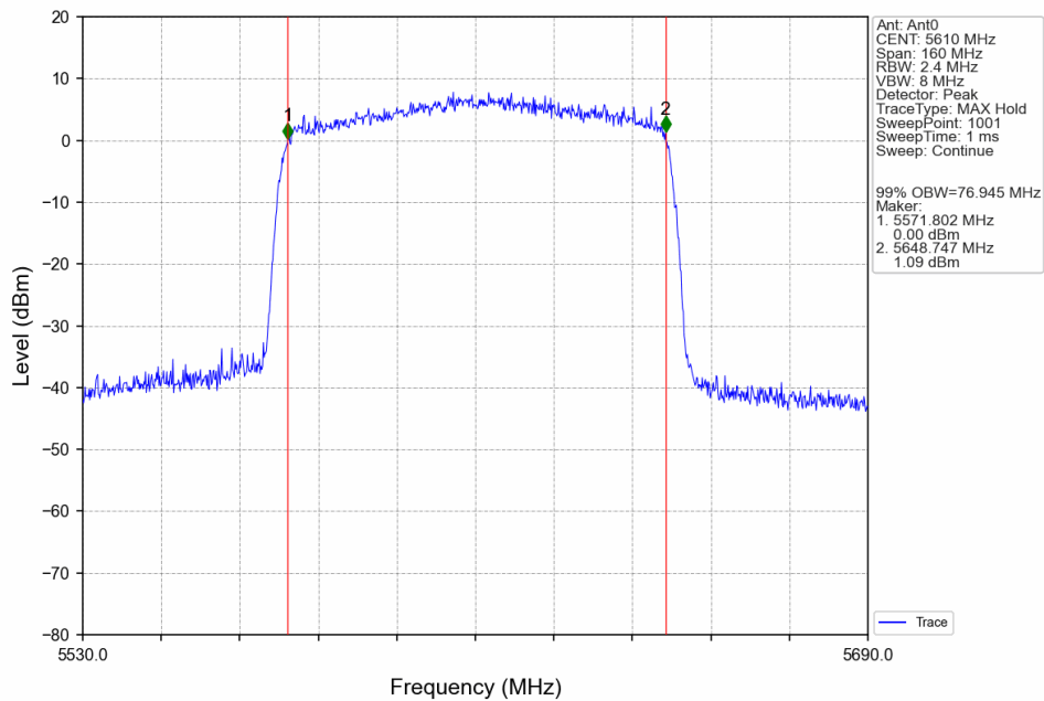
802.11ax(HEW80)_HCH_5610MHz_RU996_Left_Ant0_NTNV
