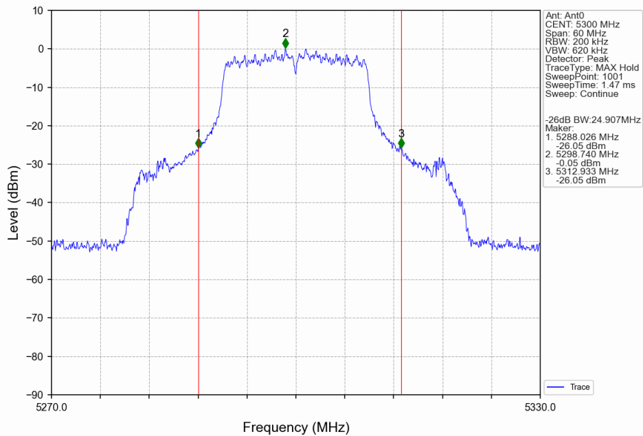
802.11n(HT20)_MCH_5300MHz_Ant0_NTNV
