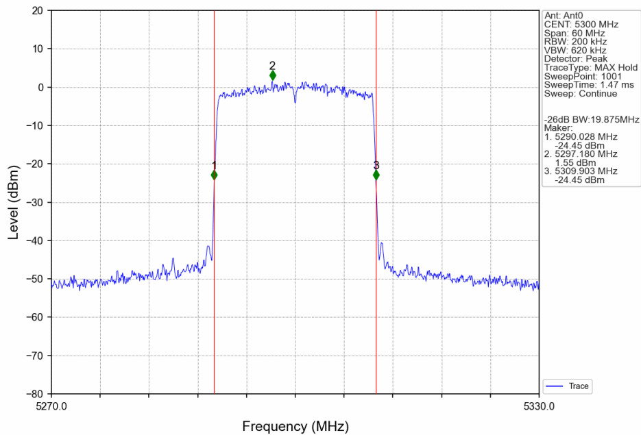
802.11ax(HEW20)_MCH_5300MHz_RU242_Left_Ant0_NTNV
