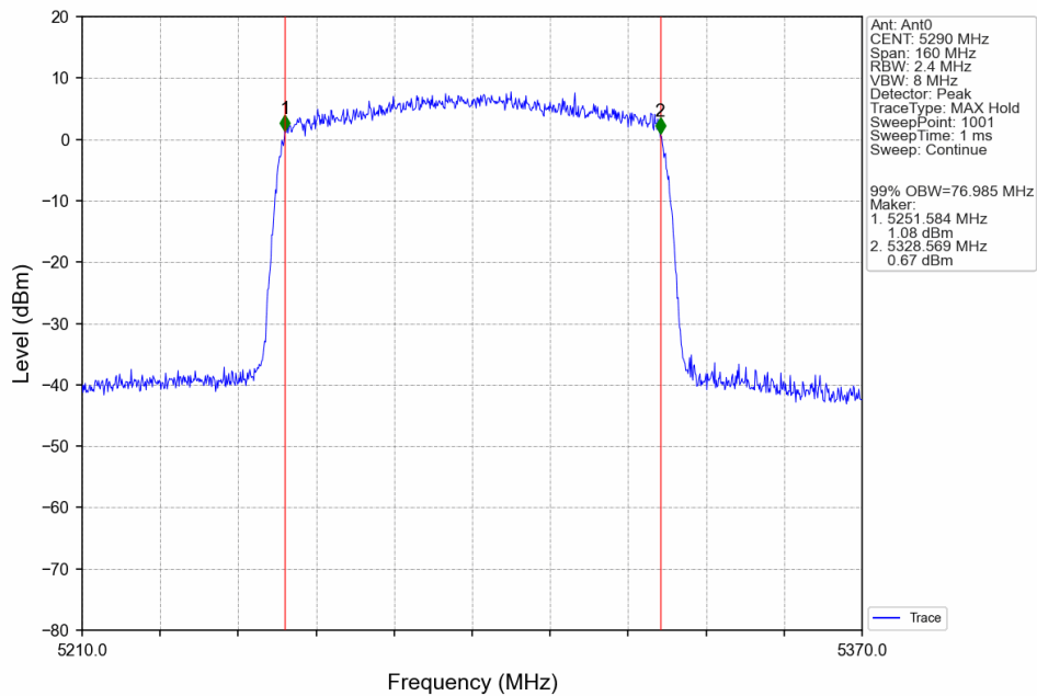
802.11ax(HEW80)_MCH_5290MHz_RU996_Left_Ant0_NTNV
