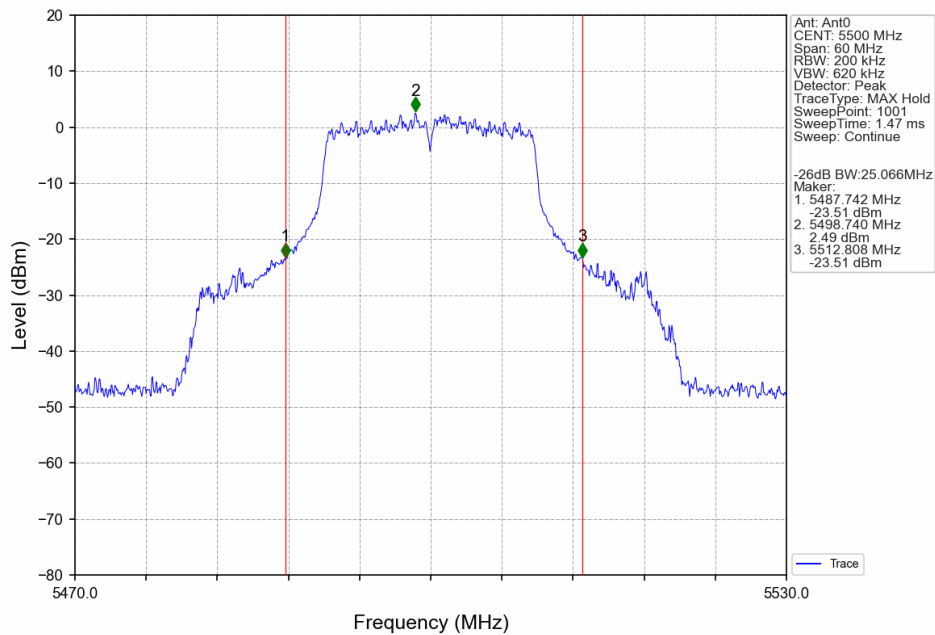
802.11n(HT20)_LCH_5500MHz_Ant0_NTNV
