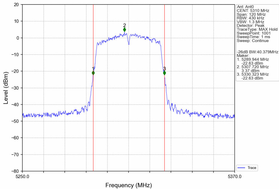
802.11ac(VHT40)_HCH_5310MHz_Ant0_NTNV
