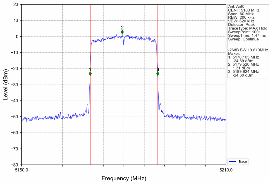
802.11ax(HEW20)_LCH_5180MHz_RU242_Left_Ant0_NTNV
