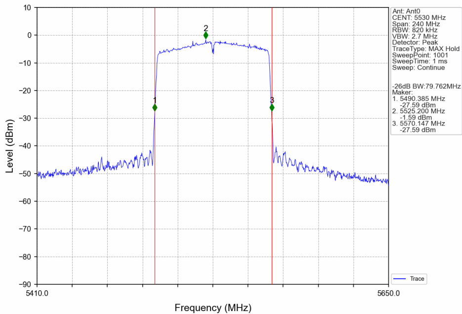
802.11ac(VHT80)_LCH_5530MHz_Ant0_NTNV
