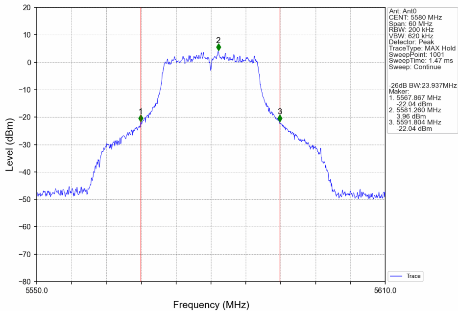
802.11a_MCH_5580MHz_Ant0_NTNV
