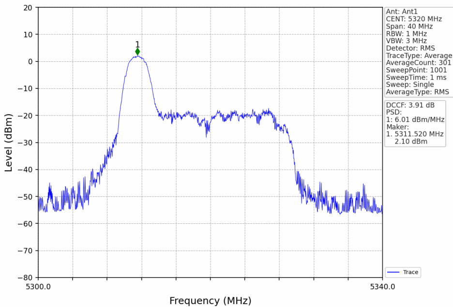
802.11ax(HEW20)_HCH_5320MHz_RU26_Left_Ant1_NTNV
