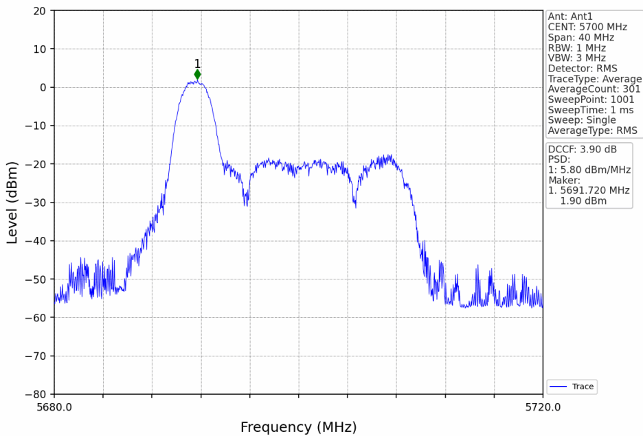
802.11ax(HEW20)_HCH_5700MHz_RU26_Left_Ant1_NTNV
