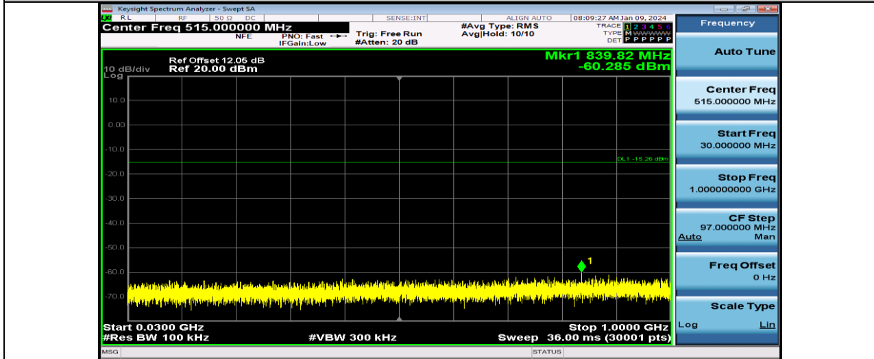
DH5-Ant1-2441-30~1000
