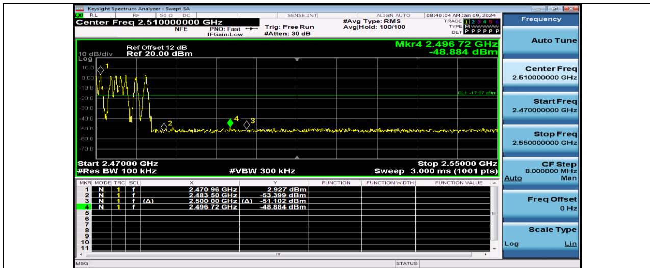
DH5-Ant1-Hop_2480
