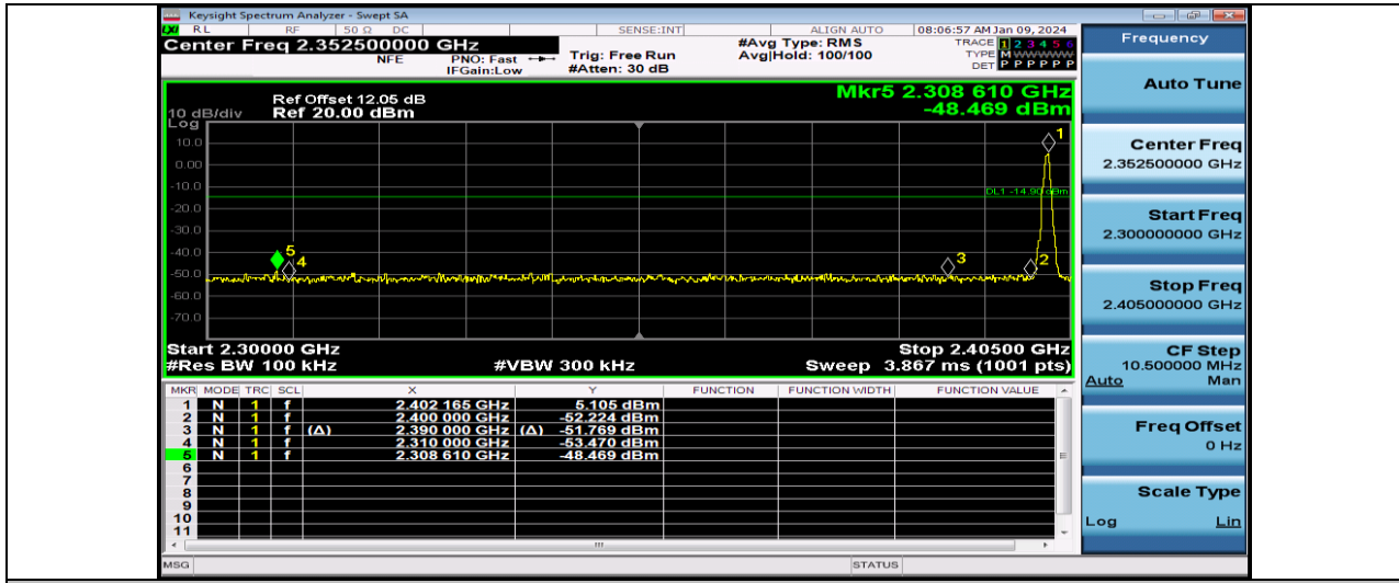
DH5-Ant1-2402
