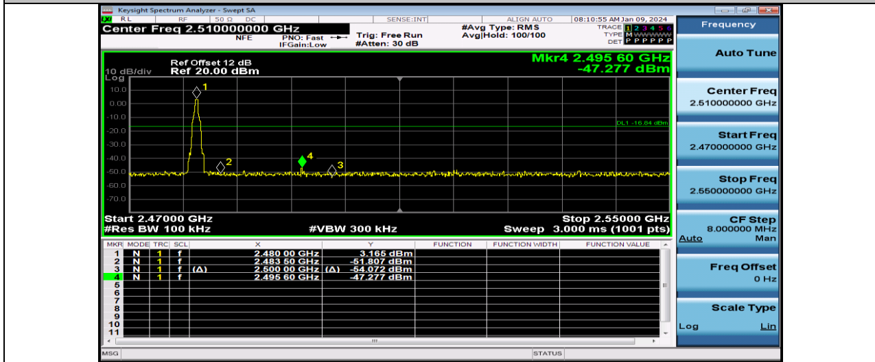
DH5-Ant1-2480
