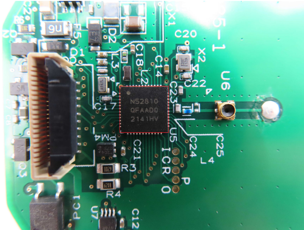
2.4G Module
