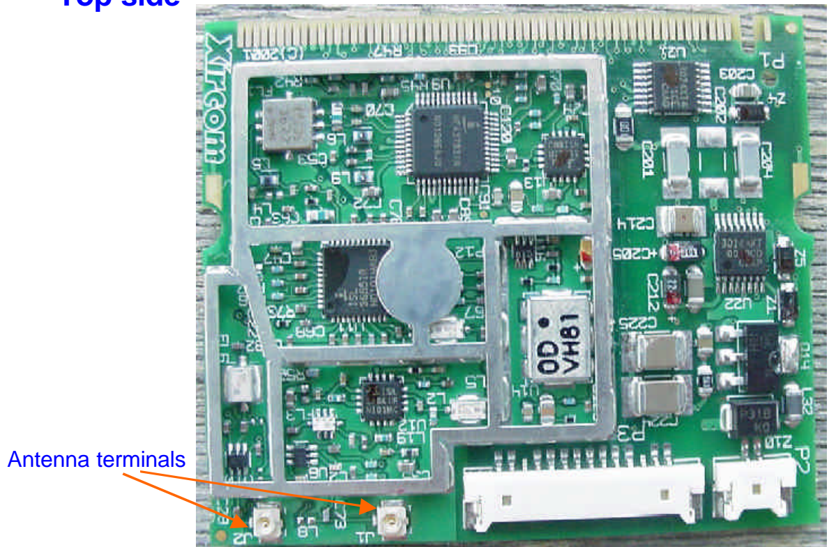
Top side
