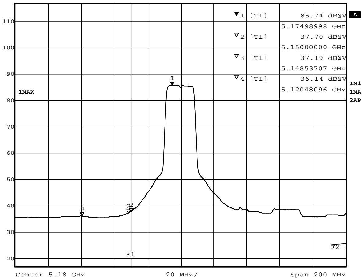
Plot 7-1-2 5180MHz TX mode (Average)
