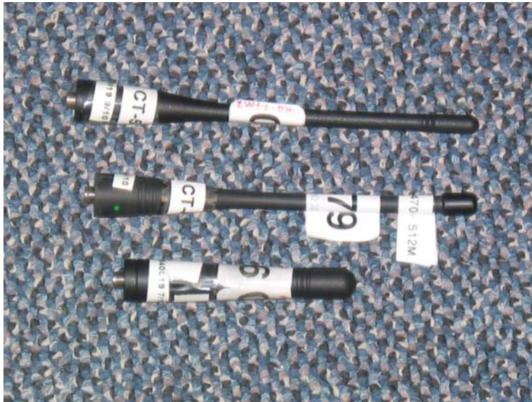
KRA-15M2, KRA-23M2, & KRA-27M2 Antennas
