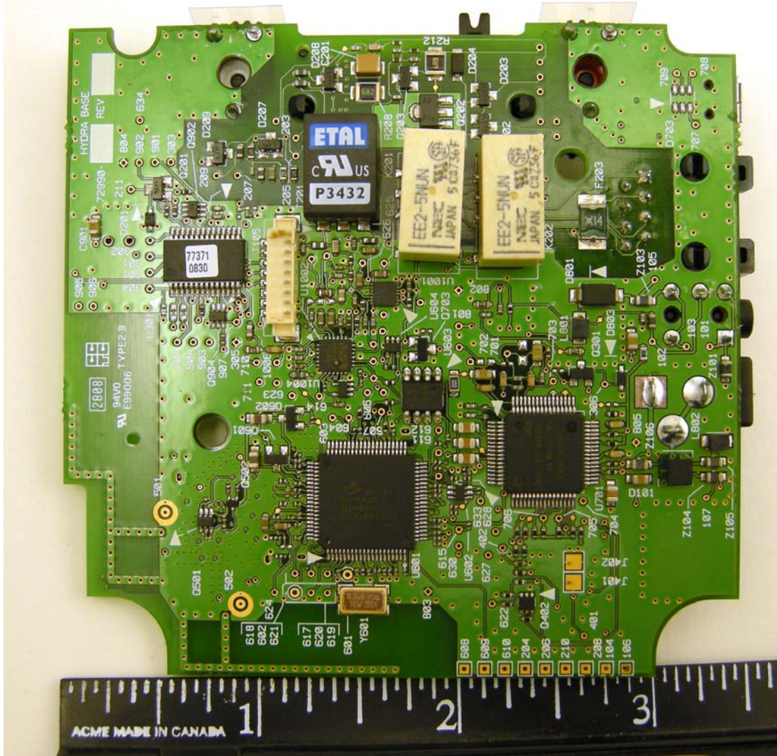
PCB Top
