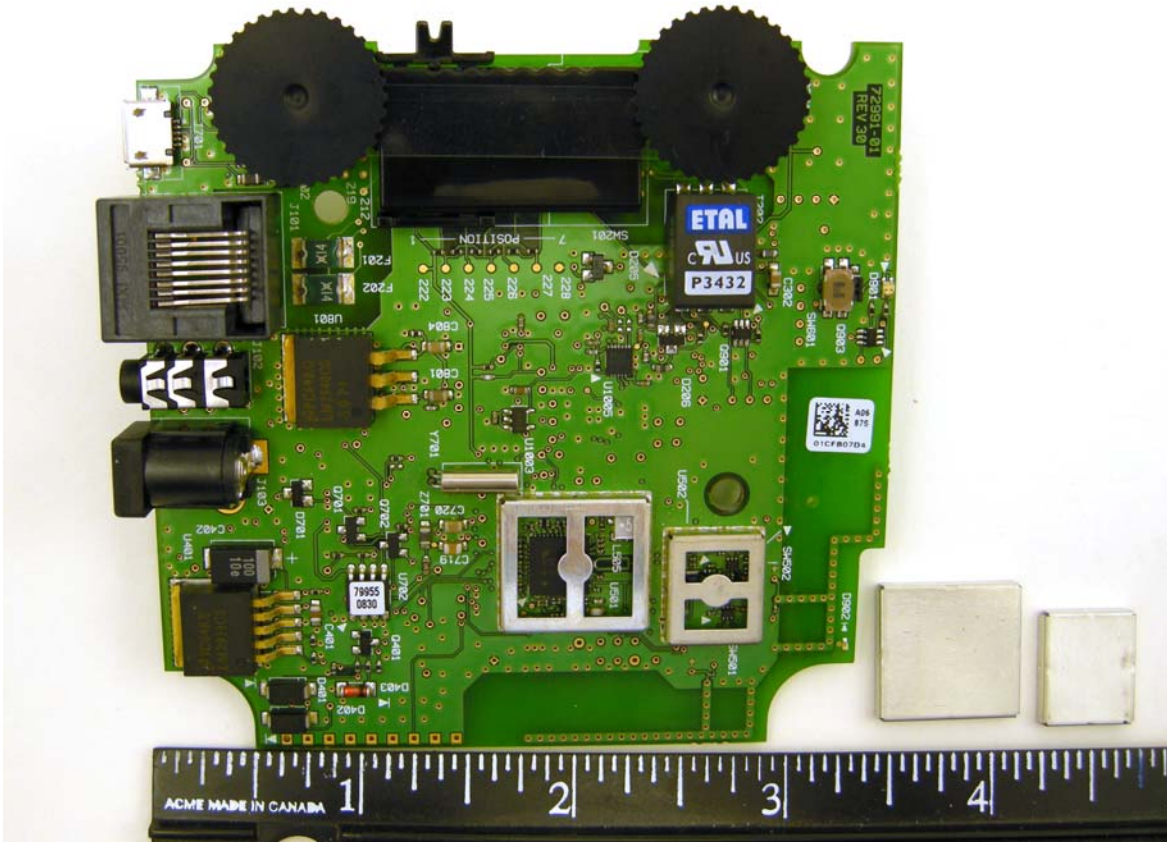
PCB Bottom
