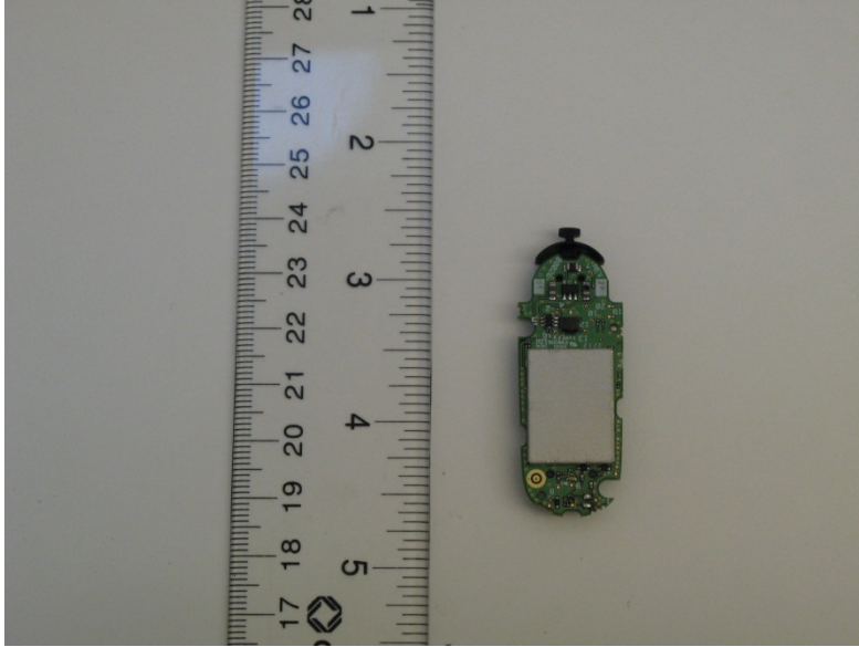
PCBA Top
