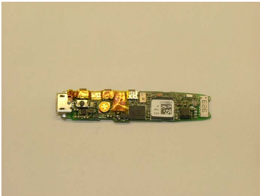
PCB Top
