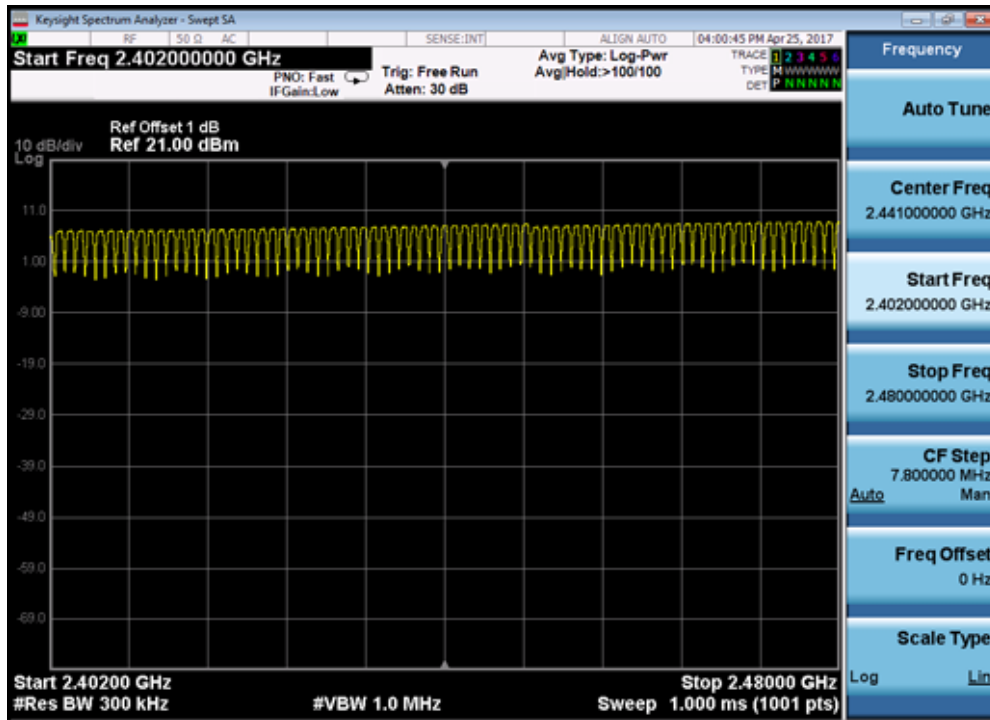
2402 - 2480MHz
