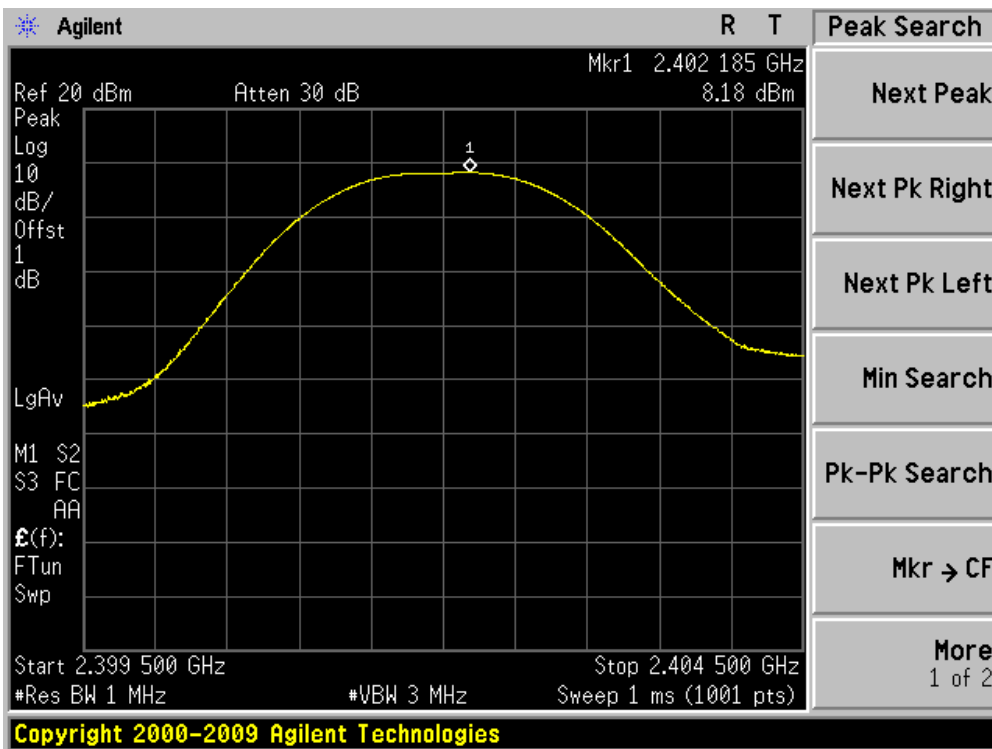
DH5 2402MHz
