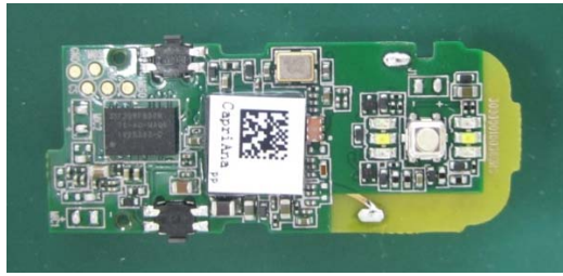
PCB Top
