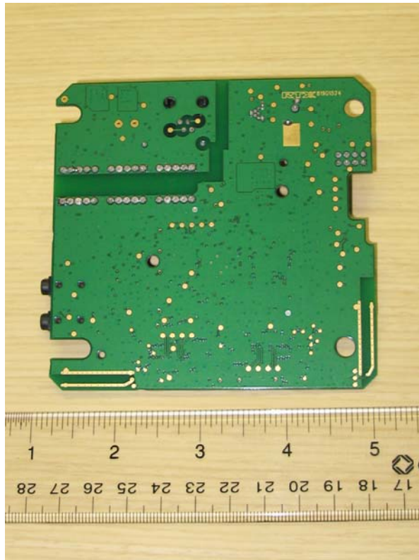
PCB Bottom
