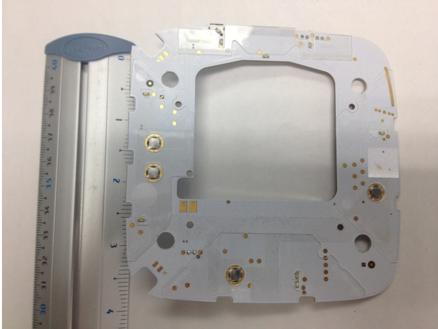
PCB Top
