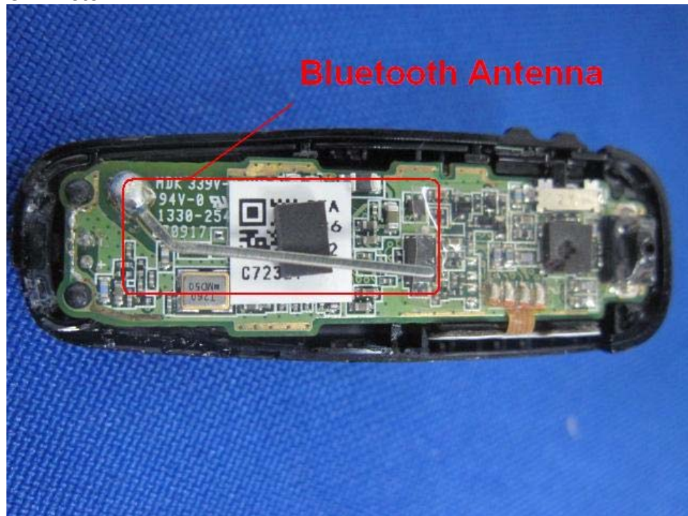
(2) EUT Photo
