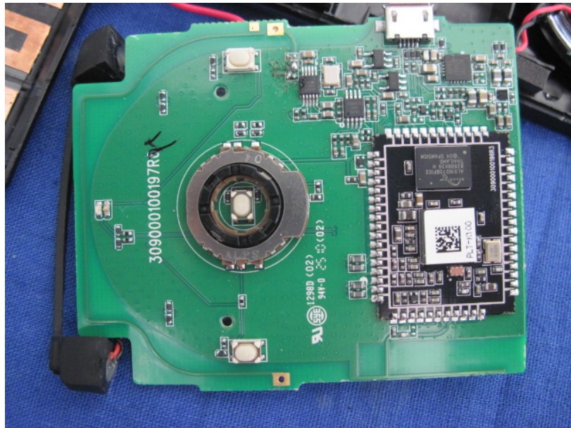
(3) EUT Photo
