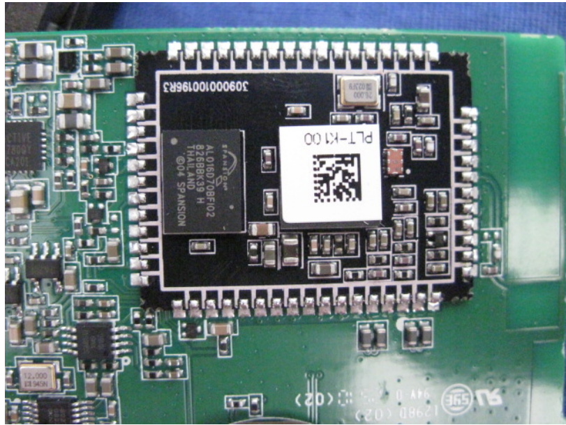
(4) EUT Photo
