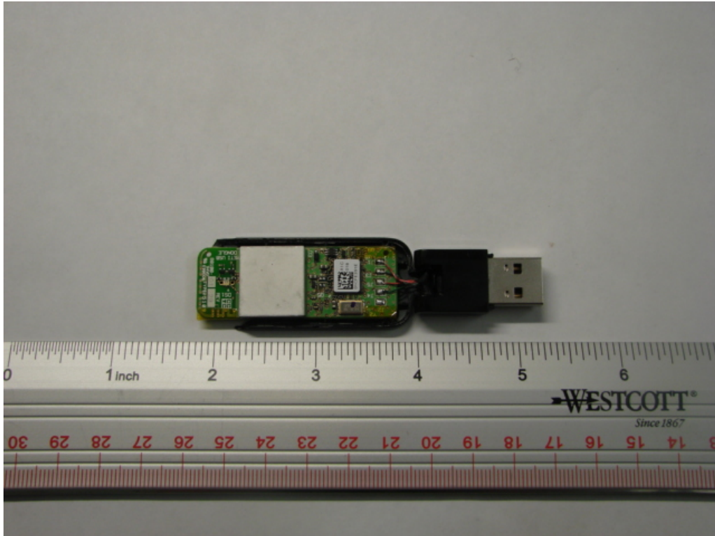
Top PCB
