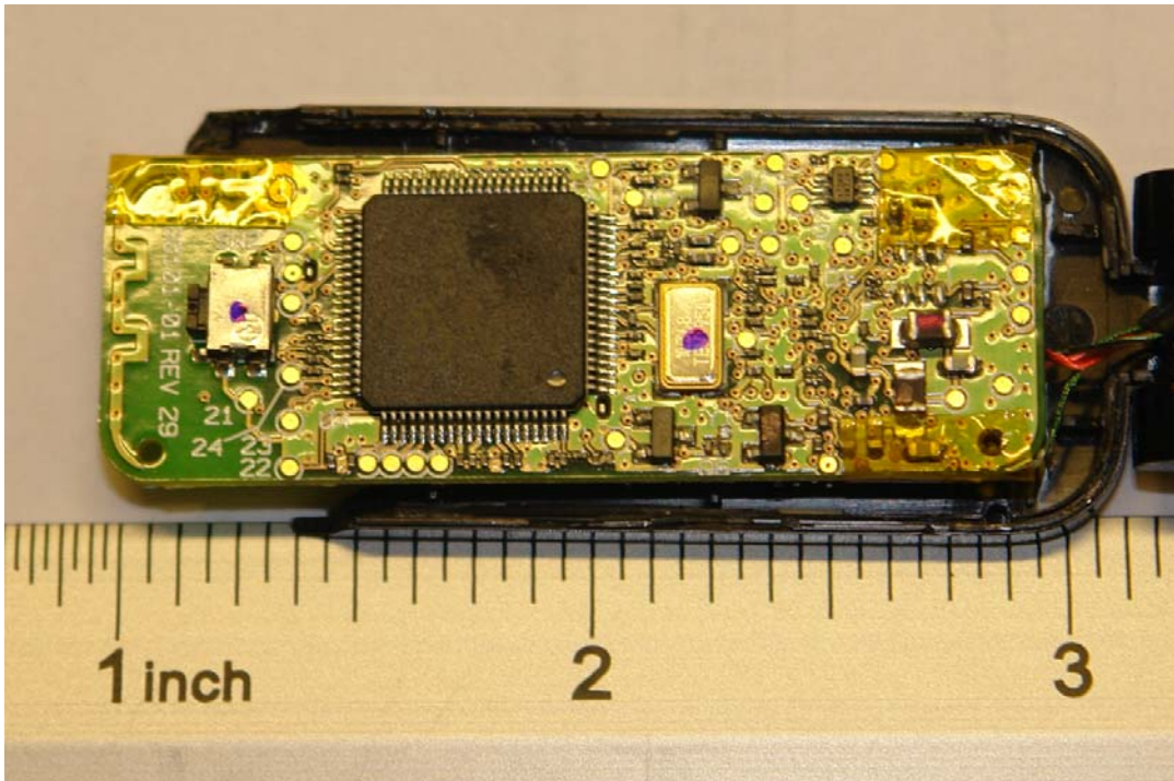
Bottom PCB
