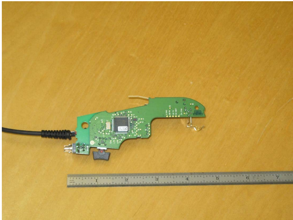
PCB Bottom
