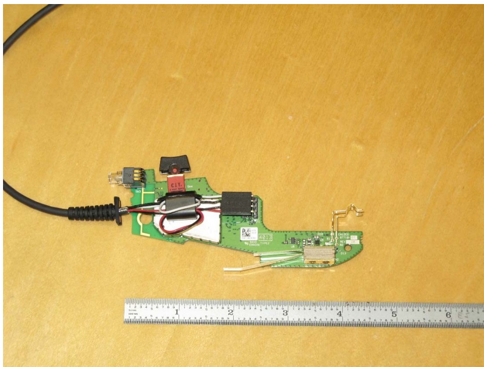
PCB Top
