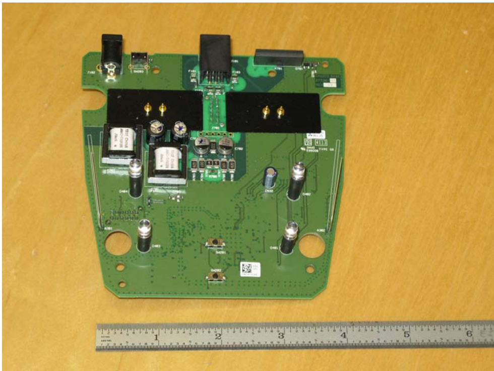
PCB Top
