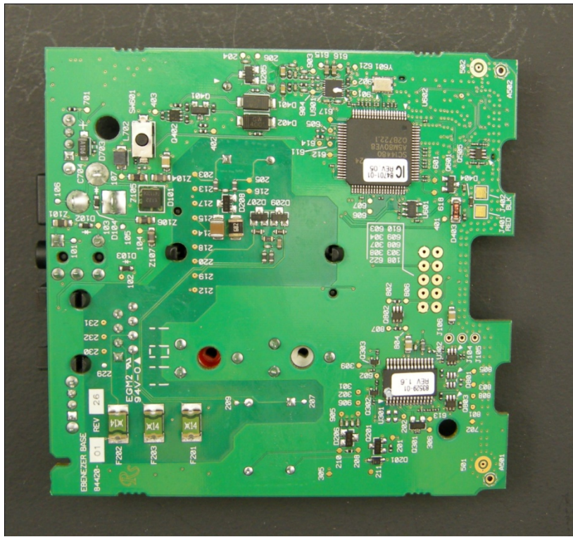
PCB TOP
