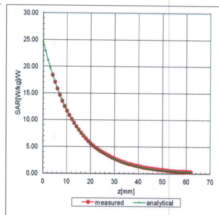
f=1750 MHz, WGLS R22(B_convF)
