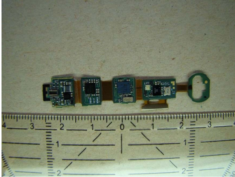
Right PCBA Top
