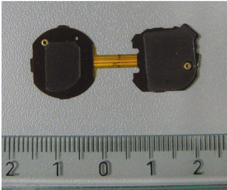
Left PCBA Bottom
