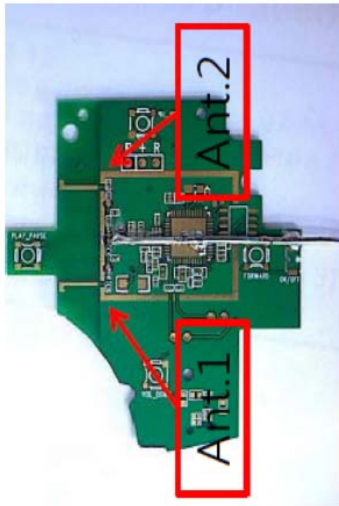
PCB BOTTOM
